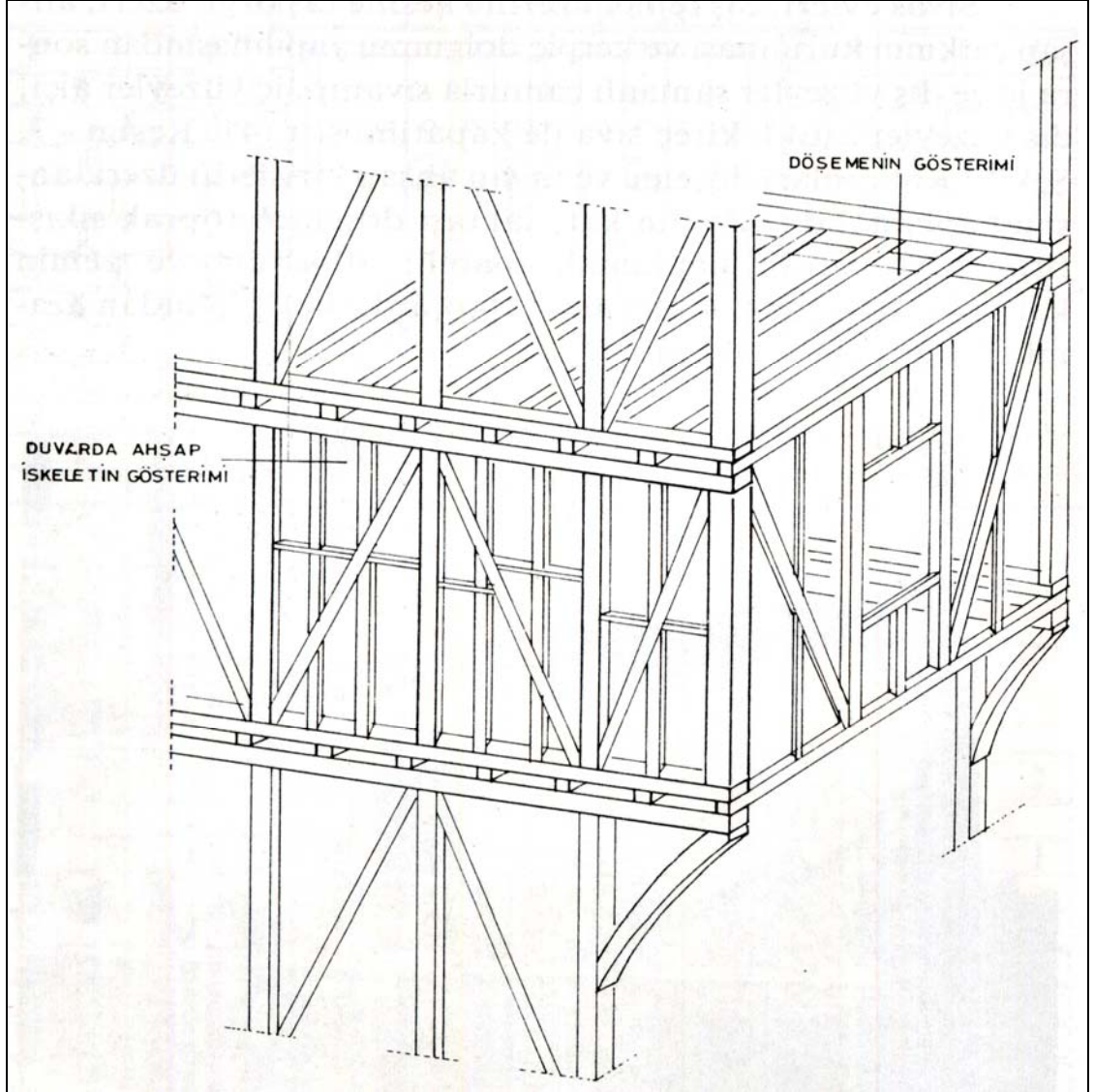
Şekil 4.55 Sivas evlerinin ahşap iskelet sistemi (Bilget 1993)
