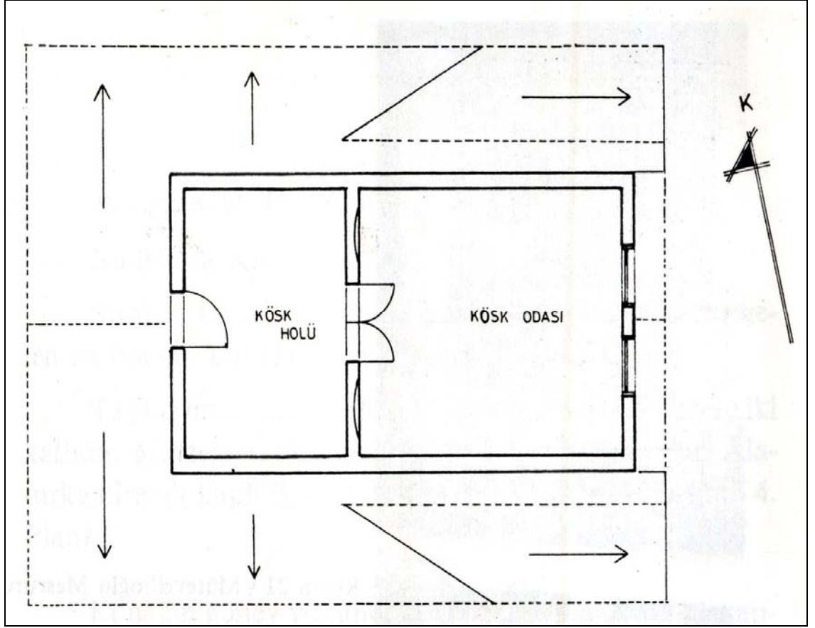
Şekil 4.48 Sivas, Mütevellioğlu Mesrur Bey evi köşk planı (Bilget 1993)
