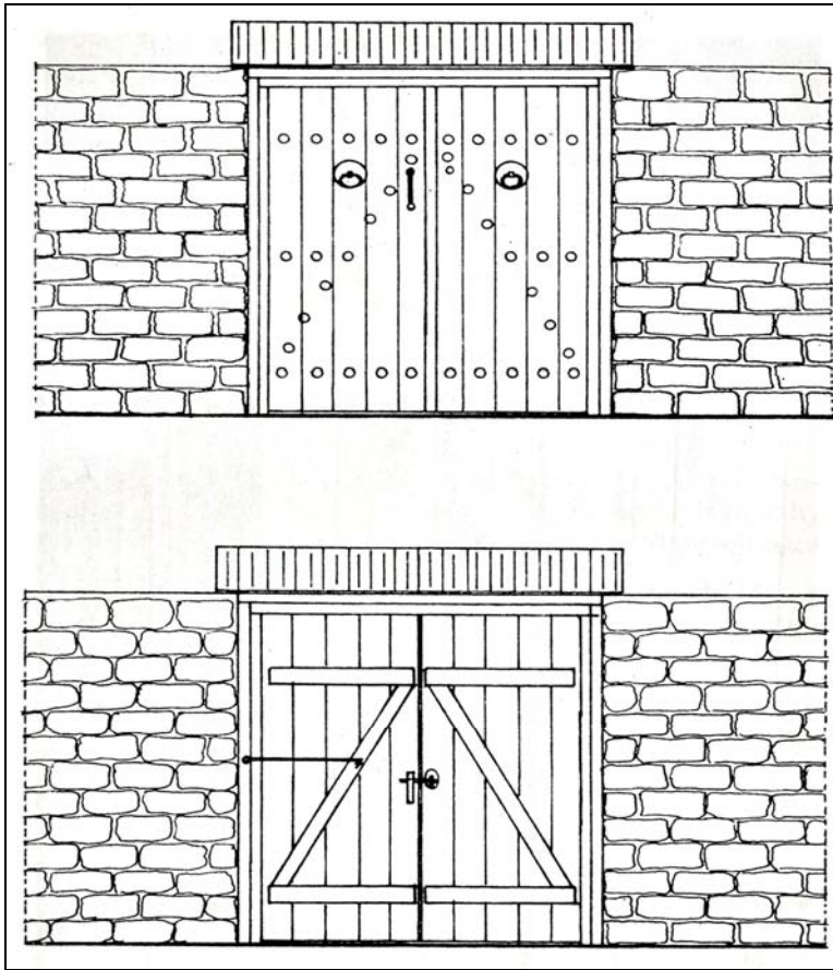
Şekil 4.44 Sivas evleri avlu giriş kapısı (Bilget 1993)
