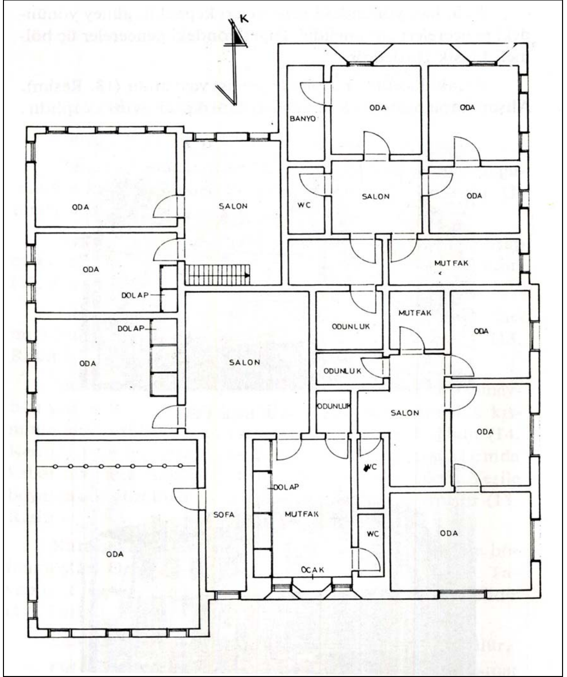
Şekil 4.51 Sivas, Abdi Başara evi birinci kat (Bilget 1993)
