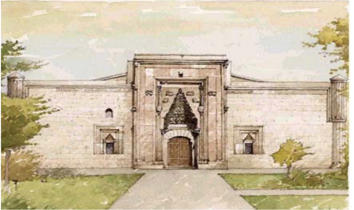
Şekil 5.15 Sivas, Buruciye Medresesi restorasyon sonrası durumu
