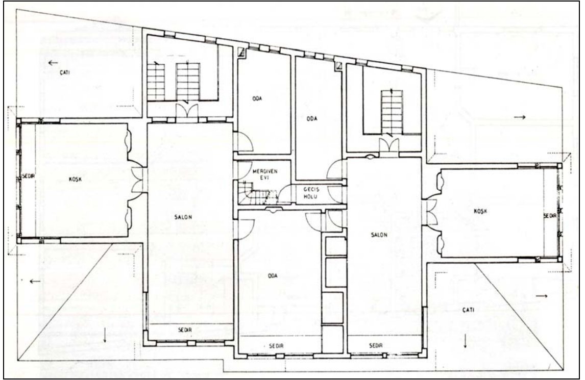
Şekil 4.50 Sivas, Feridun Kangal Konağı birinci kat planı (Bilget 1993)
