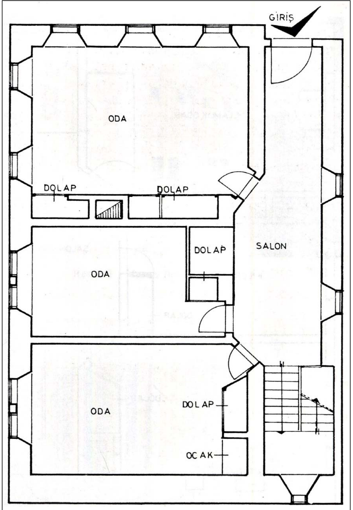
Şekil 4.45 Sivas, Hasan Başeğmez evi zemin kat planı (Bilget 1993)
