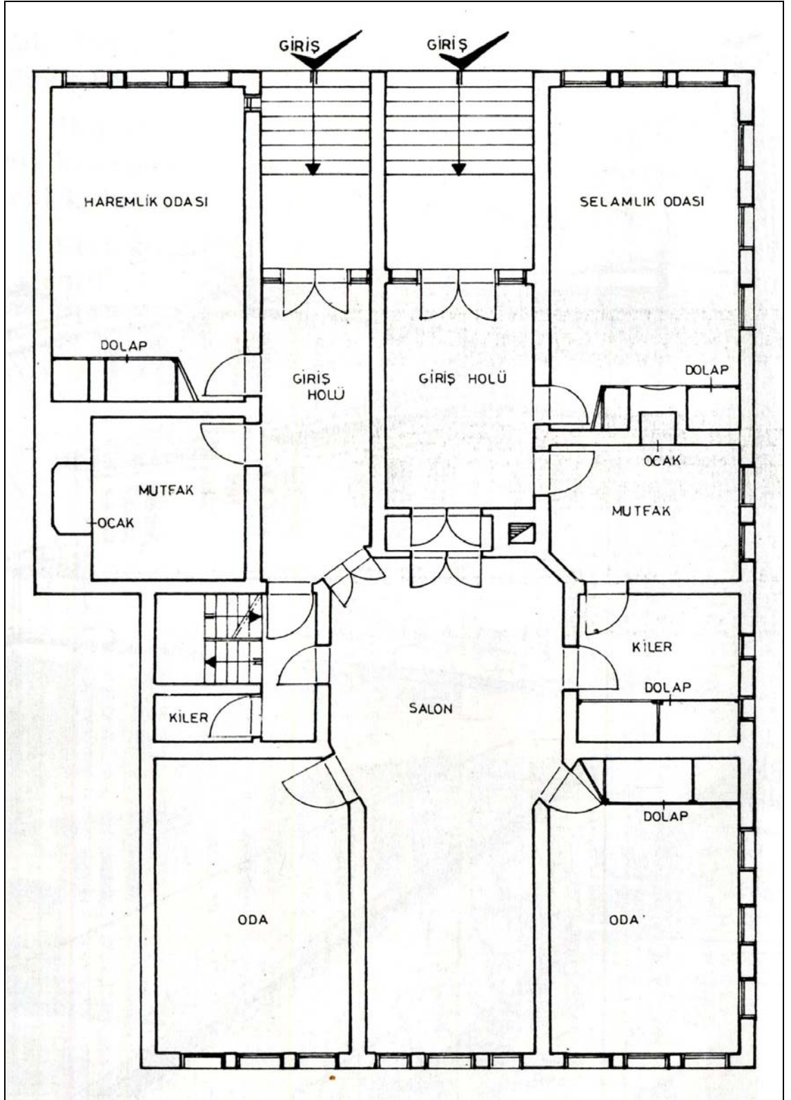
Şekil 4.47 Sivas, Mütevellioğlu Mesrur Bey evi zemin kat planı (Bilget 1993)
