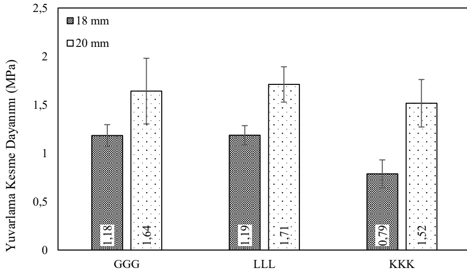
Şekil 4.11: ÇLK malzemelerin yuvarlanma kesme dayanımı.
