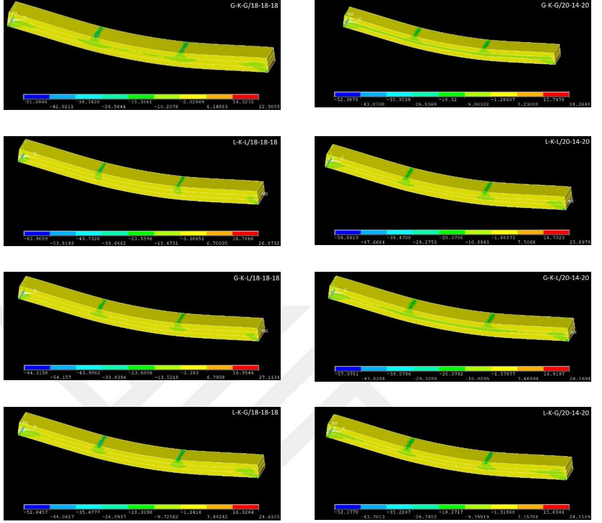
Şekil 4.25 (devamı): Sonlu elemanlar analizi sonuçları
