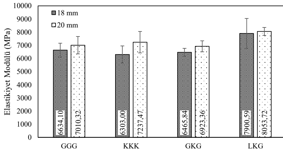
Şekil 4.6: Hibrit ÇLK malzemelerin elastikiyet modülünün göknar ve kavak odun türleri üzerinden değerlendirilmesi.
