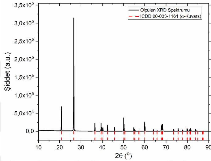
Şekil 4.1. Kuvars Mineraline Ait Ölçülen ve ICDD Referans XRD Desenleri
