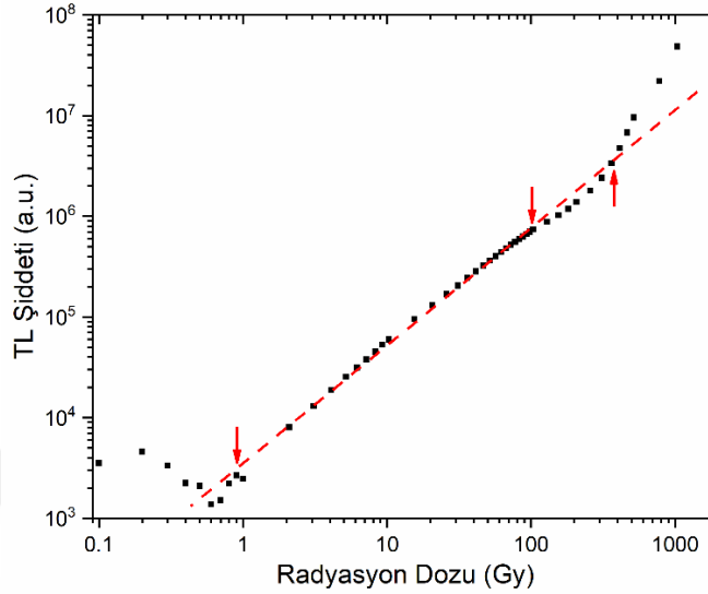
Şekil 4.10. 0,1–1034,9 Gy Doz Aralıklarında Işınlanmış Kuvars Örneklerine ait TL Işıma Eğrilerinin Altında Kalan Alanlardan Elde Edilen Doz–Yanıt Eğrisi
