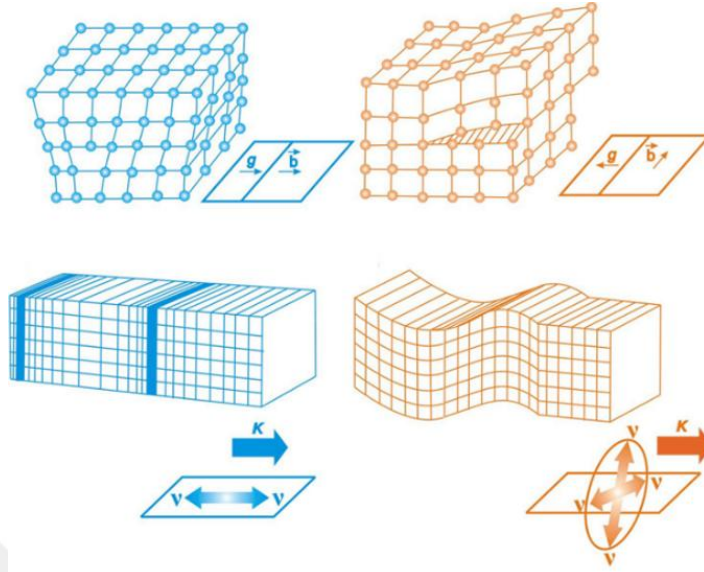
Şekil 3.5. Yüzeysel Kusurlar (Li ve Zhang, 2017)
