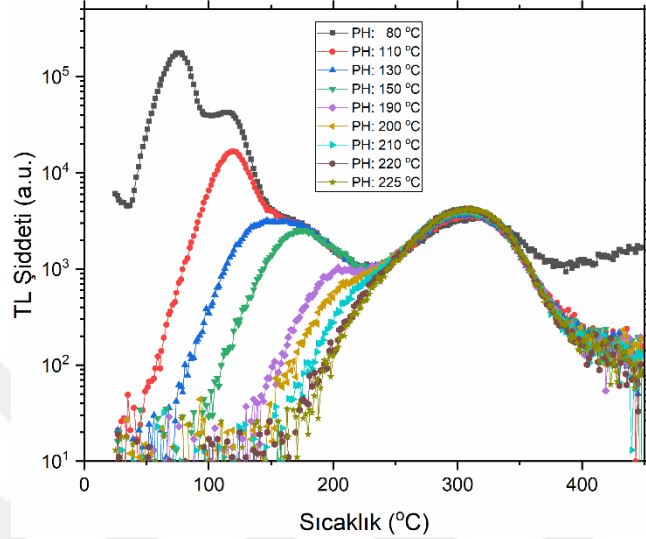
Şekil 4.4. Farklı Ön Isıtma Sıcaklıklarında Elde Edilen TL Işıma Eğrileri
