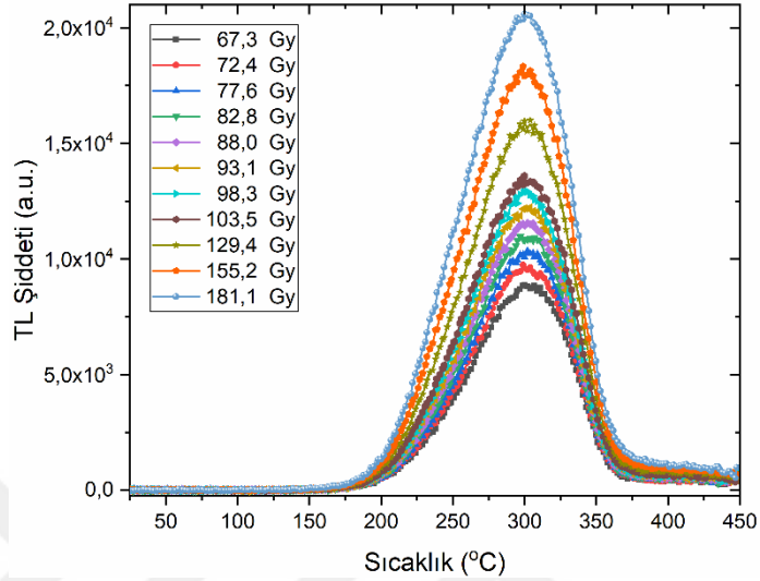
Şekil 4.8. 67,3–181,1 Gy Aralıklarındaki Farklı Dozlarda Elde Edilen TL Işıma Eğrileri
