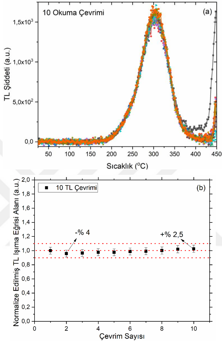
Şekil 4.12. Yeniden Kullanılabilirlik Deneyi ile Elde Edilen (a) TL Işıma Eğrileri ve (b) Ölçüm Tekrar Sayısına Karşılık Normalize Edilmiş TL Işıma Eğrisi Alanlarının Değişimleri
