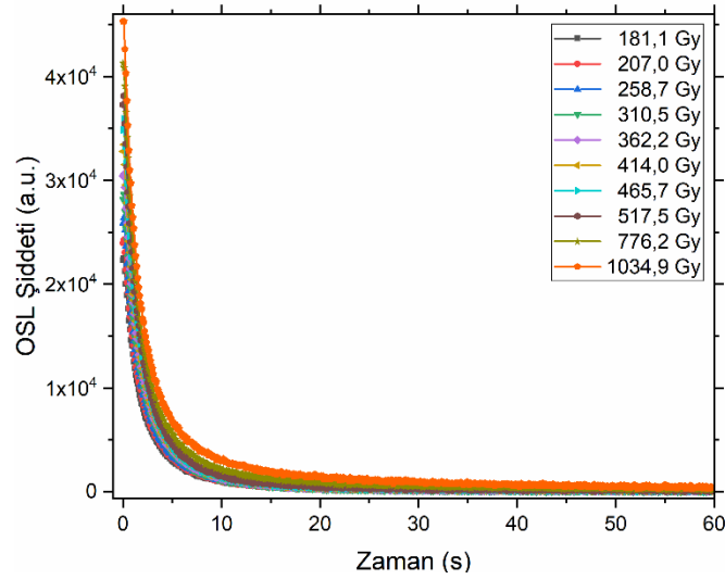
Şekil 4.22. 181,1–1034,9 Gy Aralıklarındaki Farklı Dozlarda Elde Edilen OSL Bozunum Eğrileri
