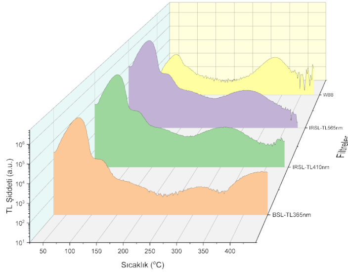
Şekil 4.3. Farklı Filtre Kombinasyonlarındaki TL Işıma Eğrileri
