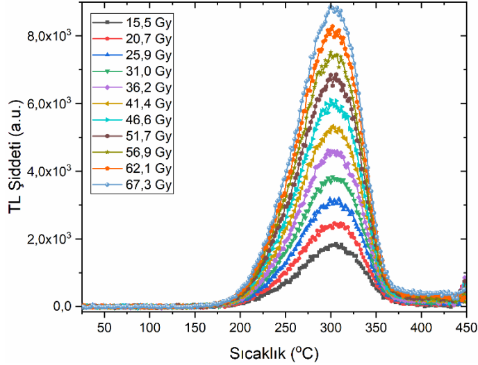
Şekil 4.7. 15,5–67,3 Gy Aralıklarındaki Farklı Dozlarda Elde Edilen TL Işıma Eğrileri
