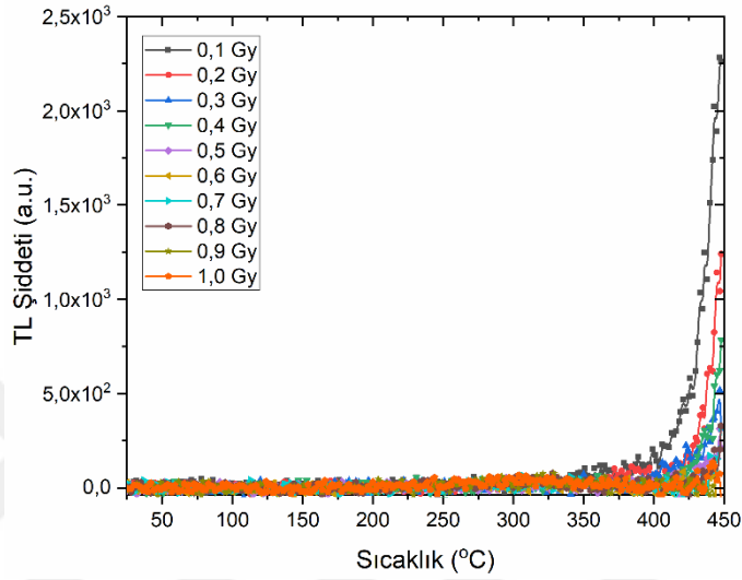
Şekil 4.5. 0,1–1 Gy Aralıklarındaki Farklı Dozlarda Elde Edilen TL Işıma Eğrileri
