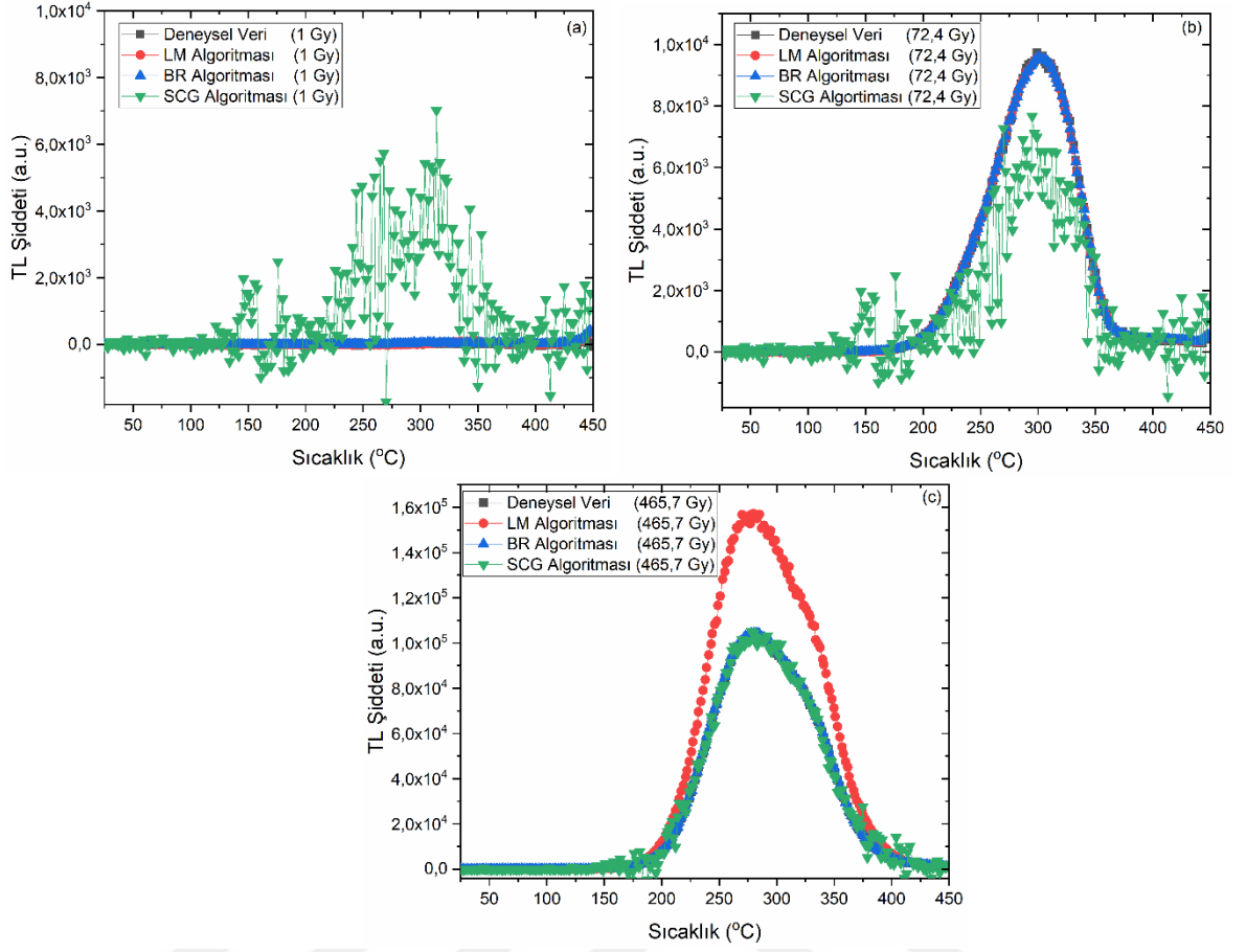
Şekil 4.17. (a) 1 Gy, (b) 72,4 Gy ve (c) 465,7 Gy Radyasyon Dozları için Deneysel, LM, BR ve SCG Algoritmaları ile Elde Edilen TL Işıma Eğrilerinin Karşılaştırması
