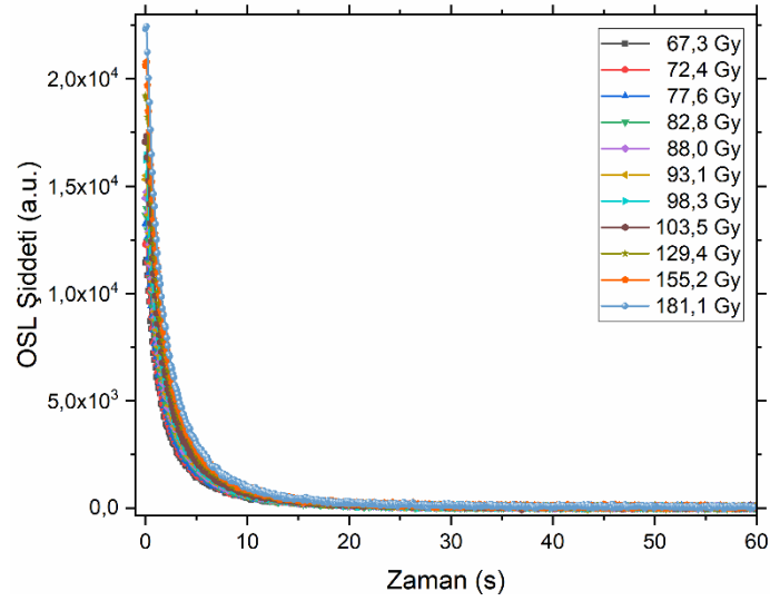
Şekil 4.21. 67,3–181,1 Gy Aralıklarındaki Farklı Dozlarda Elde Edilen OSL Bozunum Eğrileri
