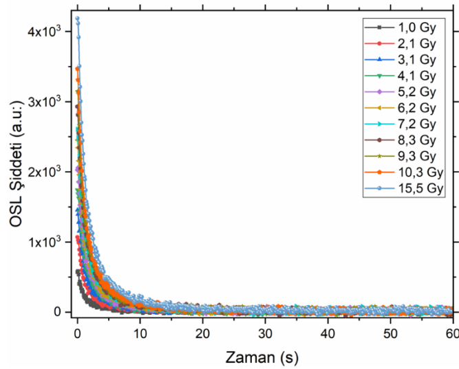
Şekil 4.19. 1–15,5 Gy Aralıklarındaki Farklı Dozlarda Elde Edilen OSL Bozunum Eğrileri
