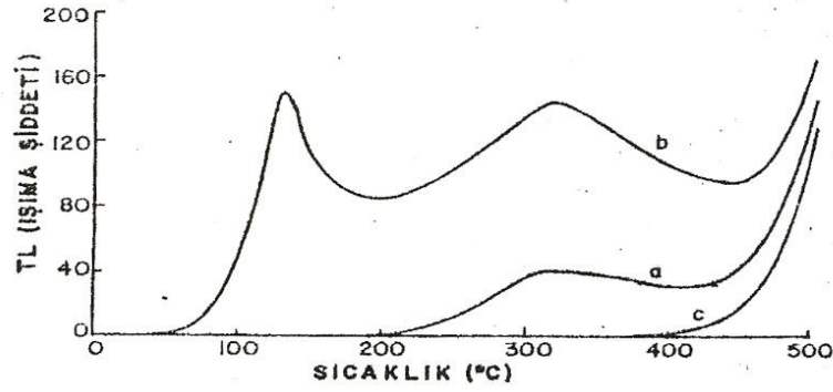
Şekil 3.8. Bir Seramik Parçasının Işıma Eğrileri (Aitken, 1985); a) Doğal Işıma Eğrisi, b) Doğal + Laboratuvar Dozu Almış Örneğin Işıma Eğrisi, c) Kara Cisim Işıması
