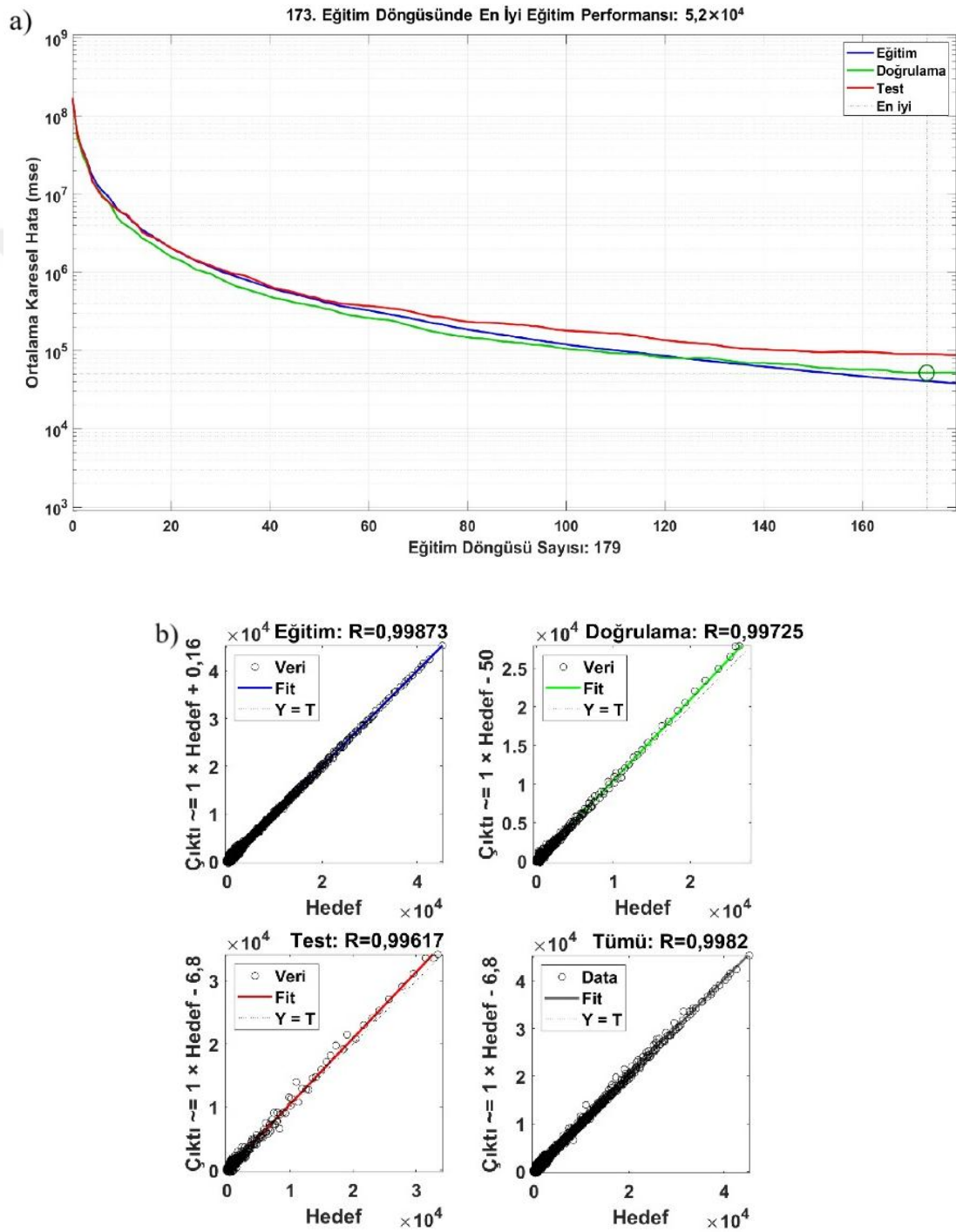
Şekil 4.28. SCG Algoritması için YSA Simülasyon Sonuçları: (a) Performans Doğrulaması, (b) Hedef ve Çıktı Arasındaki Doğrusal Regresyon Analizi
