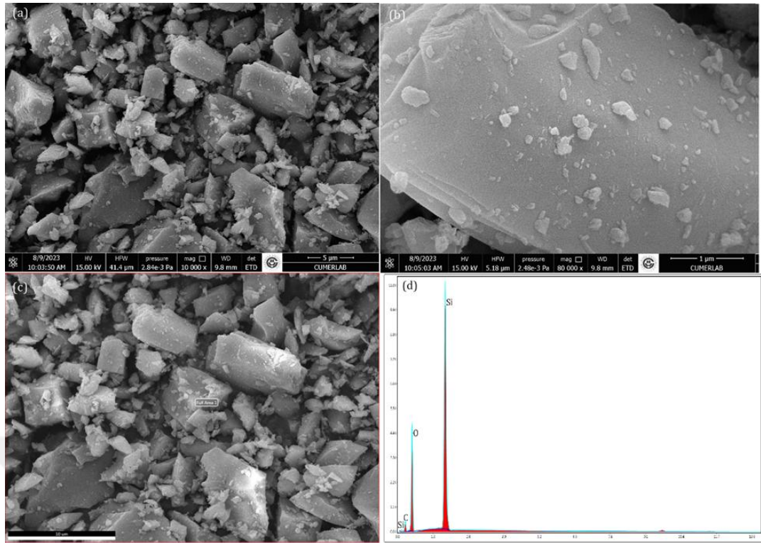
Şekil 4.2. (a) 10 kx ve (b) 80 kx Büyütme Oranlarında Elde Edilen SEM Görüntüleri, (c) EDS Analizi İçin Taranan Alan ve (d) EDS Spektrumu
