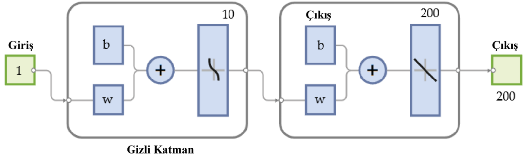
Şekil 4.25. OSL Bozunum Eğrisi Tahminleri için Oluşturulan YSA Modeline ait Yapısal Tasarım
