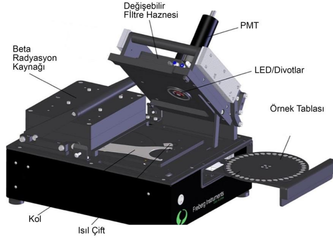
Şekil 3.3. Lexsyg Smart TL/OSL Okuyucun Temel Parçaları (Richter ve ark., 2015)
