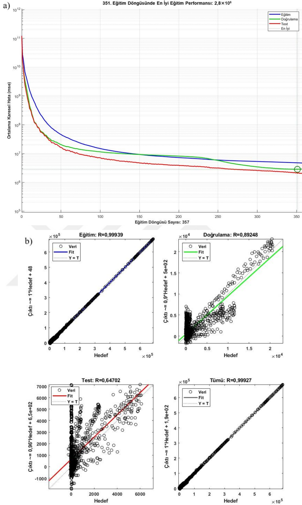
Şekil 4.16. SCG Algoritması için YSA Simülasyon Sonuçları: (a) Performans Doğrulaması, (b) Hedef ve Çıktı Arasındaki Doğrusal Regresyon Analizi
