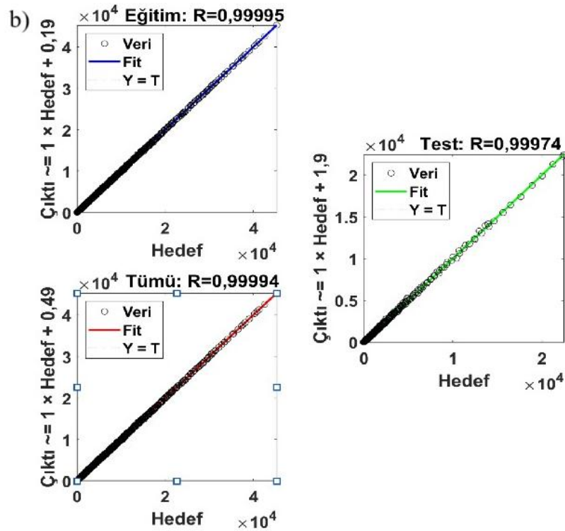
Şekil 4.27. BR Algoritması için YSA Simülasyon Sonuçları: (a) Performans Doğrulaması, (b) Hedef ve Çıktı Arasındaki Doğrusal Regresyon Analizi
