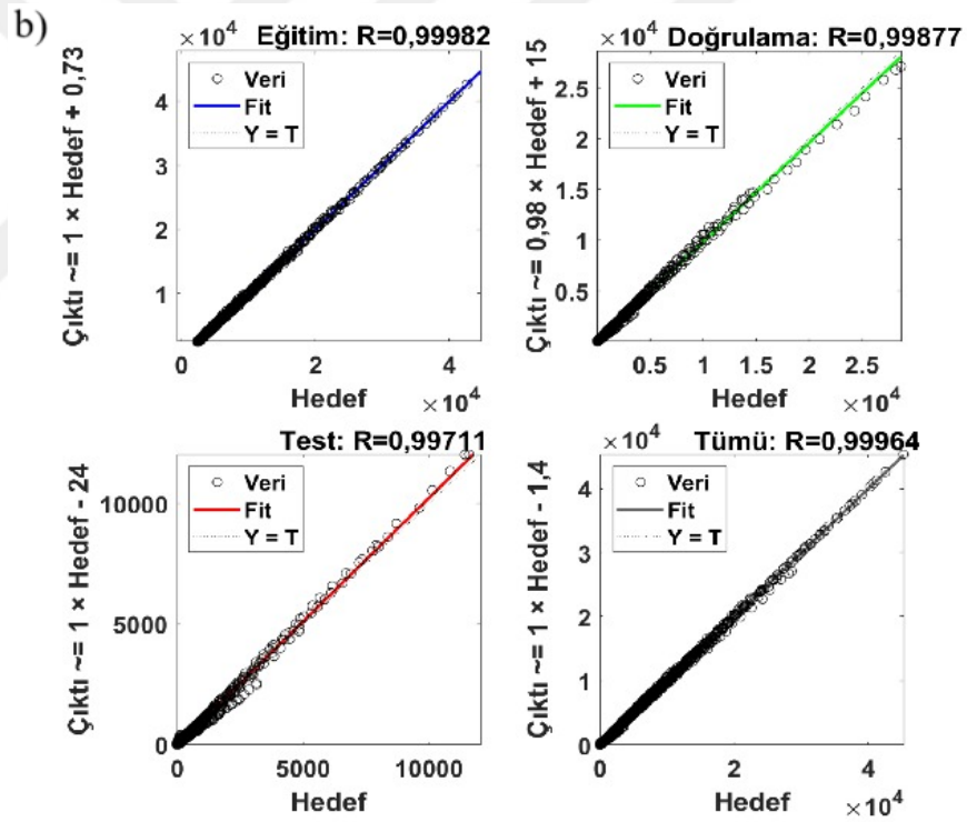
Şekil 4.26. LM Algoritması için YSA Simülasyon Sonuçları: (a) Performans Doğrulaması, (b) Hedef ve Çıktı Arasındaki Doğrusal Regresyon Analizi
