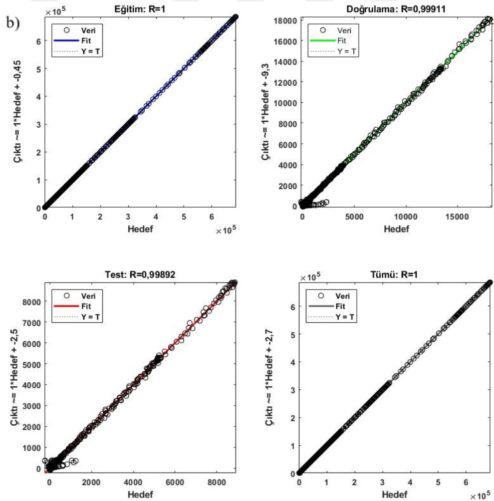
Şekil 4.14. LM Algoritması için YSA Simülasyon Sonuçları: (a) Performans Doğrulaması, (b) Hedef ve Çıktı Arasındaki Doğrusal Regresyon Analizi
