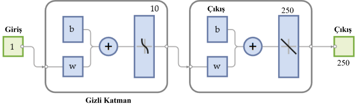
Şekil 4.13. TL Işma Eğrisi Tahminleri için Oluşturulan YSA Modeline ait Yapısal Tasarım
