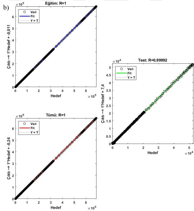
Şekil 4.15. BR Algoritması için YSA Simülasyon Sonuçları: (a) Performans Doğrulaması, (b) Hedef ve Çıktı Arasındaki Doğrusal Regresyon Analizi
