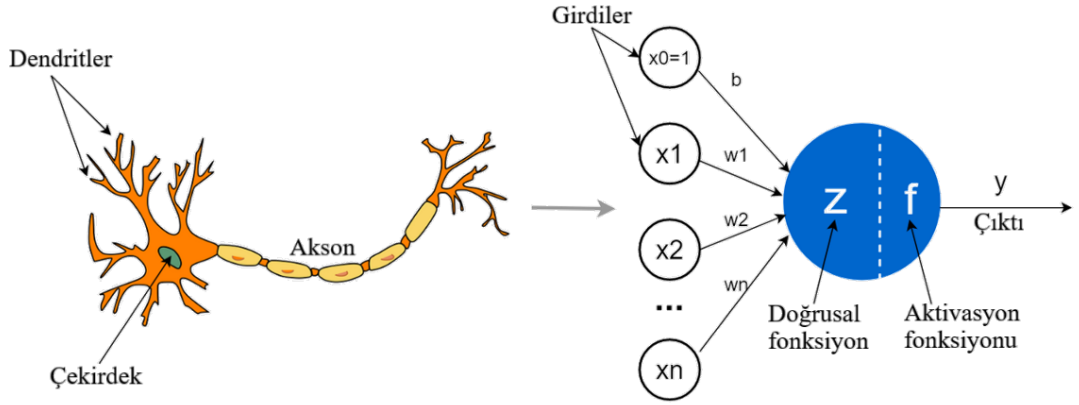
Şekil 3.10. Biyolojik Nöronlar ve Yapay Sinir Ağları (YSA) Modeli (Shah, 2020)
