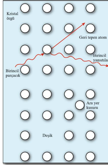
Şekil 3.6. Hacimsel Kristal Kusurları (Maurer ve ark.,2008)
