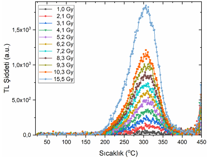
Şekil 4.6. 1–15,5 Gy Aralıklarındaki Farklı Dozlarda Elde Edilen TL Işıma Eğrileri
