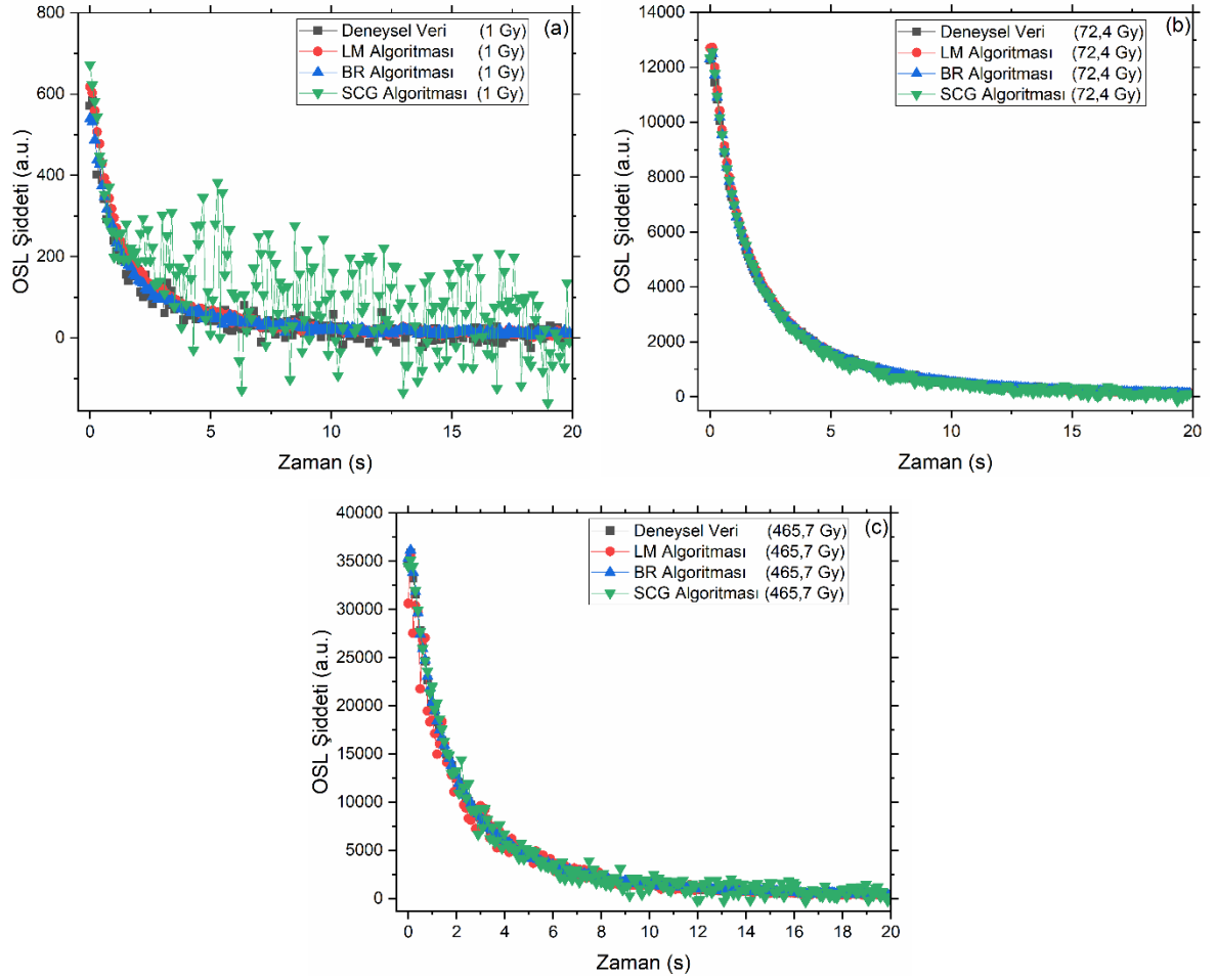
Şekil 4.29. (a) 1 Gy, (b) 72,4 Gy ve (c) 465,7 Gy Radyasyon Dozları için Deneyssel, LM, BR ve SCG Algoritmaları ile Elde Edilen OSL Bozunum Eğrilerinin Karşılaştırması
