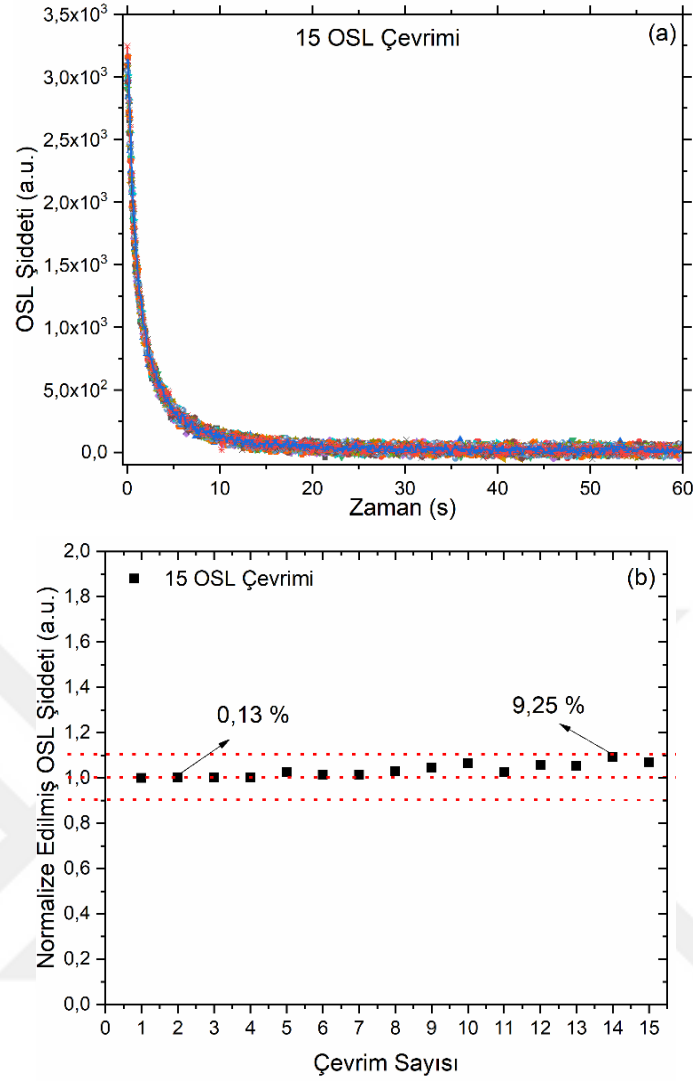
Şekil 4.24. 15 Tekrarlı Ölçüm Döngüsüne ( D = 10 Gy) ait Kuvars Örneklerinin (a) OSL Bozunum Eğrileri ve (b) Yeniden Kullanılabilirliği
