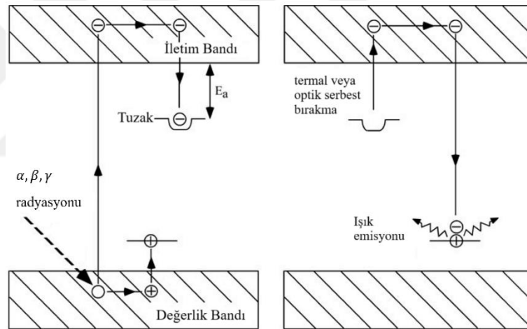
Şekil 3.7. Tuzaklanmış Elektronların Boşalması (Aitken, 1985)
