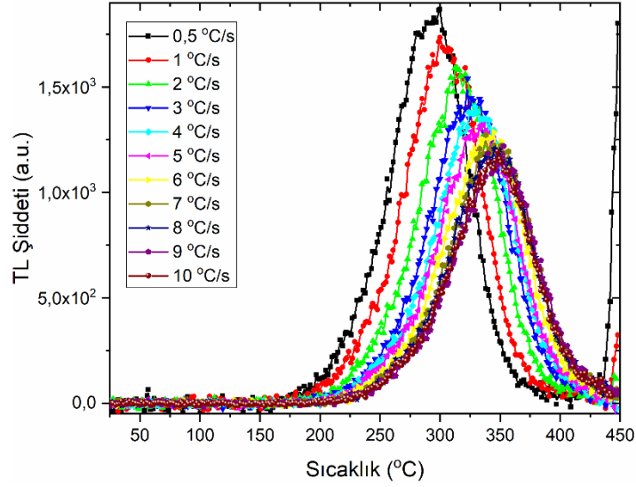
Şekil 4.11. Farklı Isıtma Hızlarında Elde Edilen TL Işıma Eğrileri
