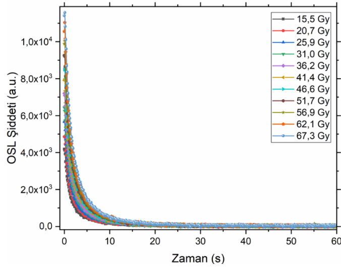
Şekil 4.20. 15,5–67,3 Gy Aralıklarındaki Farklı Dozlarda Elde Edilen OSL Bozunum Eğrileri
