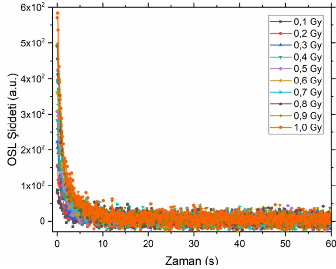
Şekil 4.18. 0,1–1 Gy Aralıklarındaki Farklı Dozlarda Elde Edilen OSL Bozunum Eğrileri
