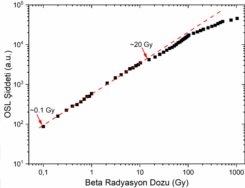
Şekil 4.23. Kuvarsın Beta Radyasyonu Altında Başlangıç OSL Sinyaline ait Doz–Yanıt Eğrisi
