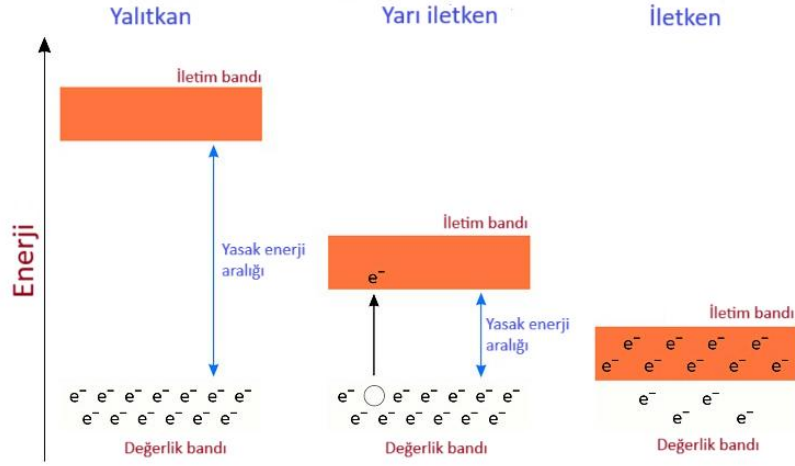
Şekil 3.4. Katılarda Bant Modeli (ScienceFacts.net, 2023 Kasım)
