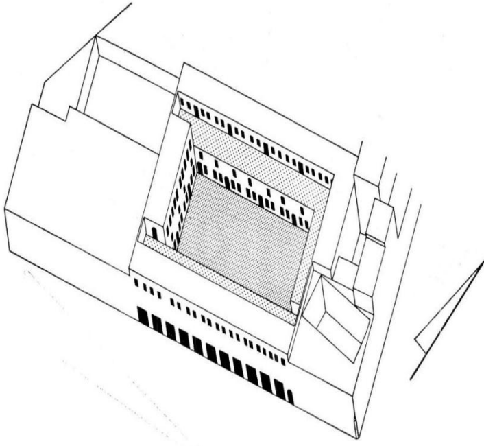
(Kayseriyyenin Aksonometri Görünümü) 274
