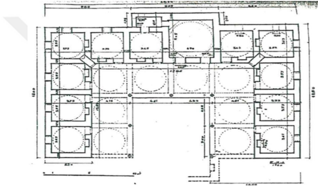
Şekil 4: Süleyman Paşa Medresesi planı (Ildız, 2006)
