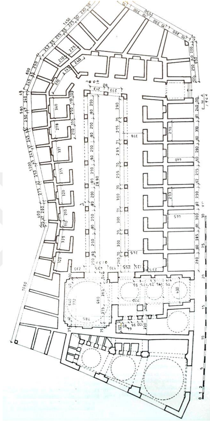
Şekil 16: Vaiziye (Mahkeme) Medresesi'nin planı (Vakıf Genel Müdürlüğü, 2024)
