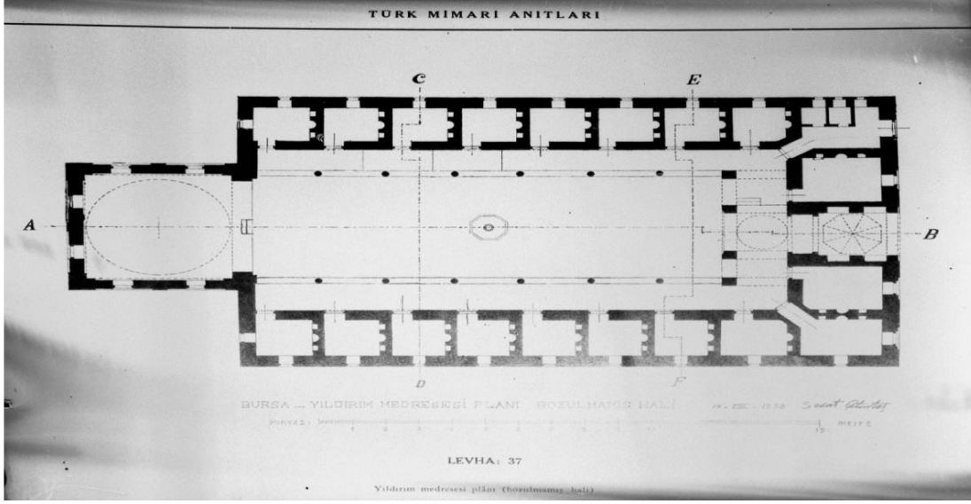
Şekil 14: Yıldırım Medresesi'nin planı (İldız, 2006)
