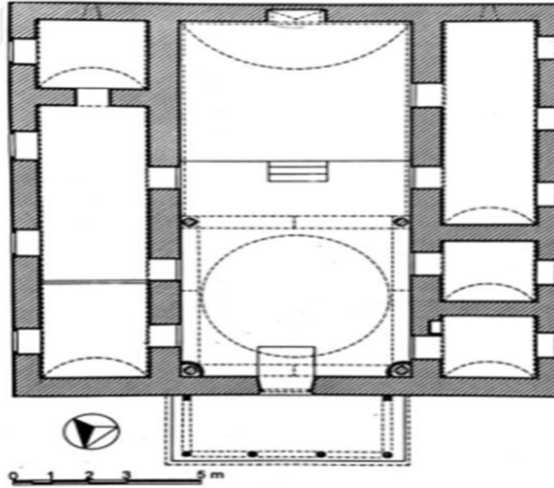
Şekil 10: Lala Şahin Paşa Medresesi günümüz planı (Demiralp, 1999)
