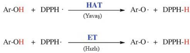
Şekil 4.2. DPPH reaksiyonunun mekanizması
