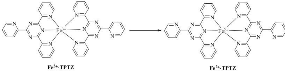
Şekil 4.5. FRAP testinde demirin indirgenmesi
