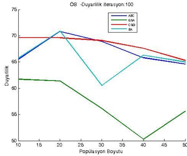
Şekil 1.61. DRD veri kümesi üzerinde 100 iterasyon için ortalama duyarlılık sonuçları
