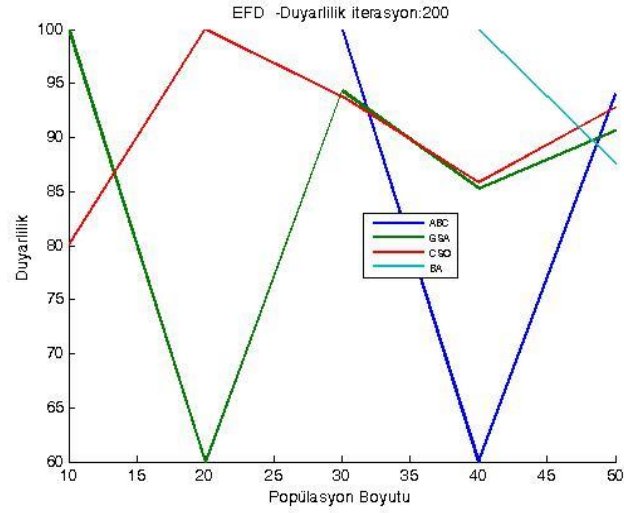
Şekil 3.62. DRD veri kümesi üzerinde 200 iterasyon için ortalama duyarlılık sonuçları
