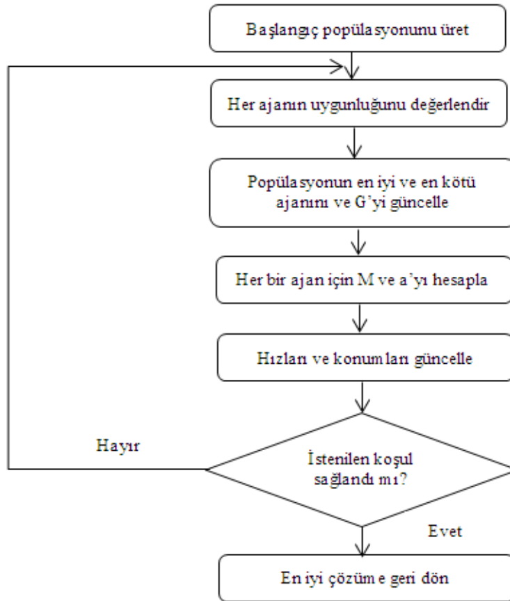
Şekil 3.2. GSA'nın akış diyagramı
