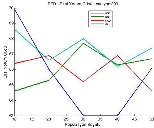
Şekil 3.54. QSAR veri kümesi üzerinde 300 iterasyon için ortalama eksi yorum gücü sonuçları
