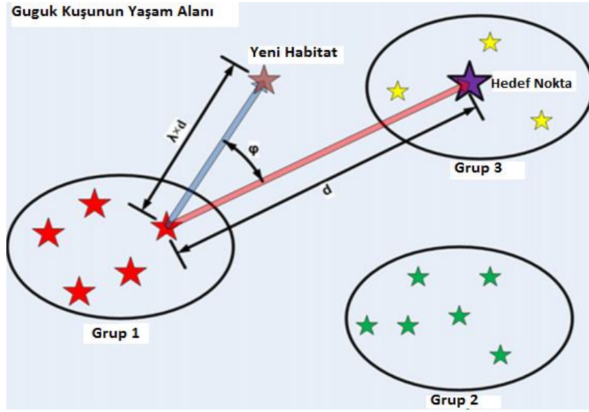
Şekil 3.5. Hedef noktaya doğru göç eden bir guguk kuşu örneği
