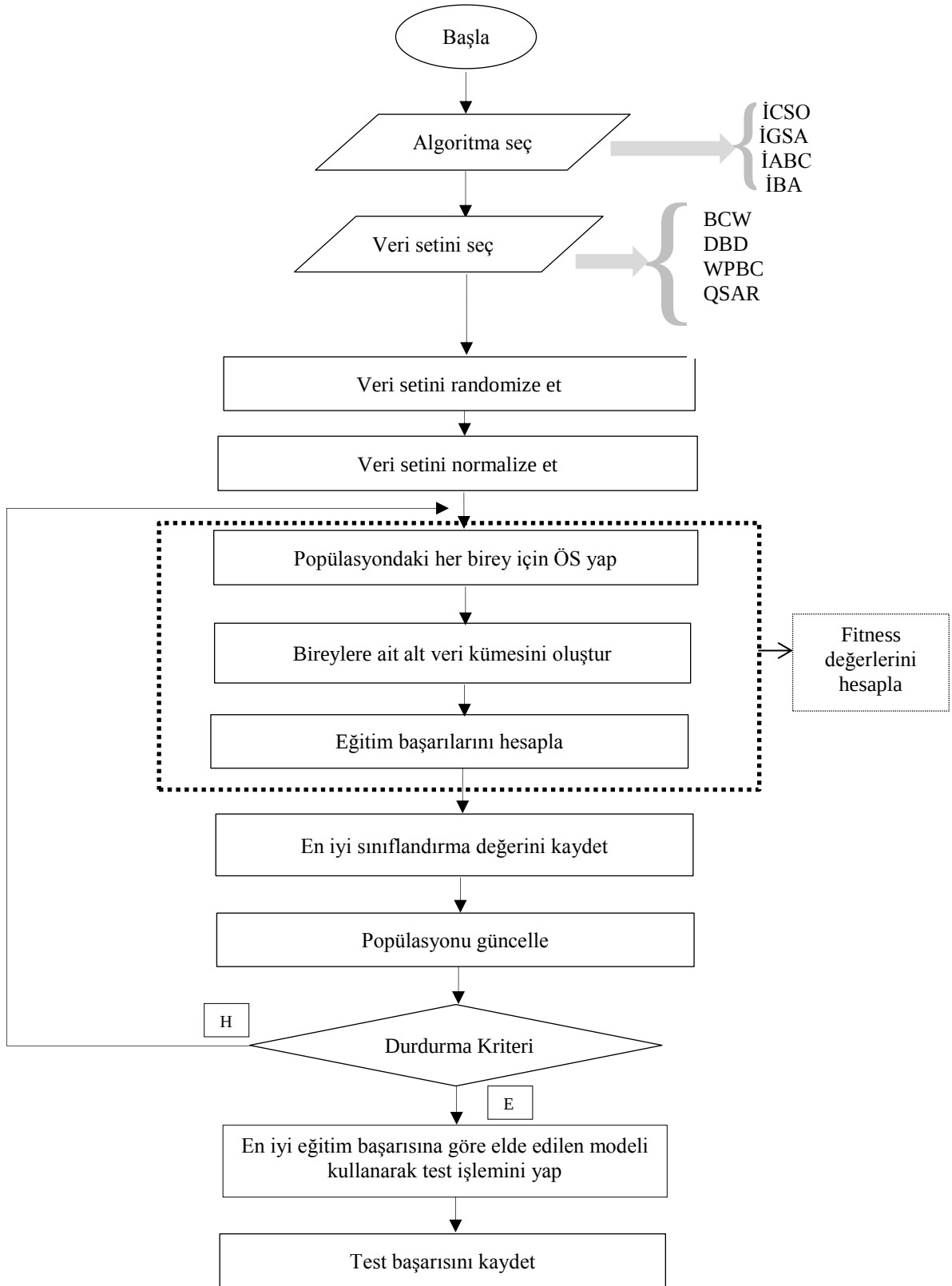
Çizelge 5.1. Önerilen ÖS sisteminin akış diyagramı
