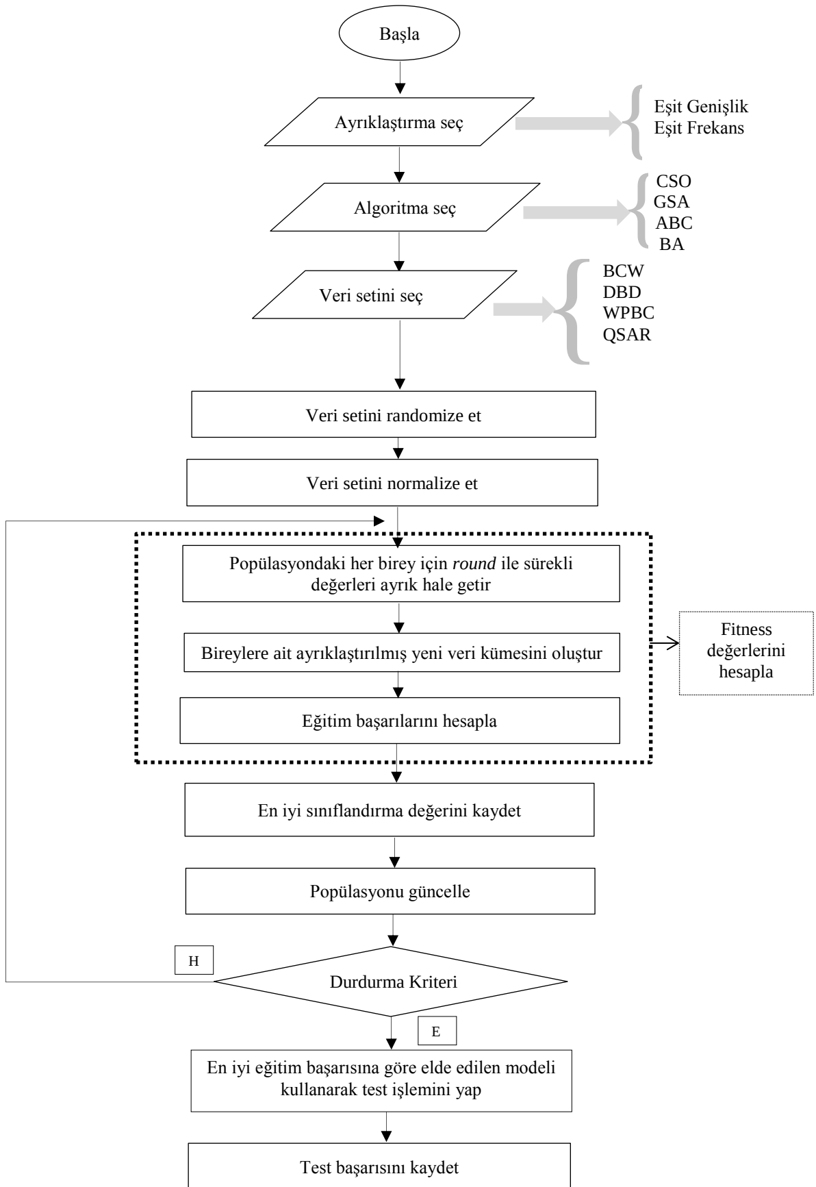
Çizelge 6.2. Önerilen Ayırıklaştırma sisteminin akış diyagramı
