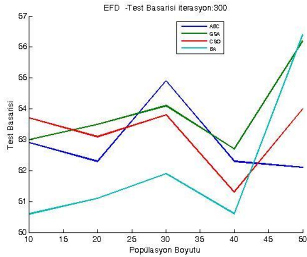
Şekil 3.60. DRD veri kümesi üzerinde 300 iterasyon için ortalama test başarıları
