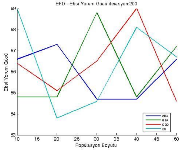
Şekil 3.53. QSAR veri kümesi üzerinde 200 iterasyon için ortalama eksi yorum gücü sonuçları
