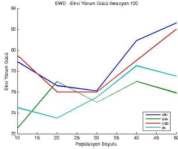
Şekil 2.16. WPBC veri kümesi üzerinde 100 iterasyon için ortalama eksi yorum gücü sonuçları
