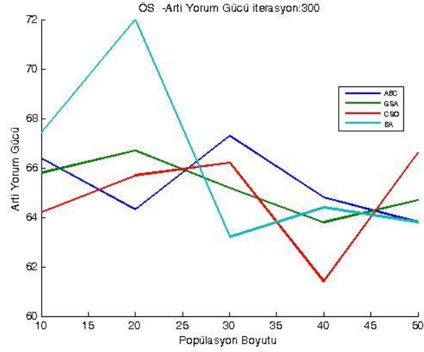
Şekil 1.69. DRD veri kümesi üzerinde 300 iterasyon için ortalama artı yorum gücü sonuçları
