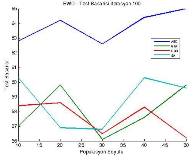
Şekil 2.58. DRD veri kümesi üzerinde 100 iterasyon için ortalama test başarıları
