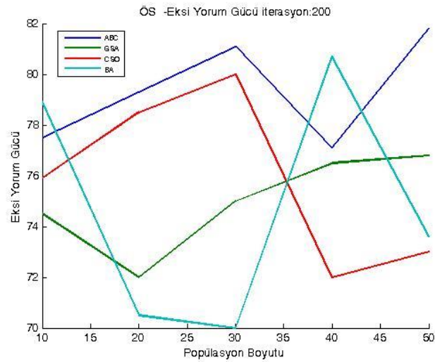
Şekil 1.17. WPBC veri kümesi üzerinde 200 iterasyon için ortalama eksi yorum gücü sonuçları
