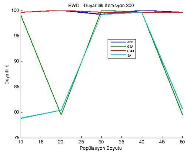
Şekil 2.27. BCW veri kümesi üzerinde 300 iterasyon için ortalama duyarlılık sonuçları
