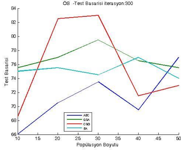
Şekil 1.6. WPBC veri kümesi üzerinde 300 iterasyon için ortalama test başarıları
