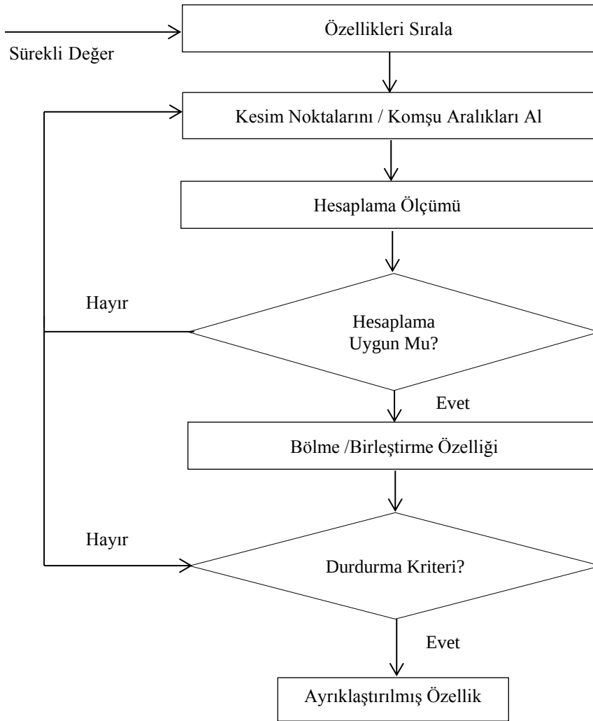
Çizelge 6.1. Ayırıklaştırma İşlemi
