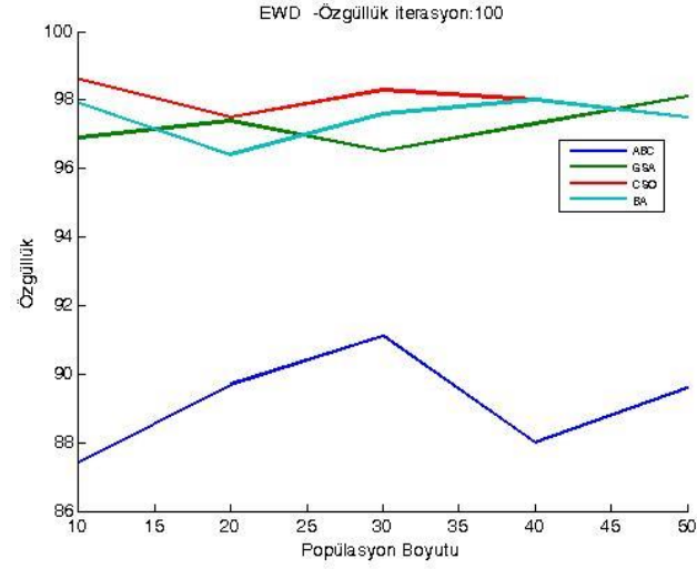
Şekil 2.46. QSAR veri kümesi üzerinde 100 iterasyon için ortalama özgüllük sonuçları
