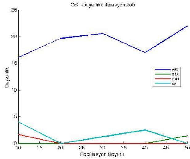
Şekil 1.8. WPBC veri kümesi üzerinde 200 iterasyon için ortalama duyarlılık sonuçları
