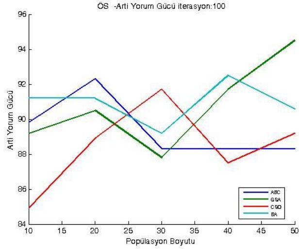
Şekil 1.31. BCW veri kümesi üzerinde 100 iterasyon için artı yorum gücü sonuçları
