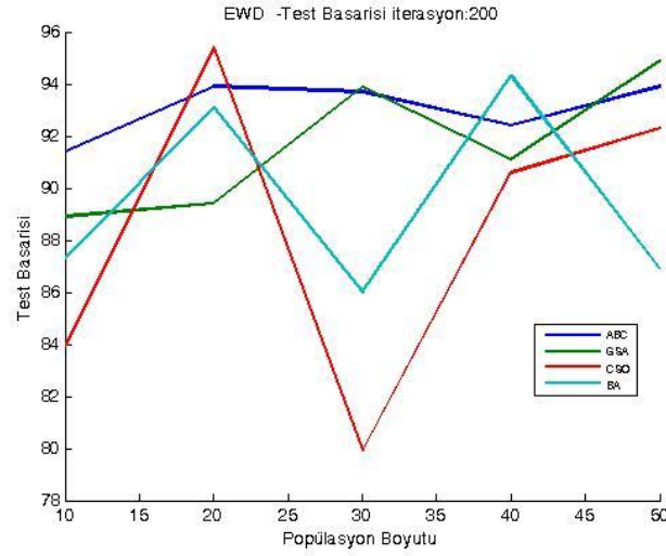
Şekil 2.23. BCW veri kümesi üzerinde 200 iterasyon için ortalama test sonuçları
