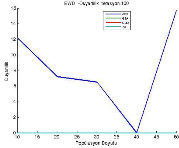
Şekil 2.7. WPBC veri kümesi üzerinde 100 iterasyon için ortalama duyarlılık sonuçları
