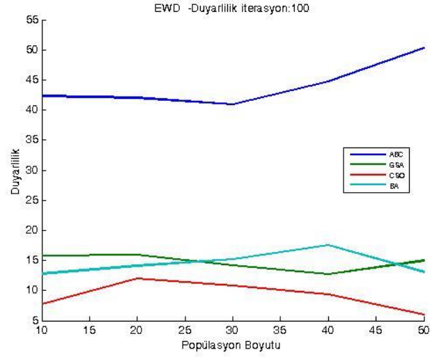
Şekil 2.43. QSAR veri kümesi üzerinde 100 iterasyon için ortalama duyarlılık sonuçları
