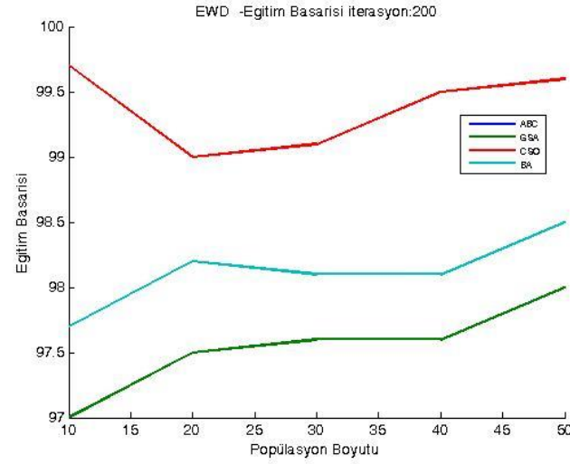
Şekil 2.38. QSAR veri kümesi üzerinde 200 iterasyon için ortalama eğitim başarıları
