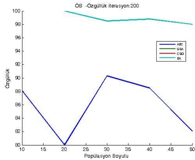
Şekil 1.11. WPBC veri kümesi üzerinde 200 iterasyon için ortalama özgüllük sonuçları
