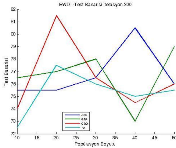
Şekil 2.6. WPBC veri kümesi üzerinde 300 iterasyon için ortalama test başarıları
