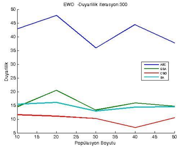
Şekil 2.45. QSAR veri kümesi üzerinde 300 iterasyon için ortalama duyarlılık sonuçları
