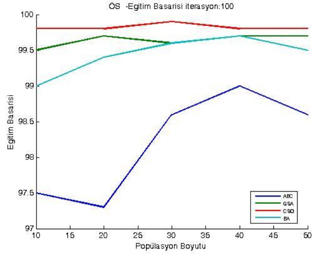
Şekil 1.55. DRD veri kümesi üzerinde 100 iterasyon için ortalama eğitim başarıları
