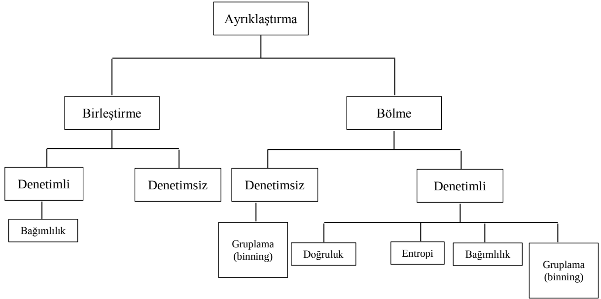
Şekil 6.1. Ayrıklaştırma yöntemleri için hiyerarşik bir çatı
