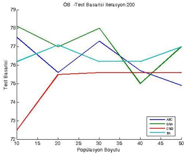
Şekil 1.41. QSAR veri kümesi üzerinde 200 iterasyon için ortalama test başarıları
