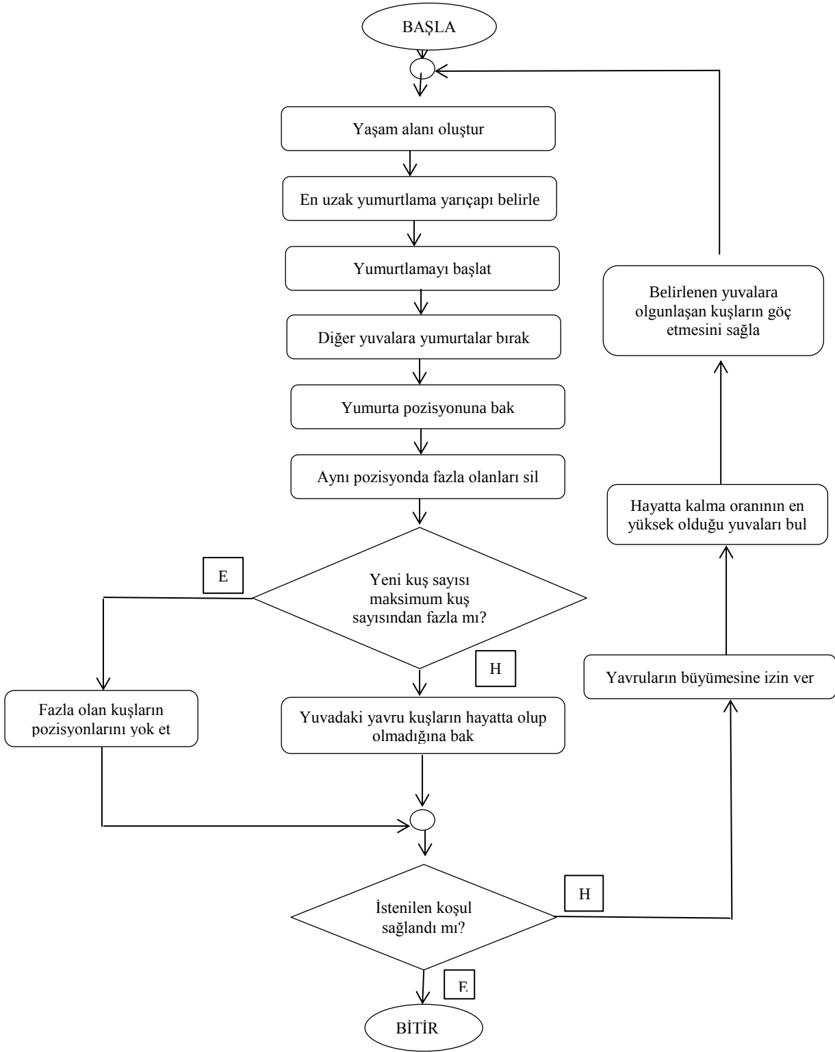
Şekil 3.3. CSO algoritmasının akış diyagramı
