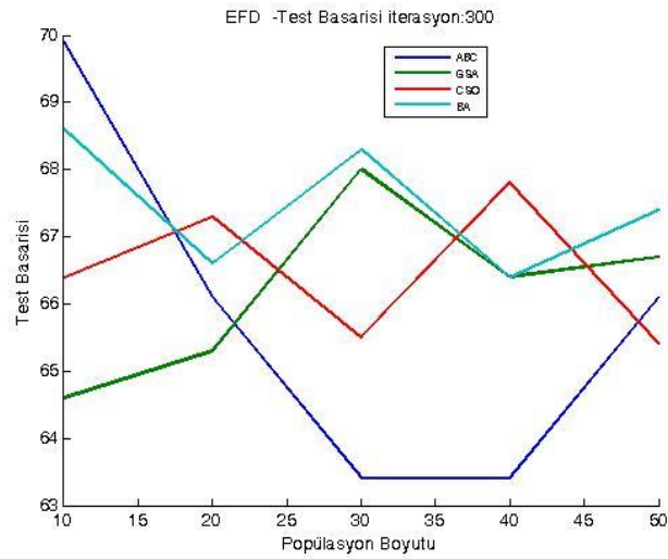
Şekil 3.42. QSAR veri kümesi üzerinde 300 iterasyon için ortalama test başarıları
