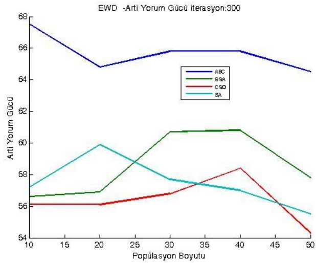
Şekil 2.69. DRD veri kümesi üzerinde 300 iterasyon için ortalama artı yorum gücü sonuçları
