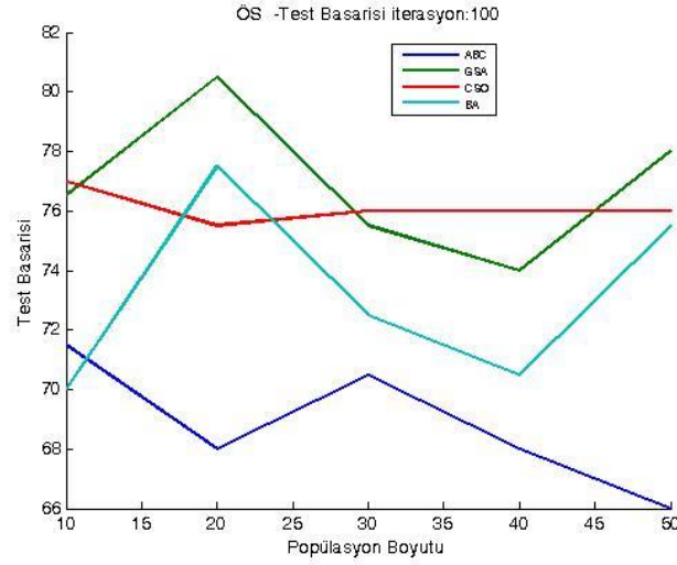
Şekil 1.4. WPBC veri kümesi üzerinde 100 iterasyon için ortalama test başarıları
