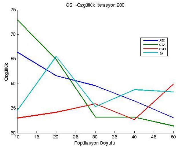
Şekil 1.65. DRD veri kümesi üzerinde 200 iterasyon için ortalama özgüllük sonuçları
