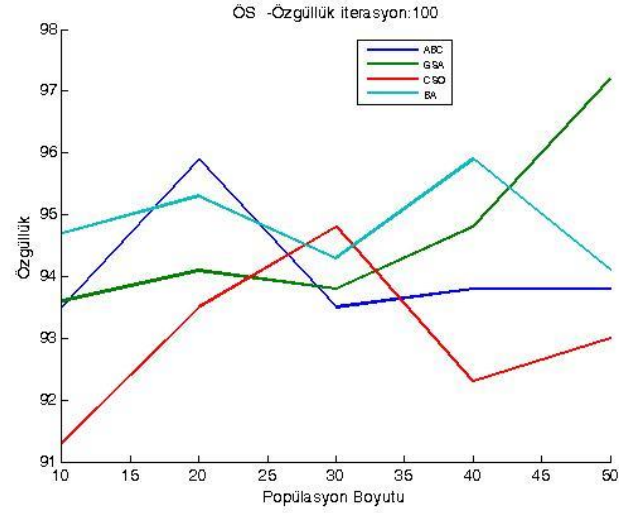
Şekil 1.28. BCW veri kümesi üzerinde 100 iterasyon için ortalama özgüllük sonuçları
