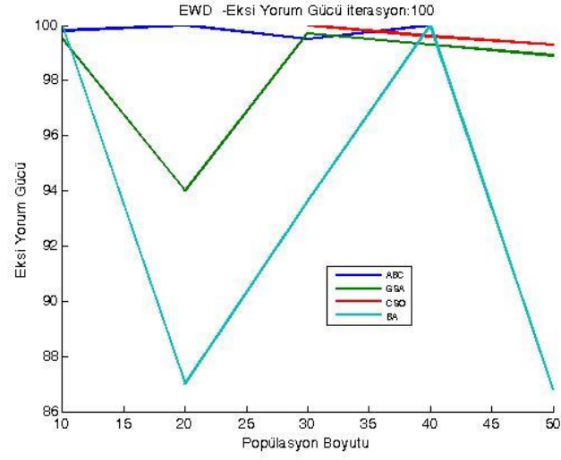
Şekil 2.34. BCW veri kümesi üzerinde 100 iterasyon için ortalama eksi yorum gücü sonuçları
