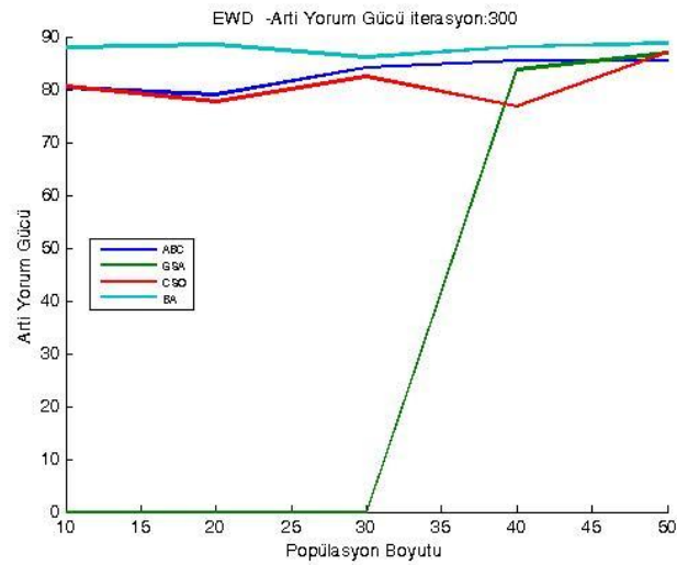
Şekil 2.33. BCW veri kümesi üzerinde 300 iterasyon için ortalama artı yorum gücü sonuçları
