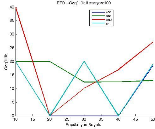
Şekil 3.64. DRD veri kümesi üzerinde 100 iterasyon için ortalama özgüllük sonuçları
