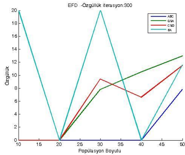
Şekil 3.66. DRD veri kümesi üzerinde 300 iterasyon için ortalama özgüllük sonuçları
