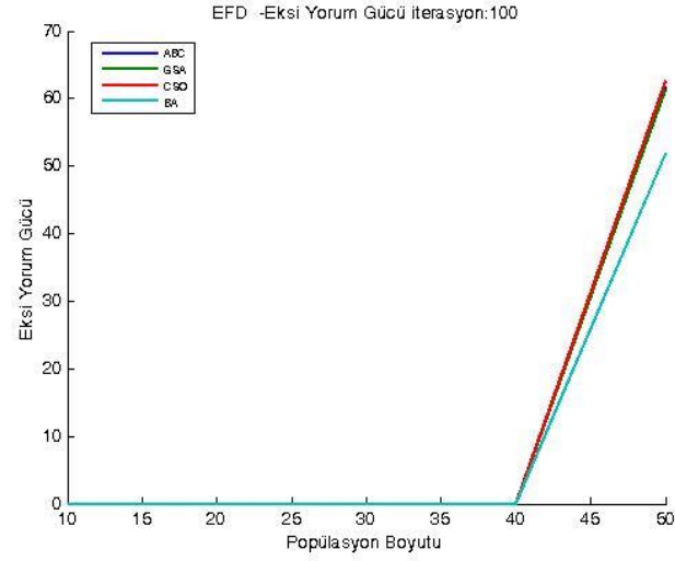
Şekil 3.70. DRD veri kümesi üzerinde 100 iterasyon için ortalama eksi yorum gücü sonuçları
