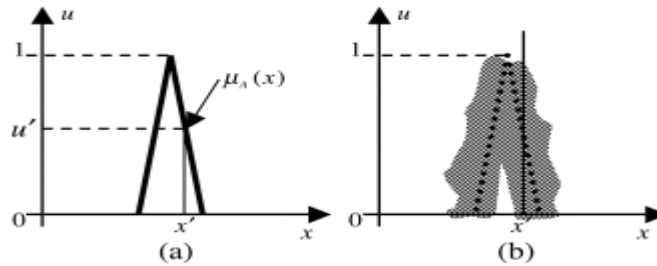
Şekil 3.3. (a) Tip-1 bulanık kümeler için üyelik fonksiyonu (b) Bulanıklaştırılmış Tip-1 üyelik fonksiyonu (Mendel ve ark., 2006).
