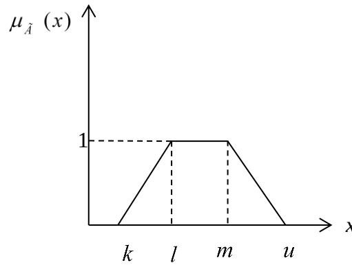
Şekil 3.2. Yamuksal bulanık sayı gösterimi
