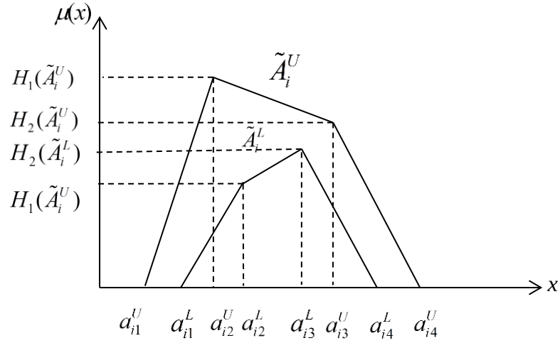
Şekil 3.7. Yamuksal Aralık Tip-2 bulanık küme (Chen ve Lee, 2010a).
