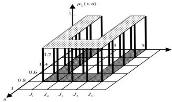
Şekil 3.5. Aralık Tip-2 bulanık kümeler için üyelik fonksiyonu örneği (Mendel ve ark.,2006).
