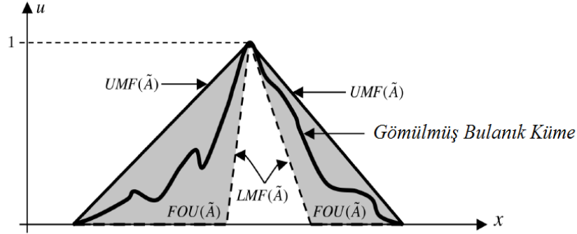
Şekil 3.6. FOU, LMF, UMF ve Aralık Tip-2 bulanık kümeler için gömülmüş bulanık küme (Mendel ve ark., 2006).
