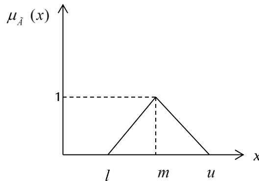
Şekil 3.1. Üçgensel bulanık sayı gösterimi
