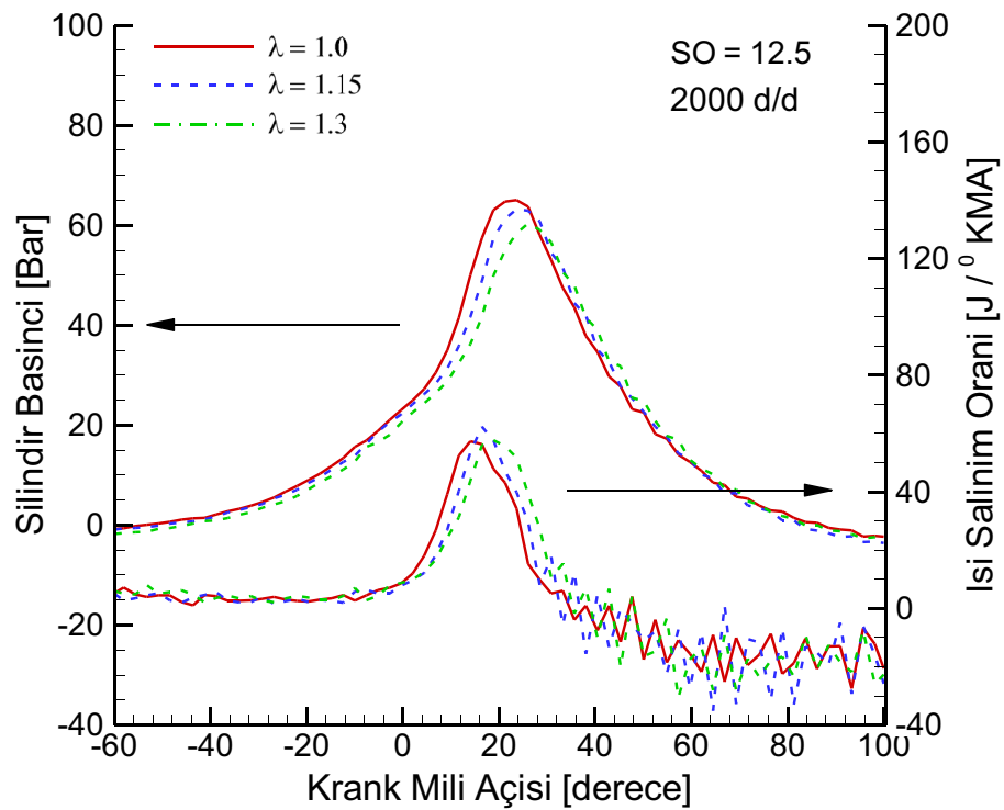
Şekil 3.13. Farklı hava fazlalık katsayılarında krank açısına göre silindir basıncı ve ısı salınım oranlarının değişimi (2000 d/d, SO=12.5).
