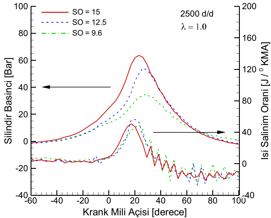
Şekil 3.12. Değişik sıkıştırma oranlarında krank mili açısına göre silindir basıncı ve ısı salınım oranlarının değişimi (2500 d/d, \lambda=1.0 ).
