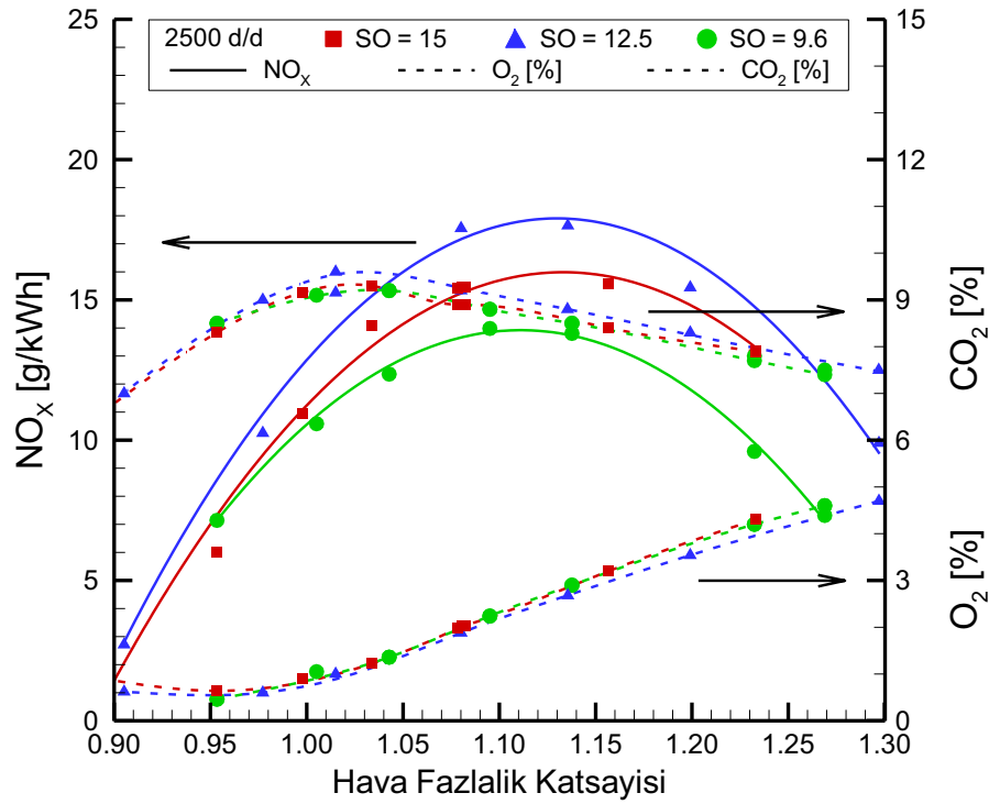
Şekil 3.21 Farklı sıkıştırma oranlarında ve 2500 d/d motor devrinde hava fazlalık katsayısına göre NO x , O 2 ve CO 2 değerleri.
