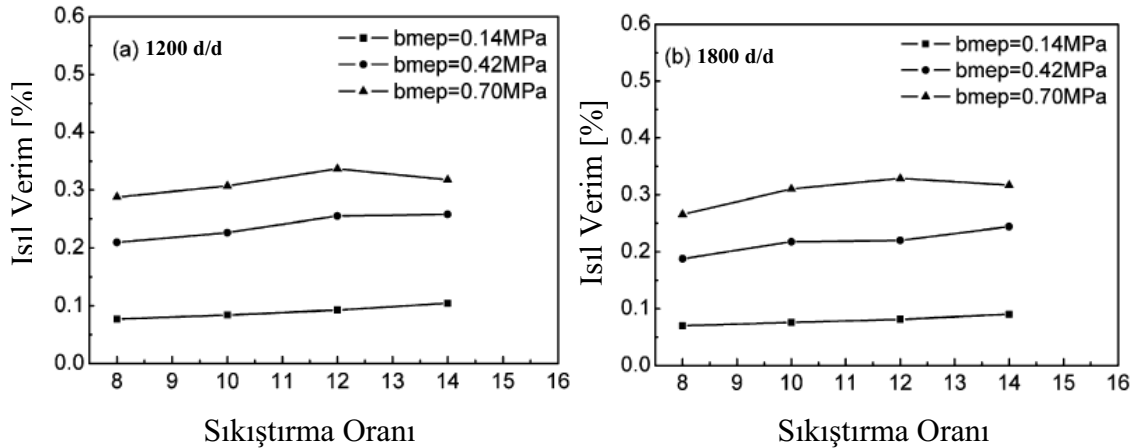
Şekil 1.1. Farklı güç ve devirlerde sıkıştırma oranının ısı verime etkisi [10].
