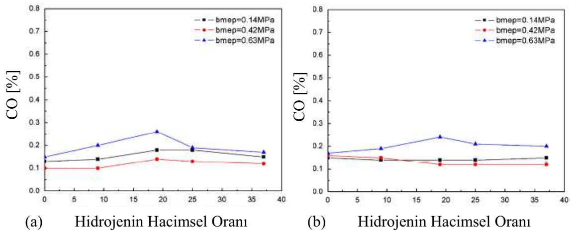
Şekil 1.14. Farklı güç değerlerinde hidrojen ilavesinin CO emisyonlarına etkisi [25].
