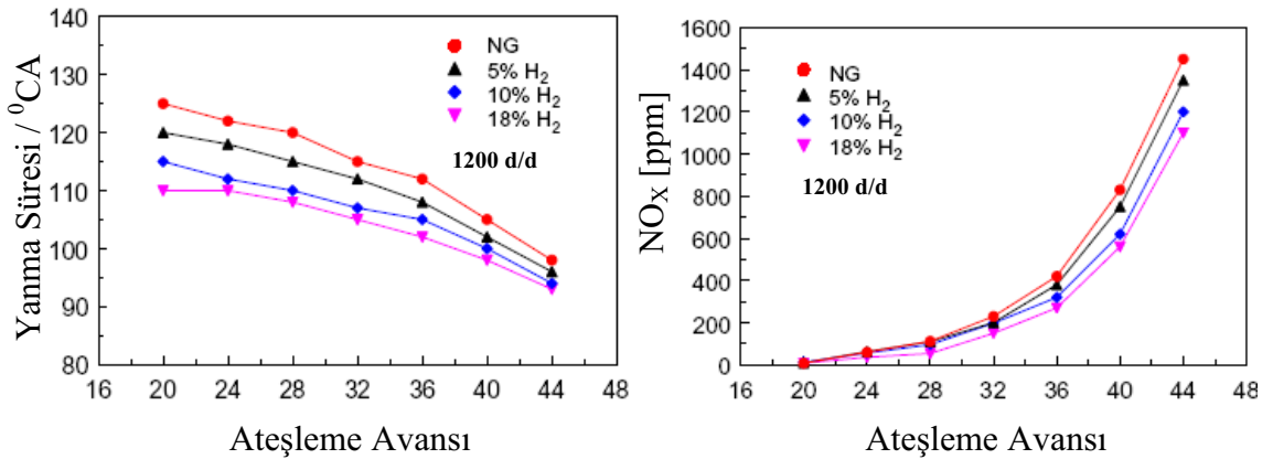
Şekil 1.6. Farklı ateşleme zamanlarında hidrojen ilavesinin yanma süresine ve NO x emisyonlarına etkisi [21].
