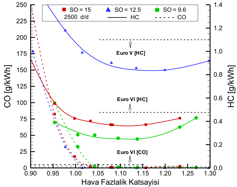
Şekil 3.17. Farklı sıkıştırma oranlarında hava fazlalık katsayısına göre CO ve HC emisyon değerleri (2000 d/d).
