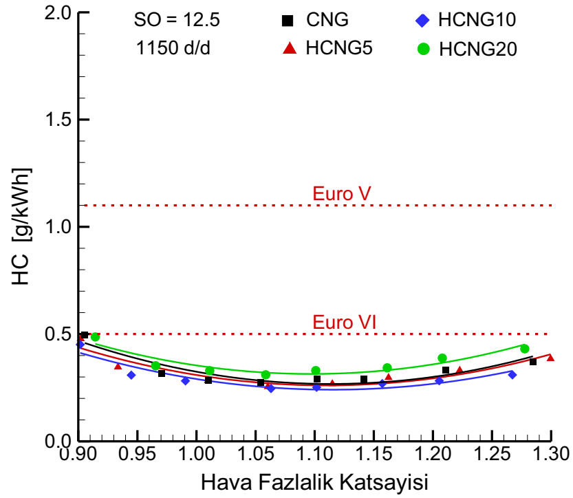
Şekil 3.59. 12.5 sıkıştırma oranında ve 1150 d/d motor devrinde hidrojen ilavesinin HC emisyonlarına etkisi.
