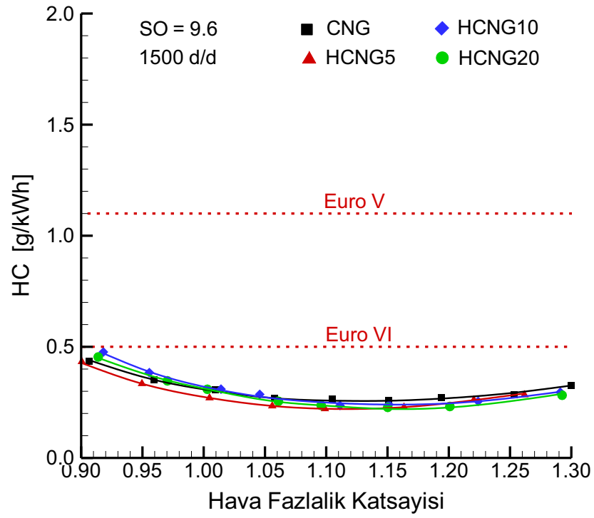
Şekil 3.56. 9.6 sıkıştırma oranında ve 1500 d/d motor devrinde hidrojen ilavesinin HC emisyonlarına etkisi.
