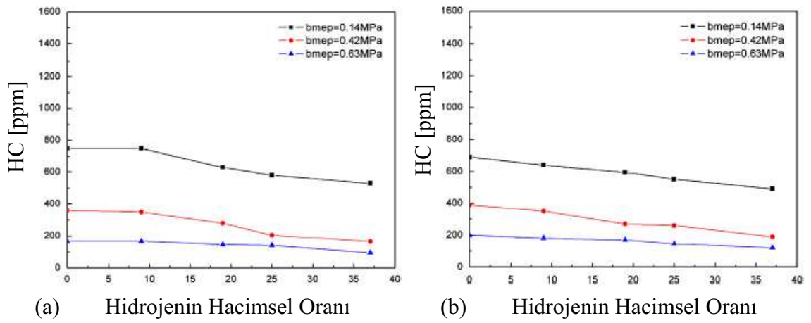
Şekil 1.13. Farklı güç değerlerinde hidrojen ilavesinin HC emisyonlarına etkisi [25].
