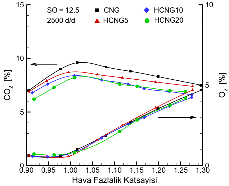
Şekil 3.77. 12.5 sıkıştırma oranında ve 2500 d/d motor devrinde hidrojen ilavesinin \text{CO}_2 ve \text{O}_2 emisyonlarına etkisi.
