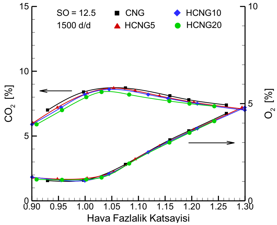
Şekil 3.73. 12.5 sıkıştırma oranında ve 1500 d/d motor devrinde hidrojen ilavesinin CO 2 ve O 2 emisyonlarına etkisi.
