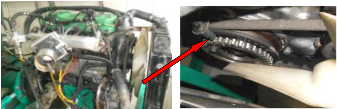
Şekil 2.8 Krank mili açılı sensörü ile dişli kasnağın görünümü.
