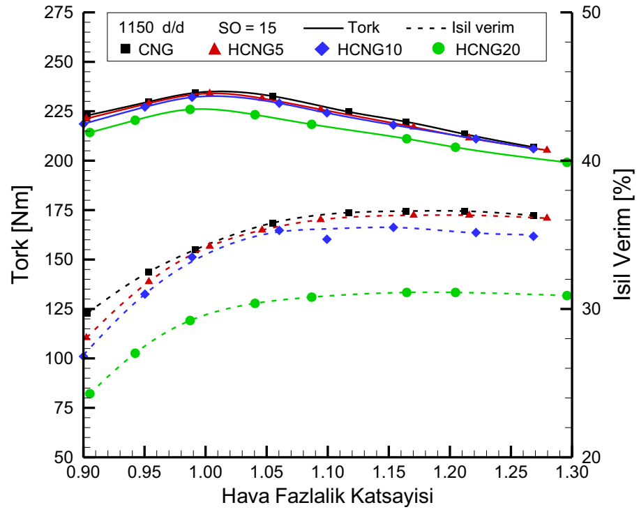
Şekil 3.22. Farklı HCNG yakıtları için hava fazlalık katsayısına göre tork ve ısı verim değerleri (1150 d/d, SO=15).
