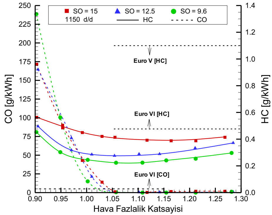
Şekil 3.14. Farklı sıkıştırma oranlarında hava fazlalık katsayısına göre CO ve HC emisyon değerleri (1150 d/d).
