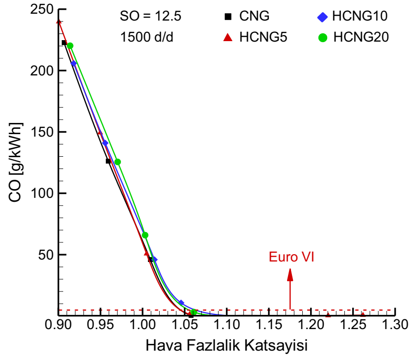
Şekil 3.63. 12.5 sıkıştırma oranında ve 1500 d/d motor devrinde hidrojen ilavesinin CO emisyonlarına etkisi.
