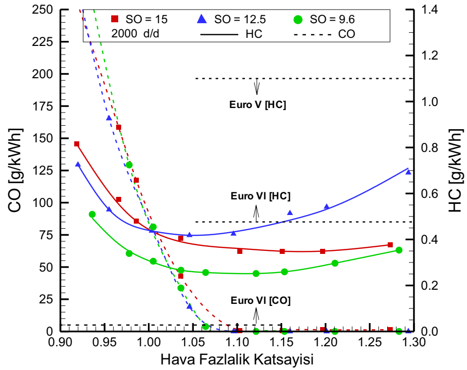
Şekil 3.16. Farklı sıkıştırma oranlarında hava fazlalık katsayısına göre CO ve HC emisyon değerleri (2000 d/d).
