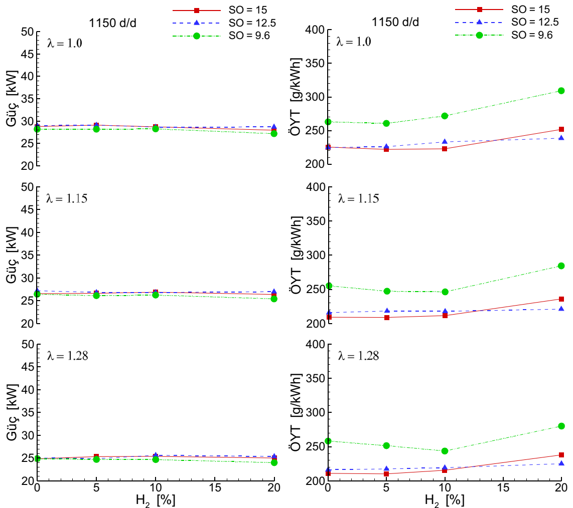
Şekil 3.34. Farklı sıkıştırma oranlarında \lambda=1.0 , \lambda=1.15 ve \lambda=1.28 değerleri için hidrojen ilavesinin motor gücü ve özgül yakıt tüketimine etkisi (1150 d/d).
