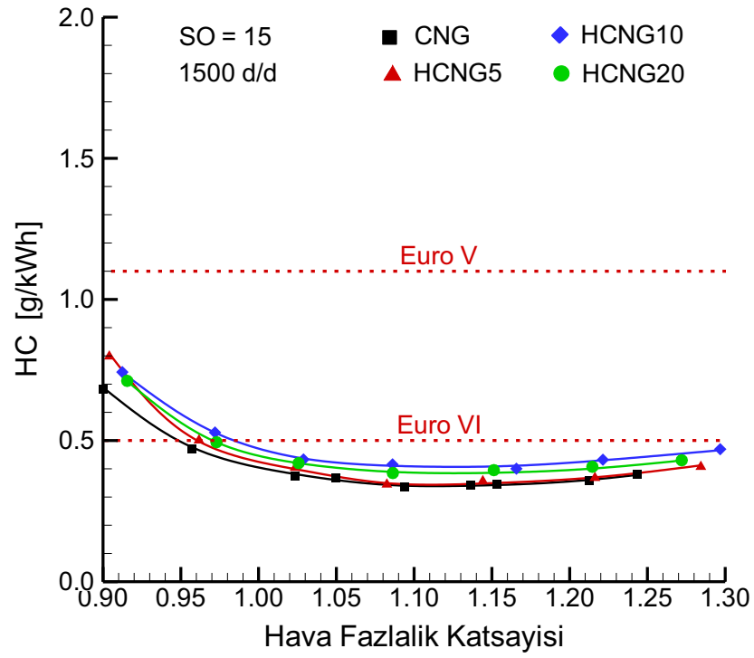
Şekil 3.58. 15 sıkıştırma oranında ve 1500 d/d motor devrinde hidrojen ilavesinin HC emisyonlarına etkisi.
