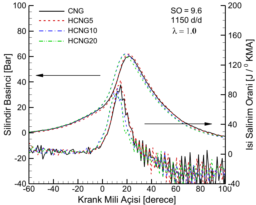
Şekil 3.38. Stokiyometrik şartlarda hidrojen ilavesinin silindir basıncına ve ısı salınım oranına etkisi (SO=9.6, 1150 d/d).
