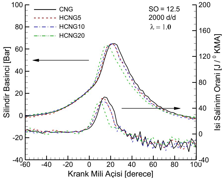
Şekil 3.44. Stokiyometrik şartlarda hidrojen ilavesinin silindir basıncına ve ısı salınım oranına etkisi (SO=12.5, 2000 d/d).
