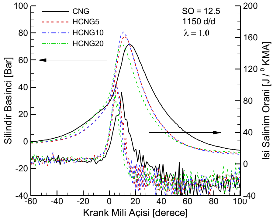
Şekil 3.42. Stokiyometrik şartlarda hidrojen ilavesinin silindir basıncına ve ısı salınım oranına etkisi (SO=12.5, 1150 d/d).
