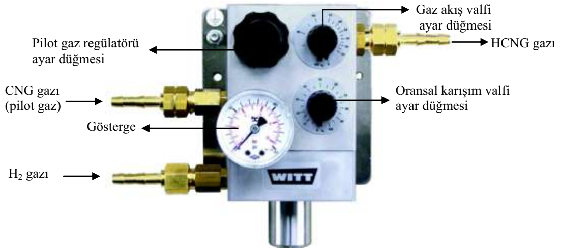
Şekil 2.20. MM-Flex gaz karışım ünitesinin görünümü [83].
