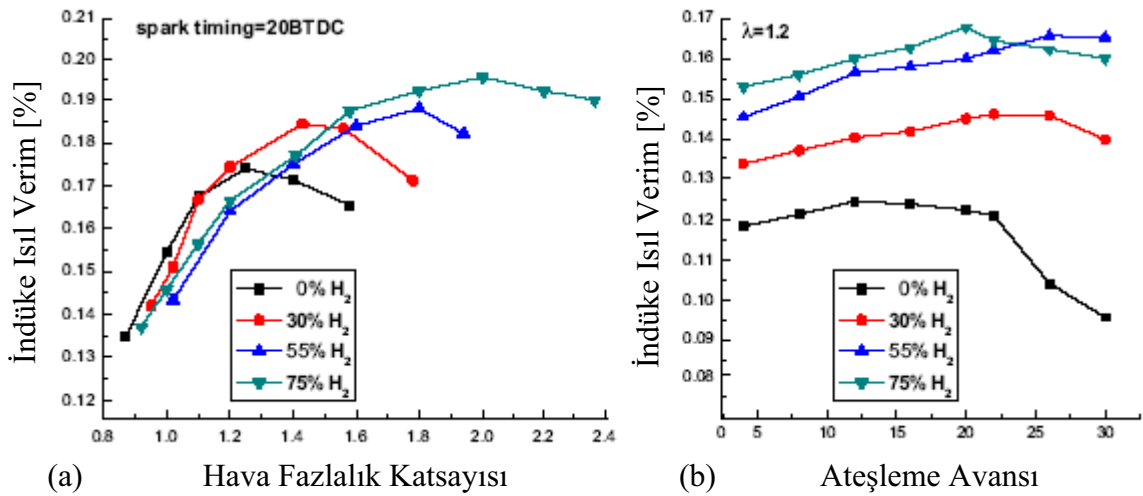
Şekil 1.18. Farklı hava fazlalık katsayılarında (a) ve ateşleme avanslarında (b) hidrojen ilavesinin indüke ısı verime etkisi [28].
