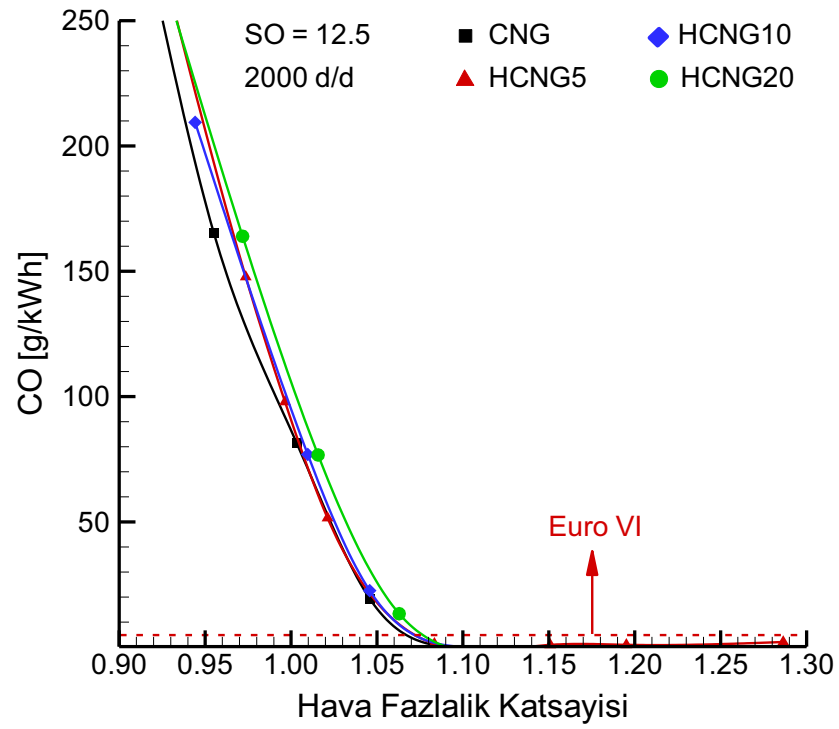
Şekil 3.66. 12.5 sıkıştırma oranında ve 2000 d/d motor devrinde hidrojen ilavesinin CO emisyonlarına etkisi.
