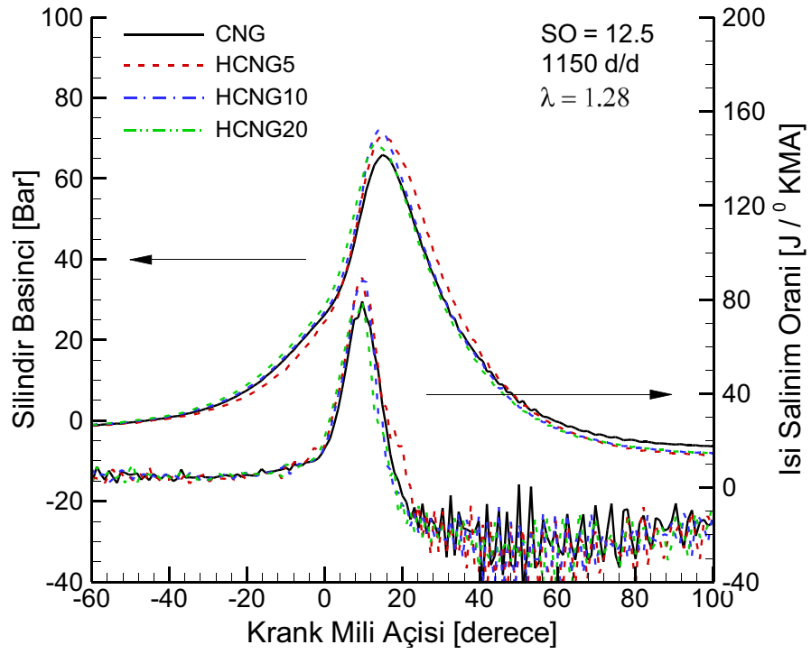
Şekil 3.50. \lambda=1.28 değerinde hidrojen ilavesinin silindir basıncına ve ısı salınım oranına etkisi ( SO=12.5 , 1150 \text{ d/d} ).
