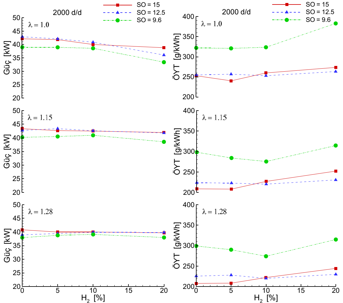
Şekil 3.36. Farklı sıkıştırma oranlarında \lambda=1.0 , \lambda=1.15 ve \lambda=1.28 değerleri için hidrojen ilavesinin motor gücü ve özgül yakıt tüketimine etkisi (2000 d/d).
