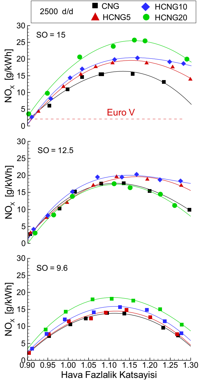
Şekil 3.71. Farklı sıkıştırma oranında ve 2500 d/d motor devrinde hidrojen ilavesinin NO x emisyonlarına etkisi.
