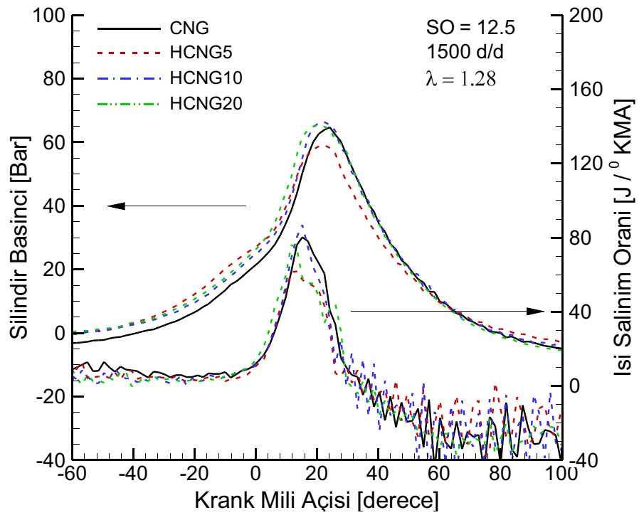
Şekil 3.51. \lambda=1.28 değerinde hidrojen ilavesinin silindir basıncına ve ısı salınım oranına etkisi ( SO=12.5 , 1500 \text{ d/d} ).
