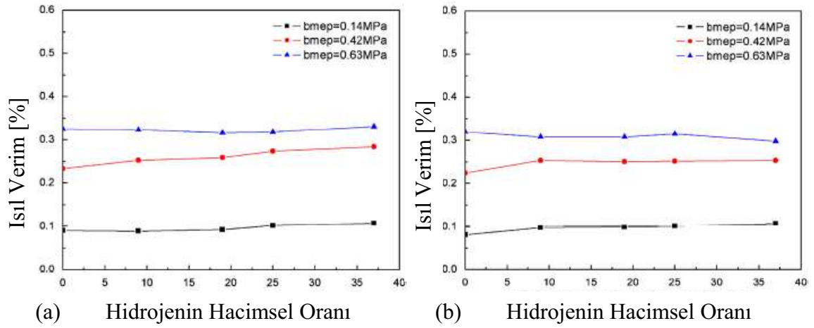
Şekil 1.12. Farklı güç değerlerinde hidrojen ilavesinin ısı verime etkisi [25].
