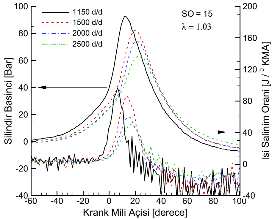
Şekil 3.10. Değişik motor devirlerinde krank mili açısına göre silindir basıncı ve ısı salınım oranlarının değişimi (SO=15, \lambda=1.03 ).
