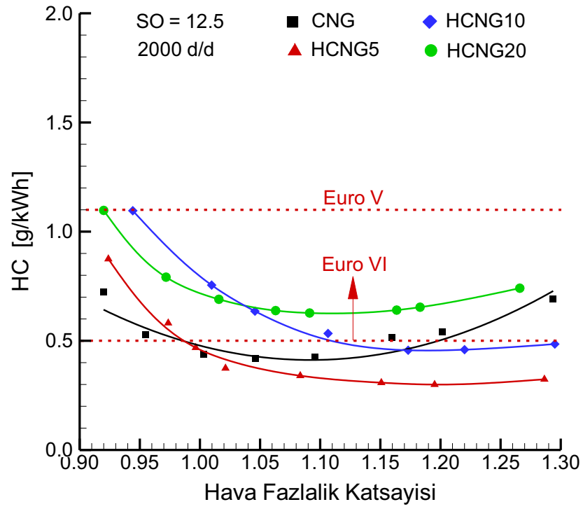
Şekil 3.60. 12.5 sıkıştırma oranında ve 2000 d/d motor devrinde hidrojen ilavesinin HC emisyonlarına etkisi.
