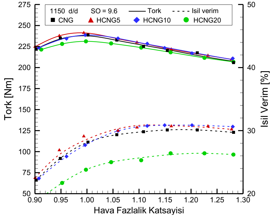
Şekil 3.24. Farklı HCNG yakıtları için hava fazlalık katsayısına göre tork ve ısı verim değerleri (1150 d/d, SO=9.6).
