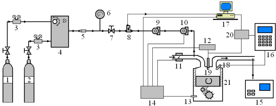
1- Hidrojen tankı 2- CNG tankı 3- Regülatör (12.5 bar) 4- Gaz karışım ünitesi 5- Alev tutucu 6- Basınç göstergesi 7- Check valf 8- Debimetre 9- Regülatör (8 bar) 10- Regülatör (1 bar) 11- Gaz keleşği konum sensörü 12- Ateşleme modülü 13- Krank açısı sensörü 14- Motor Kontrol ünitesi 15- Egzoz gaz analizörü 16- Amplitifikatör 17- Bilgisayar 18- Basınç Sensörü 19- Buji 20- Picoscope 21- Motor ve dinamometre.
