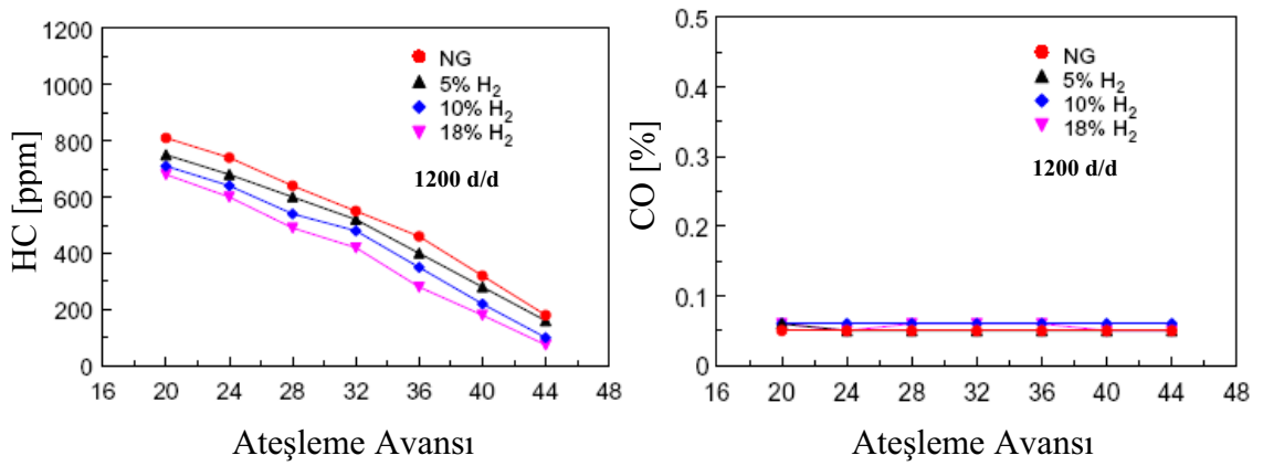
Şekil 1.5. Farklı ateşleme zamanlarında hidrojen ilavesinin HC ve CO emisyonlarına etkisi [21].
