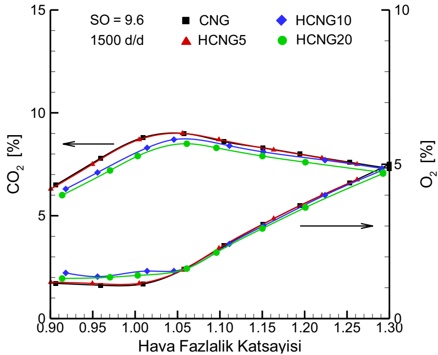
Şekil 3.72. 9.6 sıkıştırma oranında ve 1500 d/d motor devrinde hidrojen ilavesinin \text{CO}_2 ve \text{O}_2 emisyonlarına etkisi.
