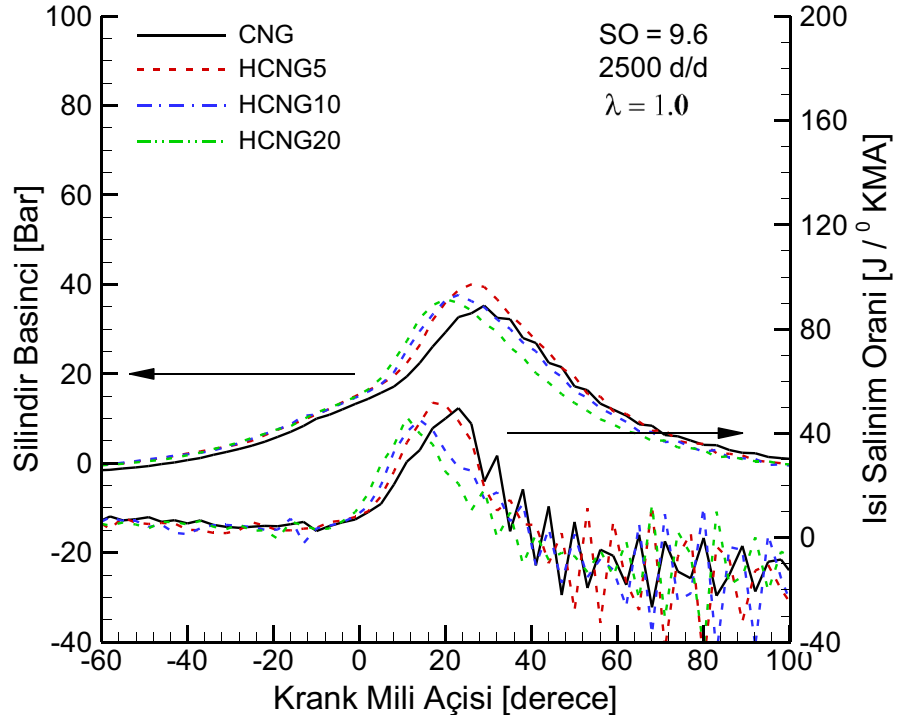
Şekil 3.41. Stokiyometrik şartlarda hidrojen ilavesinin silindir basıncına ve ısı salınım oranına etkisi (SO=9.6, 2500 d/d).
