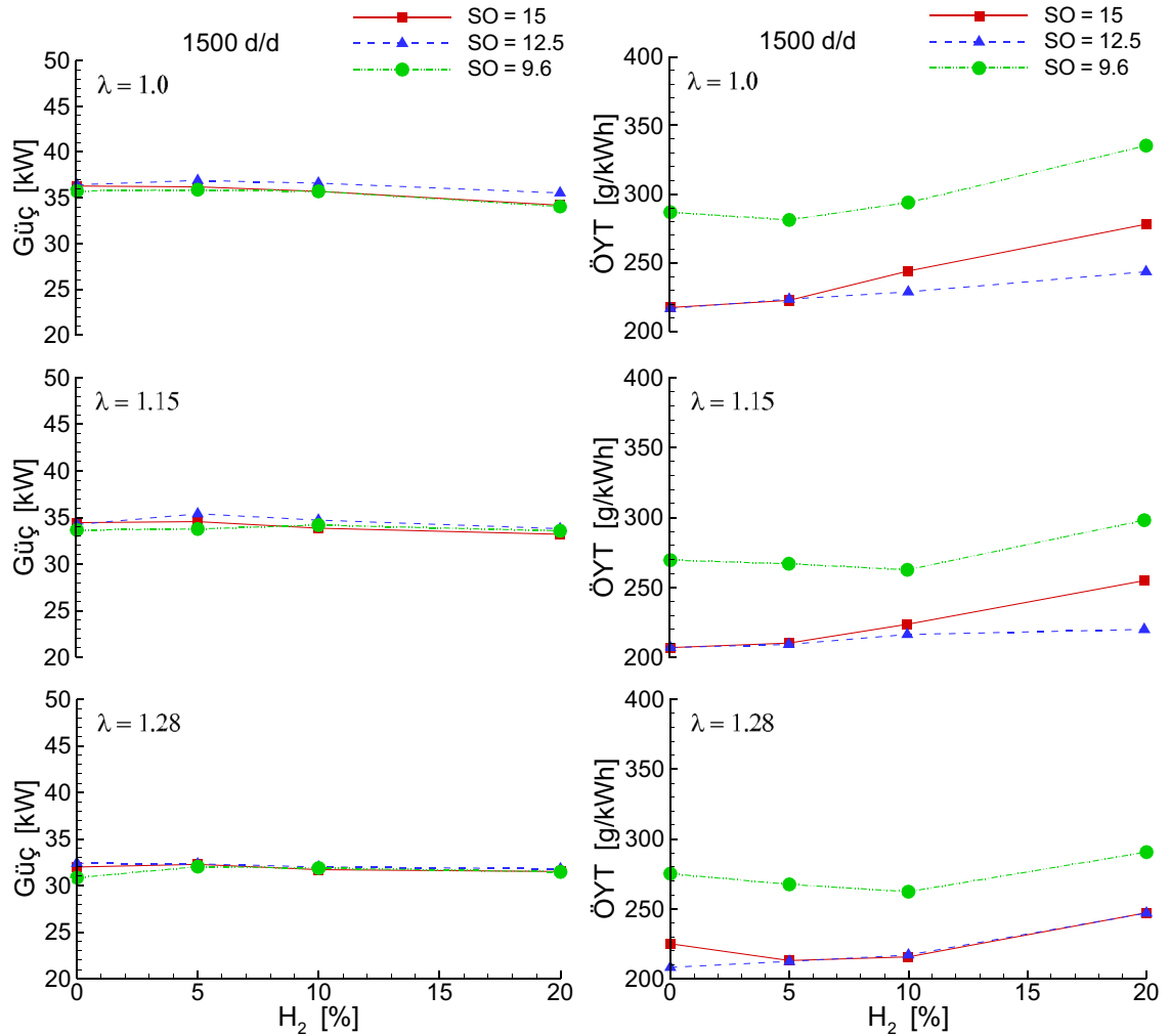
Şekil 3.35. Farklı sıkıştırma oranlarında \lambda=1.0 , \lambda=1.15 ve \lambda=1.28 değerleri için hidrojen ilavesinin motor gücü ve özgül yakıt tüketimine etkisi (1500 d/d).
