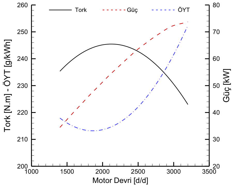
Şekil 2.1. Isuzu 4BD1 motoruna ait performans verilerinin motor devrine bağlı olarak değişimi [58].
