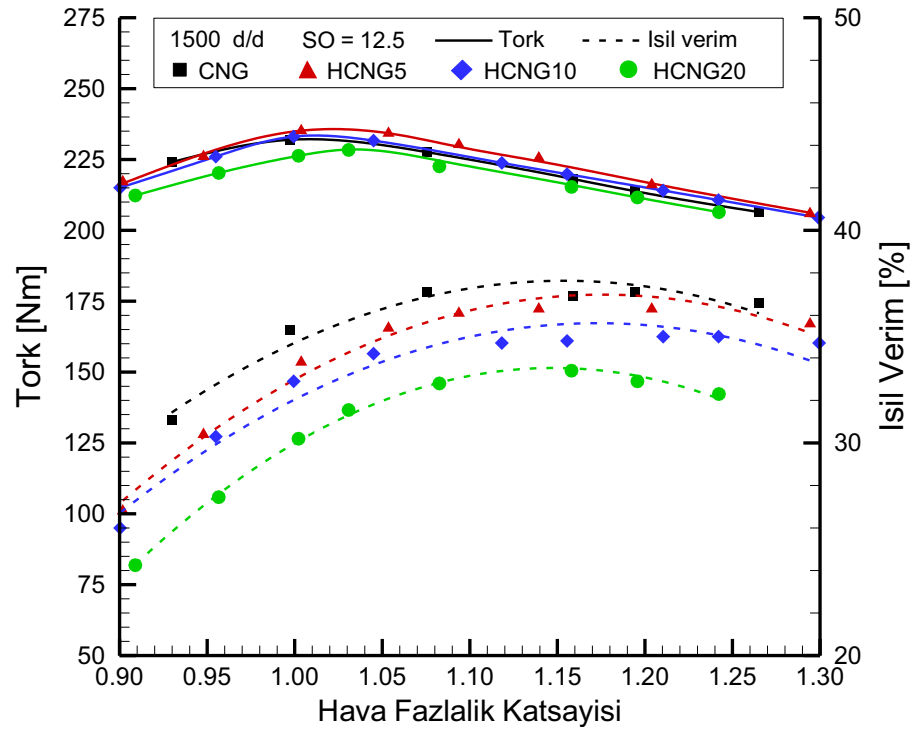
Şekil 3.26. Farklı HCNG yakıtları için hava fazlalık katsayısına göre tork ve ısı verim değerleri (1500 d/d, SO=12.5).
