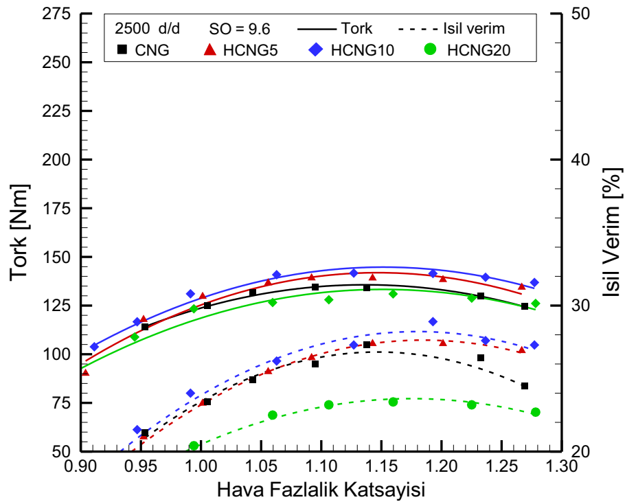
Şekil 3.33. Farklı HCNG yakıtları için hava fazlalık katsayısına göre tork ve ısı verim değerleri (2500 d/d, SO=9.6).
