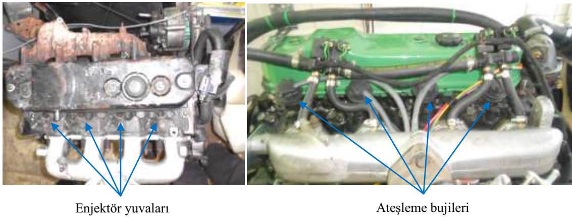
Şekil 2.5. Enjektör yuvaları ve sisteme entegre edilen bujilerin görüntüleri.
