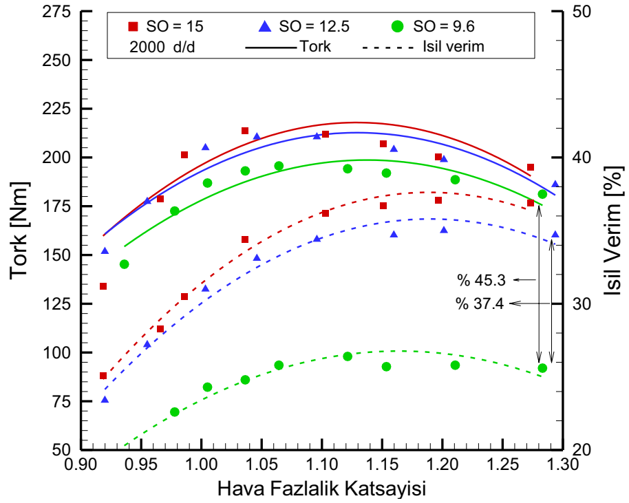
Şekil 3.4. 2000 d/d motor devrinde ve farklı sıkıştırma oranlarında hava fazlalık katsayısına göre tork ve ısı verim değerleri.
