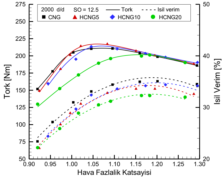
Şekil 3.29. Farklı HCNG yakıtları için hava fazlalık katsayısına göre tork ve ısı verim değerleri (2000 d/d, SO=12.5).
