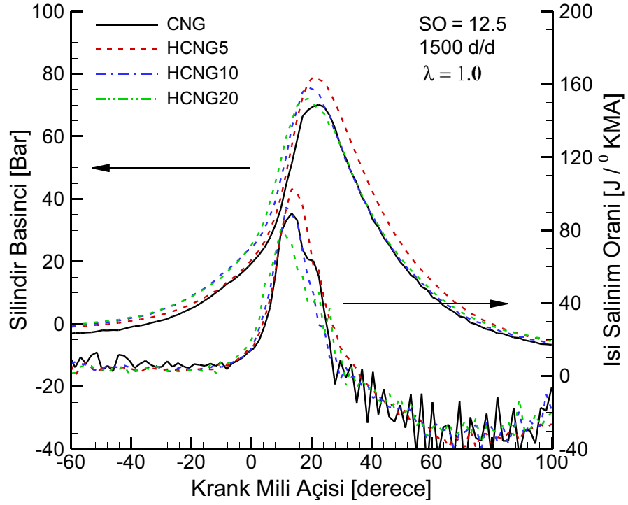
Şekil 3.43. Stokiyometrik şartlarda hidrojen ilavesinin silindir basıncına ve ısı salınım oranına etkisi (SO=12.5, 1500 d/d).
