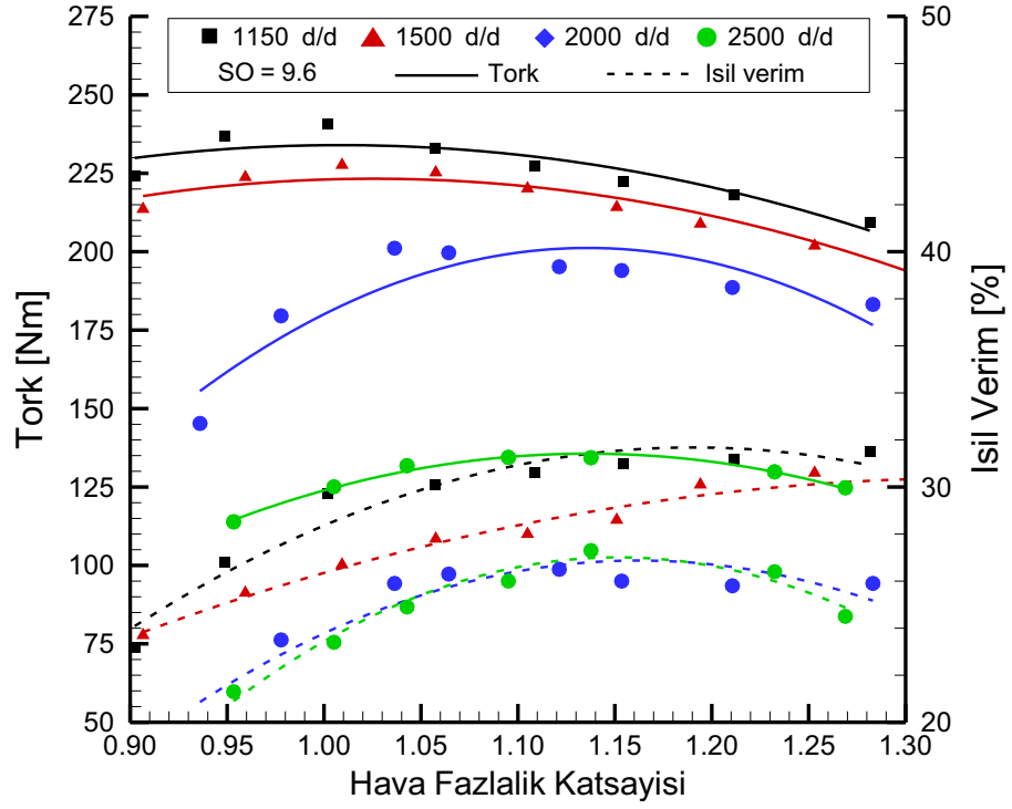
Şekil 3.3. SO=9.6 sıkıştırma oranında ve farklı motor devirlerinde hava fazlalık katsayısına göre tork ve ısı verim değerleri.
