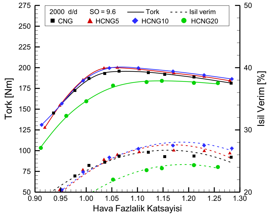
Şekil 3.30. Farklı HCNG yakıtları için hava fazlalık katsayısına göre tork ve ısı verim değerleri (2000 d/d, SO=9.6).
