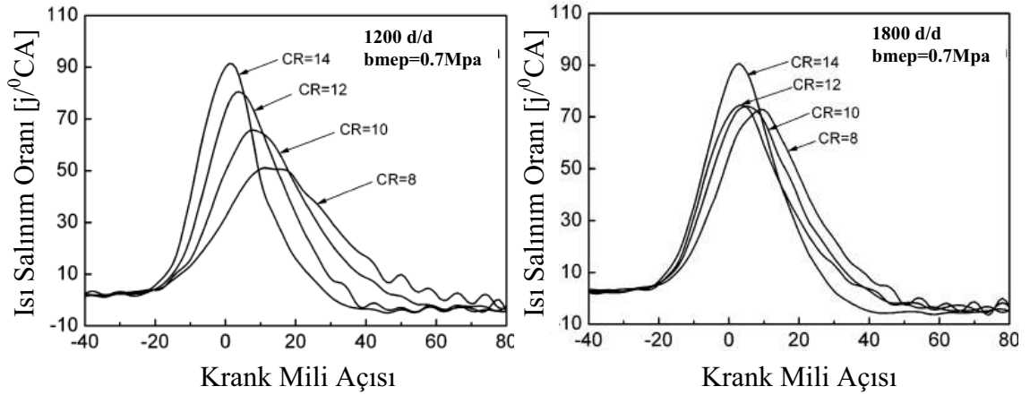
Şekil 1.2. Farklı güç ve devirlerde sıkıştırma oranının ısı salınım oranına etkisi [10].
