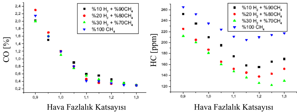
Şekil 1.16. Farklı hava fazlalık katsayılarında hidrojen ilavesinin CO ve HC emisyonlarına etkisi [26].
