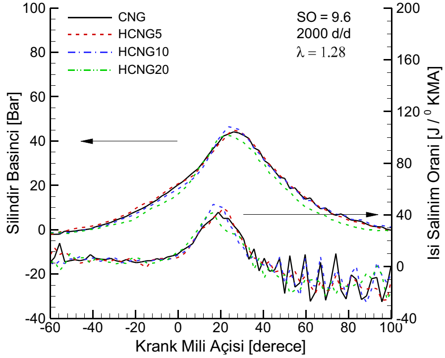
Şekil 3.54. \lambda=1.28 değerinde hidrojen ilavesinin silindir basıncına ve ısı salınım oranına etkisi (SO=9.6, 2000 d/d).
