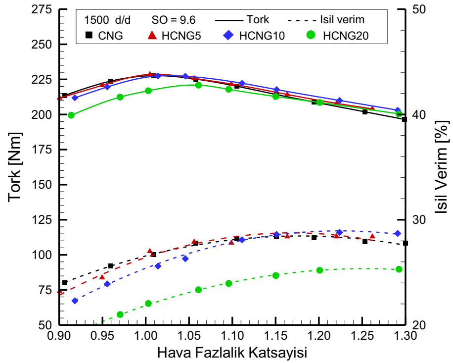
Şekil 3.27. Farklı HCNG yakıtları için hava fazlalık katsayısına göre tork ve ısı verim değerleri (1500 d/d, SO=9.6).
