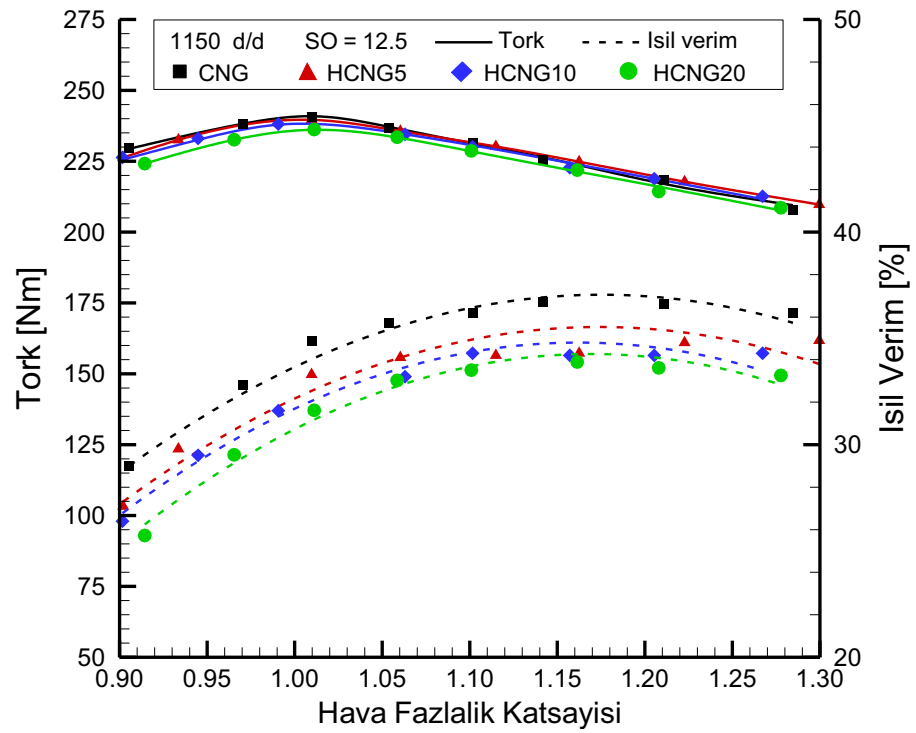
Şekil 3.23. Farklı HCNG yakıtları için hava fazlalık katsayısına göre tork ve ısı verim değerleri (1150 d/d, SO=12.5).
