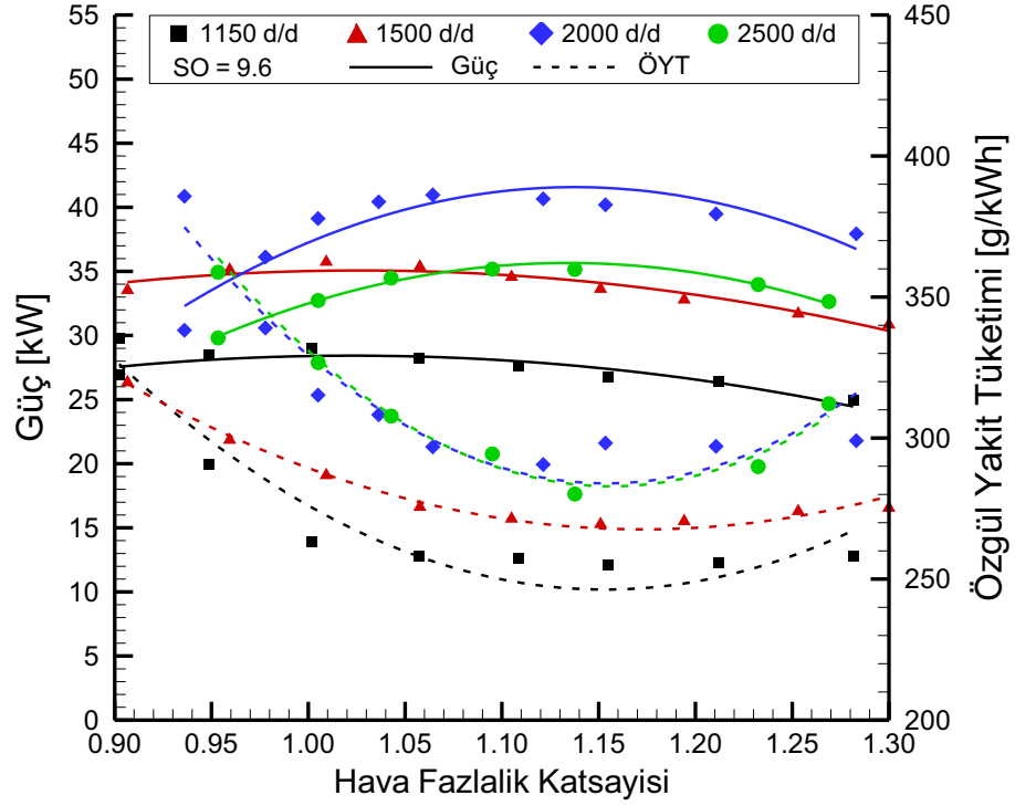
Şekil 3.5. Değişik motor devirlerinde hava fazlalık katsayısına göre güç ve özgül yakıt tüketim değerleri (SO=9.6).
