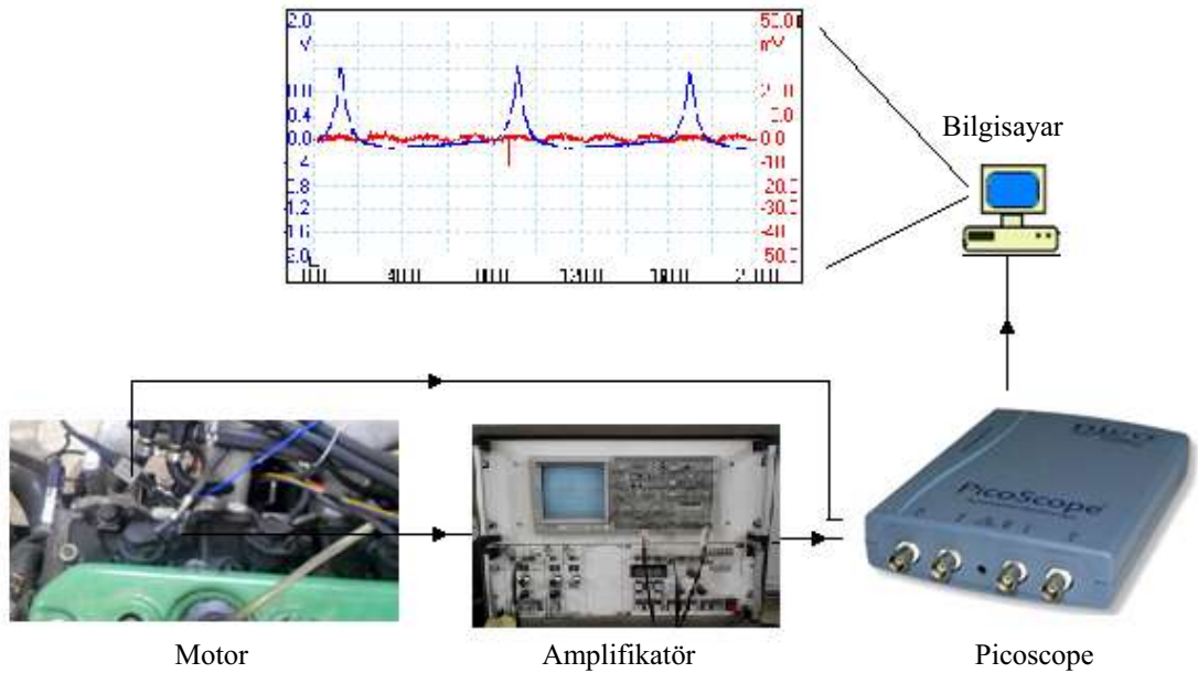
Şekil 2.17. Krank açısı ve silindir içi basınç değerlerinin bilgisayara aktarılması.
