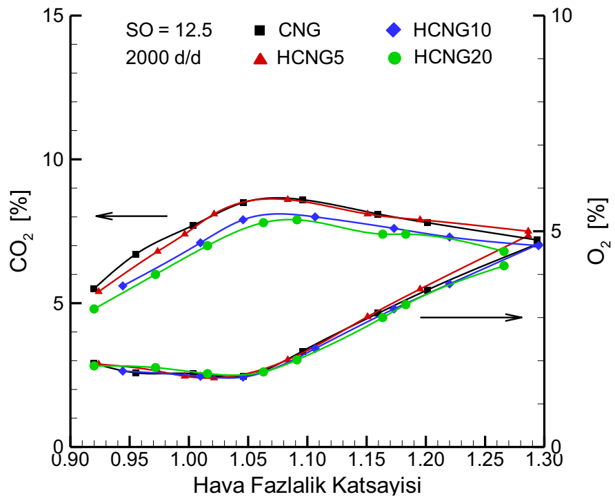
Şekil 3.76. 12.5 sıkıştırma oranında ve 2000 d/d motor devrinde hidrojen ilavesinin CO 2 ve O 2 emisyonlarına etkisi.
