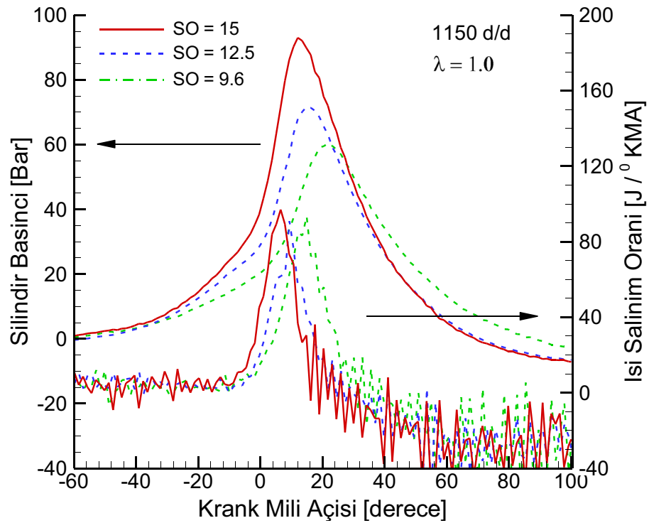
Şekil 3.11. Değişik sıkıştırma oranlarında krank mili açısına göre silindir basıncı ve ısı salınım oranlarının değişimi (1150 d/d, \lambda=1.0 ).
