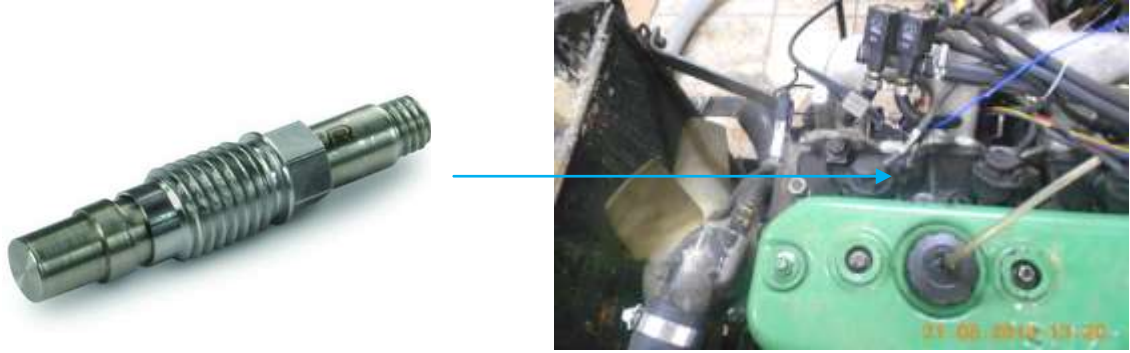
Şekil 2.16. PCB 112A05 model silindir içi basınç sensörü ve motorda yerleşimi.
