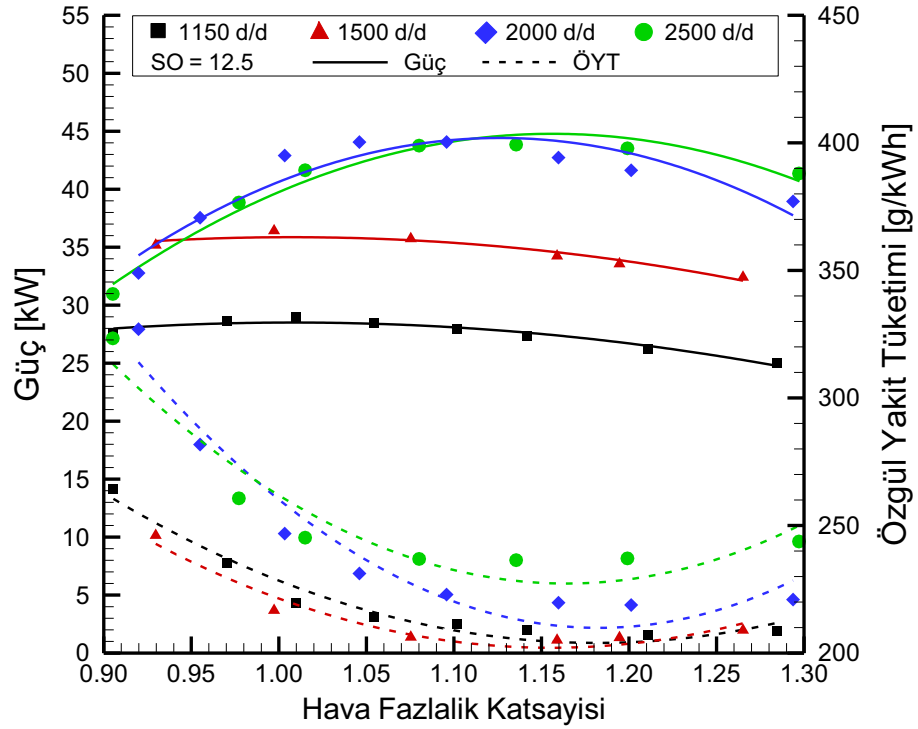
Şekil 3.6. Değişik motor devirlerinde hava fazlalık katsayısına göre güç ve özgül yakıt tüketim değerleri (SO=12.5).
