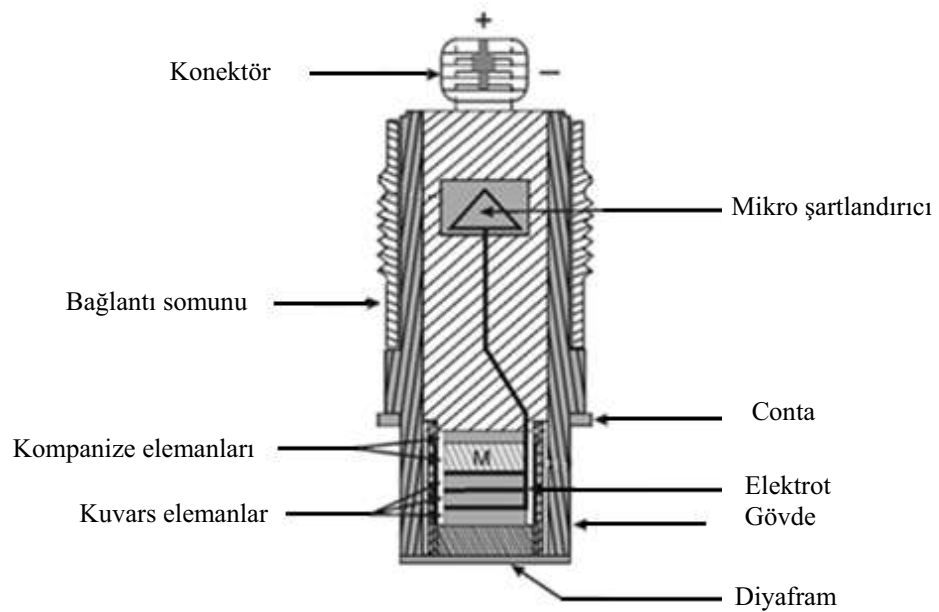
Şekil 2.14. Mikro şartlandırıcılı piezoelektrik elemanın içyapısı [75].
