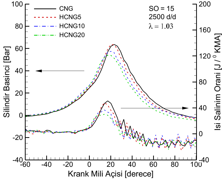
Şekil 3.49. Stokiyometrik şartlarda hidrojen ilavesinin silindir basıncına ve ısı salınım oranına etkisi (SO=15, 2500 d/d).
