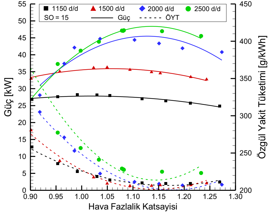
Şekil 3.7. Değişik motor devirlerinde hava fazlalık katsayısına göre güç ve özgül yakıt tüketim değerleri (SO=15).
