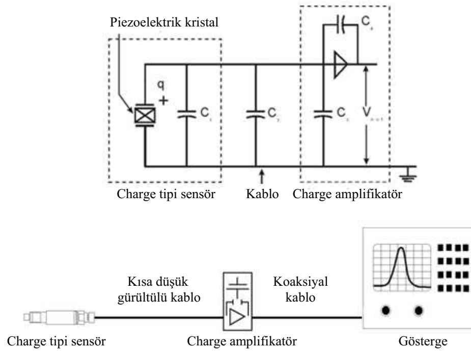
Şekil 2.15. Charge tipi sensörlerden çıkan sinyallerin şartlandırılması [75, 76].
