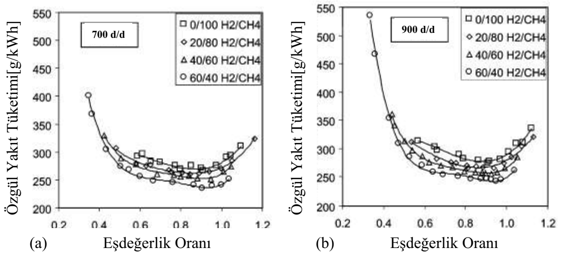
Şekil 1.8. Farklı hava-yakıt oranlarında hidrojen ilavesinin özgül yakıt tüketimine etkisi [24].
