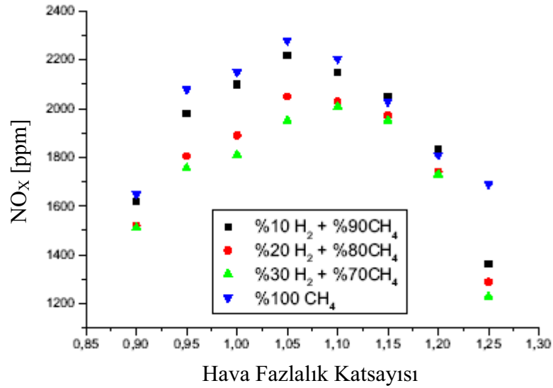
Şekil 1.17. Farklı hava fazlalık katsayılarında hidrojen ilavesinin NO x emisyonlarına etkisi [26].
