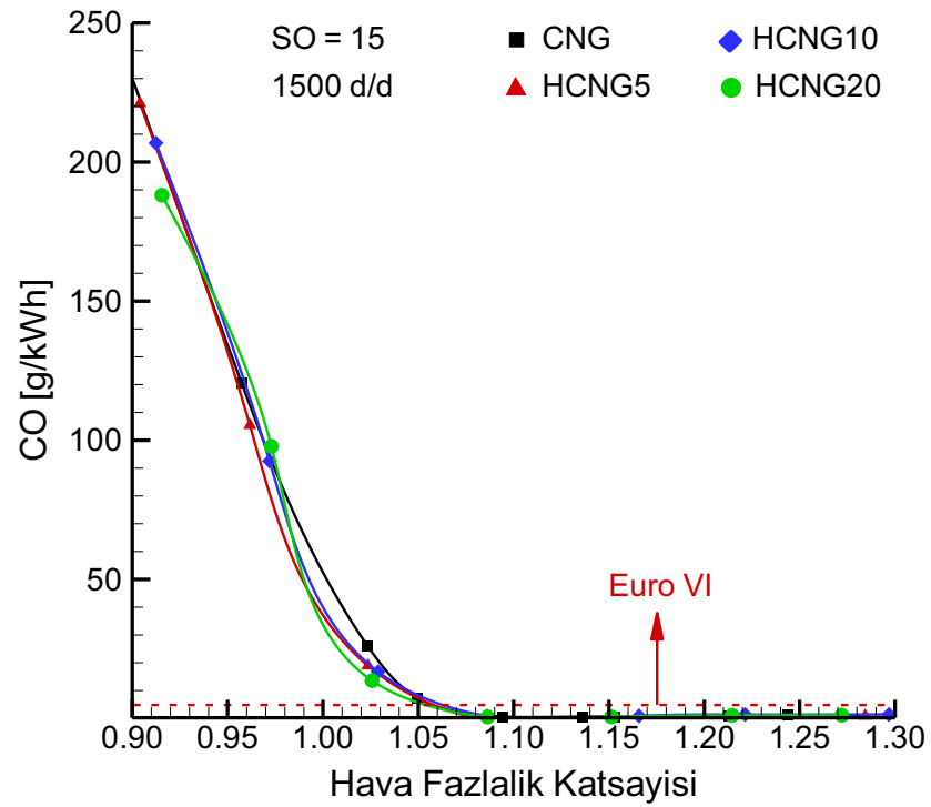
Şekil 3.64. 15 sıkıştırma oranında ve 1500 d/d motor devrinde hidrojen ilavesinin CO emisyonlarına etkisi.
