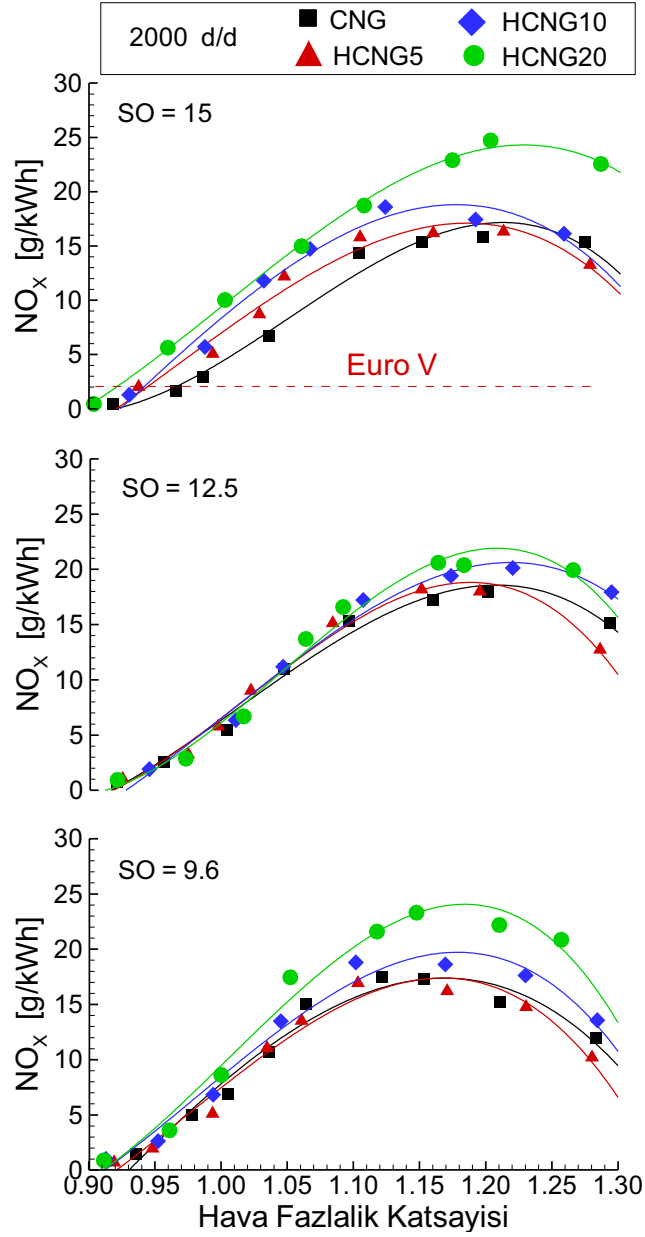
Şekil 3.70. Farklı sıkıştırma oranında ve 2000 d/d motor devrinde hidrojen ilavesinin NO x emisyonlarına etkisi.
