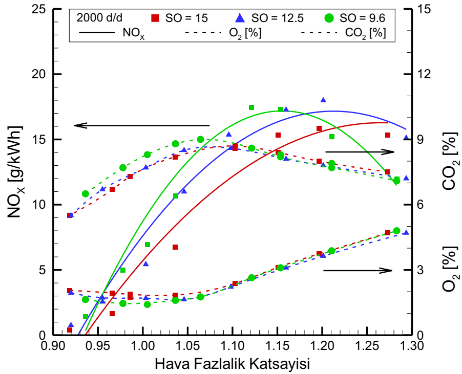
Şekil 3.20. Farklı sıkıştırma oranlarında ve 2000 d/d motor devrinde hava fazlalık katsayısına göre NO x , O 2 ve CO 2 değerleri.
