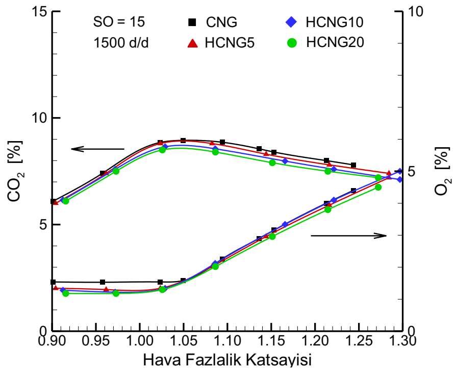
Şekil 3.74. 15 sıkıştırma oranında ve 1500 d/d motor devrinde hidrojen ilavesinin CO 2 ve O 2 emisyonlarına etkisi.
