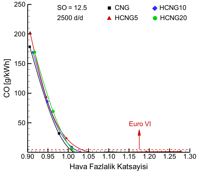
Şekil 3.67. 12.5 sıkıştırma oranında ve 2500 d/d motor devrinde hidrojen ilavesinin CO emisyonlarına etkisi.
