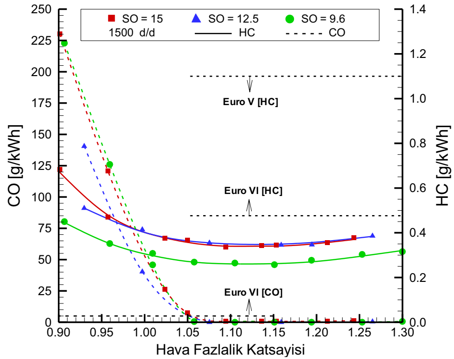
Şekil 3.15. Farklı sıkıştırma oranlarında hava fazlalık katsayısına göre CO ve HC emisyon değerleri (1500 d/d).
