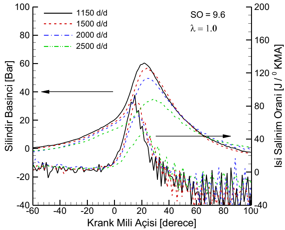
Şekil 3.8. Değişik motor devirlerinde krank mili açısına göre silindir basıncı ve ısı salınım oranlarının değişimi (SO=9.6, \lambda=1.0 ).
