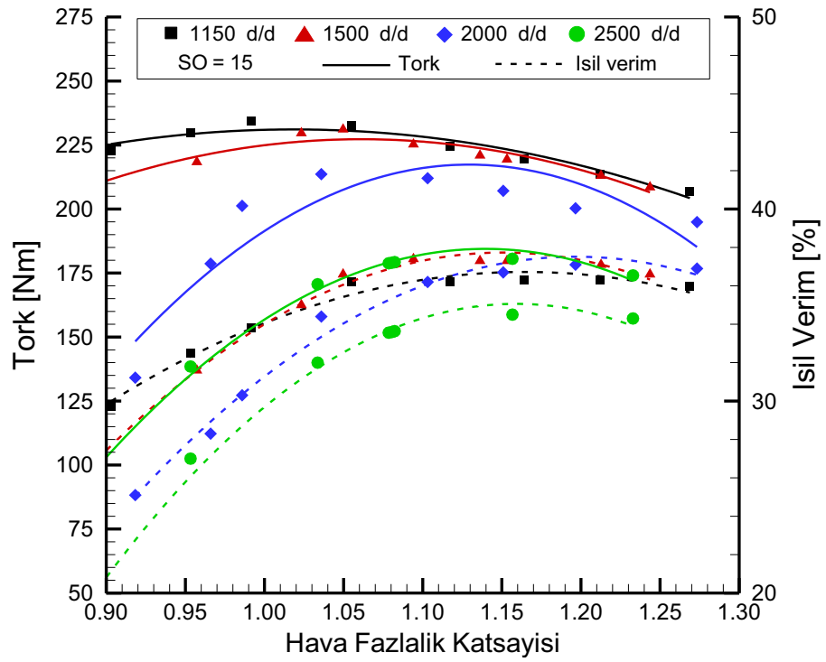
Şekil 3.1. SO=15 sıkıştırma oranında ve farklı motor devirlerinde hava fazlalık katsayısına göre tork ve ısı verim değerleri.
