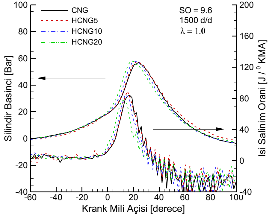
Şekil 3.39. Stokiyometrik şartlarda hidrojen ilavesinin silindir basıncına ve ısı salınım oranına etkisi (SO=9.6, 1500 d/d).
