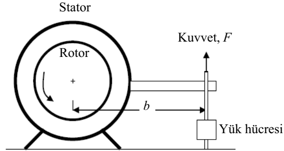
Şekil 2.12. Tork ölçme prensibi [67].
