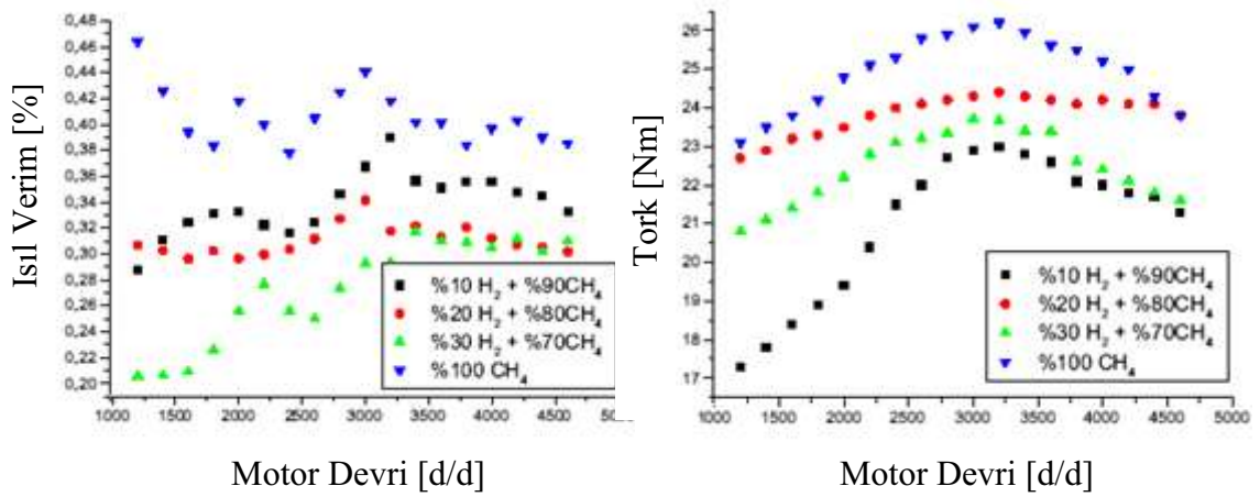
Şekil 1.15. Farklı motor devir sayılarında hidrojen ilavesinin ısı verim ve torka etkisi [26].
