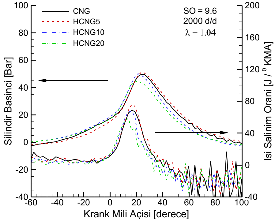
Şekil 3.40. Stokiyometrik şartlarda hidrojen ilavesinin silindir basıncına ve ısı salınım oranına etkisi (SO=9.6, 2000 d/d).
