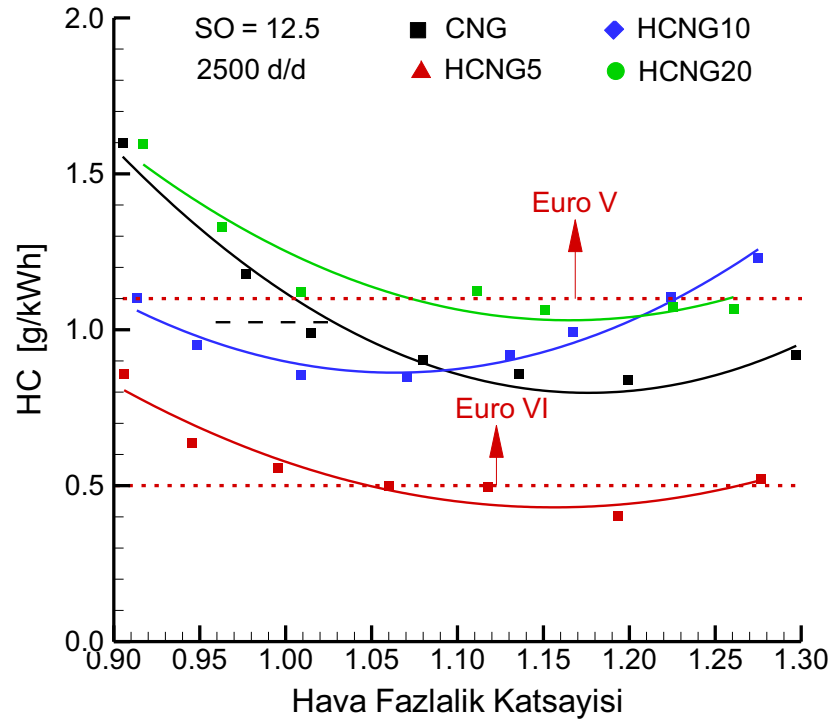
Şekil 3.61. 12.5 sıkıştırma oranında ve 2500 d/d motor devrinde hidrojen ilavesinin HC emisyonlarına etkisi.
