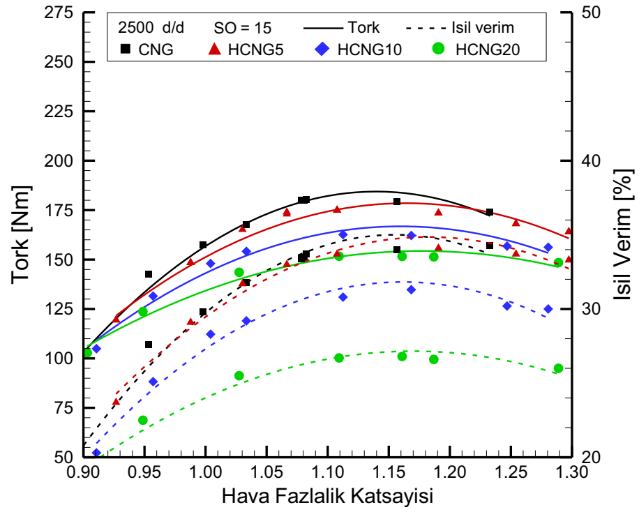
Şekil 3.31. Farklı HCNG yakıtları için hava fazlalık katsayısına göre tork ve ısı verim değerleri (2500 d/d, SO=15).
