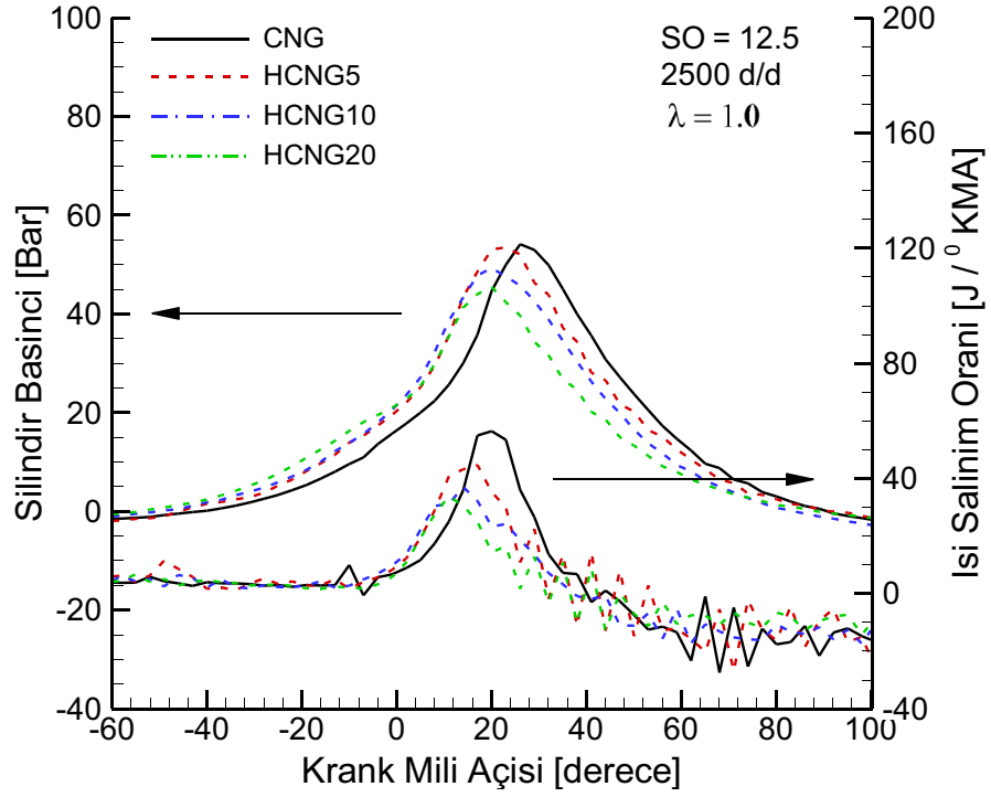
Şekil 3.45. Stokiyometrik şartlarda hidrojen ilavesinin silindir basıncına ve ısı salınım oranına etkisi (SO=12.5, 2500 d/d).
