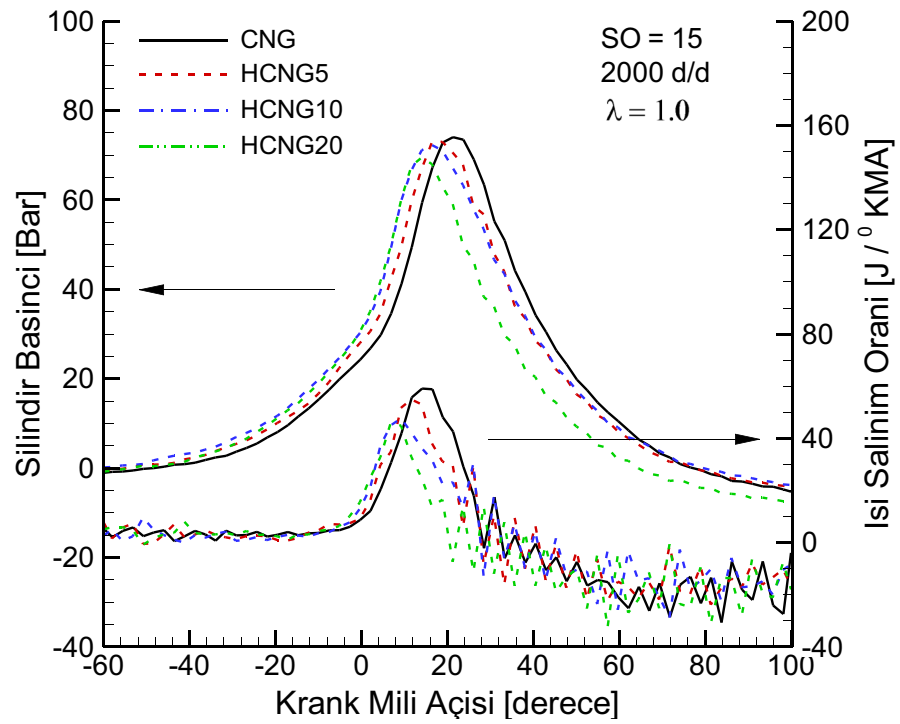
Şekil 3.48. Stokiyometrik şartlarda hidrojen ilavesinin silindir basıncına ve ısı salınım oranına etkisi (SO=15, 2000 d/d).
