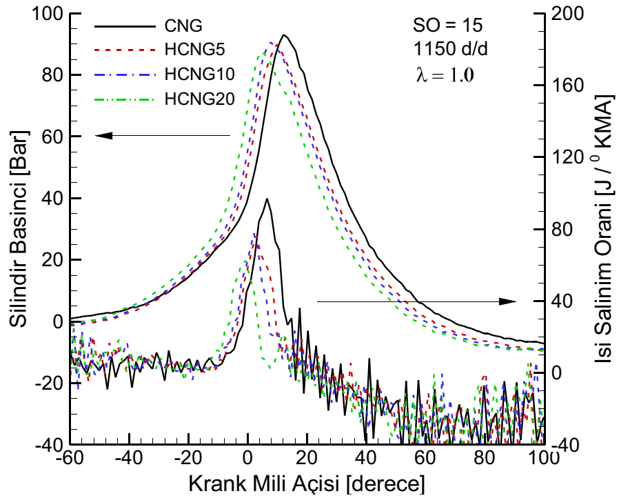
Şekil 3.46. Stokiyometrik şartlarda hidrojen ilavesinin silindir basıncına ve ısı salınım oranına etkisi (SO=15, 1150 d/d).
