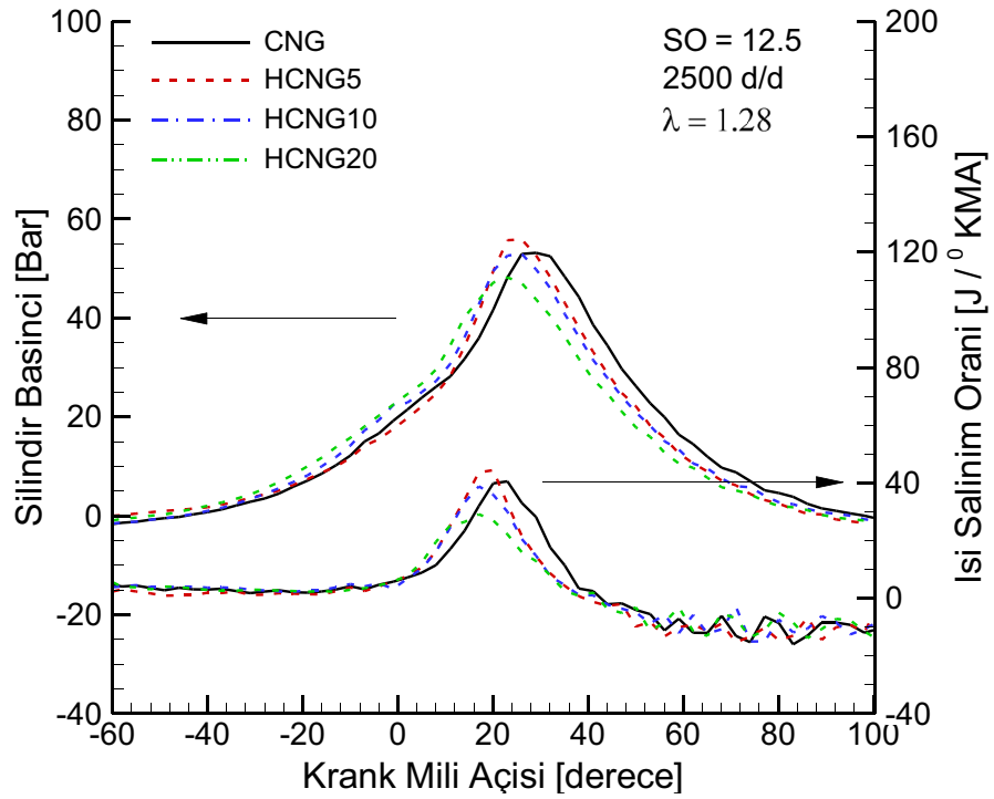
Şekil 3.53. \lambda=1.28 değerinde hidrojen ilavesinin silindir basıncına ve ısı salınım oranına etkisi ( SO=12.5 , 2500 \text{ d/d} ).
