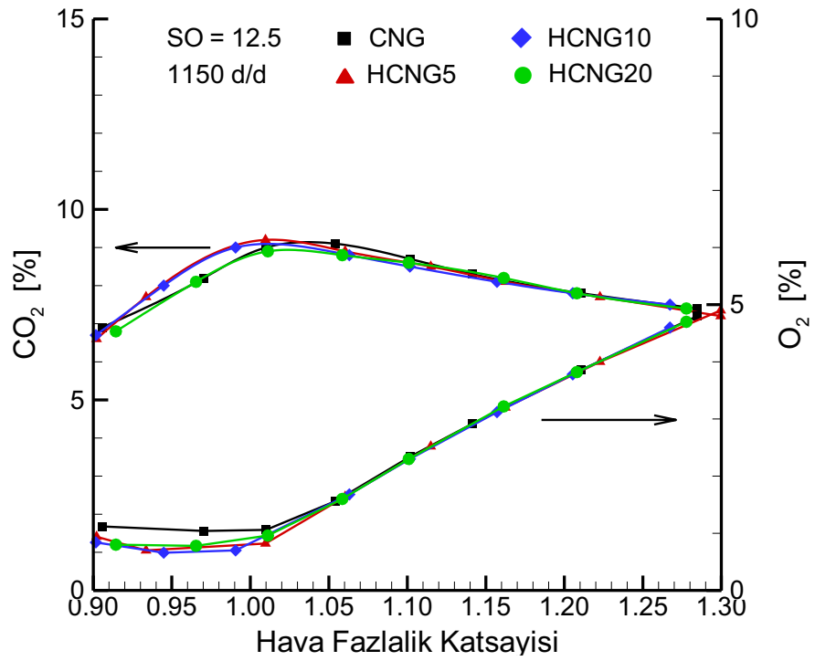
Şekil 3.75. 12.5 sıkıştırma oranında ve 1150 d/d motor devrinde hidrojen ilavesinin CO 2 ve O 2 emisyonlarına etkisi.
