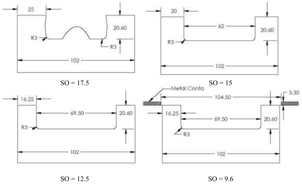
Şekil 2.3. Farklı sıkıştırma oranlarında piston şekilleri (mm).
