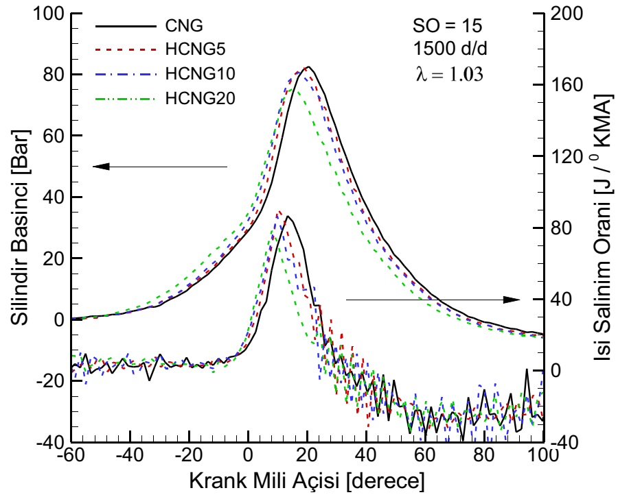
Şekil 3.47. Stokiyometrik şartlarda hidrojen ilavesinin silindir basıncına ve ısı salınım oranına etkisi (SO=15, 1500 d/d).
