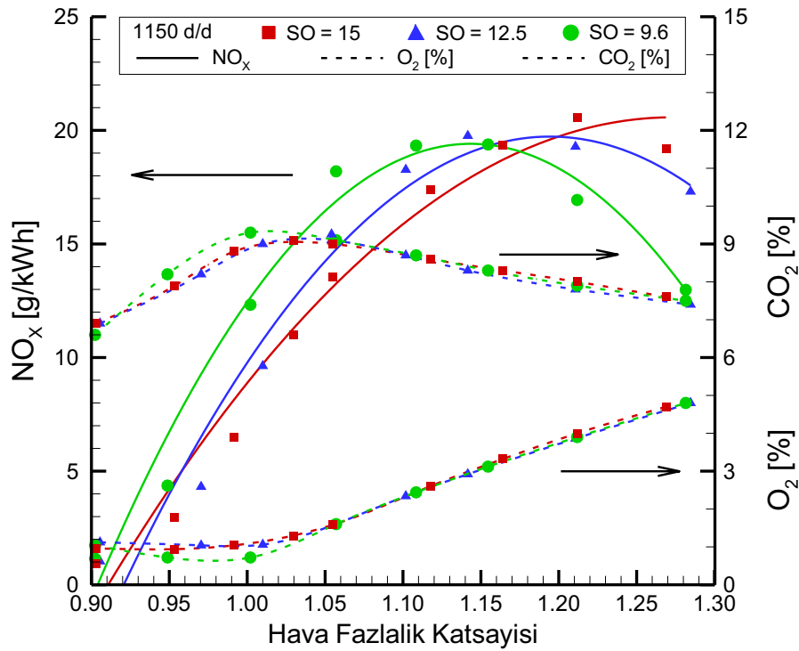
Şekil 3.18. Farklı sıkıştırma oranlarında ve 1150 d/d motor devrinde hava fazlalık katsayısına göre \text{NO}_x , \text{O}_2 ve \text{CO}_2 değerleri.
