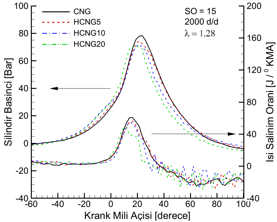
Şekil 3.55. \lambda=1.28 değerinde hidrojen ilavesinin silindir basıncına ve ısı salınım oranına etkisi (SO=15, 2000 d/d).
