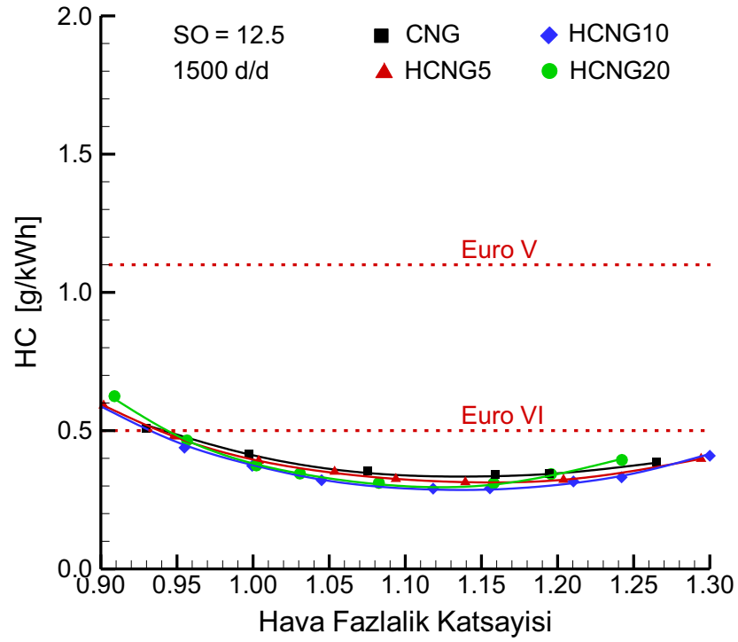
Şekil 3.57. 12.5 sıkıştırma oranında ve 1500 d/d motor devrinde hidrojen ilavesinin HC emisyonlarına etkisi.
