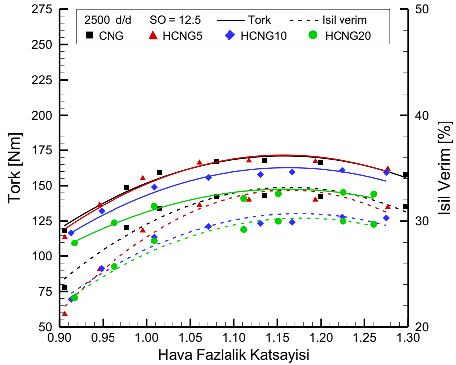
Şekil 3.32. Farklı HCNG yakıtları için hava fazlalık katsayısına göre tork ve ısı verim değerleri (2500 d/d, SO=12.5).
