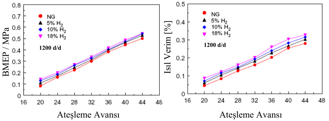
Şekil 1.4. Farklı ateşleme zamanlarında hidrojen ilavesinin motor gücüne ve ısı verime etkisi [21].
