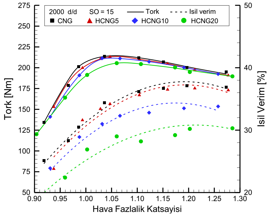
Şekil 3.28. Farklı HCNG yakıtları için hava fazlalık katsayısına göre tork ve ısı verim değerleri (2000 d/d, SO=15).
