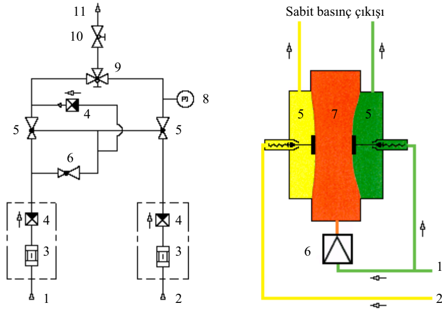
1- CNG gazı (pilot gaz) 2- H 2 gazı 3- Filtre 4- Check valf 5- Tek kubbeli basınç regülatörü 6- Pilot gaz regülatörü 7- Çift kubbeli basınç regülatörü 8- Gösterge 9- Oransal karışım valfi 10- Gaz akış valfi 11-Ayarlanmış HCNG gazı
