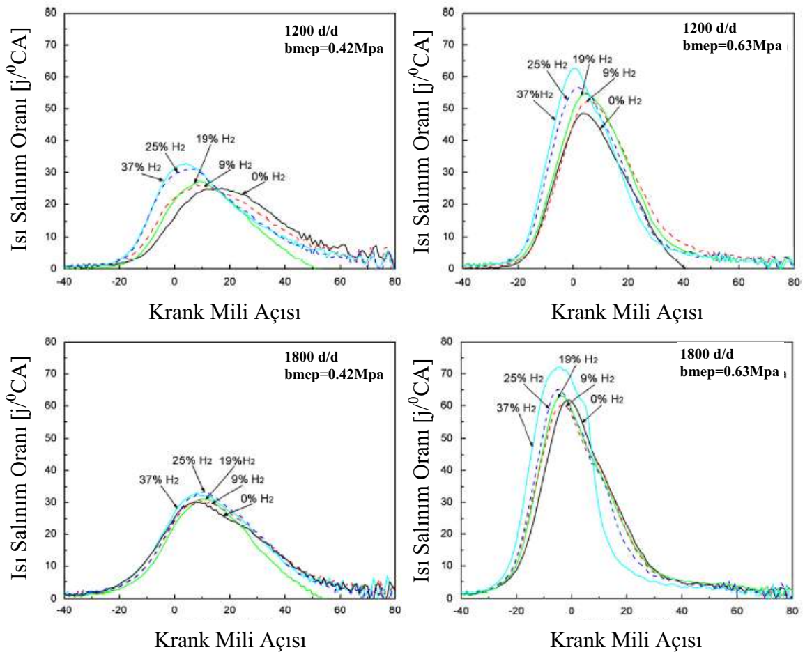
Şekil 1.11. Farklı güç değerlerinde hidrojen ilavesinin ısıl salınım oranına etkisi [25].
