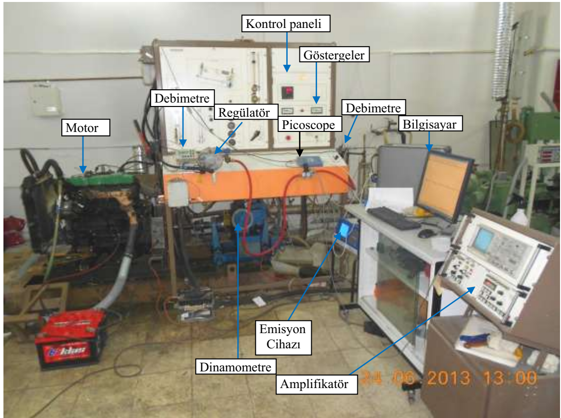
řekil 2.10. Deney düzeneđinde yer alan komponentler.
