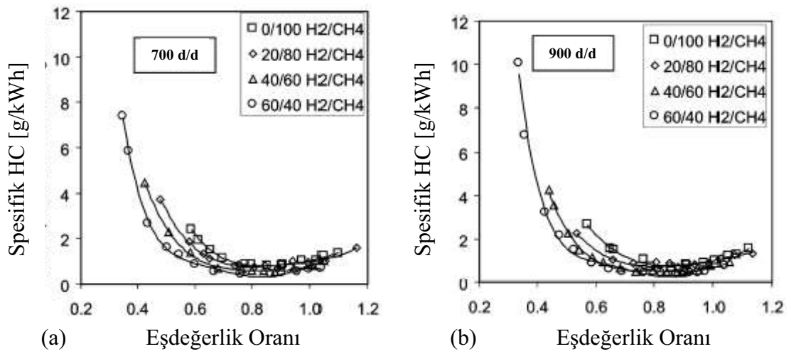
Şekil 1.9. Farklı hava-yakıt oranlarında hidrojen ilavesinin HC emisyonlarına etkisi [24].
