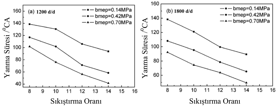
Şekil 1.3. Farklı güç ve devirlerde sıkıştırma oranının yanma süresine etkisi [10].
