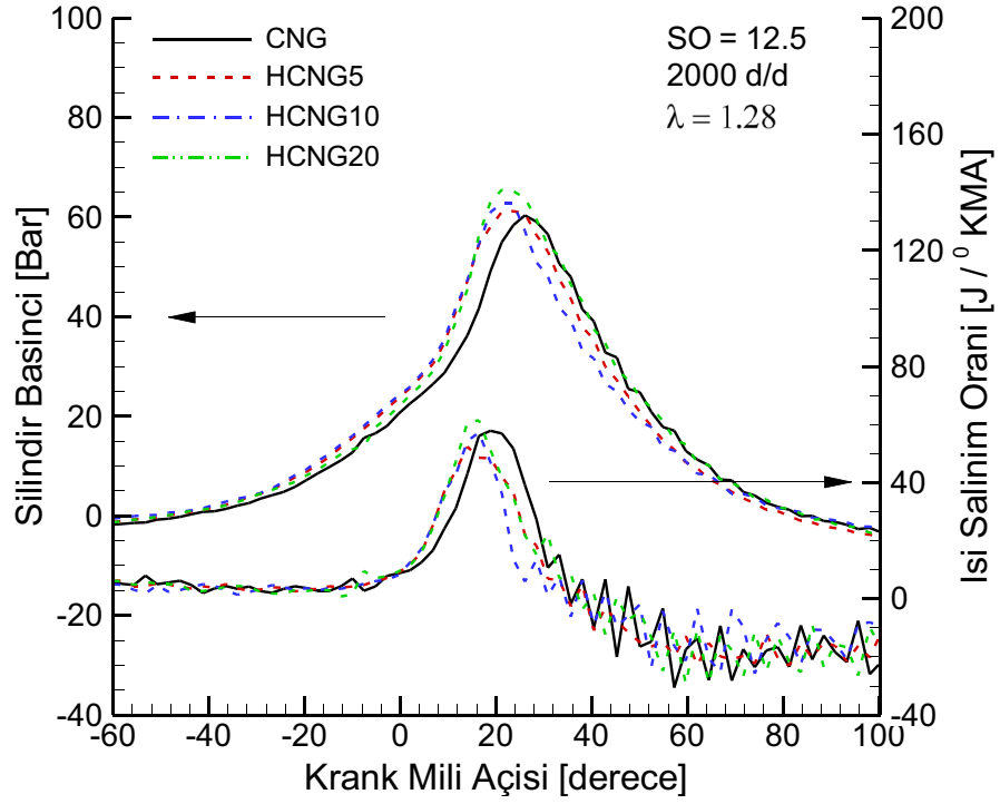
Şekil 3.52. \lambda=1.28 değerinde hidrojen ilavesinin silindir basıncına ve ısı salınım oranına etkisi ( SO=12.5 , 2000 \text{ d/d} ).
