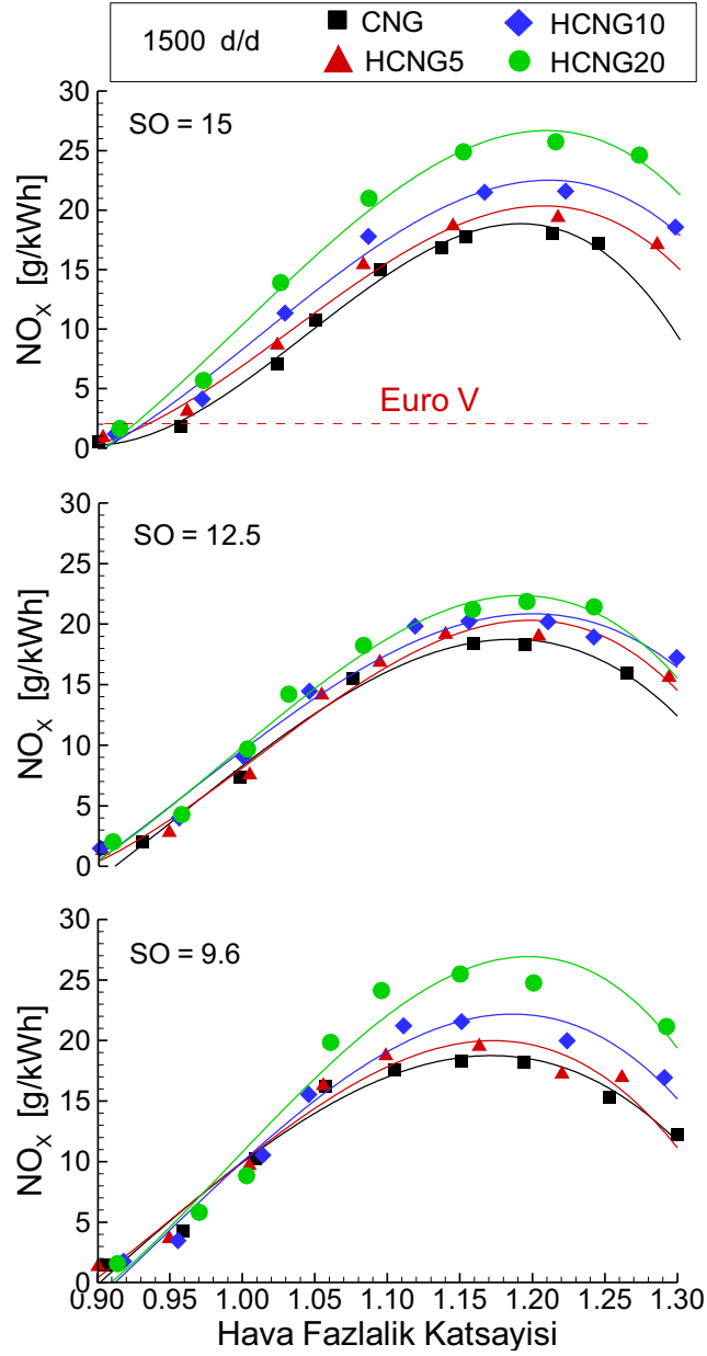
Şekil 3.69. Farklı sıkıştırma oranında ve 1500 d/d motor devrinde hidrojen ilavesinin \text{NO}_x emisyonlarına etkisi.
