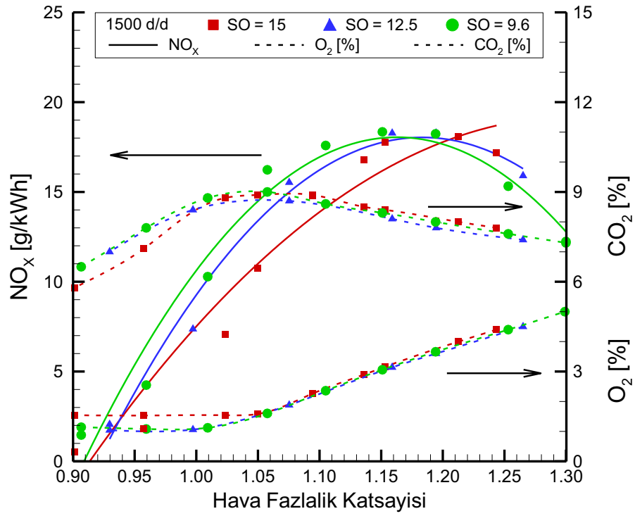
Şekil 3.19. Farklı sıkıştırma oranlarında ve 1500 d/d motor devrinde hava fazlalık katsayısına göre NO x , O 2 ve CO 2 değerleri.
