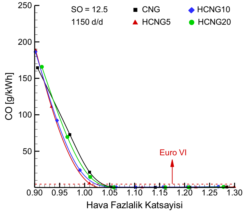
Şekil 3.65. 12.5 sıkıştırma oranında ve 1150 d/d motor devrinde hidrojen ilavesinin CO emisyonlarına etkisi.
