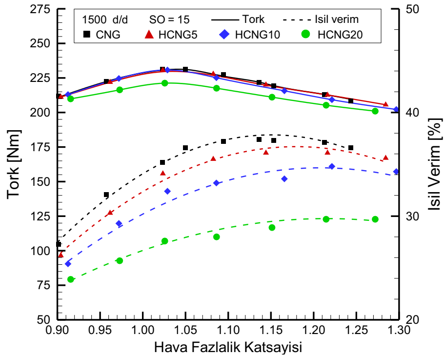
Şekil 3.25. Farklı HCNG yakıtları için hava fazlalık katsayısına göre tork ve ısı verim değerleri (1500 d/d, SO=15).
