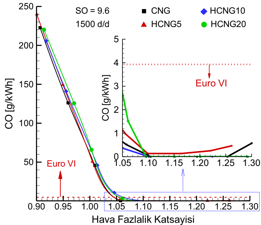
Şekil 3.62. 9.6 sıkıştırma oranında ve 1500 d/d motor devrinde hidrojen ilavesinin CO emisyonlarına etkisi.
