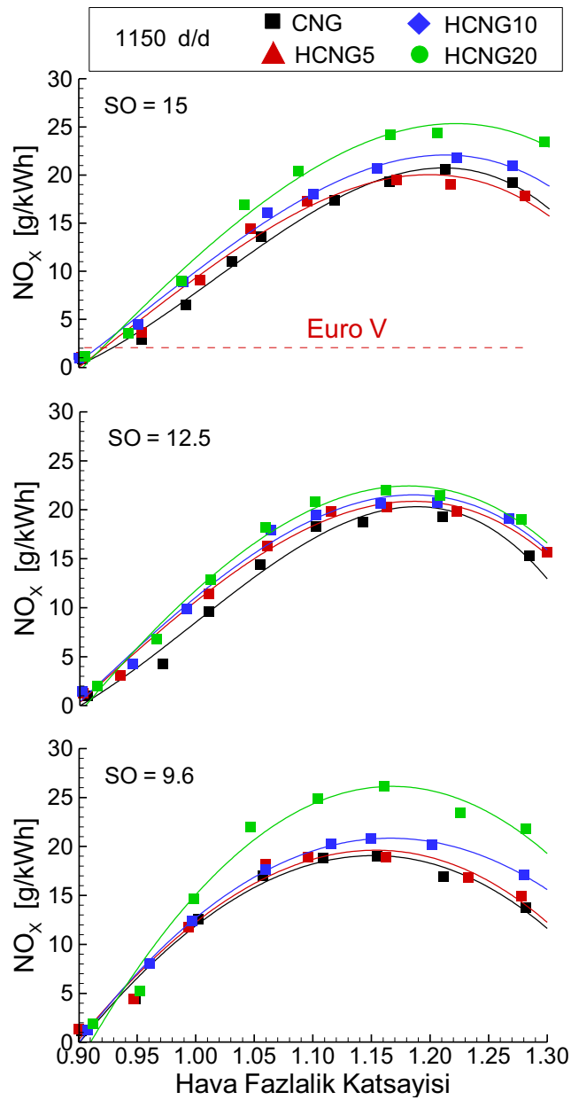
Şekil 3.68. Farklı sıkıştırma oranında ve 1150 d/d motor devrinde hidrojen ilavesinin \text{NO}_x emisyonlarına etkisi.
