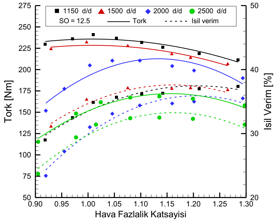
Şekil 3.2. SO=12.5 sıkıştırma oranında ve farklı motor devirlerinde hava fazlalık katsayısına göre tork ve ısı verim değerleri.
