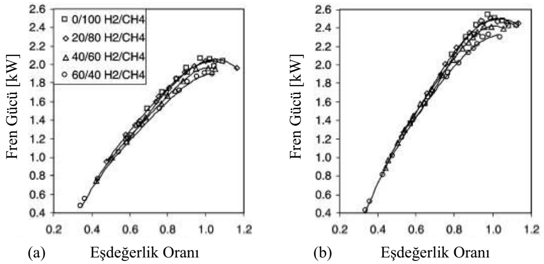
Şekil 1.7. Farklı hava-yakıt oranlarında hidrojen ilavesinin motor fren gücüne etkisi [24].
