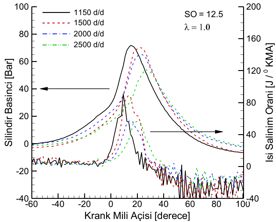
Şekil 3.9. Değişik motor devirlerinde krank mili açısına göre silindir basıncı ve ısı salınım oranlarının değişimi (SO=12.5, \lambda=1.0 ).
