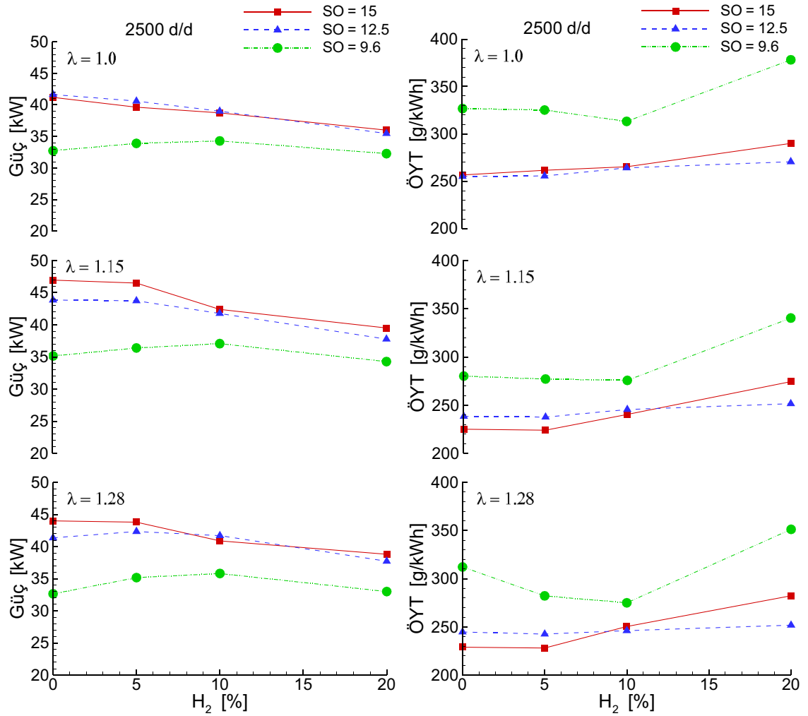
Şekil 3.37. Farklı sıkıştırma oranlarında \lambda=1.0 , \lambda=1.15 ve \lambda=1.28 değerleri için hidrojen ilavesinin motor gücü ve özgül yakıt tüketimine etkisi (2500 d/d).
