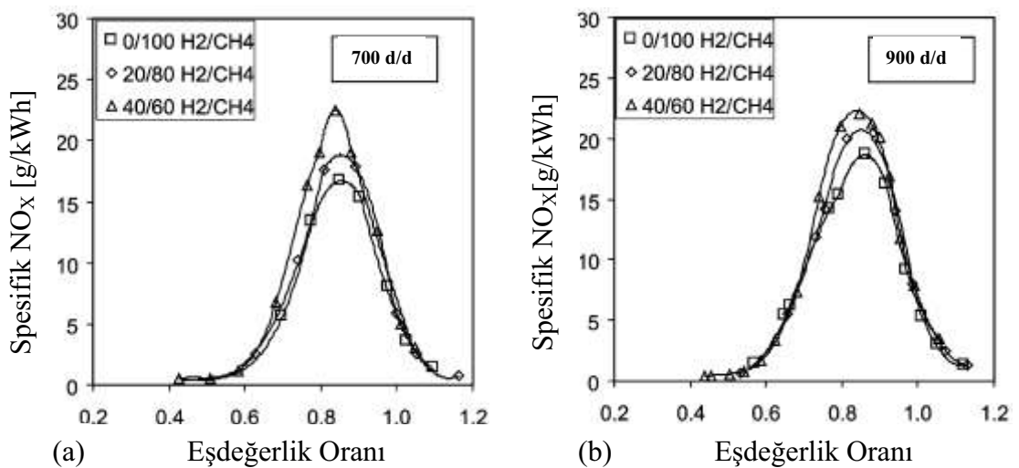
Şekil 1.10. Farklı hava-yakıt oranlarında hidrojen ilavesinin \text{NO}_x değerlerine etkisi [24].
