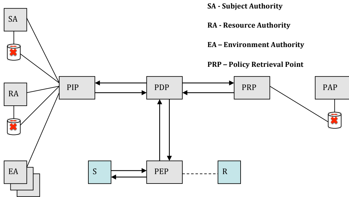
Şekil 2.1 Yetkilendirme Mimarisi [85]
