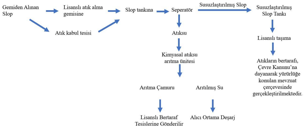
Şekil 3.7 Atık Kabul Tesisine Slop Kabulü ve Gönderimine Ait İş Akım Şeması.
