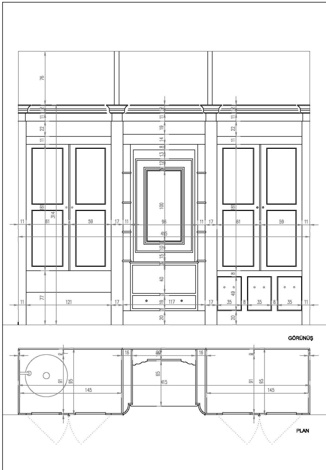
Şekil 3.28. Rölöve 103 numaralı oda dolabı
