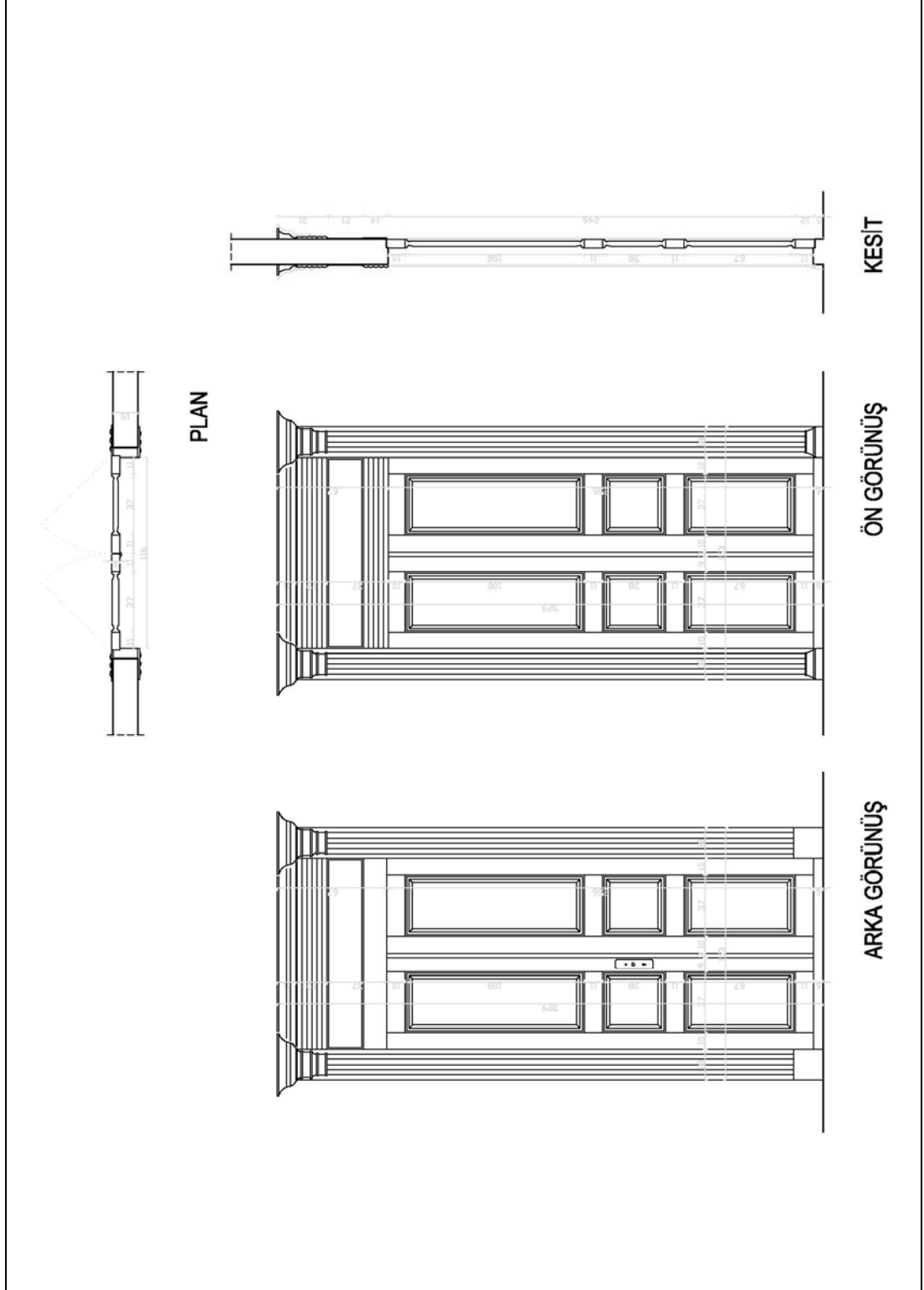
Şekil 3.21. Rölöve K14 kapısı
