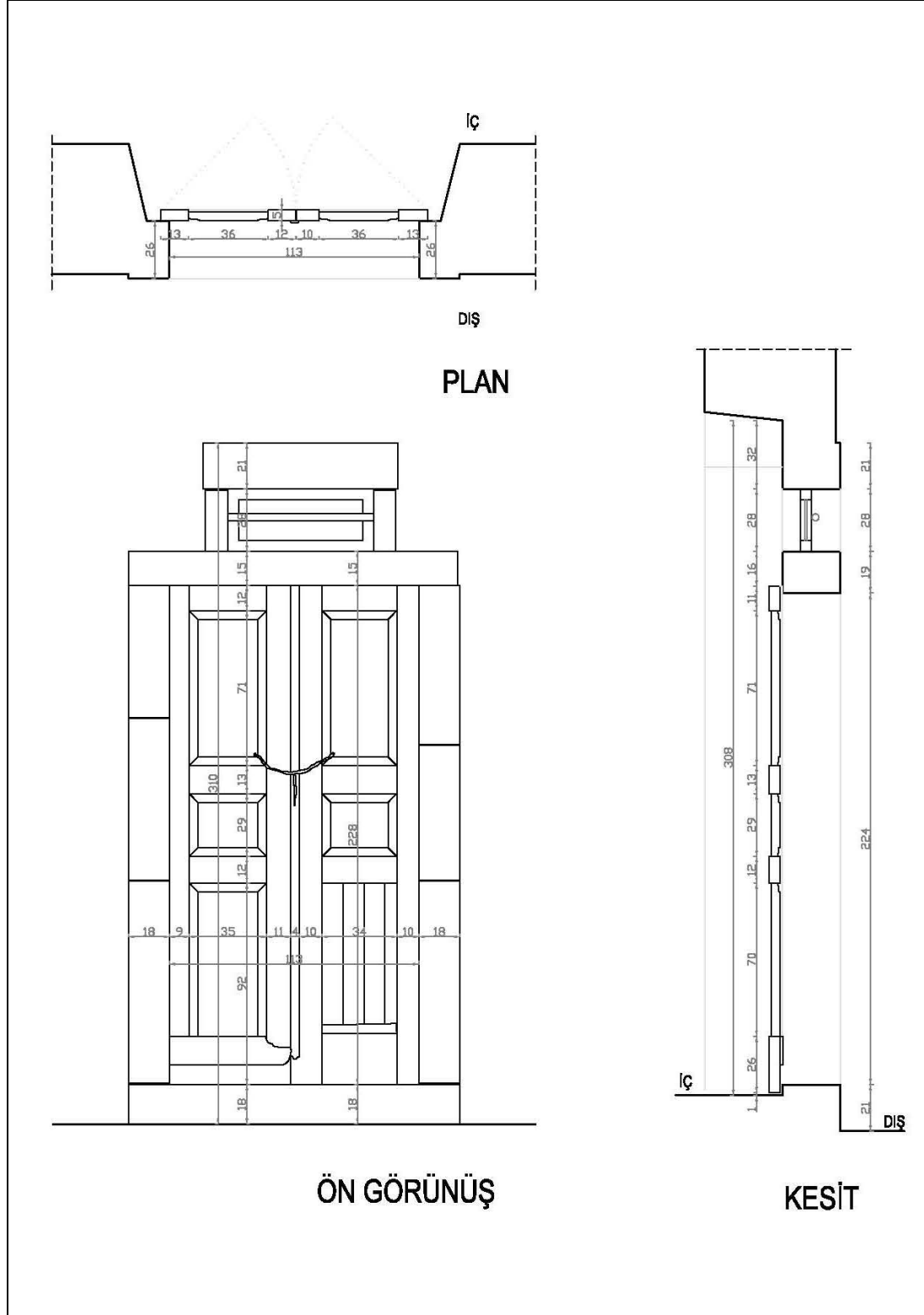
Şekil 3.18. Rölöve K3 kapısı
