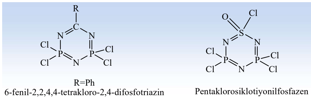
Şekil 1.4. Farklı süstitüent bağlı bileşiklerin adlandırılması.
