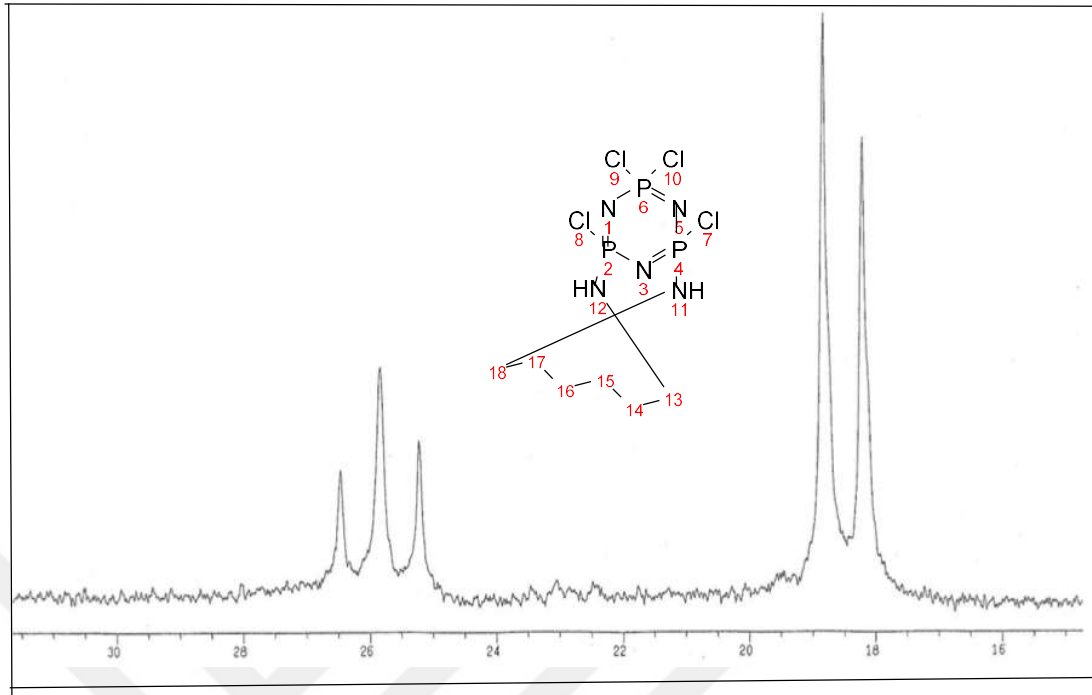
Şekil 3.5. mono-anse bileşiğinin (6), ^{31}\text{P}\{-^1\text{H}\} NMR spektrumu. Oda sıcaklığı, \text{CDCl}_3 içerisinde ve 202.38 MHz de alınmıştır.
