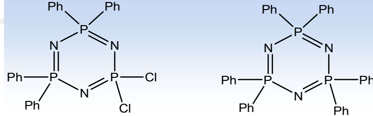
Şekil 1.30. Gem-tetrafenildikloro ve hekzafeñilsiklotrifosfazatrien bileşikleri.
