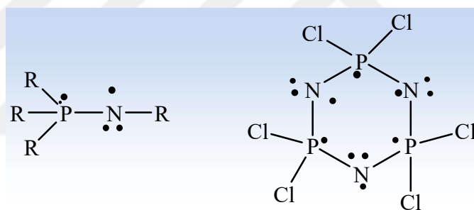
Şekil 1.5. Monofosfazen ve siklotrifosfazenlerdeki P-N bağlanmaları.
