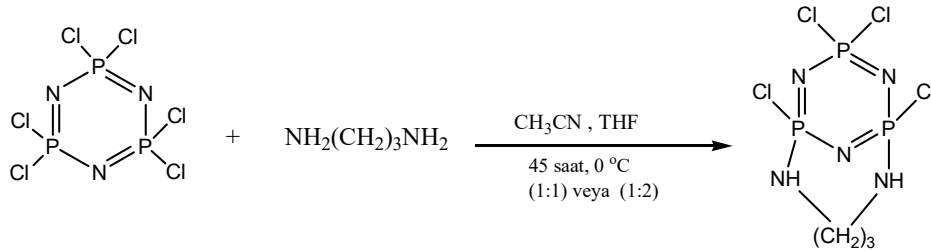
Şekil 2.16. Sikloklorotrifosfazenden 2,4-(1,3-diamin)-tetraklorosiklotrifosfazen’in sentezi.
