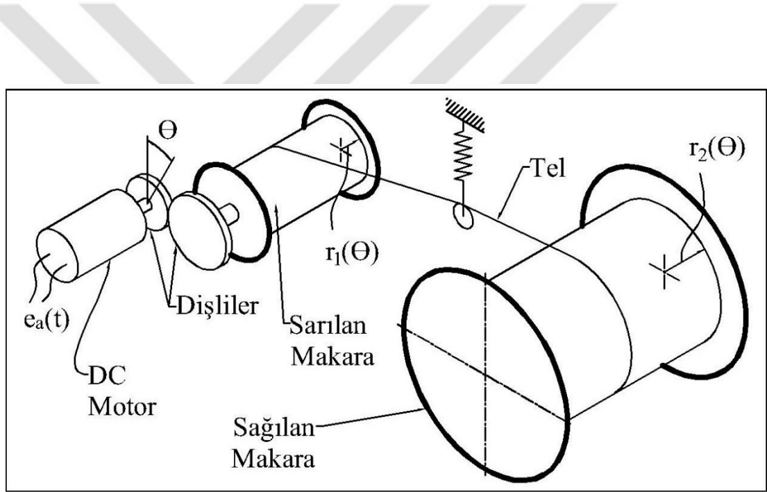
Şekil 3.1. Sarım Sistemi Şematik Görünümü
