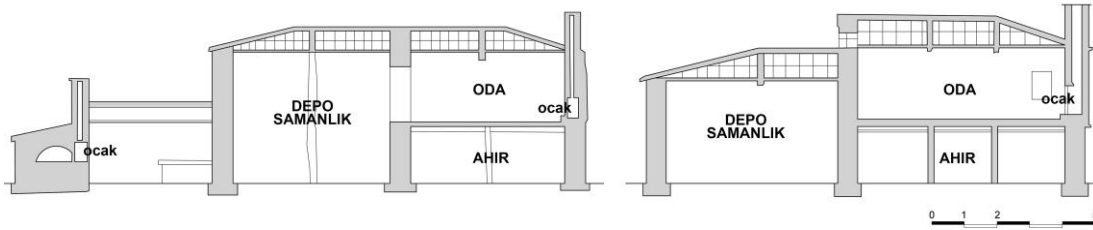
Şekil 2.72 : İki katlı dam örneklerinin kesitleri.
