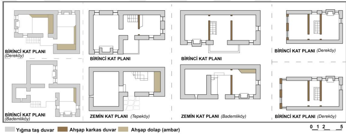
Şekil 2.77 : Eski yapıyla aynı sahanlığı kullanarak (solda) ve merdivenin içeriye alınmasıyla (diğ.) gelişen konut plan tipleri.
