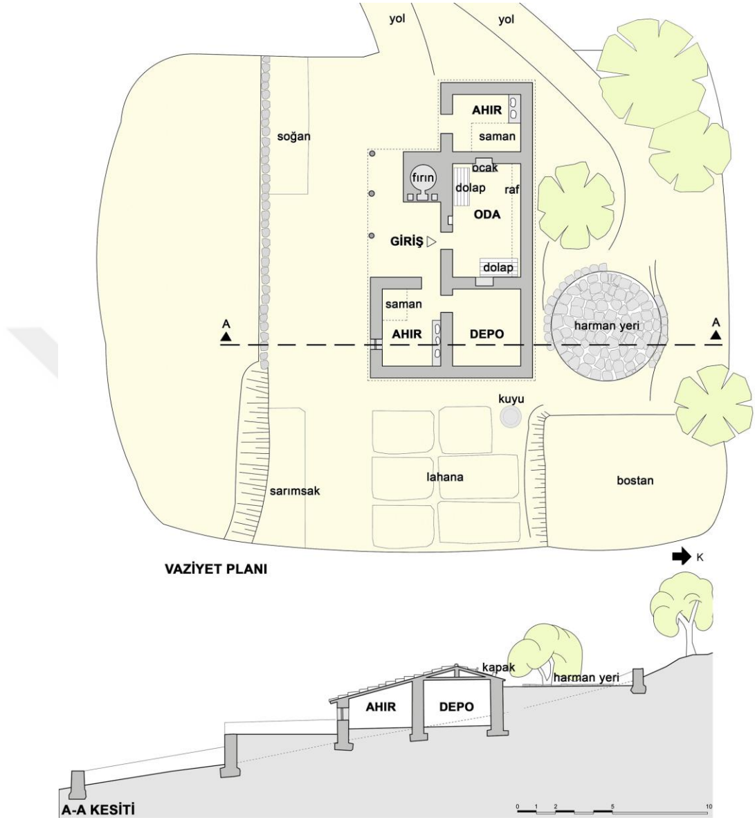
Şekil 2.71 : Dam yapılarına örnek; vaziyet planı ve kesit 30 .
