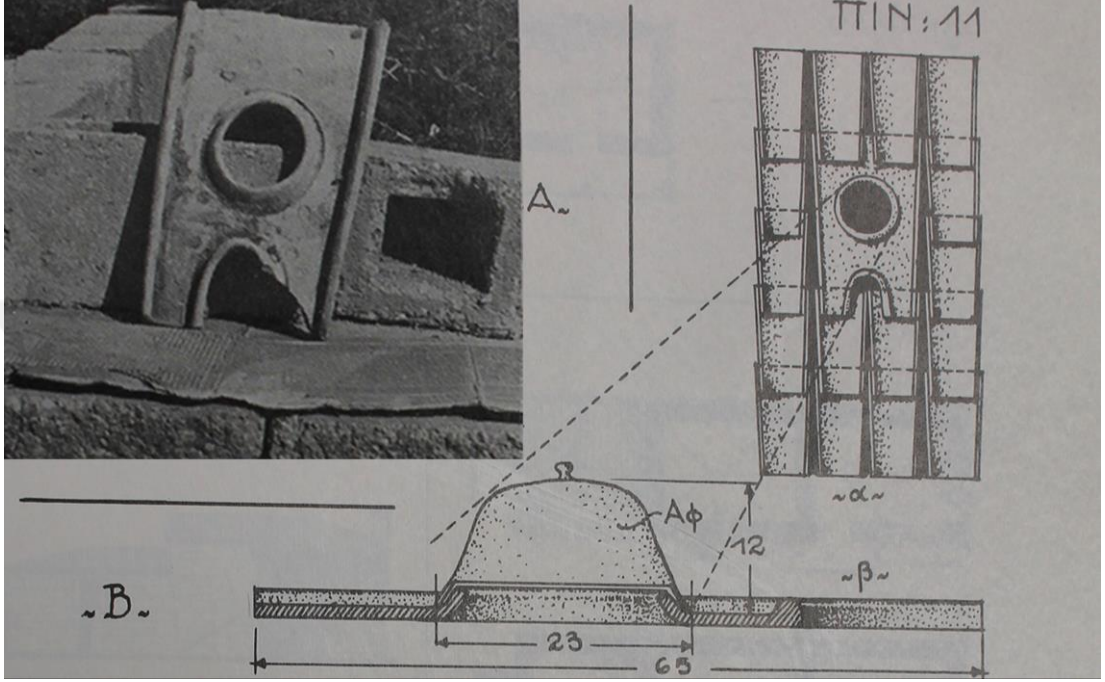
Şekil 2.86 : Çatıda ıslıklık olarak kullanılan kiremitler (Pasadaios, 1973, ss. 92, 102).
