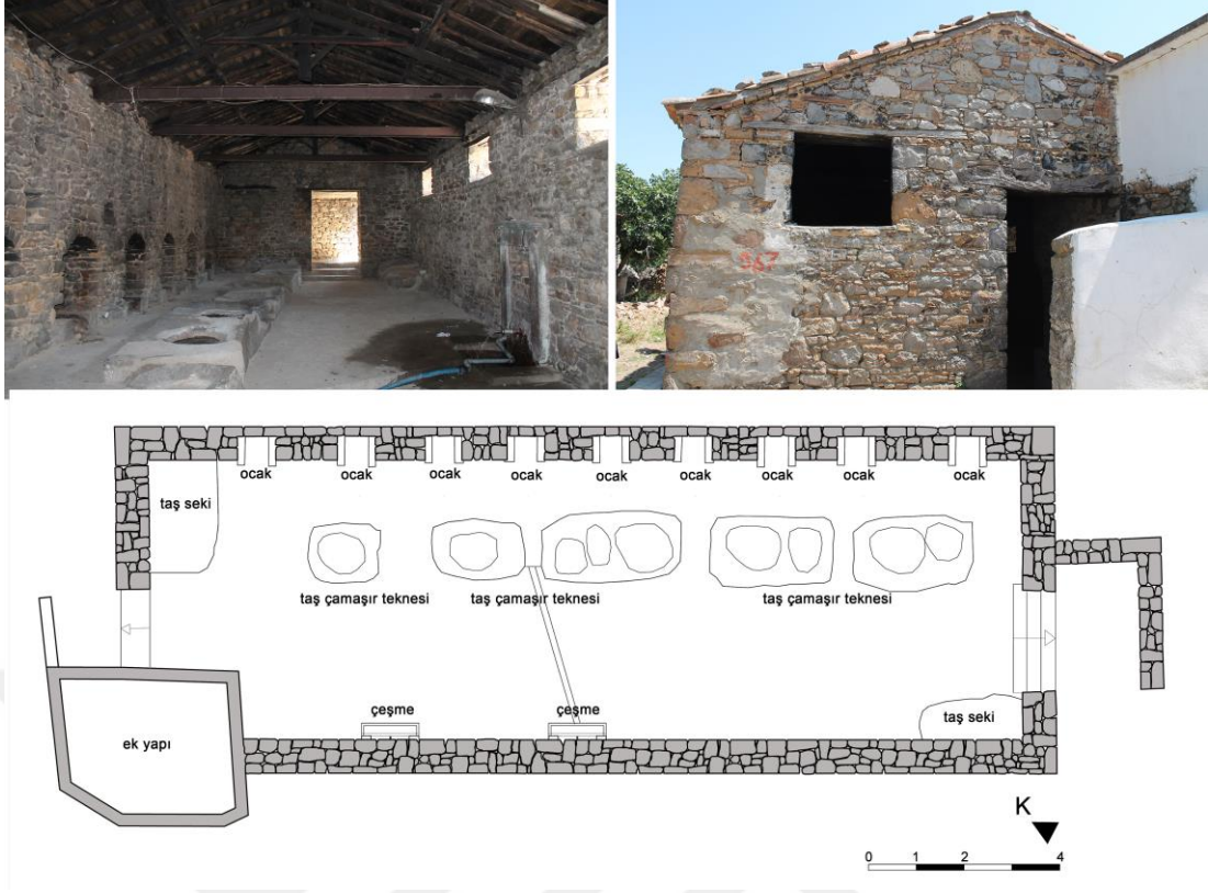
Şekil 2.66 : Dereköy çamaşırhanesi; günümüz fotoğrafları ve planı.
