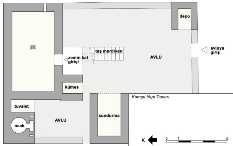
Şekil 2.75 : Avlulu konut plan şeması örneği.
