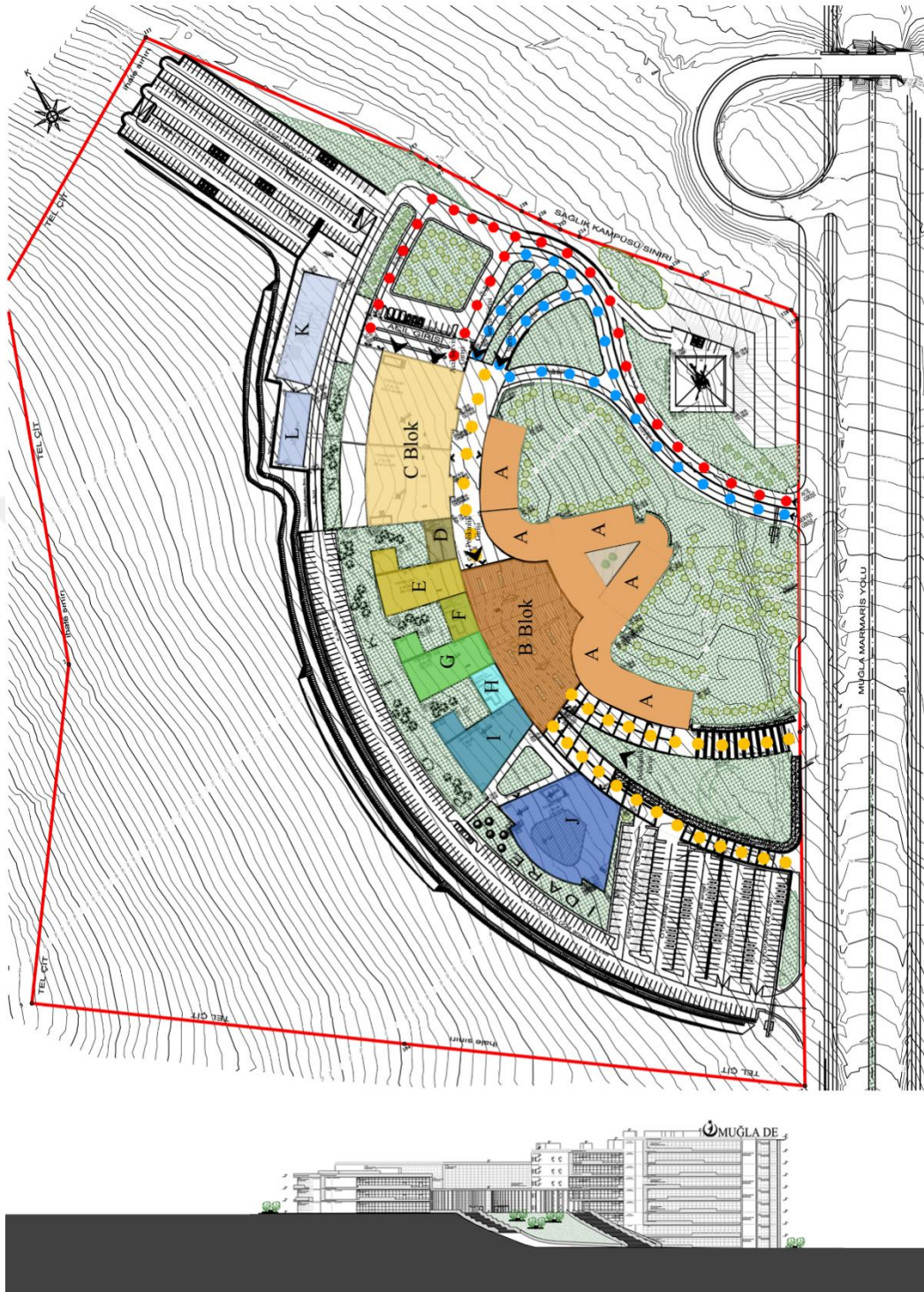
Şekil 4.2. Muğla Sıtkı Koçman Eğitim ve Araştırma Hastanesi vaziyet planı ve arazi kesiti (Aydın 2015)
