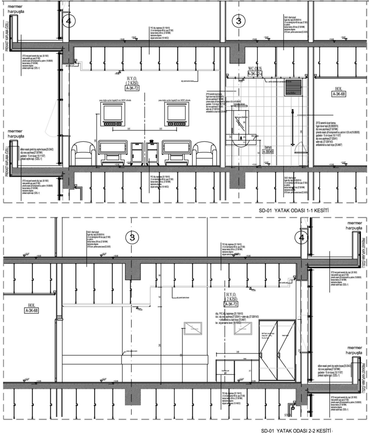
Şekil 4.19. Hasta odası sistem detayı kesiti (Aydın 2015)
