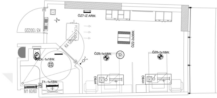
Şekil 4.28. Çift kişilik hasta bakım odası (1.Tip) aydınlatma tasarımı (EMT 2018)
