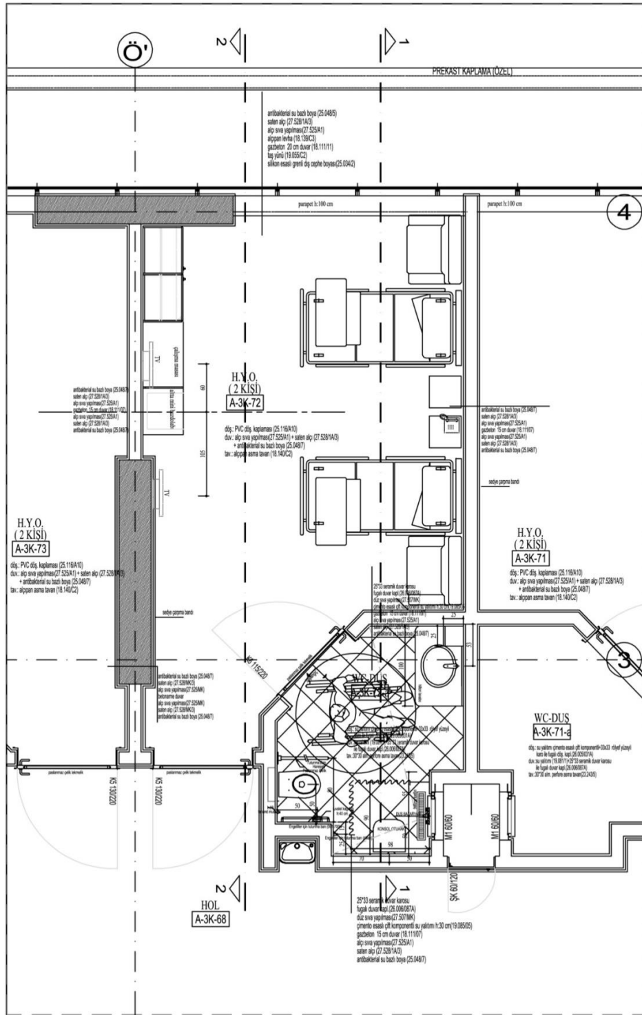
Şekil 4.18. Hasta odası sistem detayı planı (Aydın 2015)
