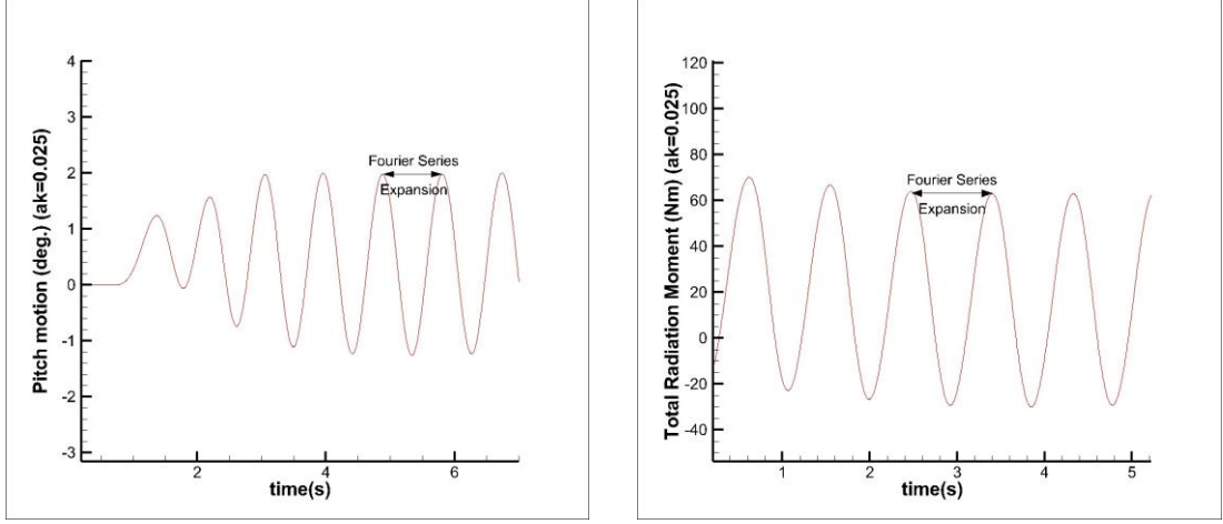
Şekil 4. 3 6.Senaryo için baş-kıç vurma hareketi (URANS) ve baş-kıç vurma radyasyon momenti (URANS-Katsayı) zaman cevabı
