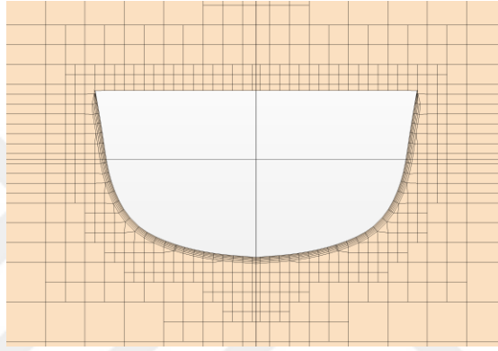
Şekil 2. 14 x/L=0.60 En kesitindeki ağ yapısı
