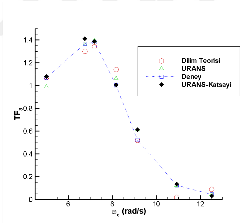
Şekil 4. 1 Dalıp-çıkma TF
