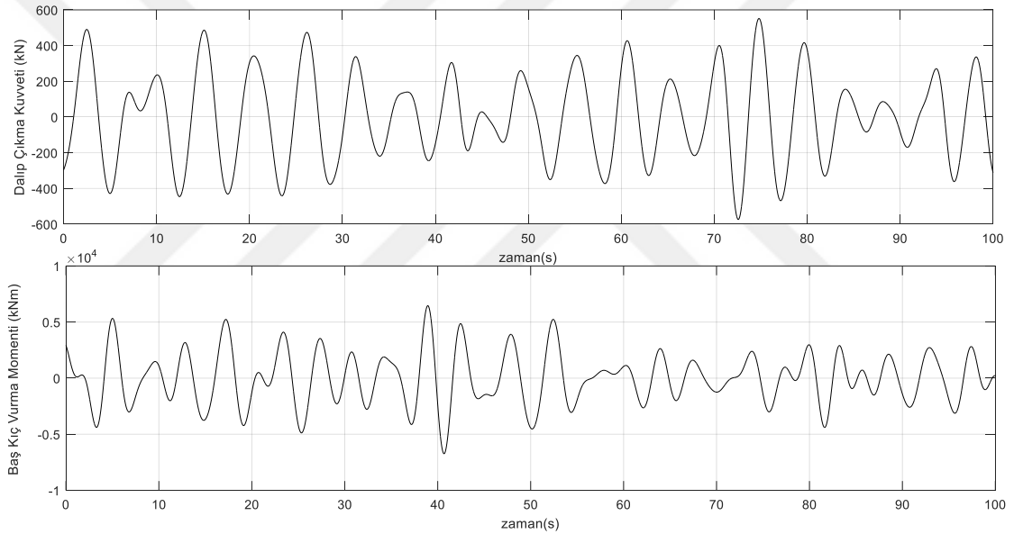
Şekil 3. 8 Dalıp-çıkma kuvveti ve baş-kıç vurma momenti zaman düzlemi cevapları
