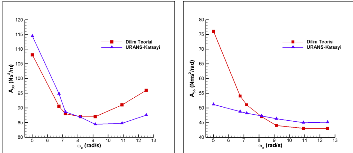
Şekil 2. 19 Ek kütle karşılaştırması ( A_{33} , A_{55} )
