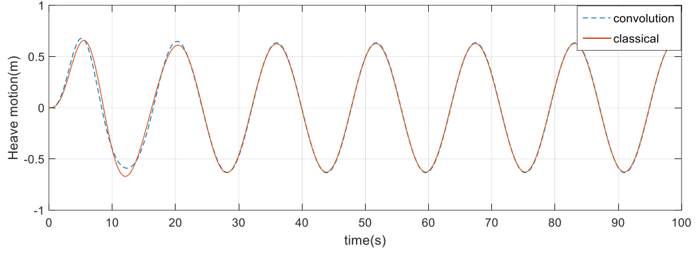
Şekil B. 2 \omega=0.4 rad/s için dalıp-çıkma hareketi zaman cevabı
