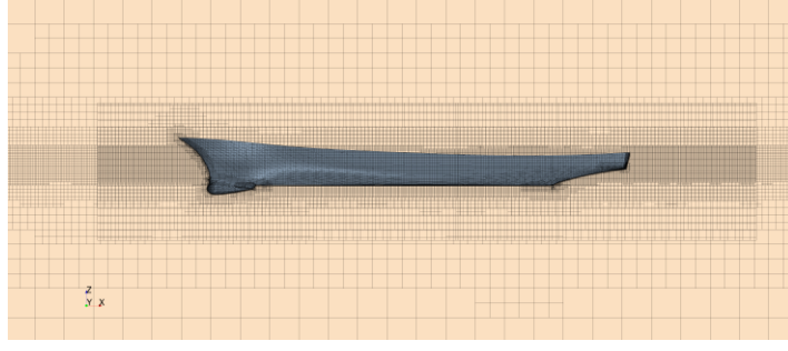
Şekil 2. 13 Tekne etrafındaki ağ yapısı
