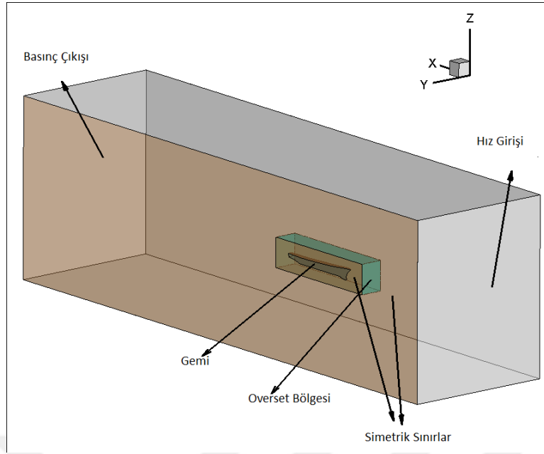
Şekil 2. 12 Dikdörtgen hesaplama hacmi için sınır koşulları
