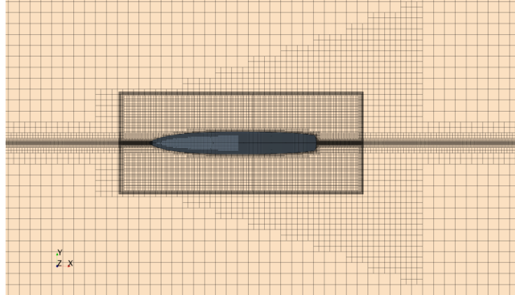
Şekil 2. 15 Kelvin dalga sistemi ile uyumlu ağ yapısı
