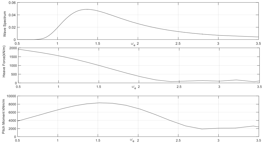
Şekil 3. 6 Karşılaşma dalga spektrumu ve dalıp-çıkma kuvveti/baş-kıç vurma momenti
