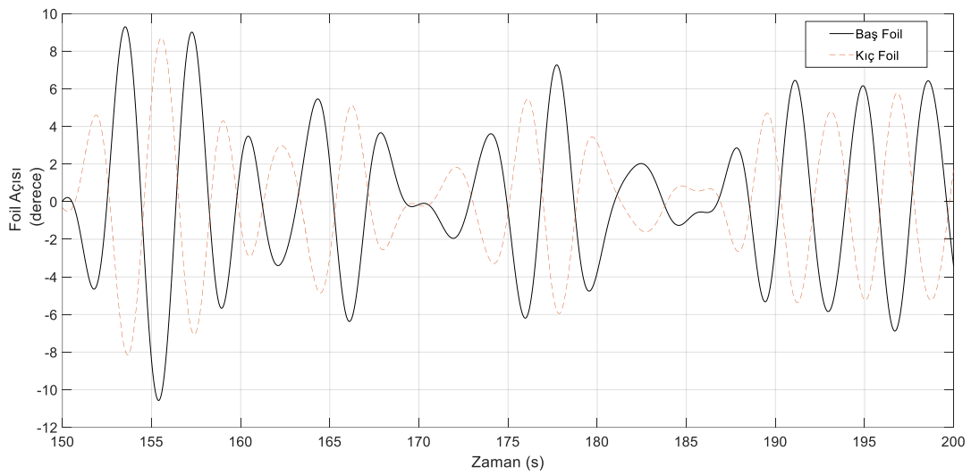
Şekil 3. 17 Baş ve kıç foil hücum açıları
