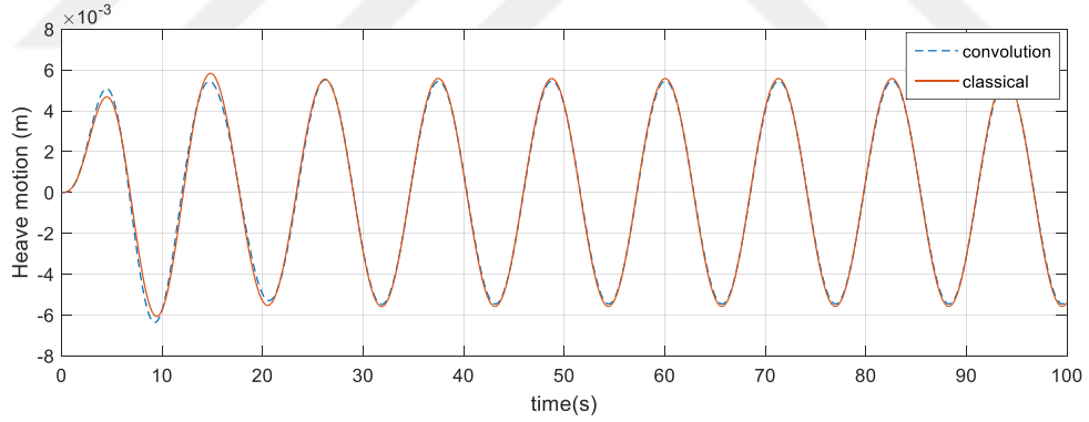
Şekil B. 4 \omega=0.557 rad/s için dalıp-çıkma hareketi zaman cevabı
