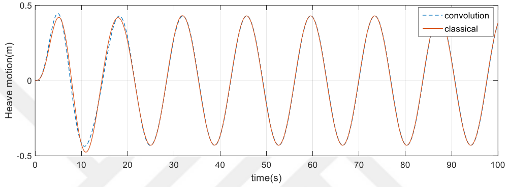
Şekil B. 3 \omega=0.454 rad/s için dalıp-çıkma hareketi zaman cevabı
