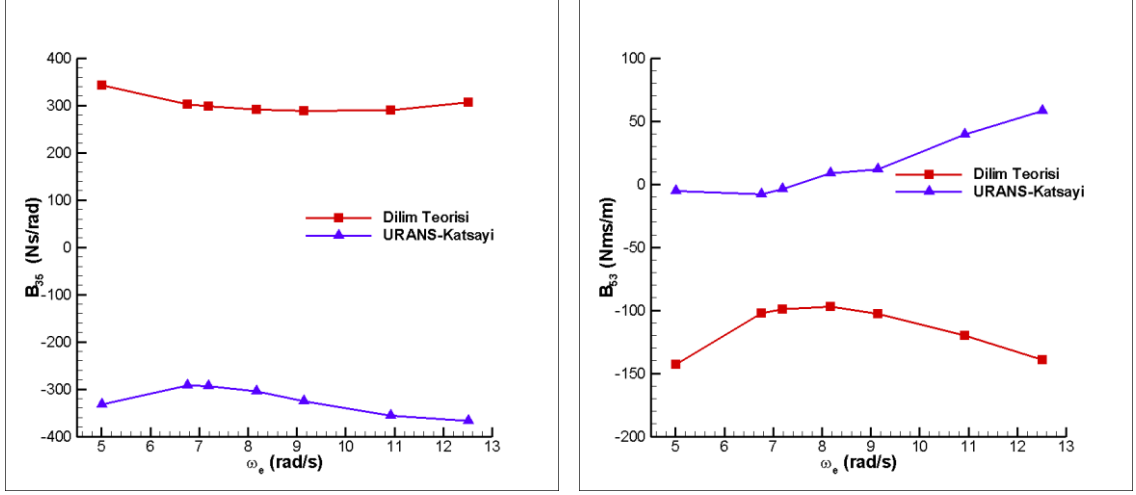
Şekil 2. 22 Sönüm karşılaştırması ( B_{35} , B_{53} ).
