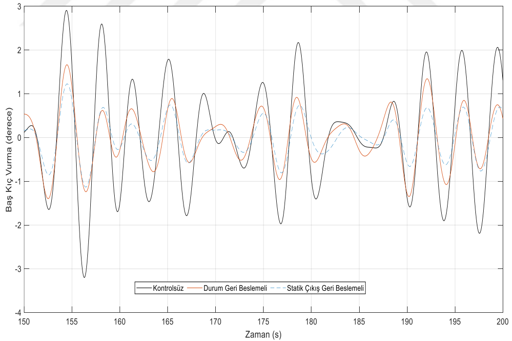
Şekil 3. 12 Gemi baş-kıç vurma hareketi kontrollü ve kontrolsüz cevapları
