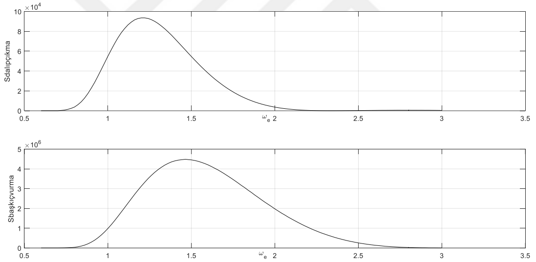
Şekil 3. 7 Dalıp-çıkma kuvveti ve baş-kıç vurma momenti cevap fonksiyonları
