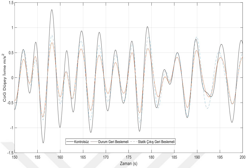
Şekil 3. 15 Gemi orta düşey ivme kontrollü ve kontrolsüz cevapları
