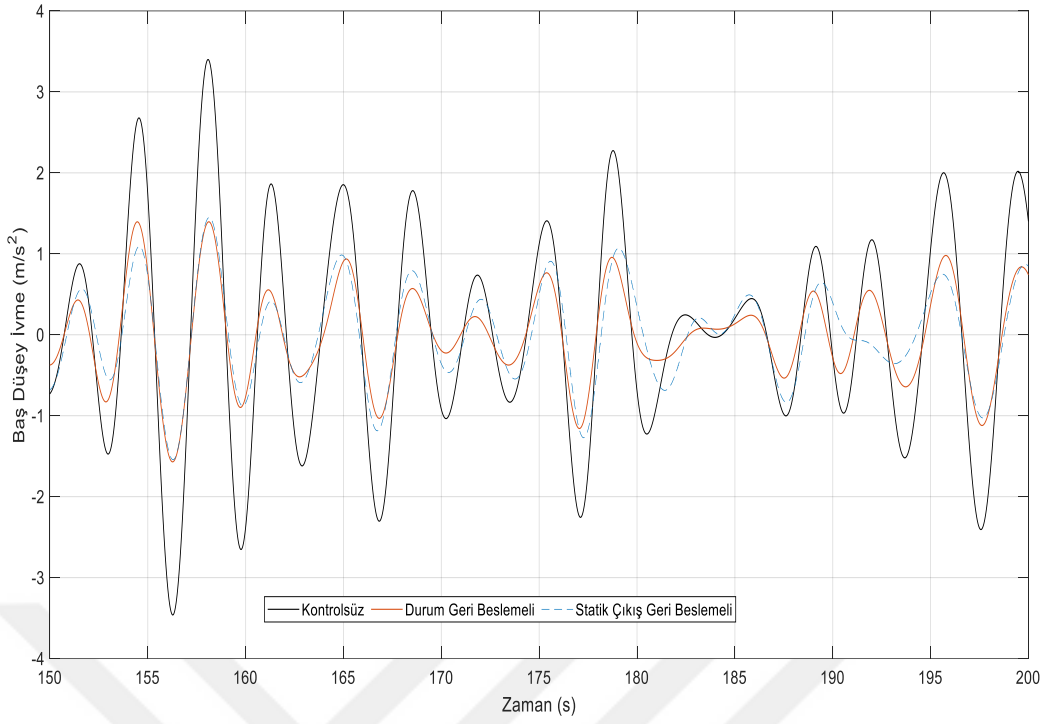
Şekil 3. 13 Gemi baş düşey ivme kontrollü ve kontrolsüz cevapları
