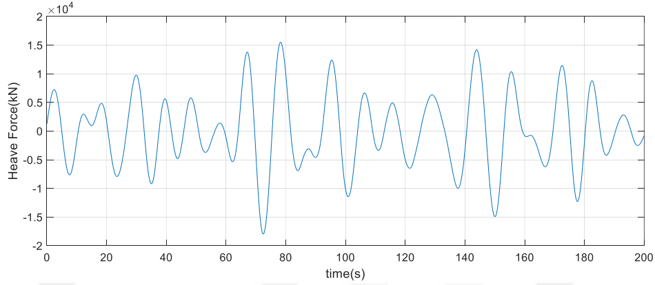
Şekil B. 5 Dalıp-çıkma kuvveti zaman düzlemi cevabı ( H_s=5 m, RMS: 6442 kN)
