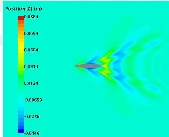
Şekil 2. 18 Zorlanmış dalıp-çıkma hareketi F_n=0.41 ( t=8.3601 s, 9T_E )
