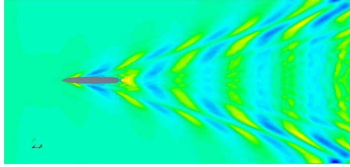
Şekil 2. 16 Kelvin dalga sistemi ( F_n=0.41 )
