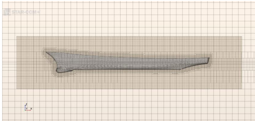
Şekil 2. 8 Profil görünüş ağ yapısı
