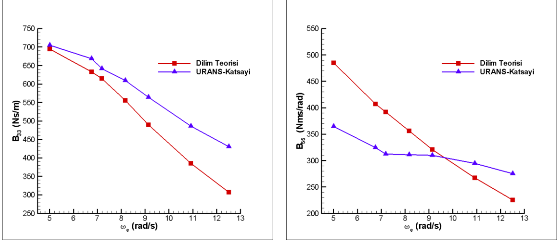
Şekil 2. 20 Sönüm karşılaştırması (B 33 , B 55 )
