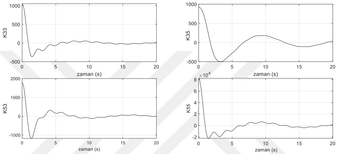
Şekil 3. 5 Elde edilen anlık darbe fonksiyonları
