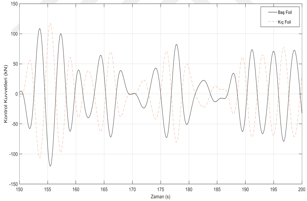
Şekil 3. 16 Gemi baş ve kıç eyleyici kuvvetleri
