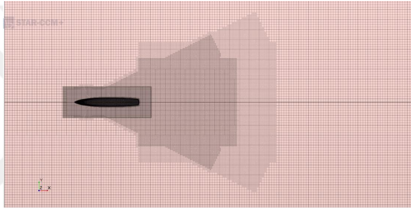
Şekil 2. 7 Serbest su yüzeyi ağ yapısı
