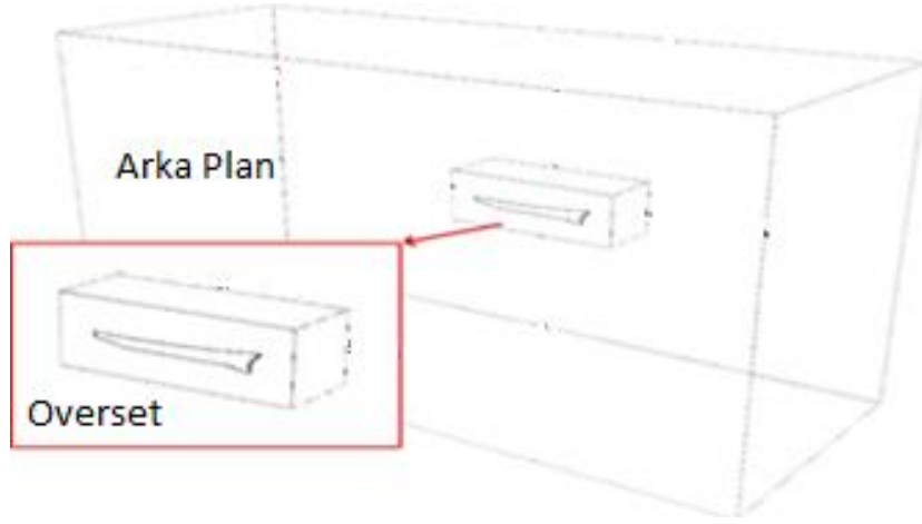
Şekil 2. 6 Overset ve arka plan blokları
