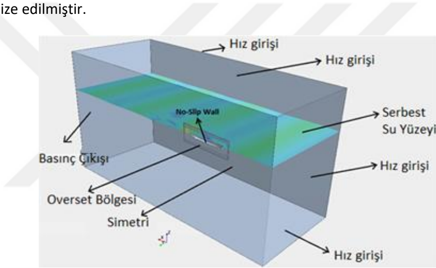
Şekil 2. 4 Sınır koşulları
