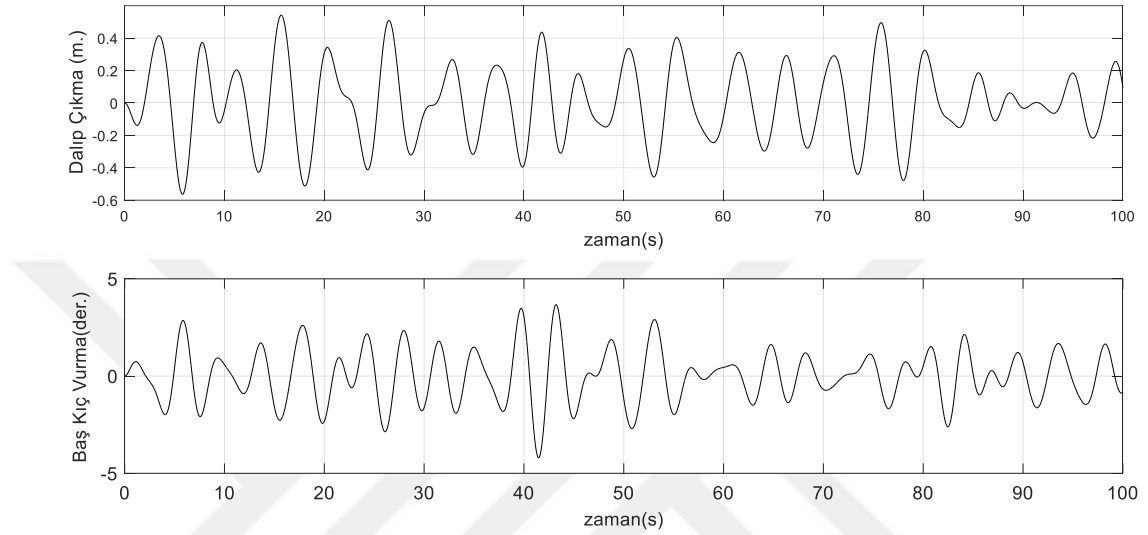
Şekil 3. 9 Dalıp-çıkma ve baş-kıç vurma karışık deniz cevapları( H_S=1m .)
