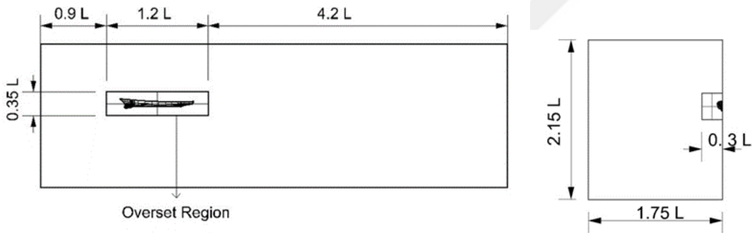
Şekil 2. 5 Hesaplamalı akışkan hacminin boyutları
