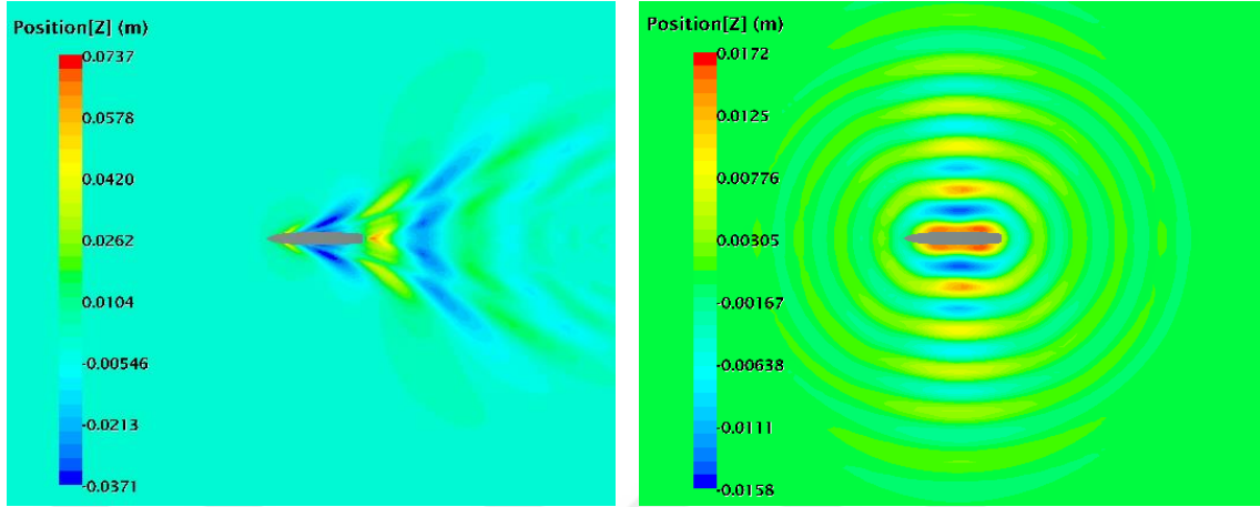
Şekil 2. 17 Kelvin dalga sistemi F_n=0.41 (sol, t=8.3601 s, 9T_E ) ve zorlanmış dalıp-çıkma hareketi F_n=0 (sağ, t=8.3601 s, 9T_E )
