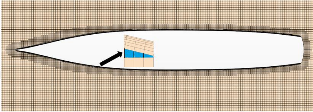
Şekil 2. 10 CFL sayısının hesaplandığı akış bölgesi
