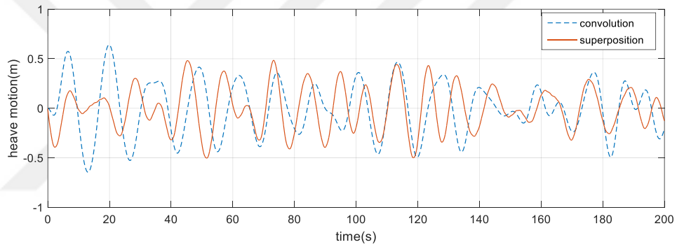
Şekil B. 6 Dalıp-çıkma hareketi zaman düzlemi cevabı ( H_s=5 m)
