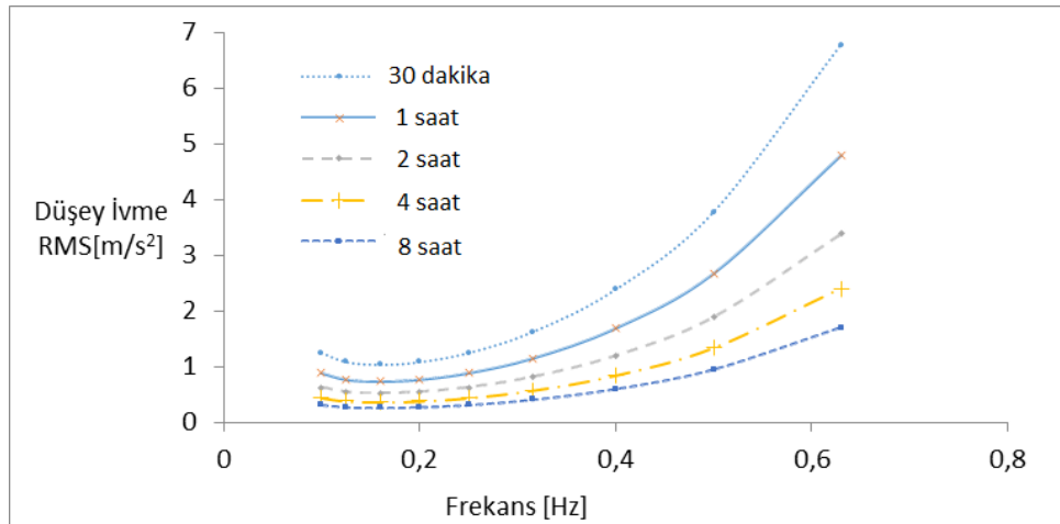
Şekil 3. 10 Farklı maruz kalınan süreler için MSI %10 limit eğrisi
