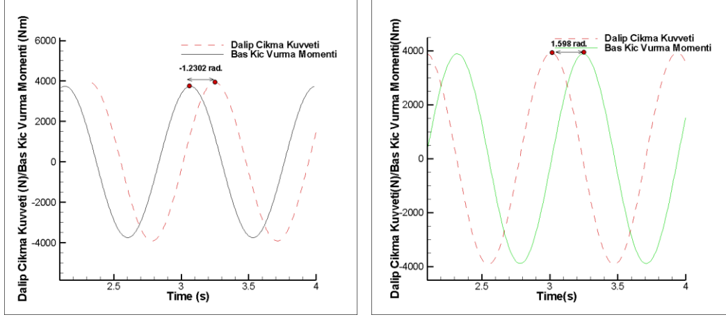
Şekil 2. 23 Zaman düzleminde 6. Senaryo için URANS-Katsayı (sol) ve Dilim teorisi (sağ)
