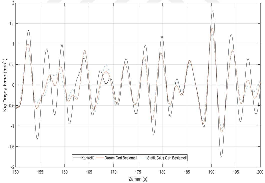
Şekil 3. 14 Gemi kıç düşey ivme kontrollü ve kontrolsüz cevapları
