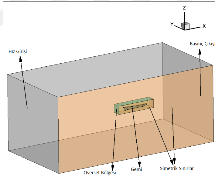
Şekil 2. 11 Kare hesaplama hacmi için sınır koşulları
