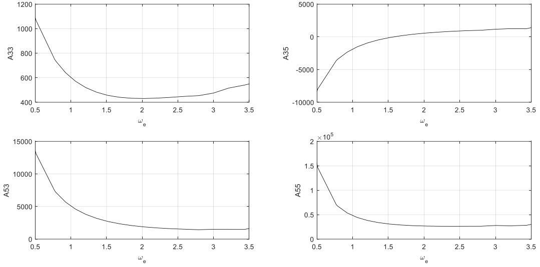
Şekil 3. 3 Ek kütle- \omega_e grafikleri.
