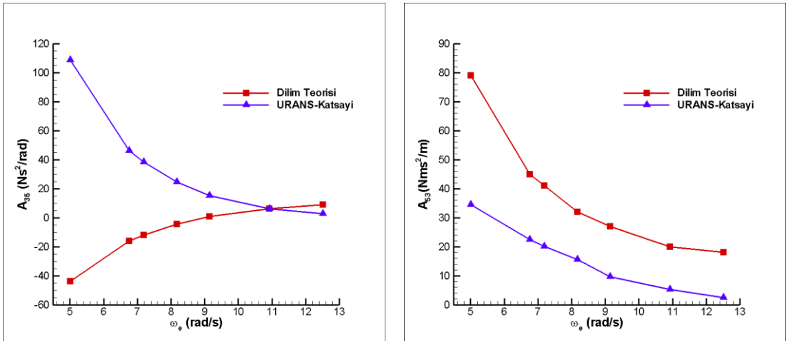
Şekil 2. 21 Ek kütle karşılaştırması (A 35 , A 53 ).
