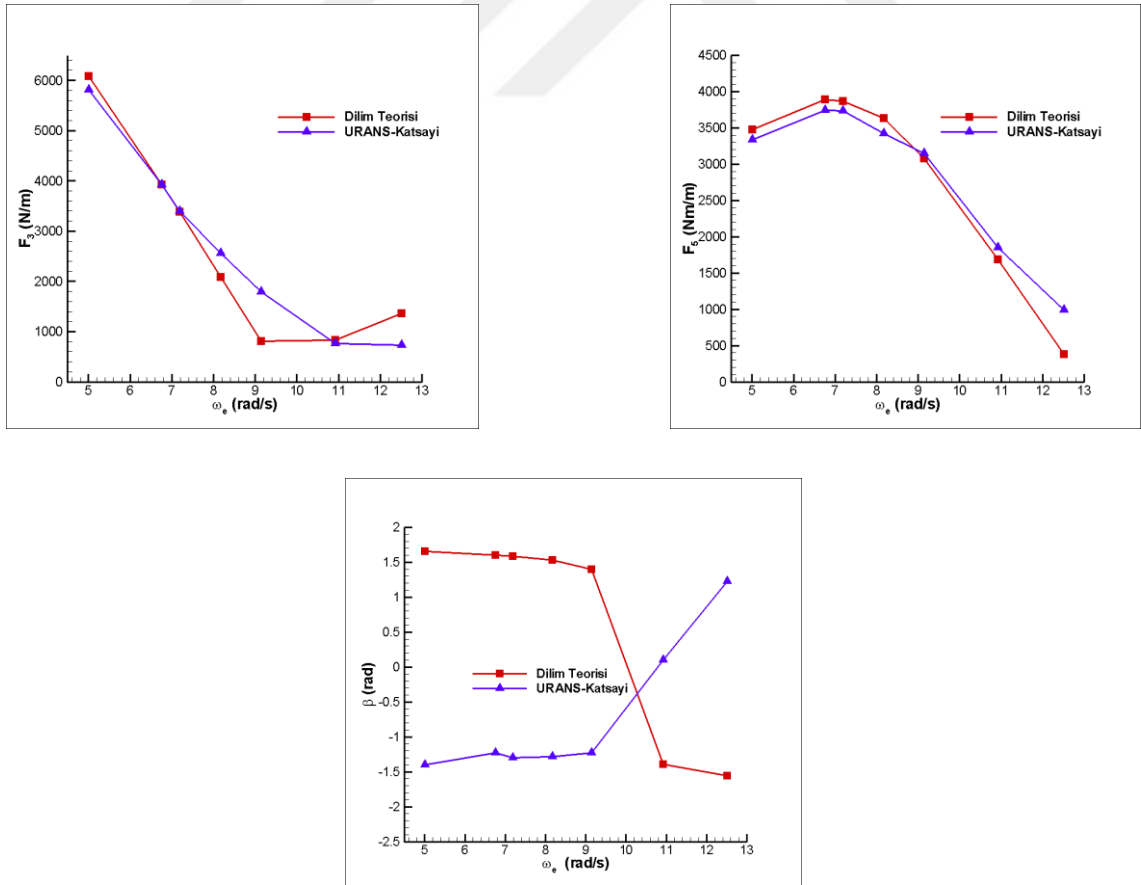
Şekil 2. 24 Faz açıları ile birlikte bozucu terimlerin karşılaştırılması
