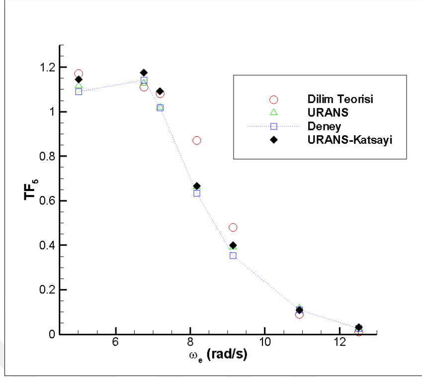
Şekil 4. 2 Baş-kıç vurma TF
