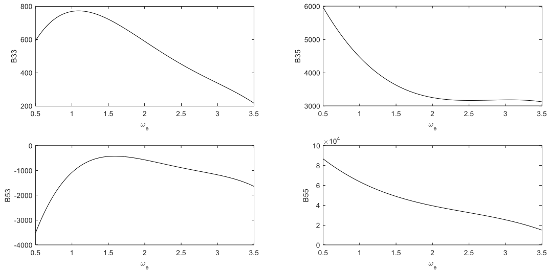
Şekil 3. 4 Sönüm- \omega_e grafikleri
