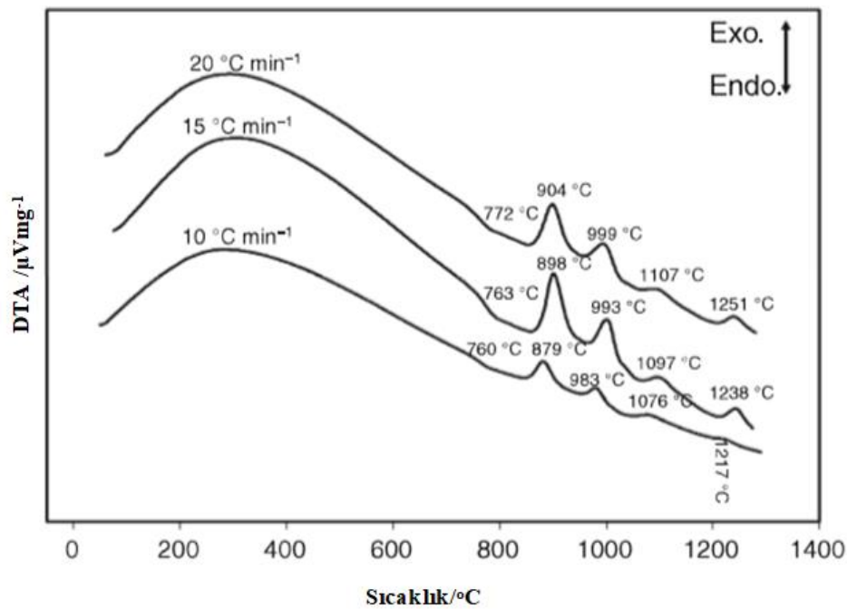
Şekil 4.7. M-Bi-Ti-3 bileşiminin farklı ısıtma oranlarında DTA analizi
