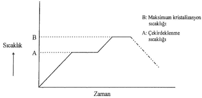
Şekil 2.8. Cam-seramik ısıtma işlemi genel karakteristiği [87]
