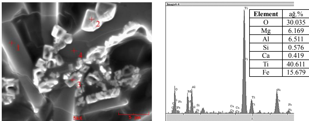
Şekil 4.11. M-Bi-Ti-O için 1250 ° C'de 1 saat ısıtılma sonrası EDS görüntüsü (4 numara)
