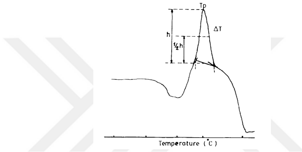
Şekil 2.7. n değerinin hesaplanmasında kullanılan \Delta T 'nin ölçülmesini gösteren DTA kristallenme piki [30]
