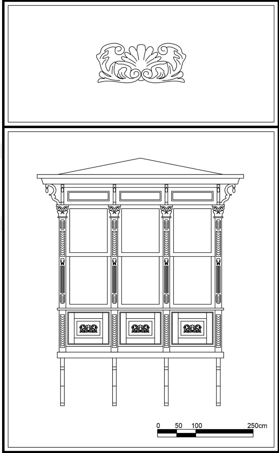
Çizim 29. Alsancak Mahallesi, Cumhuriyet Bul., No:224, Konak adresindeki konutun cumbası.
