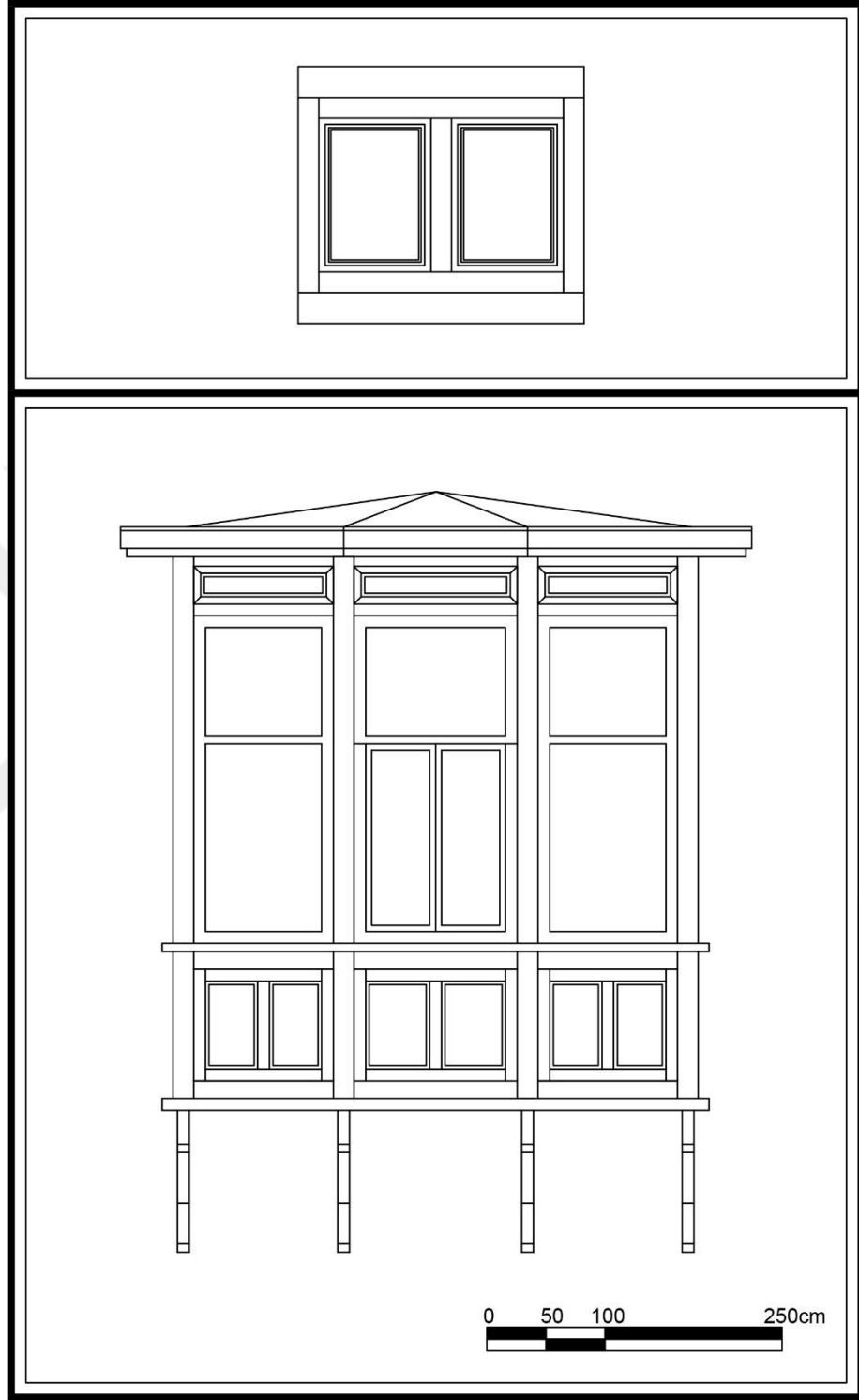
Çizim 75. Donanmacı Mahallesi, 1728 Sok. ve Kemalpaşa Cad. kesişimi, No:1, Karşıyaka adresindeki konutun cumbası.
