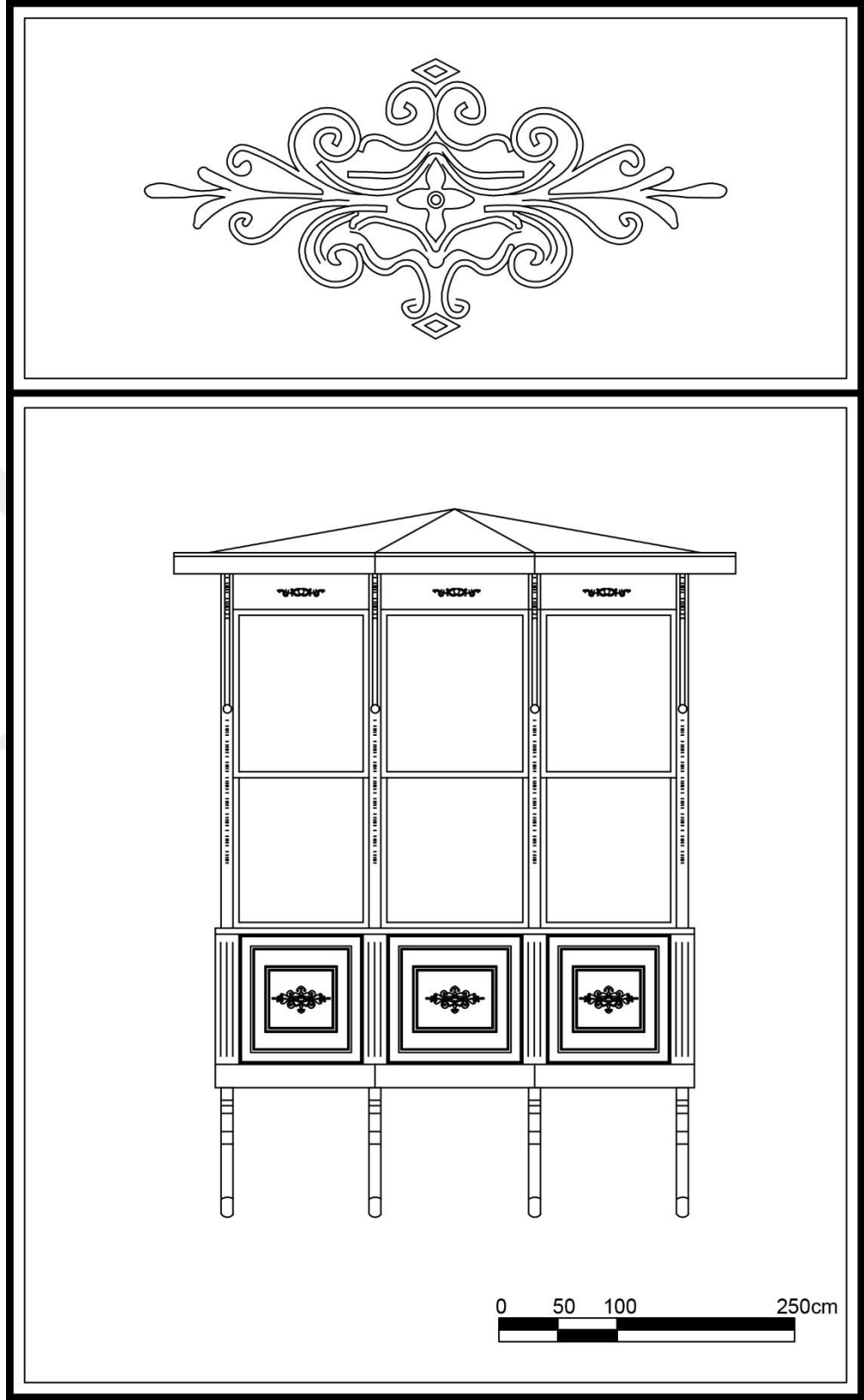
Çizim 6. Göztepe Mahallesi, 77 Sok., No:18, Konak adresindeki konutun cumbası.
