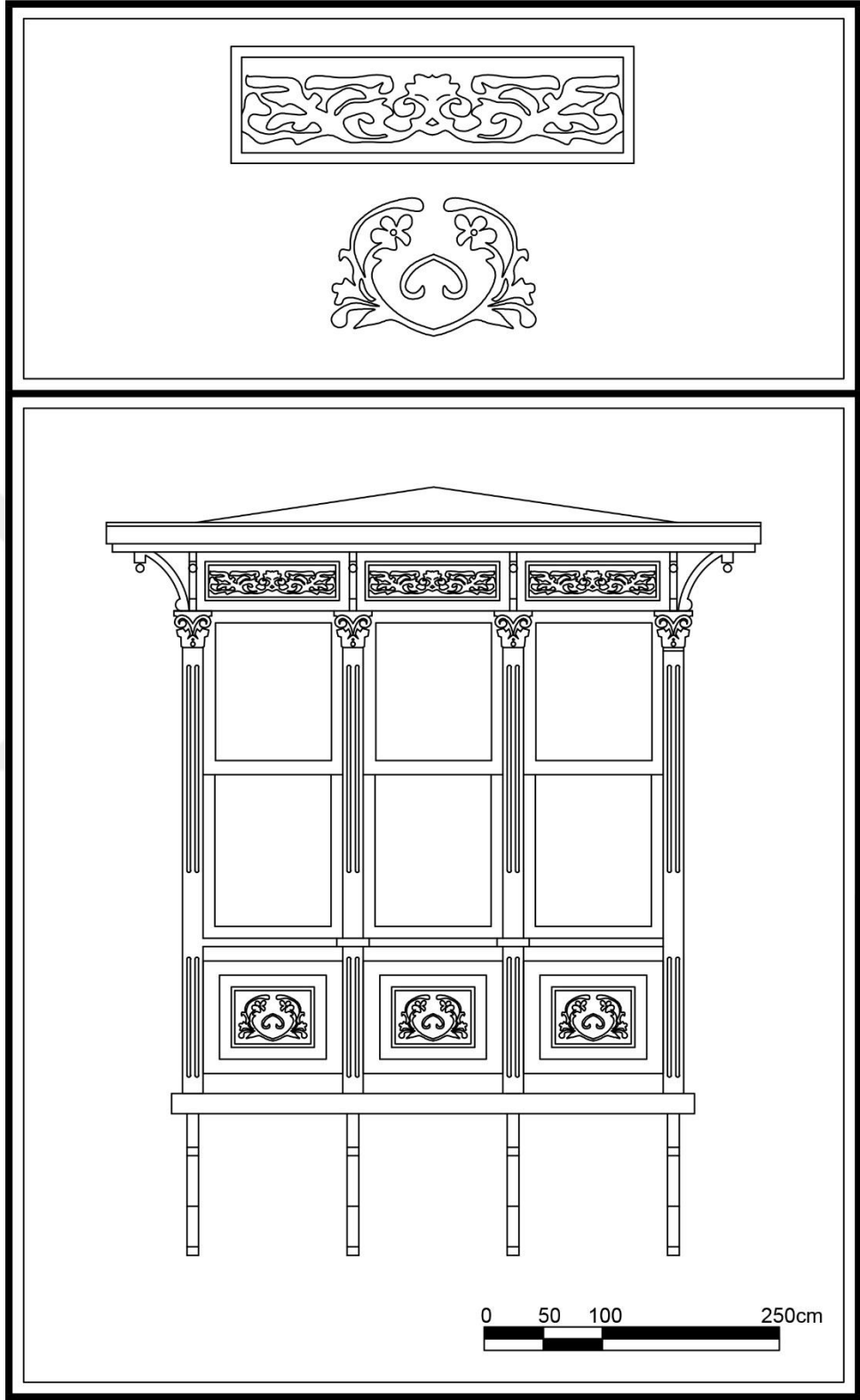
Çizim 73. Bayraklı Mahallesi, 1642 Sok., No:12, Bayraklı adresindeki konutun cumbası.
