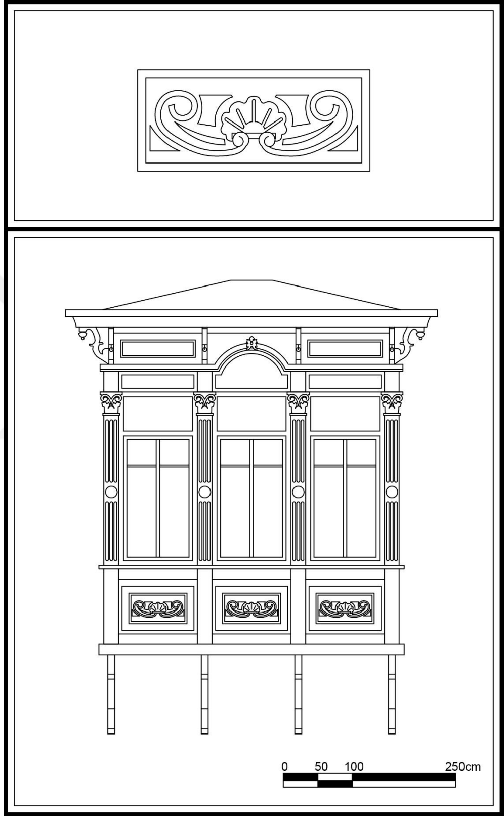
Çizim 22. Alsancak Mahallesi, Cumhuriyet Bul., No:4, Konak adresindeki konutun cumbası.
