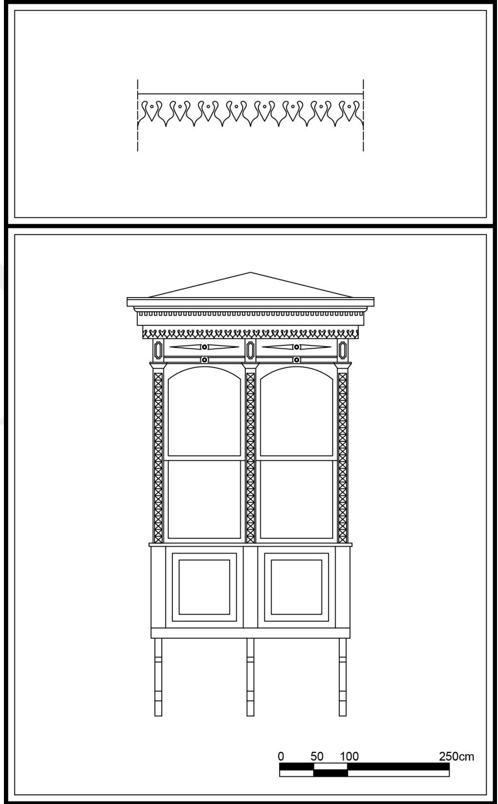
Çizim 37. Alsancak Mahallesi, 1453 Sok., No:26, Konak adresindeki konutun cumbası.
