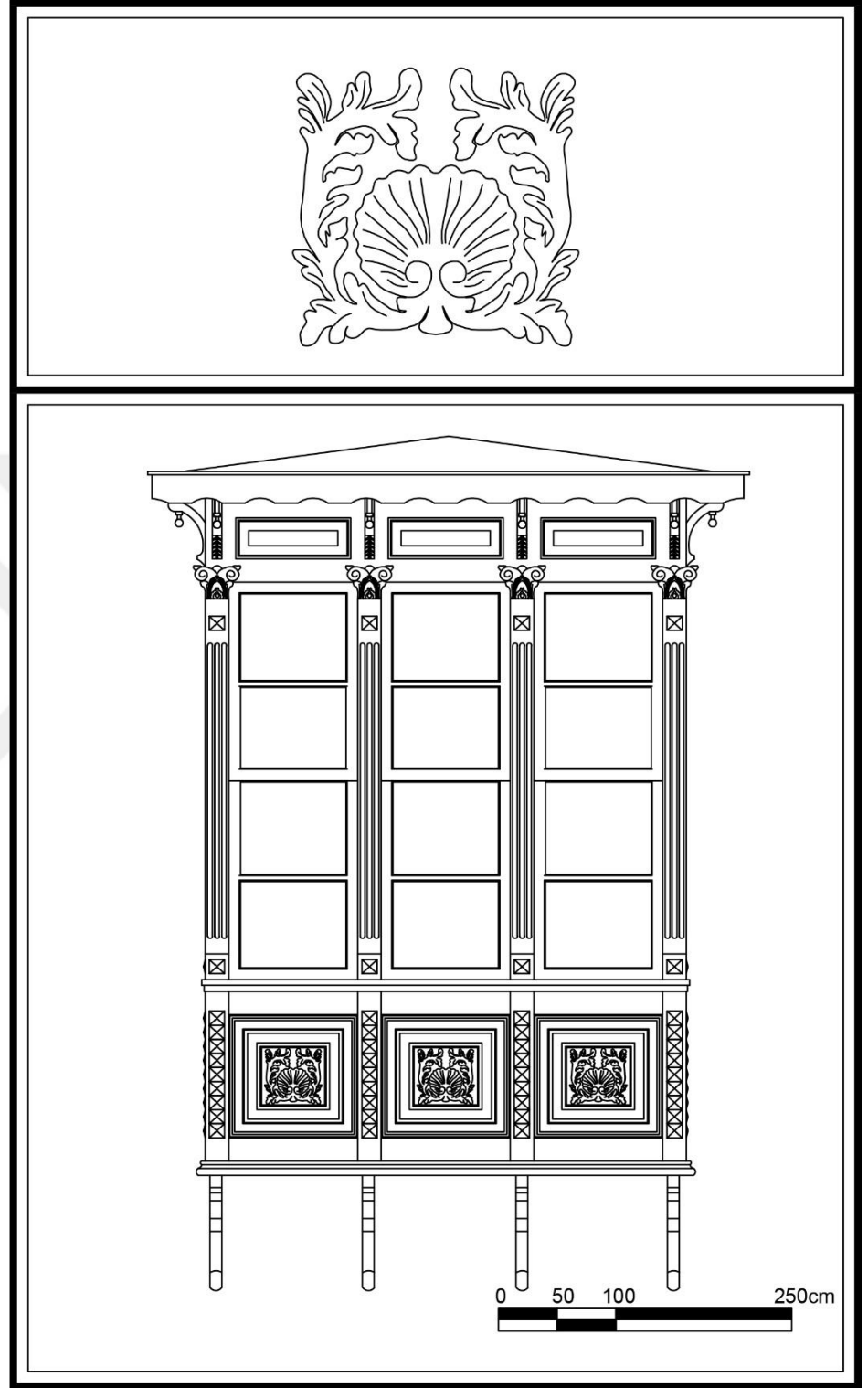
Çizim 3. Güzelyalı Mahallesi, Mithatpaşa Cad., No:1021, Konak adresindeki konutun cumbası
