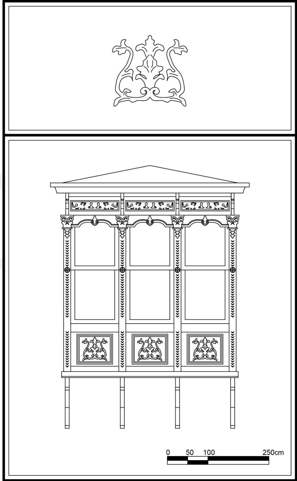
Çizim 77. Donanmacı Mahallesi, Hüseyin Çağlayan Sok., no:6, Karşıyaka adresindeki konutun cumbası.
