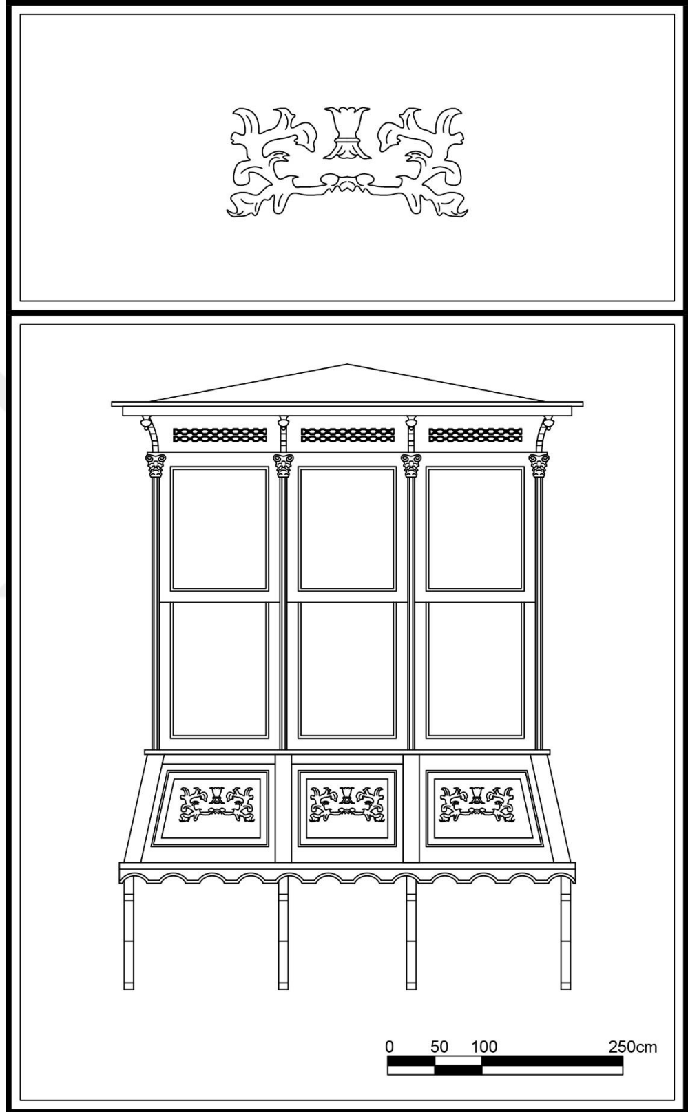
Çizim 39. Alsancak Mahallesi, 1482 Sok., No:7A, Konak adresindeki konutun cumbası.
