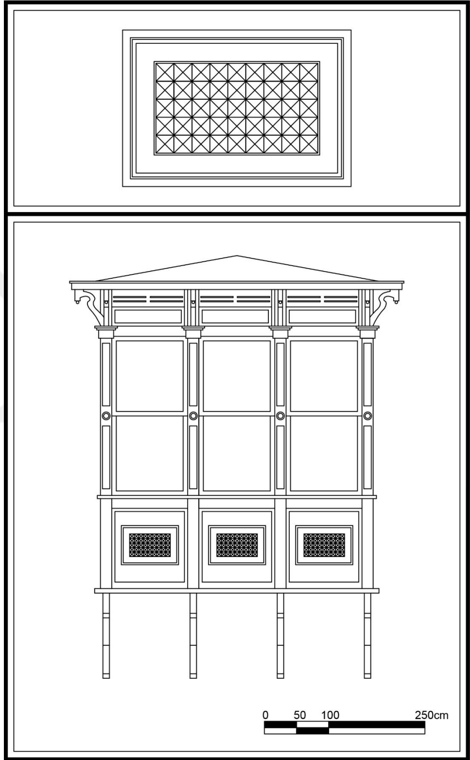
Çizim 65. Dumlupınar Mahallesi, Uğur Mumcu Cad. No:11, Buca adresindeki konutun cumbası.
