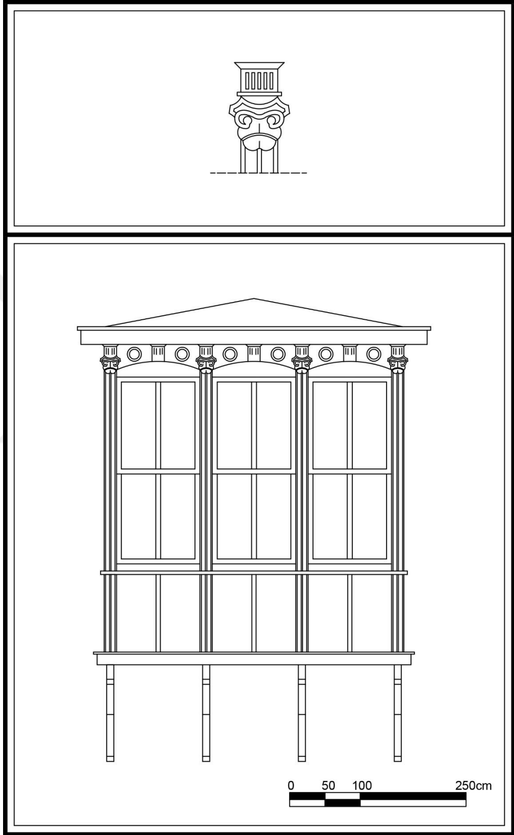
Çizim 28. Alsancak Mahallesi, Cumhuriyet Bul., No:240, Konak adresindeki konutun cumbası.
