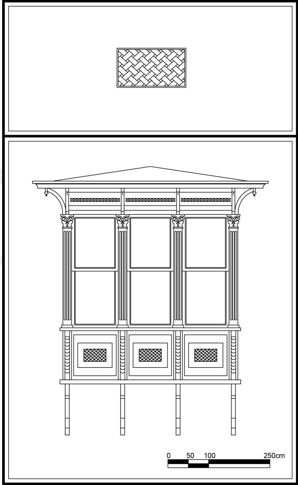
Çizim 46. Alsancak Mahallesi, Enver Başar Dünder Sok., No:7, Konak adresindeki konutun cumbası.
