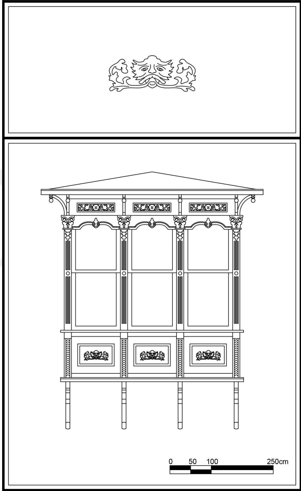
Çizim 48. Alsancak Mahallesi, 1469 Sok., No:6, Konak adresindeki konutun cumbası.
