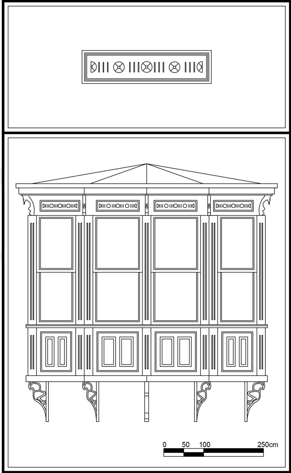
Çizim 44. Alsancak Mahallesi, Kıbrıs Şehitleri Cad., No:26, Konak adresindeki konutun cumbası.
