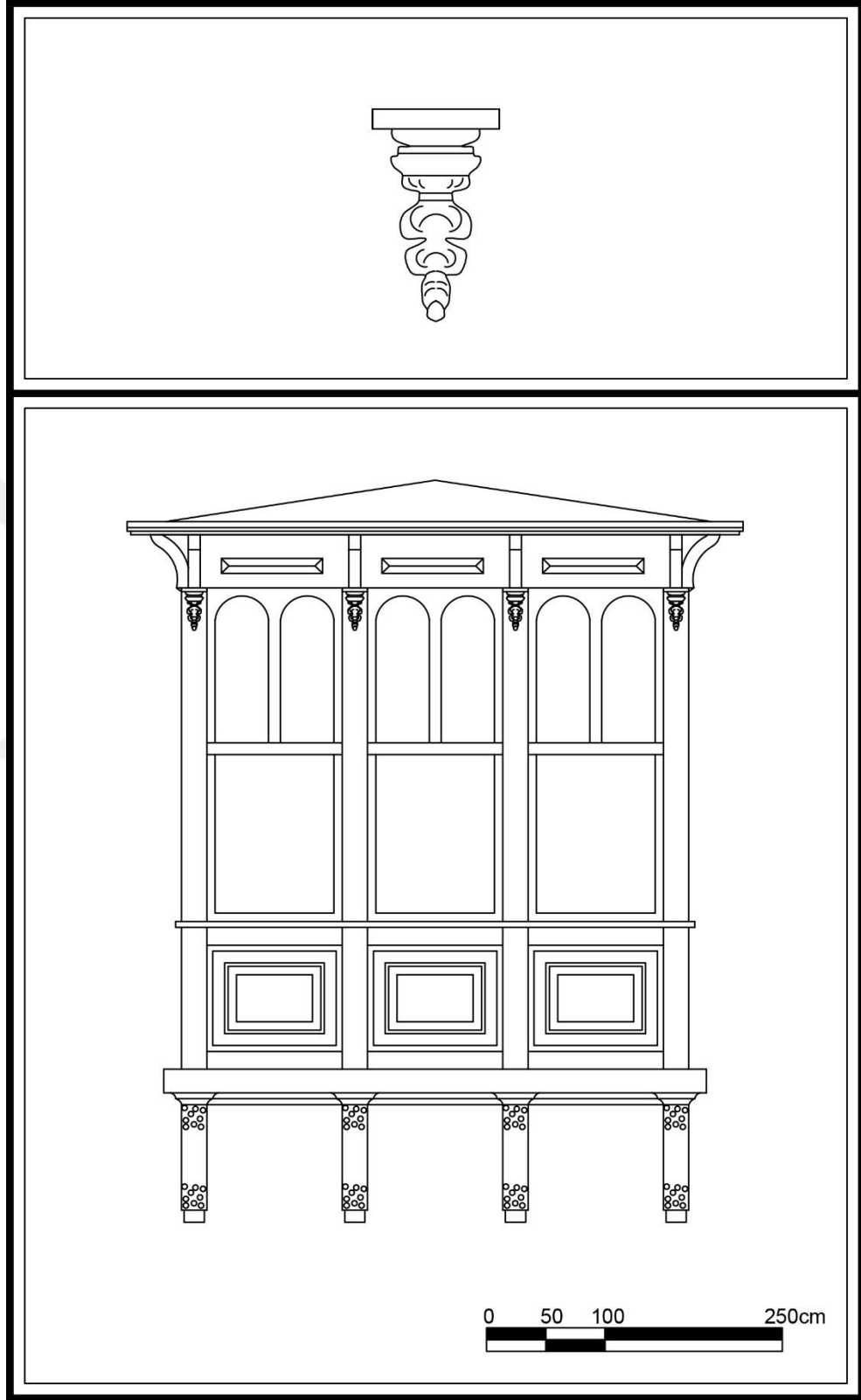
Çizim 38. Alsancak Mahallesi, 1482 Sok., No:3A, Konak adresindeki konutun cumbası.
