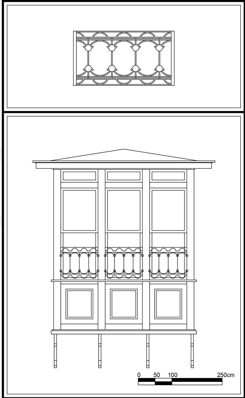
Çizim 63. Kurtuluş Mahallesi, 940 Sok, No: 4, Konak adresindeki konutun cumbası.
