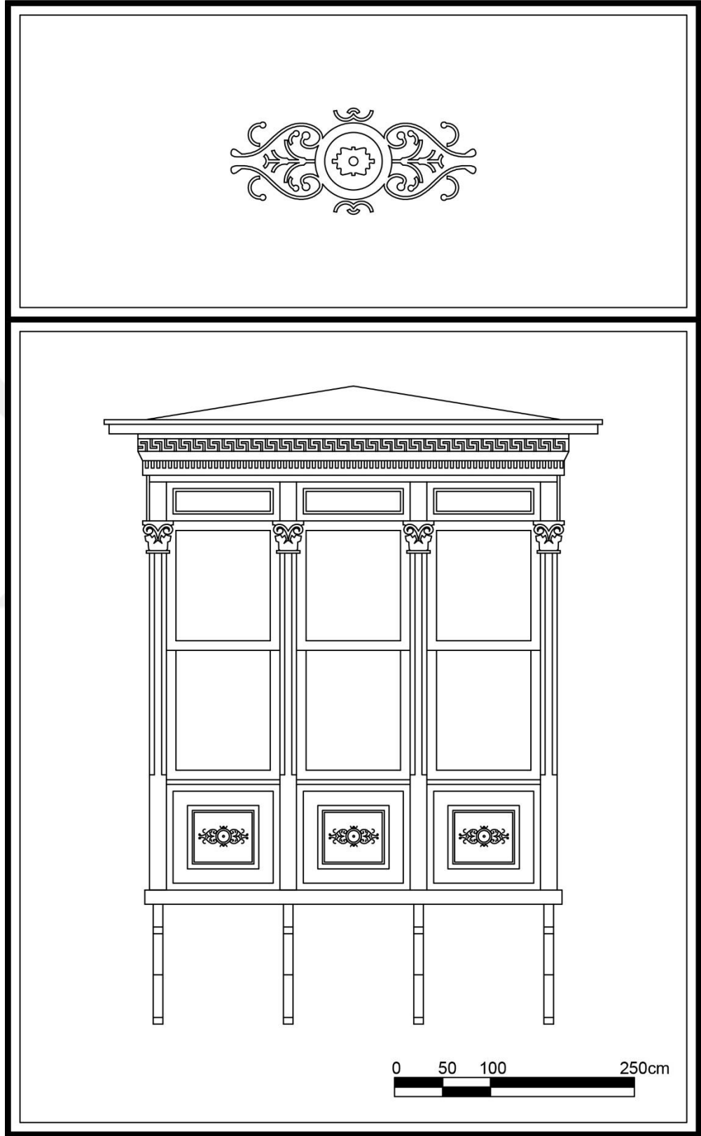
Çizim 30. Alsancak Mahallesi, 1451 Sok., No:7, Konak adresindeki konutun cumbası.
