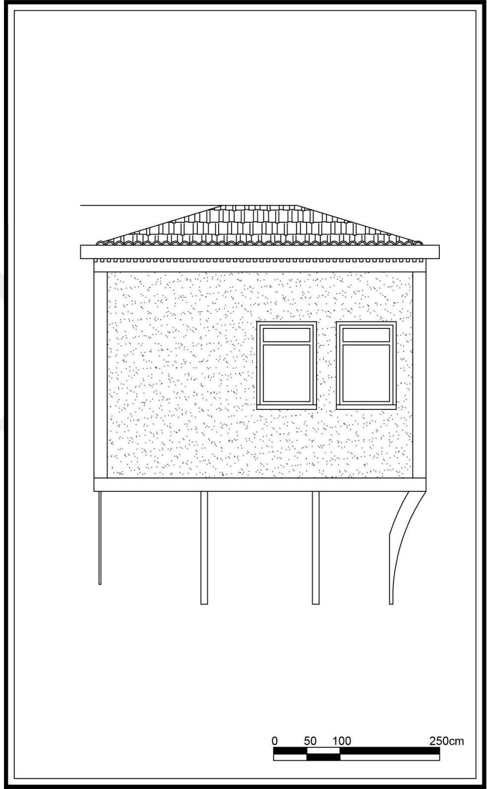
Çizim 82. Pazaryeri Mahallesi, 954 Sok., No:2- 2A, Konak adresindeki konutun çıkması.
