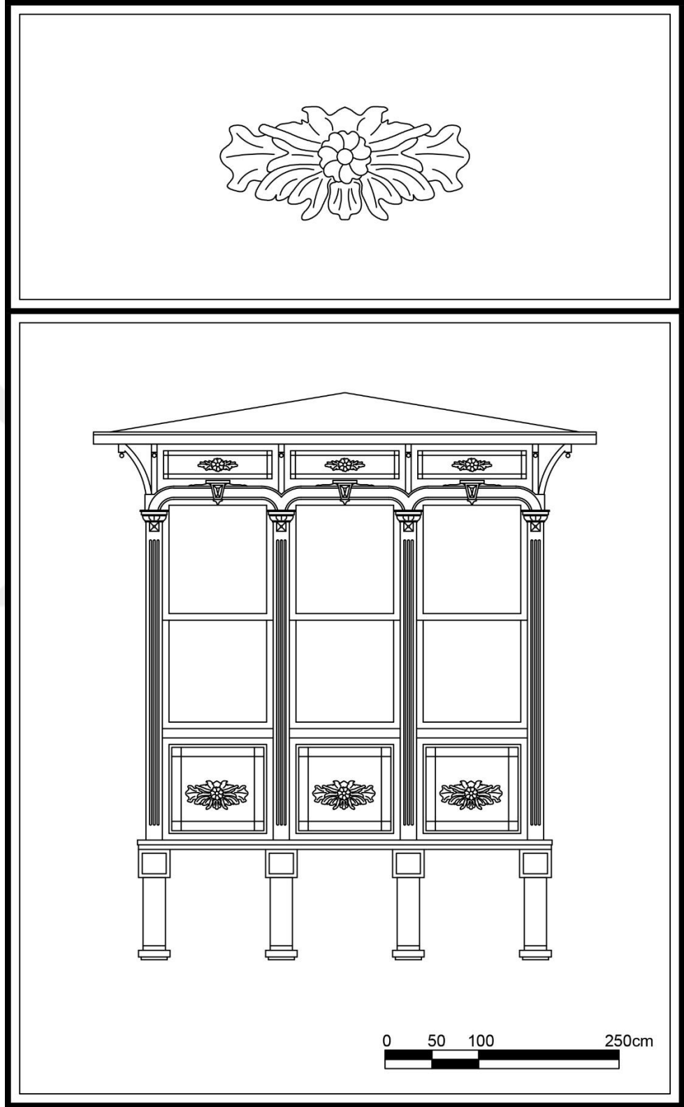
Çizim 35. Alsancak Mahallesi, 1453 Sok., No:17, Konak adresindeki konutun cumbası.
