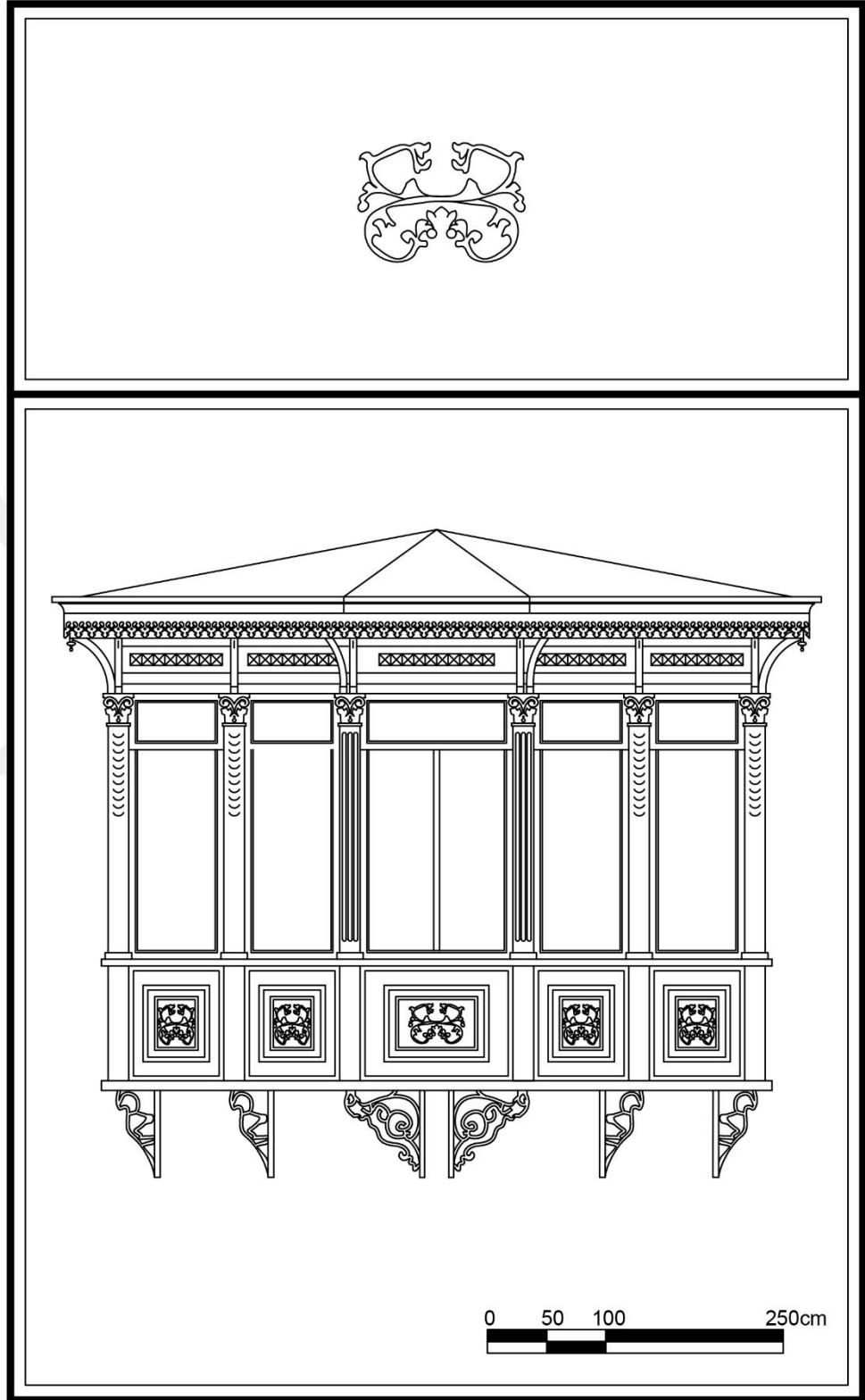
Çizim 59. Akıncı Mahallesi, 1296 Sok., No:25, Konak adresindeki konutun köşede yer alan cumbası.
