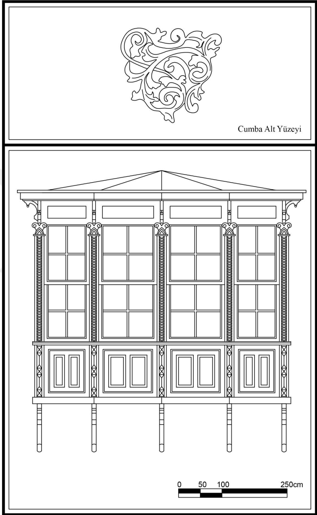
Çizim 19. Mithatpaşa Mahallesi, 211 Sok., No:10-12, Konak adresindeki konutun cumbası.
