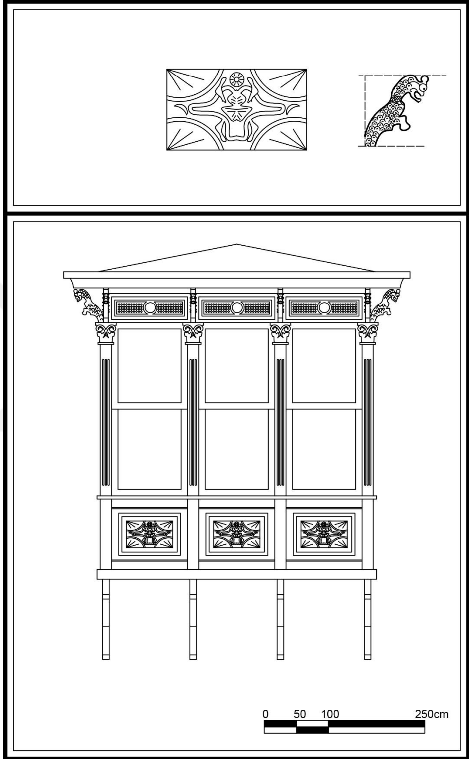
Çizim 40. Alsancak Mahallesi, Muzaffer İzgü Sok., No:10, Konak adresindeki konutun cumbası
