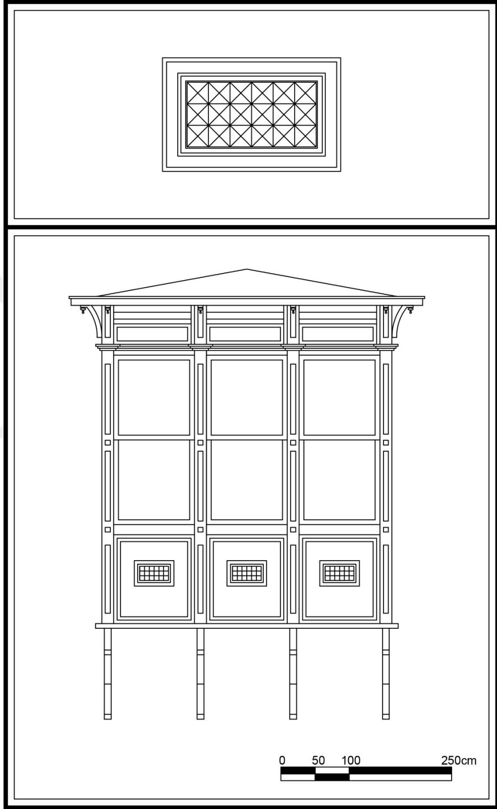
Çizim 27. Alsancak Mahallesi, Cumhuriyet Bul., No:2, Konak adresindeki konutun cumbası.
