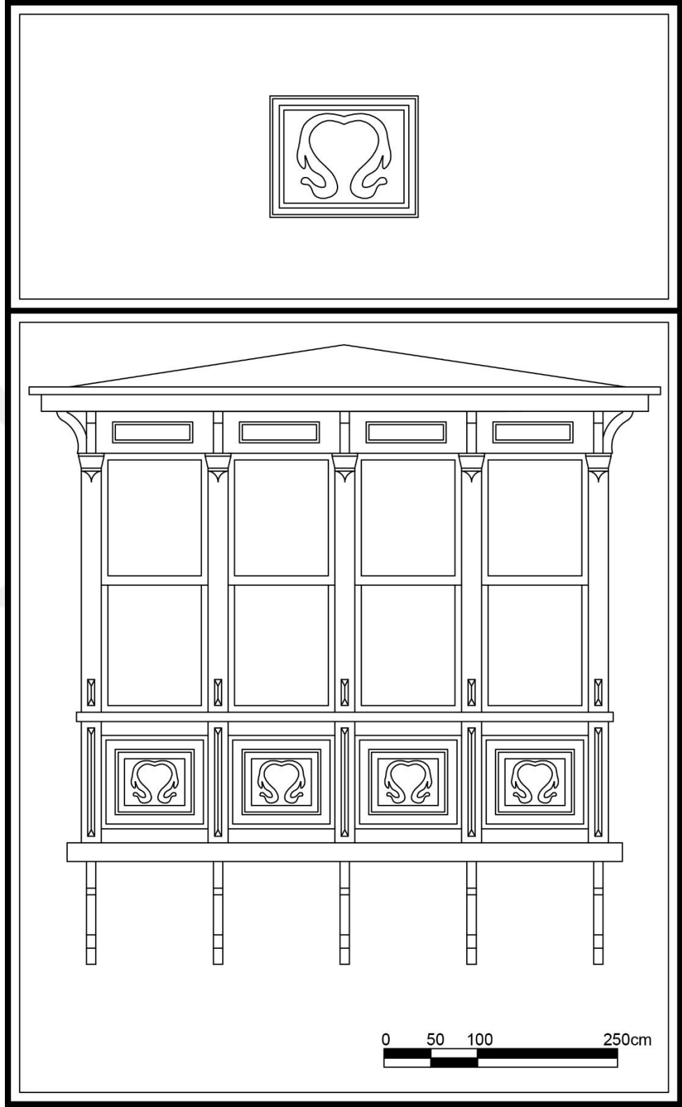
Çizim 45. Alsancak Mahallesi, Kıbrıs Şehitleri Caddesi., No.:29-31A, Konak adresindeki konutun cumbası.
