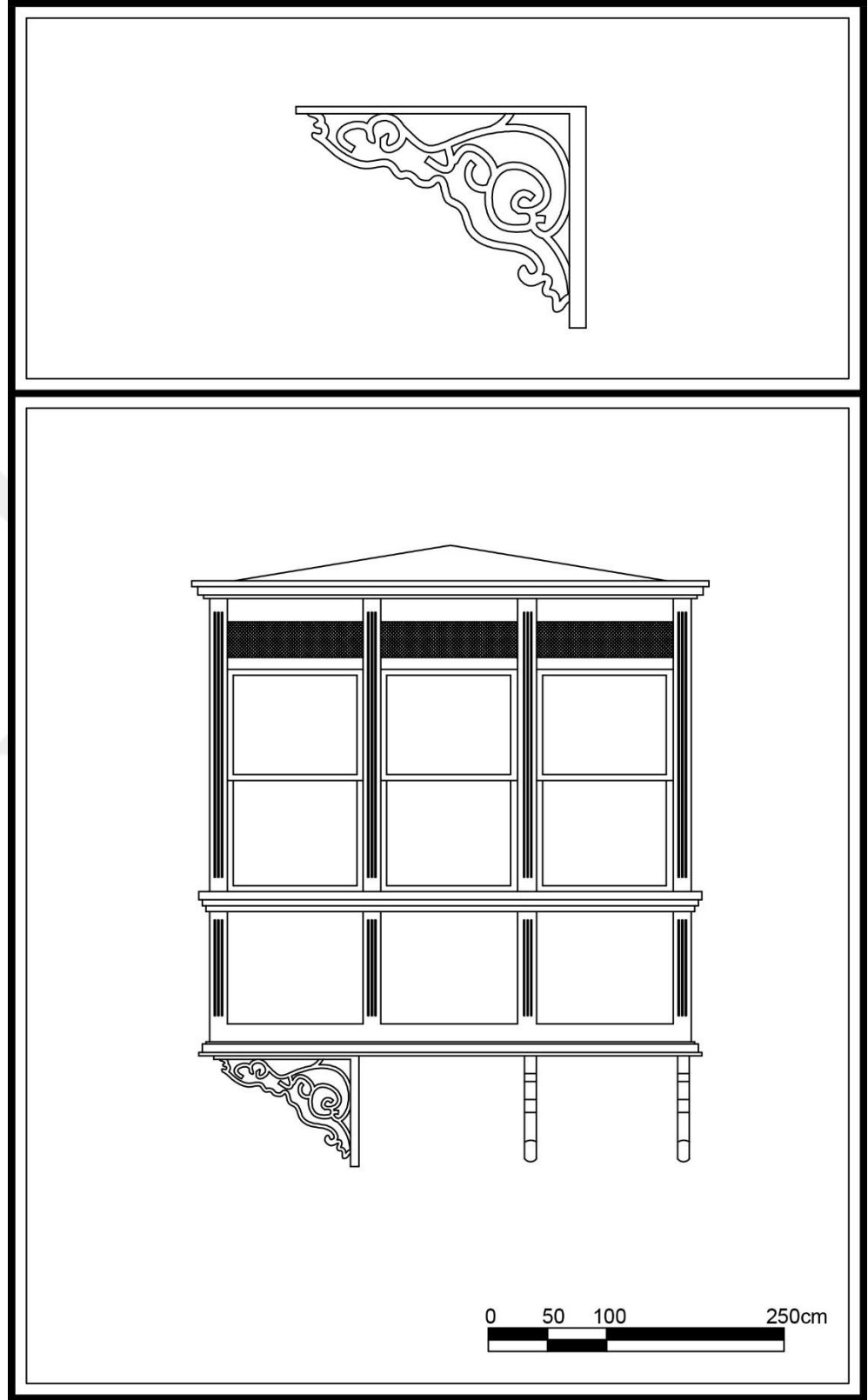
Çizim 9. Çankaya Mahallesi, 133 Sok., No:14, Konak adresindeki konutun cumbası.
