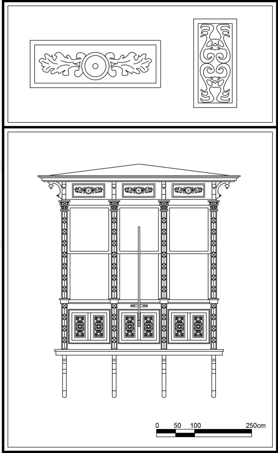
Çizim 13. Çankaya Mahallesi, 141 Sok., No:53, Konak adresindeki konutun cumbası.
