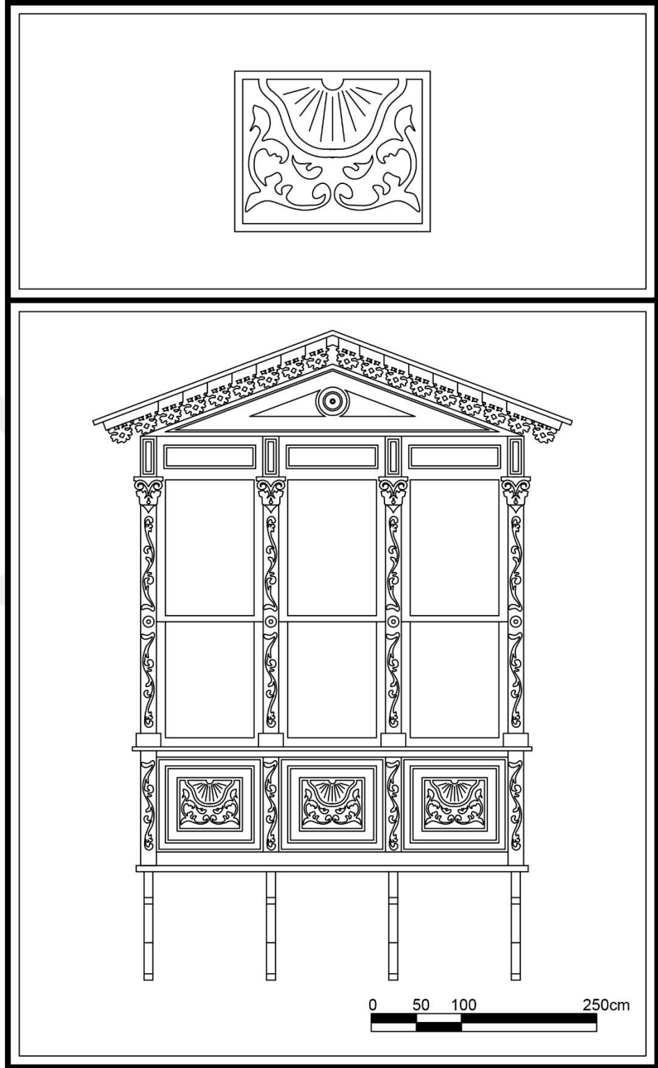
Çizim 74. Tuna Mahallesi, Şehit Üsteğmen Ahmet Konuksever Sok., No:46, Karşıyaka adresindeki konutun cumbası.
