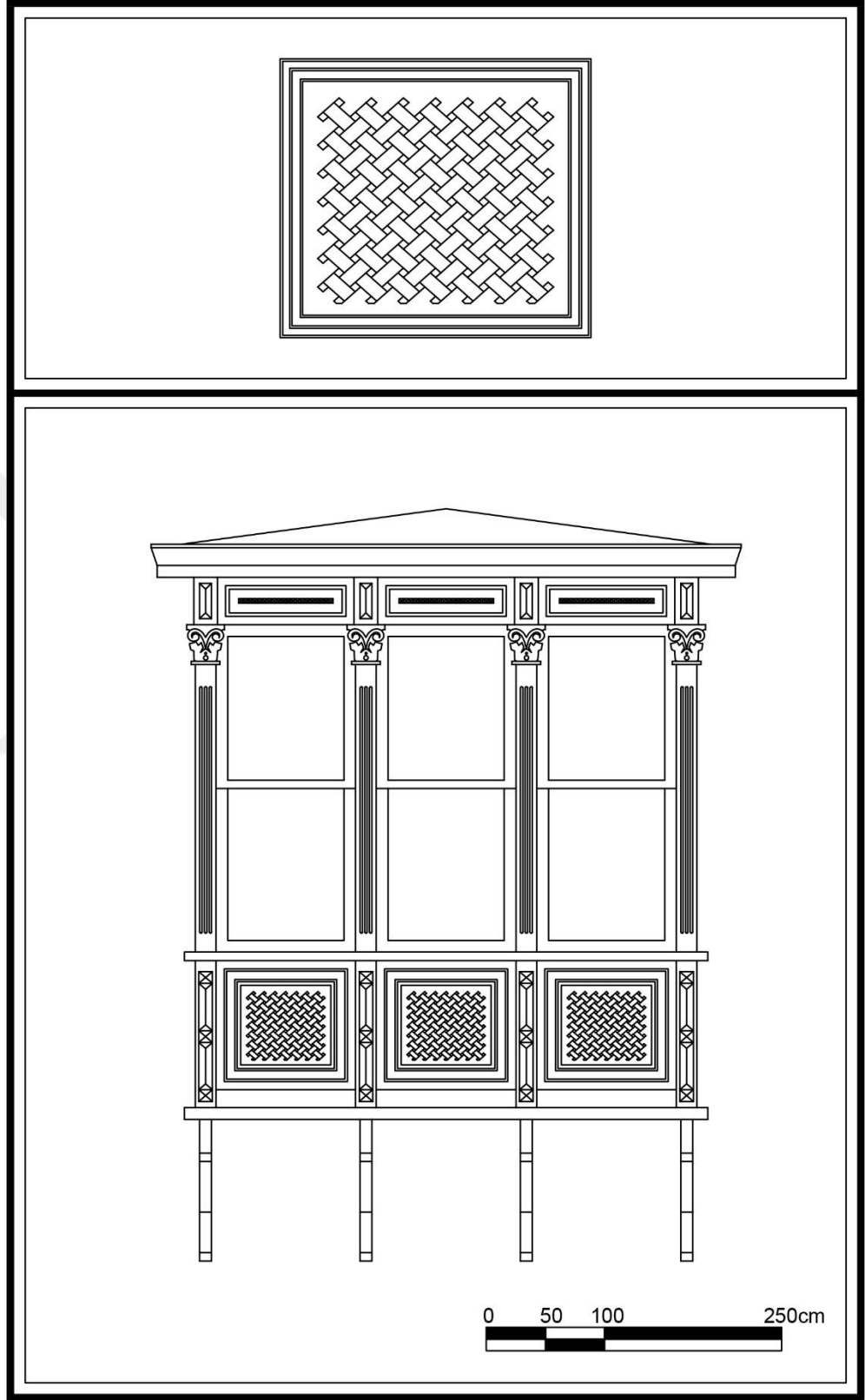
Çizim 24. Alsancak Mahallesi, Cumhuriyet Bul., No:252, Konak adresindeki konutun cumbası.
