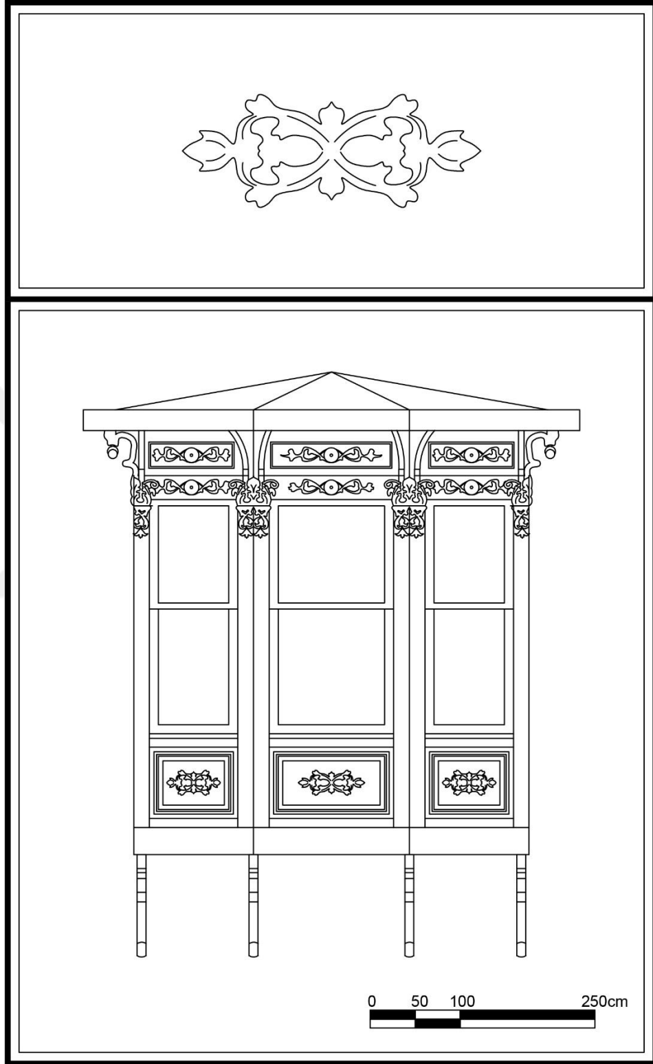
Çizim 51. Alsancak Mahallesi, 1462 Sok.( Yüzbaşı Şerafettin Bey Sok.), No:2, Konak adresindeki konutun cumbası.
