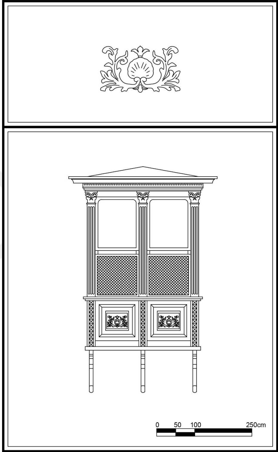
Çizim 20. Mithatpaşa Mahallesi, Mithatpaşa Cad., No:441, Konak adresindeki konutun cumbası.
