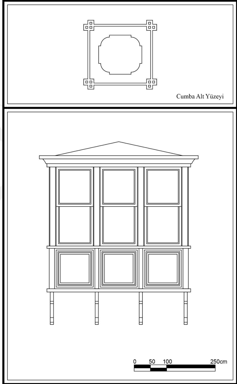
Çizim 21. Turgut Reis Mahallesi, Şehit Kemal Keser Sok., No:59- 59 A, Konak adresindeki konutun cumbası.
