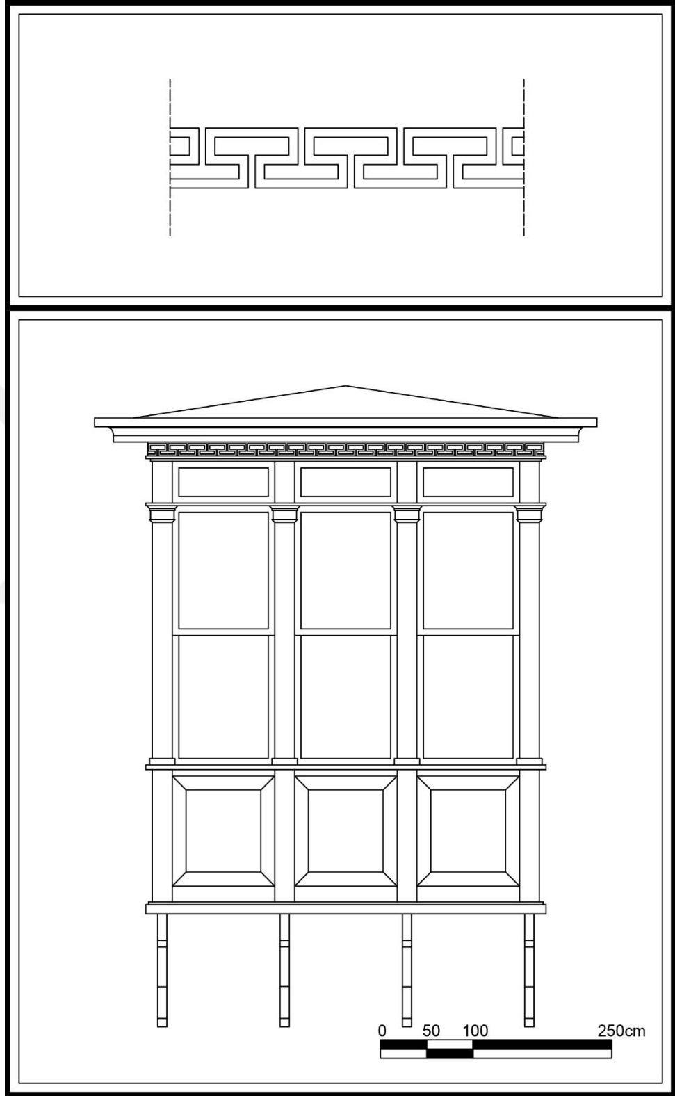
Çizim 18. Mithatpaşa Mahallesi, Mithatpaşa Cad., No:2- 2 A, Konak adresindeki konutun yan cephede yer alan cumbası.
