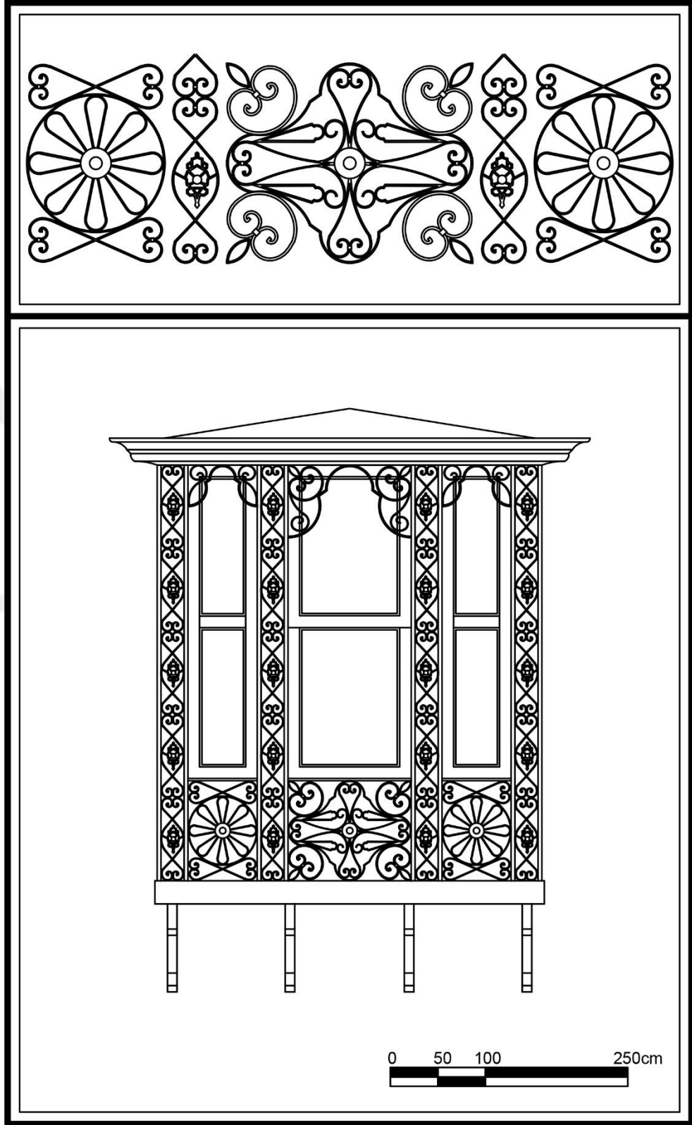
Çizim 60. Akıncı Mahallesi, 945 Sok., No:18, Konak adresindeki konutun cumbası.
