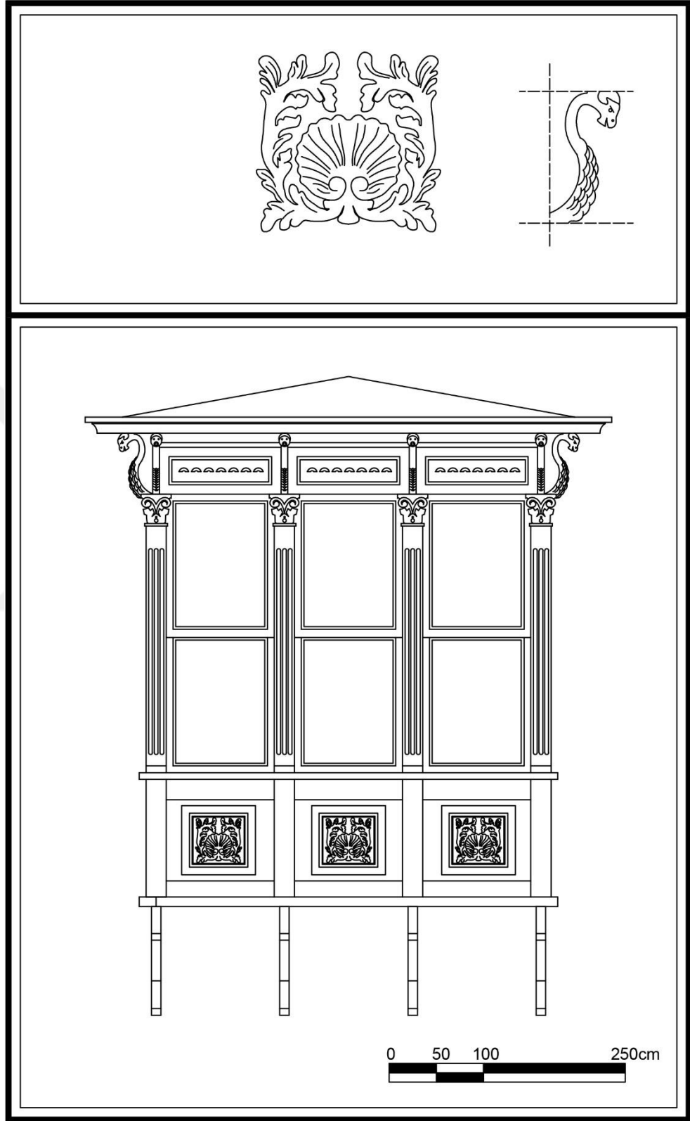
Çizim 53. Alsancak Mahallesi, 1462 Sok., No:50-52A Konak adresindeki konutun cumbası.
