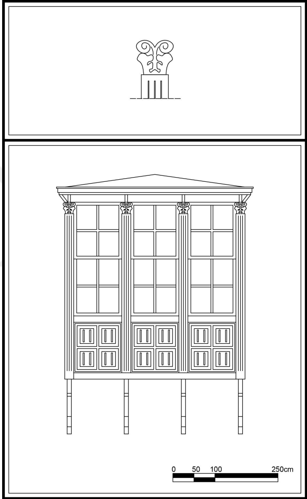
Çizim 32. Alsancak Mahallesi, 1453 Sok., No:11, Konak adresindeki konutun cumbası.
