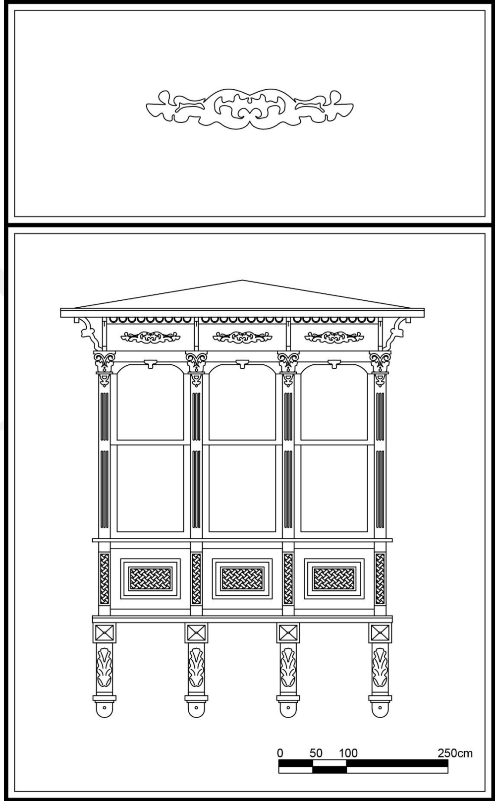
Çizim 34. Alsancak Mahallesi, 1453 Sok., No:15, Konak adresindeki konutun cumbası.
