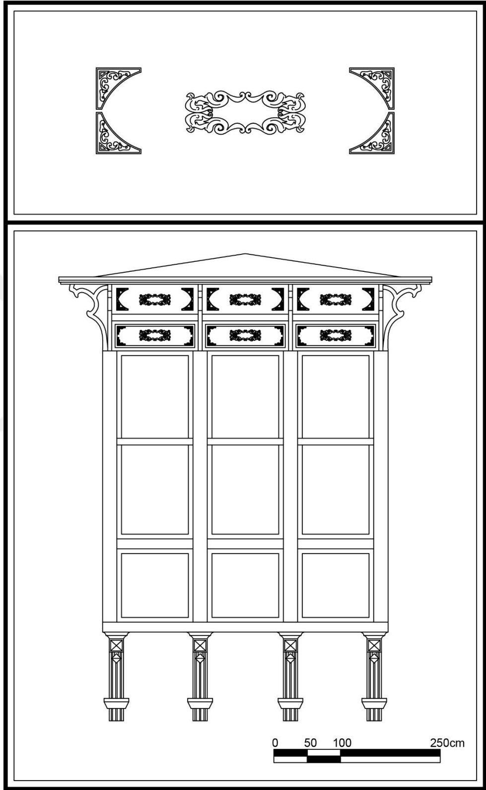
Çizim 49.. Alsancak Mahallesi, Atatürk Cad., No: 364 A, Konak adresindeki konutun cumbası.
