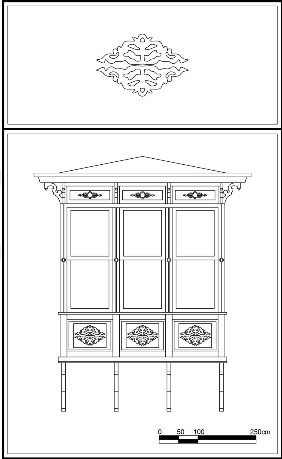
Çizim 64. Dumlupınar Mahallesi, 77 ve 79 Sok. kesişimi No:9, Buca adresindeki konutun cumbası.
