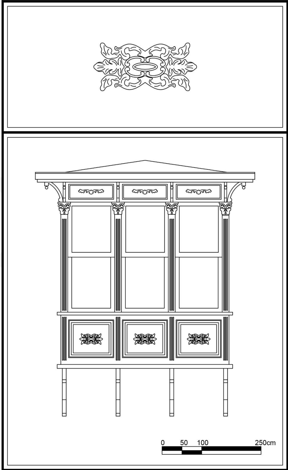
Çizim 71.. Dumlupınar Mahallesi, Barış Manço Sok., No:9. Buca adresindeki. konutun cumbası.
