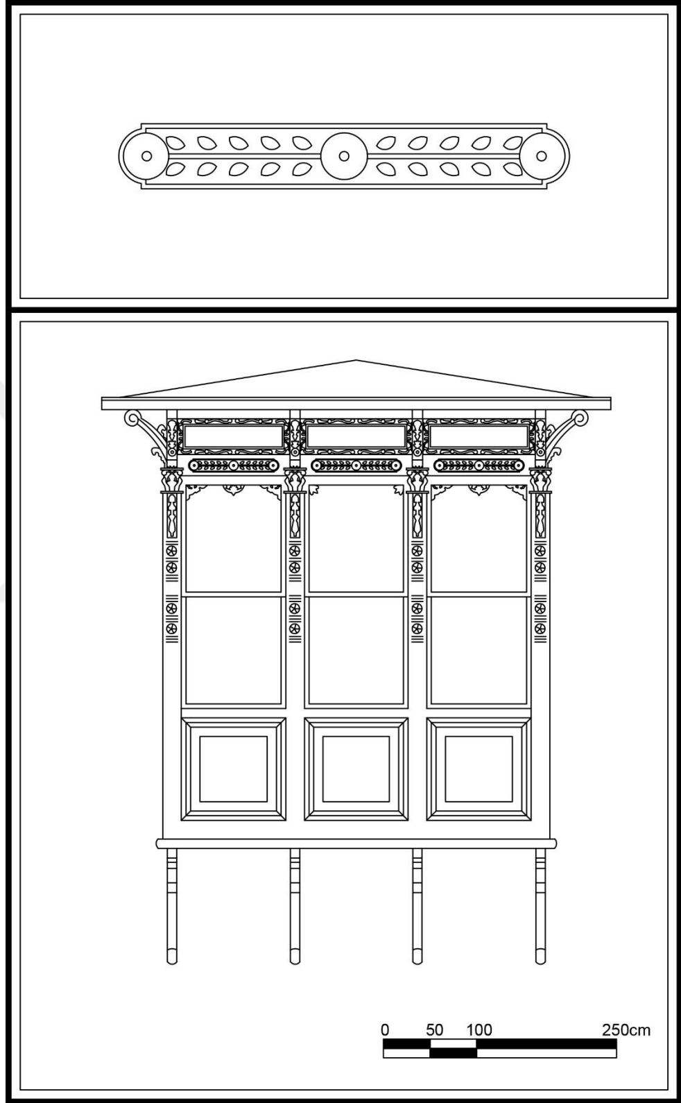
Çizim 4. Güzelyalı Mahallesi, 59 Sok., No:17, Konak adresindeki konutun cumbası.
