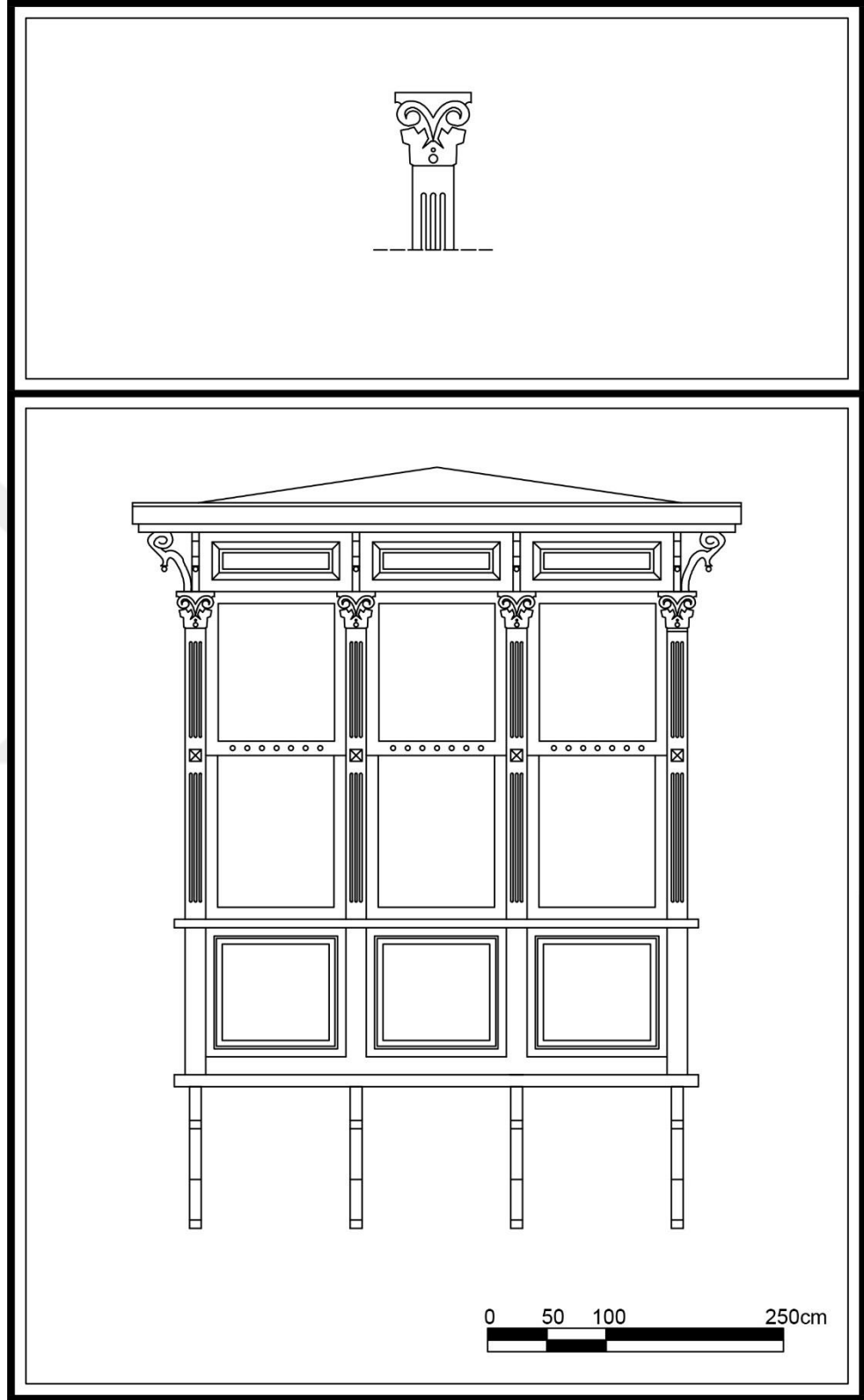
Çizim 69. Dumlupınar Mahallesi, Uğur Mumcu Cad., No:47, Buca adresindeki konutun cumbası.
