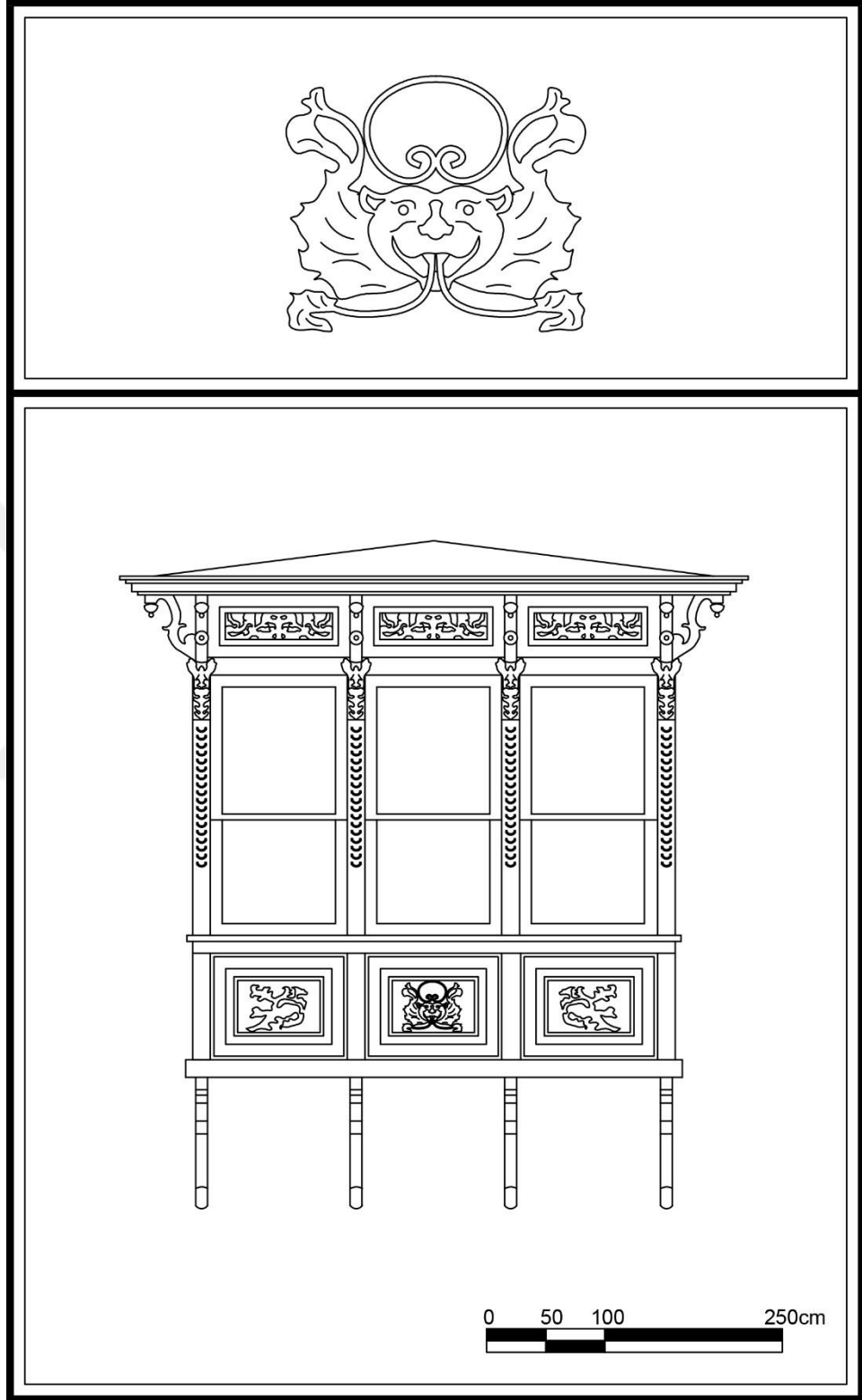
Çizim 12. Çankaya Mahallesi, 141 Sok., No:51- 51 A- 51 B, Konak adresindeki konutun cumbası.
