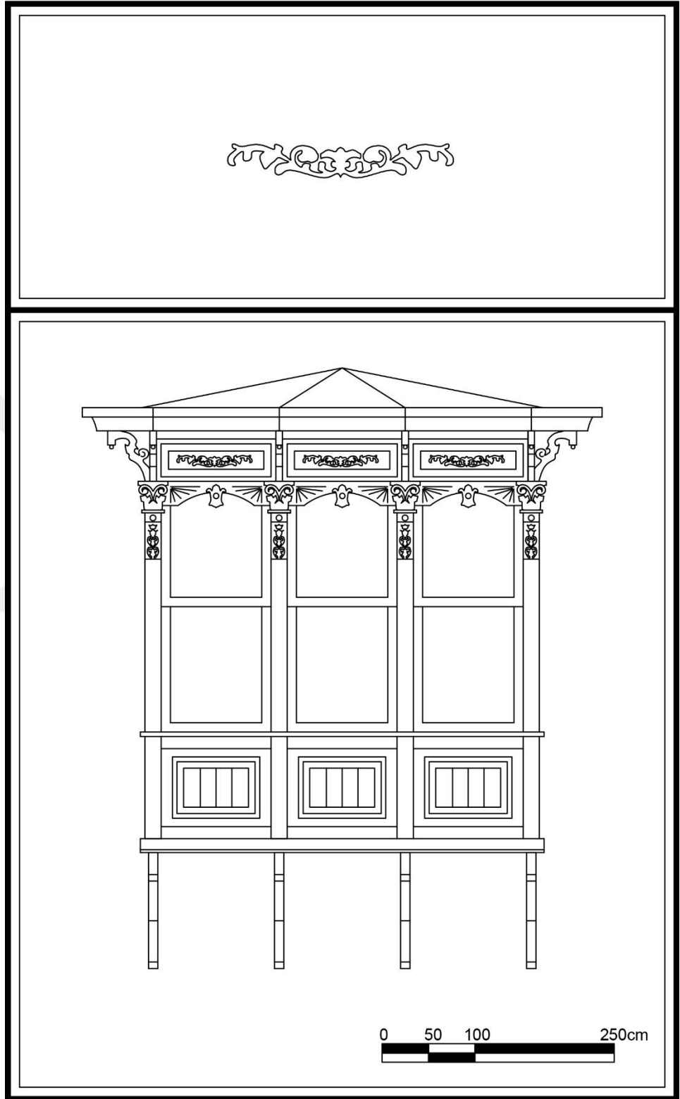
Çizim 54. Alsancak Mahallesi, 1460 Sok., No:33-35, Konak adresindeki konutun cumbası.
