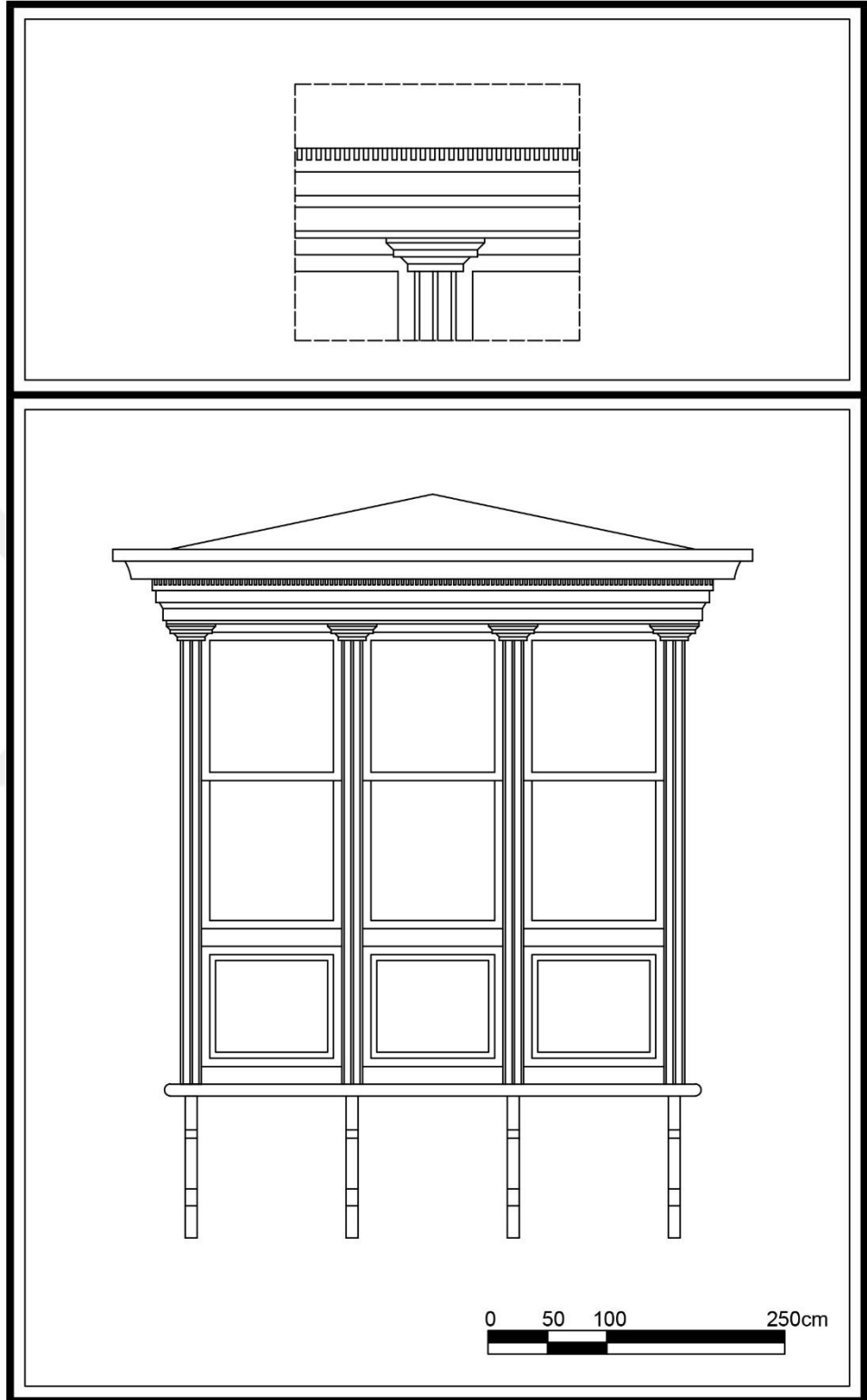
Çizim 23. Alsancak Mahallesi, Cumhuriyet Bul., No:266, Konak adresindeki konutun cumbası.
