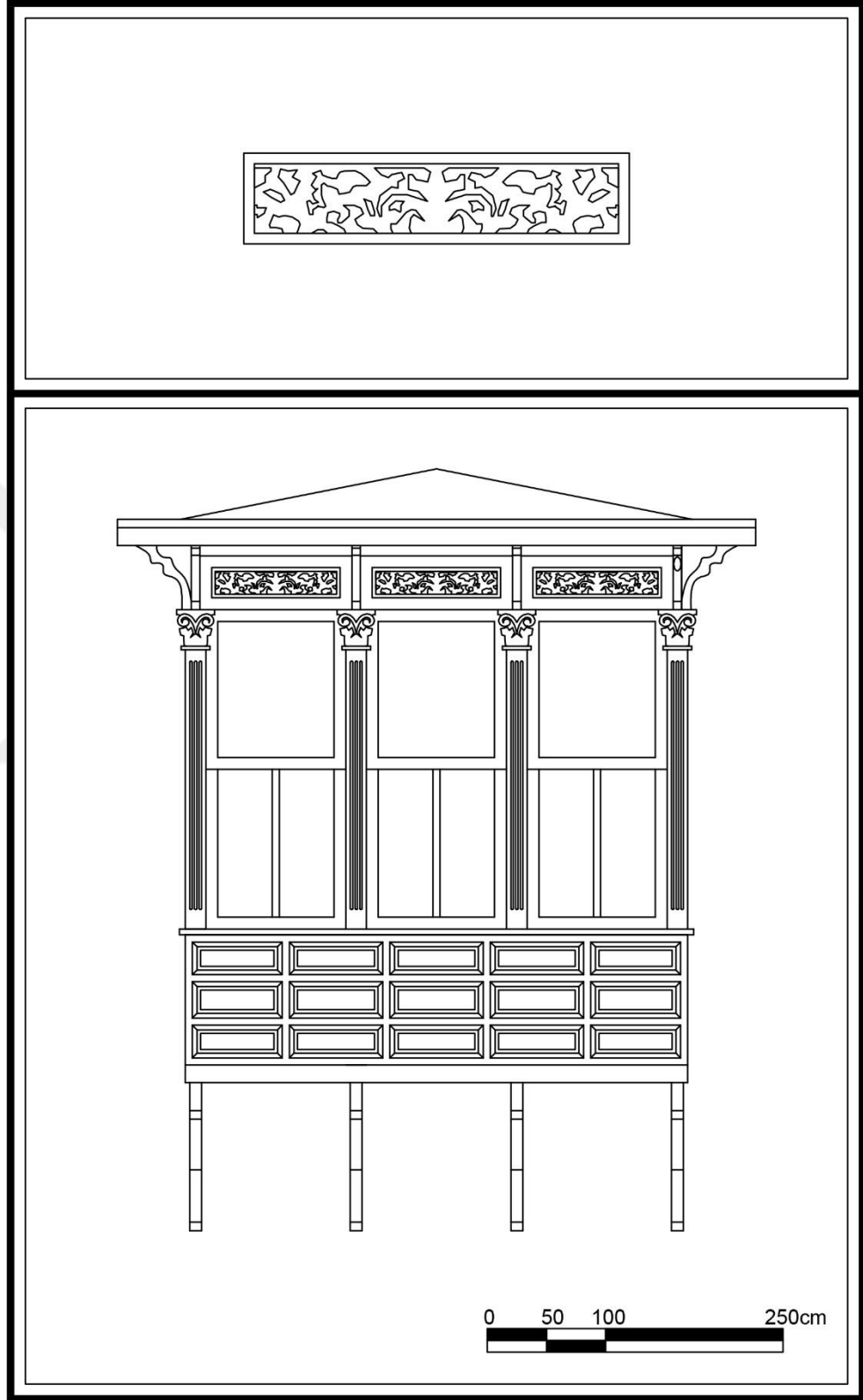
Çizim 66. Vali Rahmi Bey Mahallesi ,Uğur Mumcu Cad., No:16, Buca adresindeki konutun cumbası.
