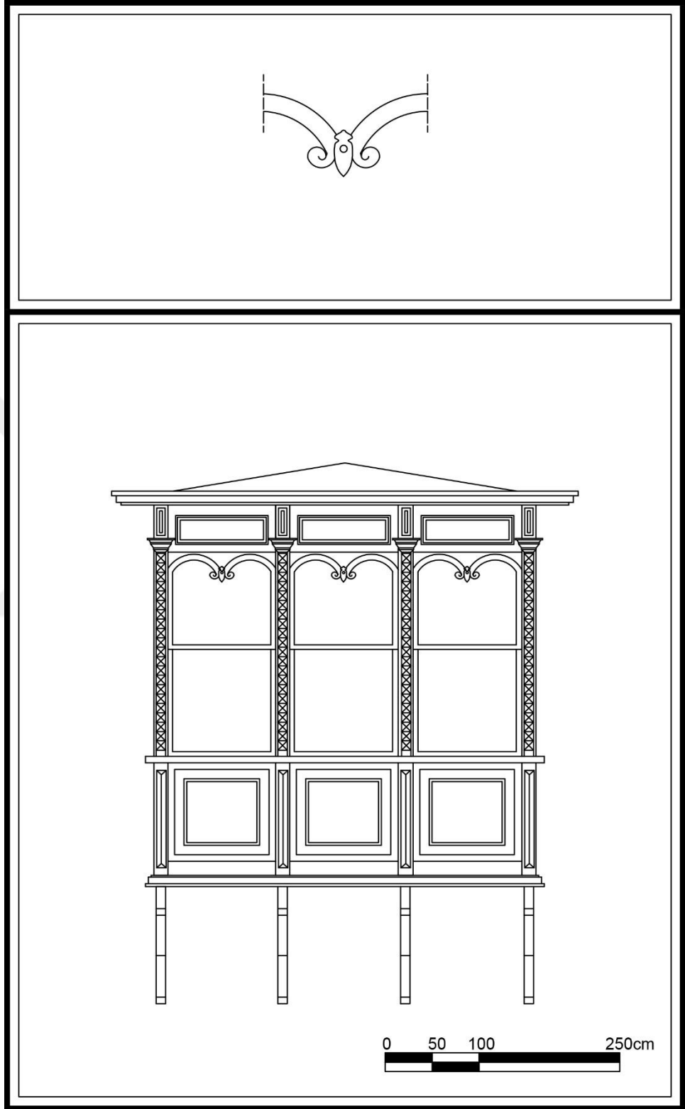
Çizim 67. Dumlupınar Mahallesi ,Uğur Mumcu Cad., No:15, Buca adresindeki konutun cumbası.
