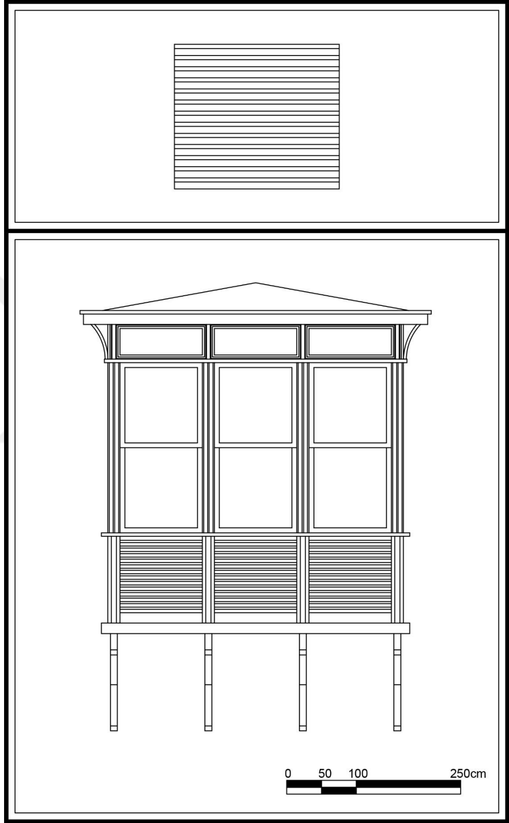
Çizim 26. Alsancak Mahallesi, Cumhuriyet Bul., No:244, Konak adresindeki konutun cumbası.
