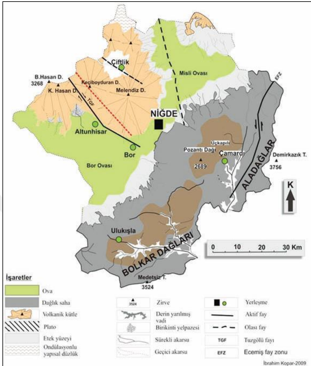
Harita 3. Niğde İlinin Genelleştirilmiş Jeomorfoloji Haritası (Kopar, 2014: 24).
