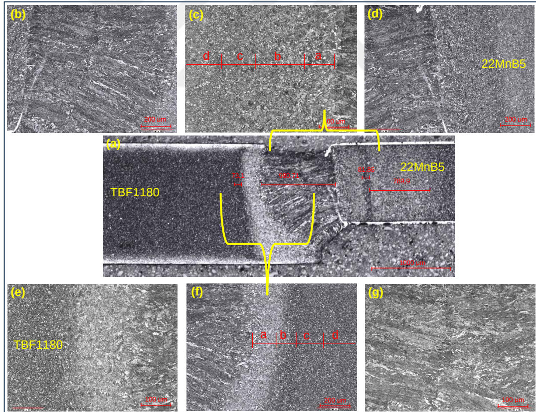
Şekil 6.5. TBF1180-22MnB5 birleştirmesi mikroyapı görüntüleri (150 mm/sn).
