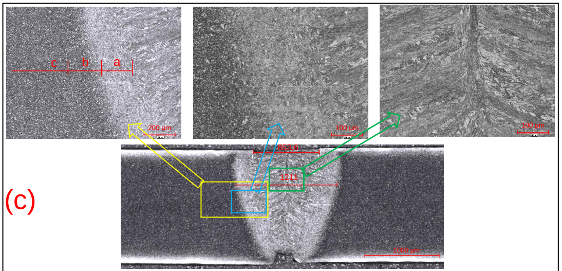
Şekil 6.11. TBF1180-TBF1180 birleştirme makro/mikroyapısı (kaynak hızı (a) 130mm/sn, (b) 150 mm/sn ve (c) 170 mm/sn.
