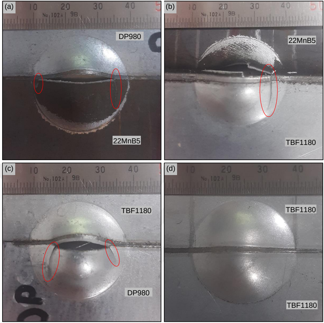
Şekil 6.25. Erichsen çöktürme testi sonrası numune görselleri a) DP980-22MnB5, b) TBF1180-22MnB5, c) TBF1180-DP980 ve d) TBF1180-TBF1180.
