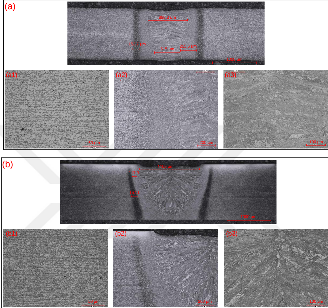
řekil 6.3. 1 ve 2 numaralı numunelerin mikroyapıları; a) DP800GA, b) DP800GI.
