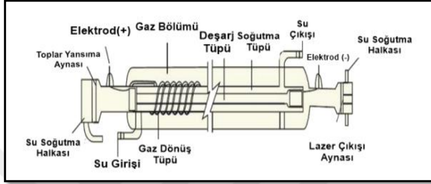
Şekil 3.7. CO 2 lazer rezonatörünün şematik gösterimi [60].
