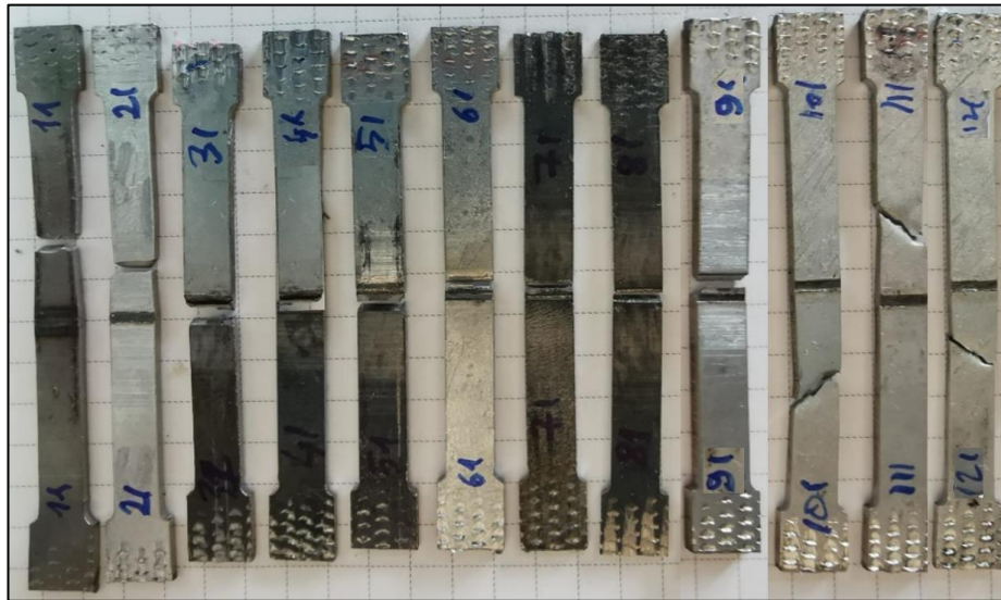
Şekil 6.22. Çekme testi sonrasında kaynaklı numune görselleri
