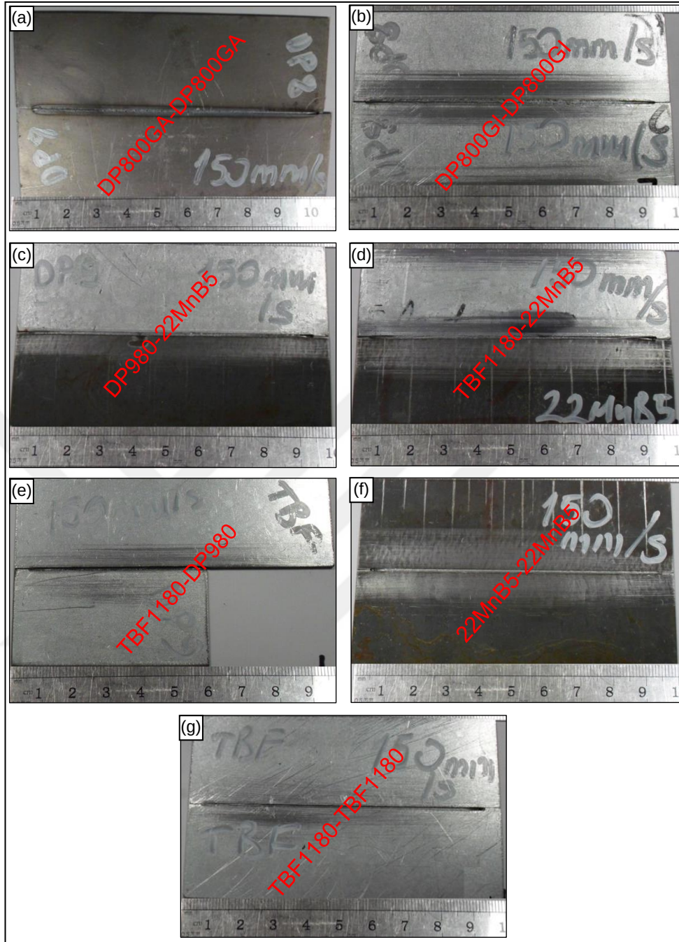
Şekil 6.1. Kaynaklı numunelerin makro görüntüleri, a) DP800GA-DP800GA, b) DP800GI-DP800GI, c) DP980-22MnB5, d) TBF1180-22MnB5, e) TBF1180-DP980, f) 22MnB5-22MnB5, g) TBF1180-TBF1180
