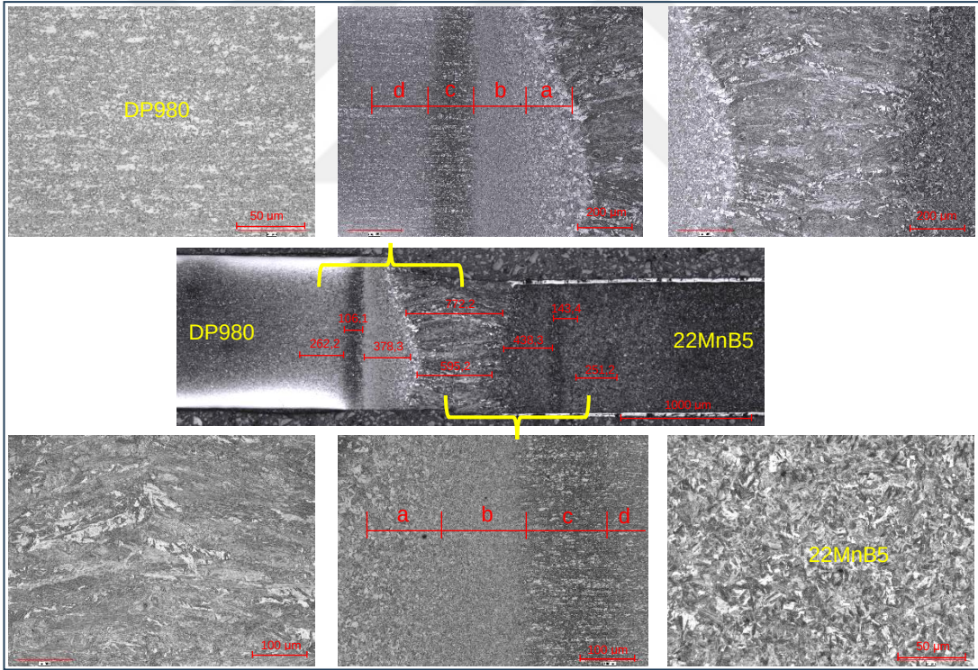
Şekil 6.4. DP980 ile 22MnB5 birleştirmesinin makro/mikroyapısı.
