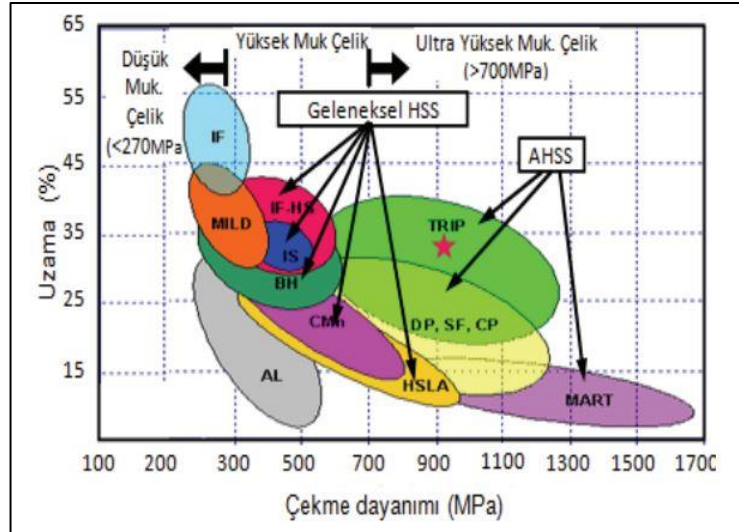
Şekil 2.2. Otomotiv endüstrisinde kullanılan sacların mekanik özellikleri [7].
