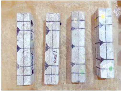
Resim 2.22. Betonun hızlı dondurulması ve çözölmesi için standart test yöntemi olan ASTM C666'yı geen Biyomimetik Antifriz Polimer Modifiye Beton numunesi (Dada vd., 2022)
