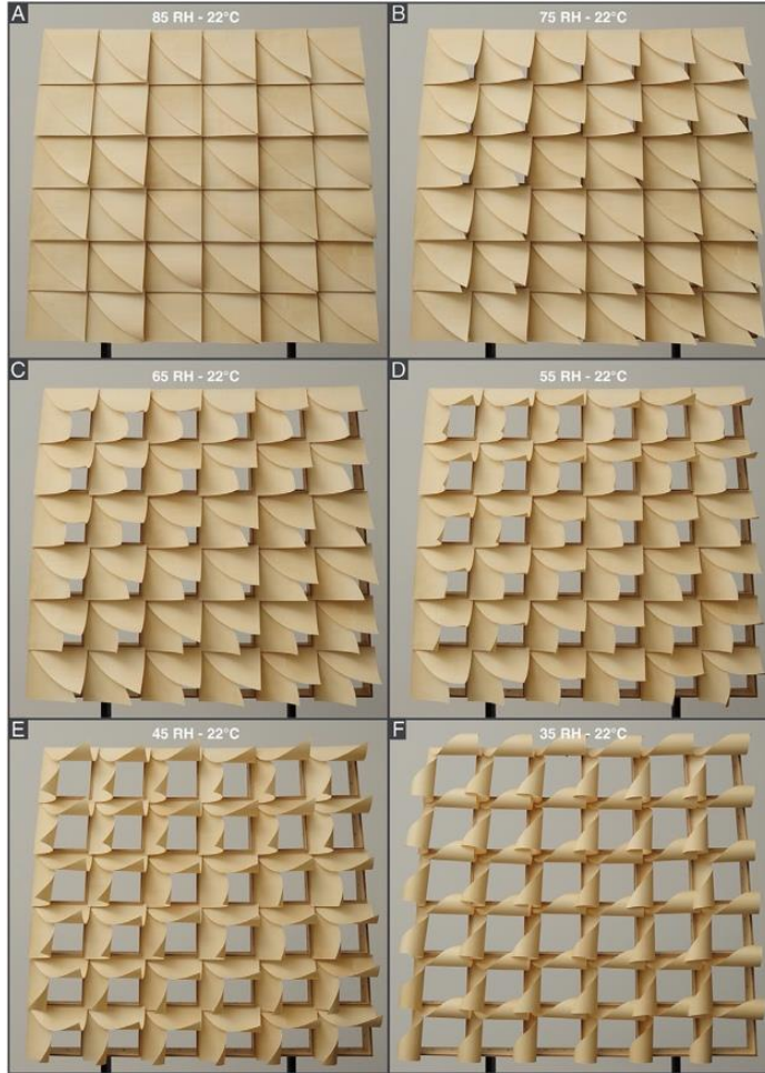
Resim 2.39. İklımsel kořullara baęlı olarak malzemenin sıcaklıęa ve nem seviyesine baęlı testi (Reichert vd., 2015)
