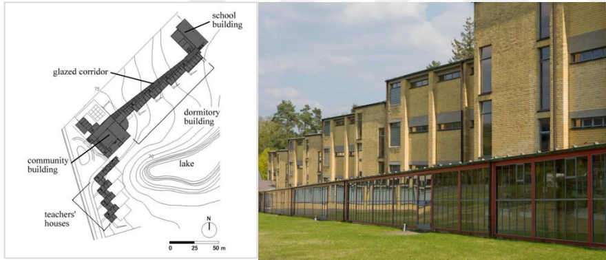
Resim 2.36. Hannes Meyer, Bernau ADGB Ticaret Birliği Okulu, 1928 (Tomita, 2008)
