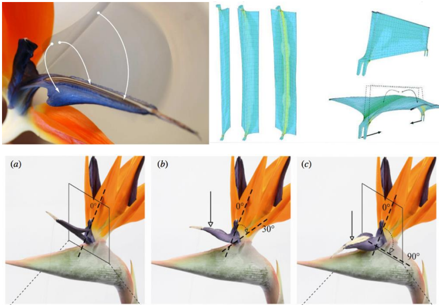
Resim 2.41. Cennet kuşu çiçeğinin hareketi ve çift katmanlı Flectofin® malzemesinin açılıp kapanması (Schleicher vd., 2011)
