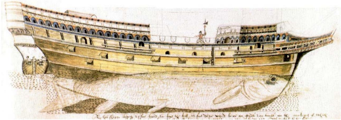
Resim 2.12. Matthew Baker'ın geminin şeklini optimize eden taslağı (Zwick, 2013)
