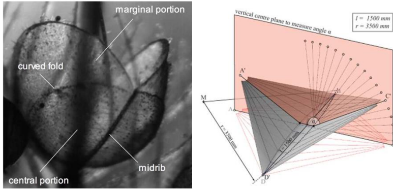
Resim 2.42. Böcek yiyen bitkisi morfolojik özellikleri ve katlanma hareketinin simülasyonu ve açı ölçümü (Schleicher vd., 2011)
