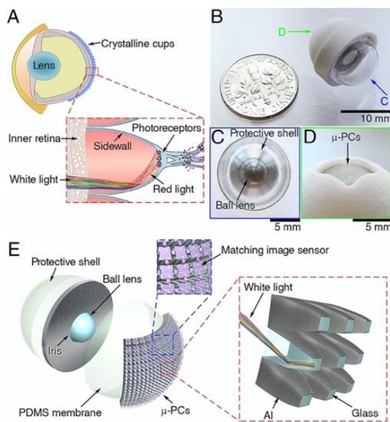
Resim 2.16. Liu, Huang ve Jiang (2016) tarafından geliştirilen yapay göz
