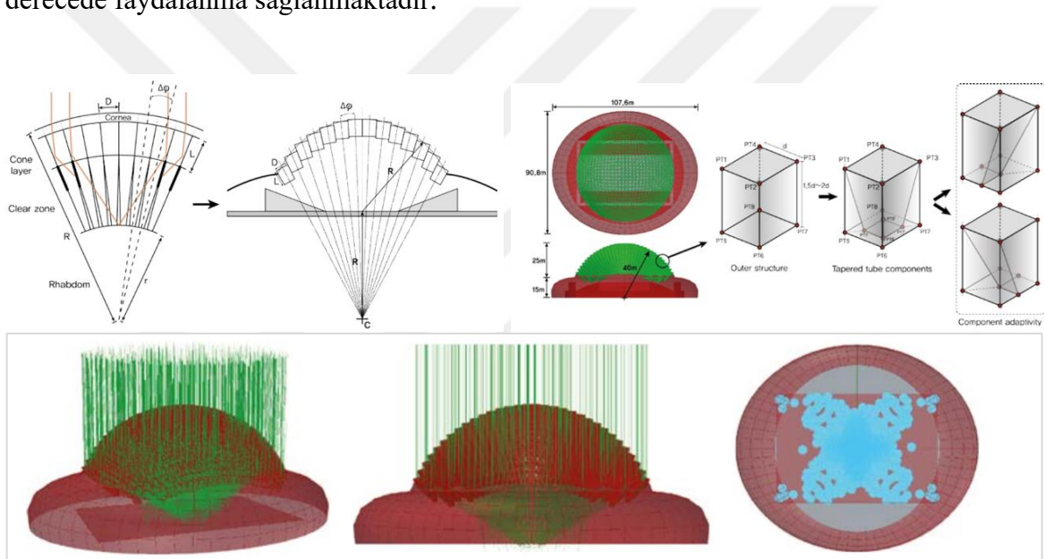
Resim 2.37. Bileşik gözden yola çıkılarak gerçekleştirilen adaptif stadyum cephesi (Park ve Dave, 2014)
