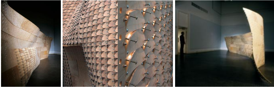
Resim 2.46. Rice Mimarlık Okulunda 2004 yılında gerçekleştirilen Metapatch adlı prototip (Hensel, Menges ve Weinstock, 2013: 170-171; Hensel vd., 2004:82)
