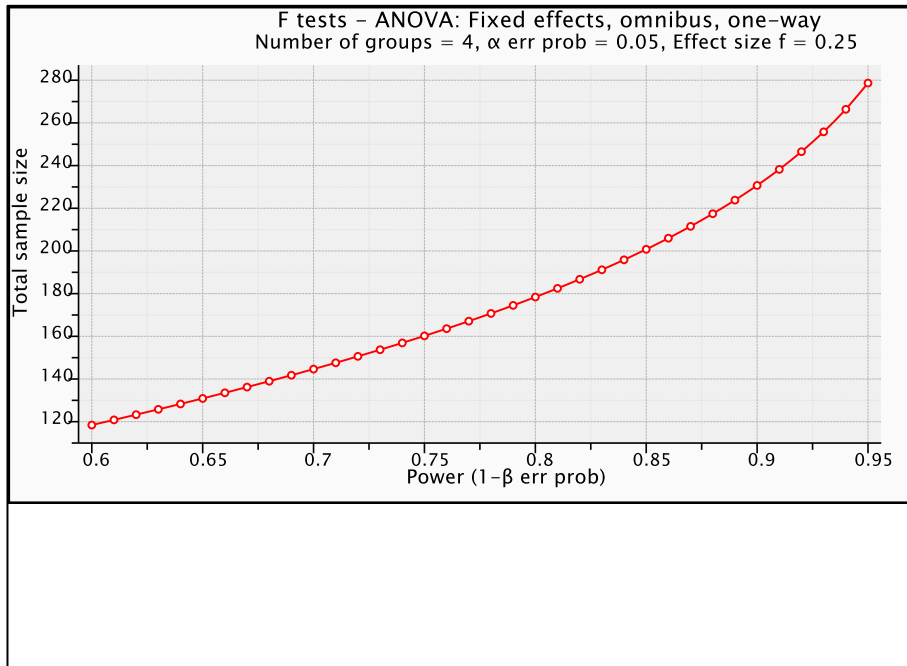
Şekil 3: G*Power analizi
