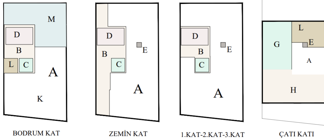
Şekil 4.36. Örnek Yapı (8) Kat Şemaları
