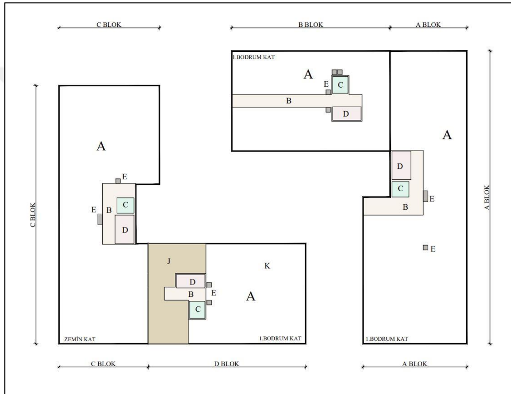
Şekil 4.4. Örnek Yapı (1) 1.Bodrum Kat Şeması
