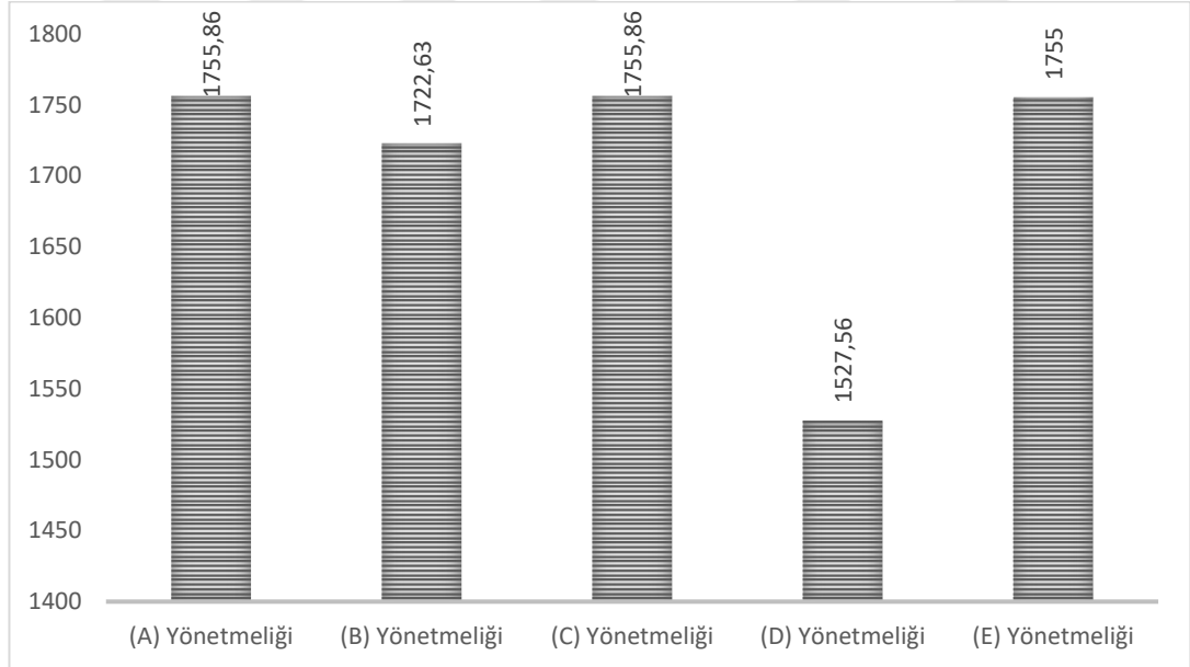
Şekil 4.33. Örnek Yapı (7) Yoğunluk Değişim Grafiği
