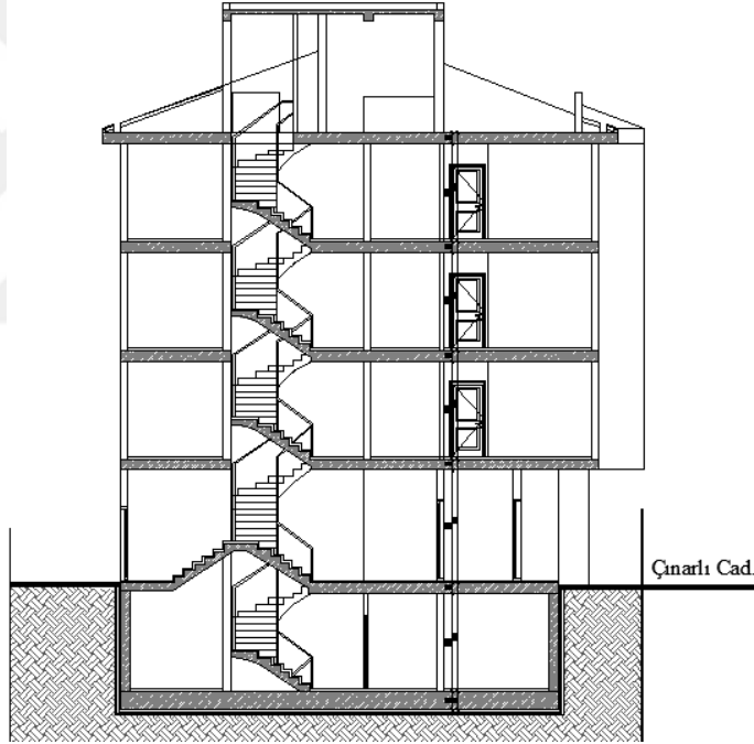
Şekil 4.35. Örnek Yapı (8) Şematik Kesit
