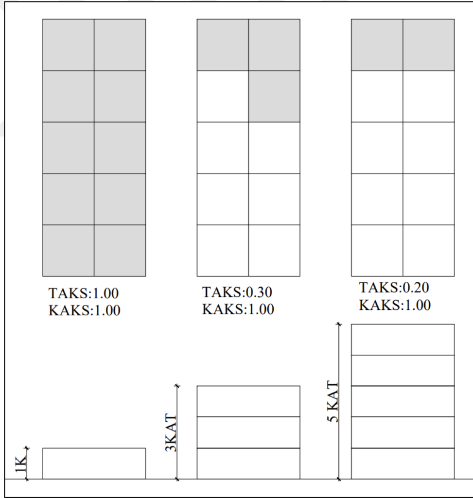
Şekil 3. 2 . TAKS – KAKS Kullanımı Anlatım Şeması
