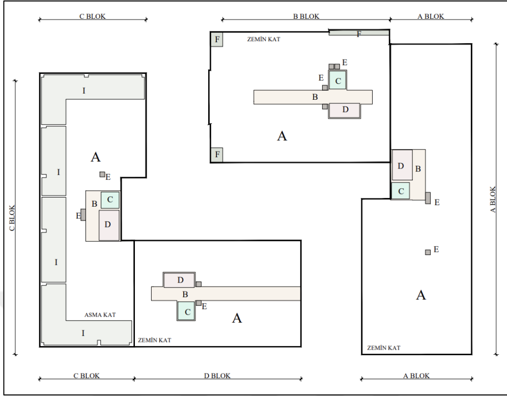
Şekil 4.5. Örnek Yapı (1) Zemin Kat Şeması
