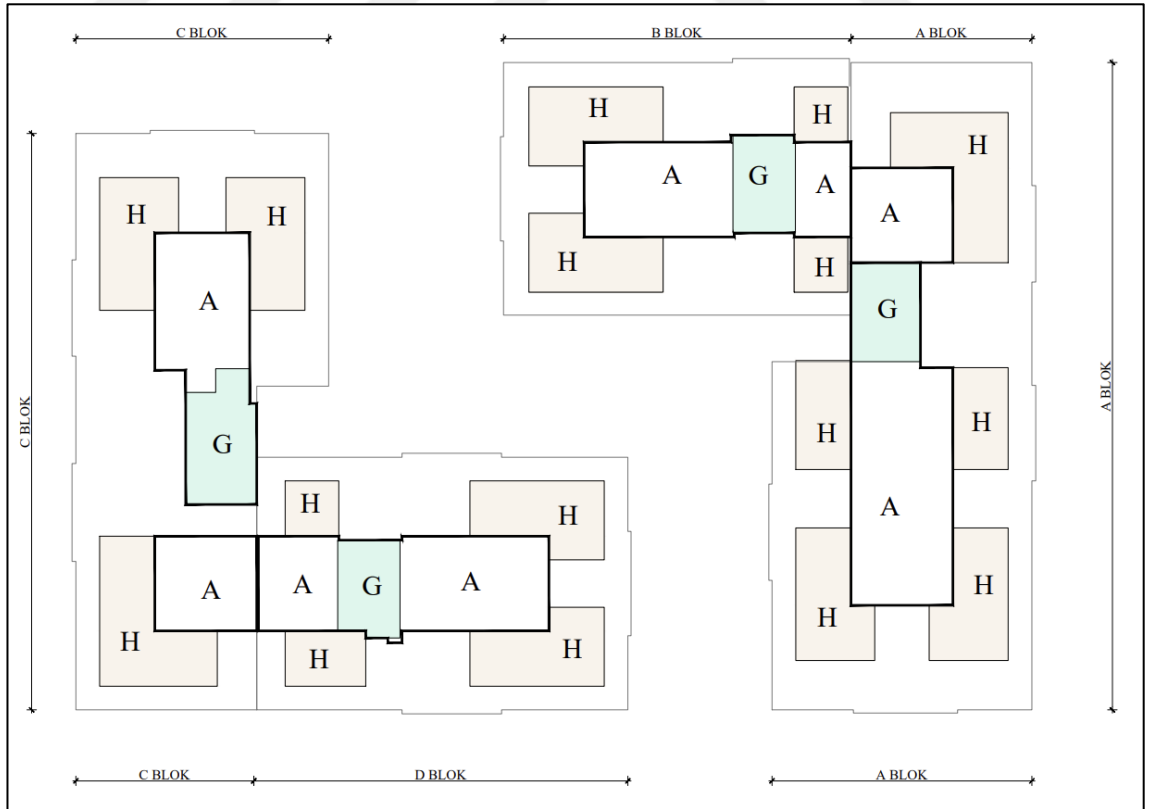
Şekil 4.8. Örnek Yapı (1) Çatı Katı Kat Şeması
