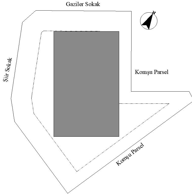
Şekil 4.30. Örnek Yapı (7) Şematik Vaziyet Planı
