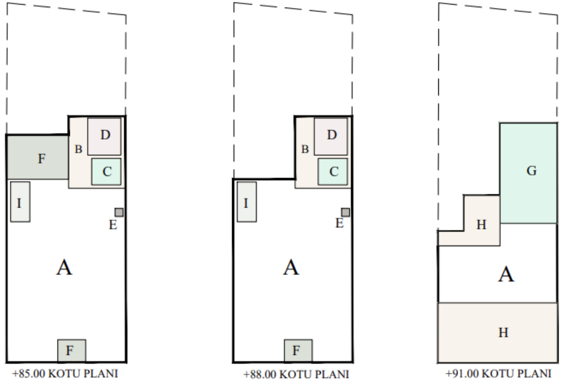
Şekil 4.12. Örnek Yapı (2) Kat Şemaları
