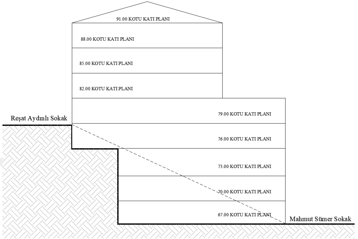
Şekil 4.11. Örnek Yapı (2) Şematik Yapı Kesiti
