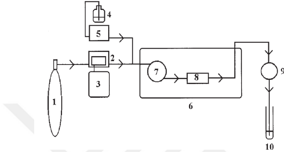
Şekil 2.3. Süperkritik karbondioksit ekstraksiyon sisteminin şematik gösterimi [67]
