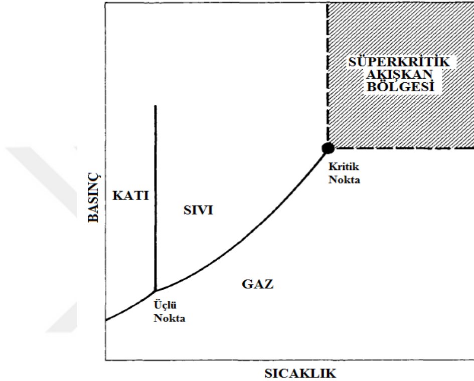
Şekil 2.2. Saf maddenin sıcaklık-basınç diyagramı [17]
