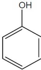
Şekil 2.1. Fenol bileşiği [28]
