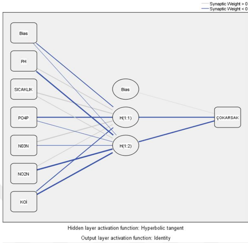
Şekil 4.9. Sölöz, ÇO parametresi için oluşturulan 6-2-1 YSA model 3
