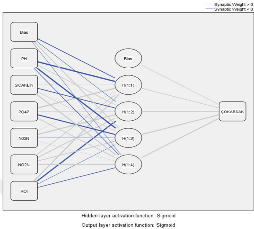
Şekil 4.35. Karasu, ÇO parametresi için oluşturulan 6-4-1 YSA model 4
