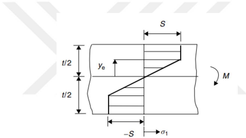
Şekil 3.29 : Elastik, mükemmel plastik sacın gerilme uygulanmadan bükümü durumu için gerilme dağılımı [22]
