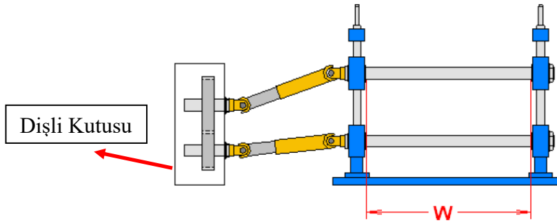
Şekil 3.19 : İstasyonunun millerine bağlı tahrik mili ve dişli kutusu görseli [18]
