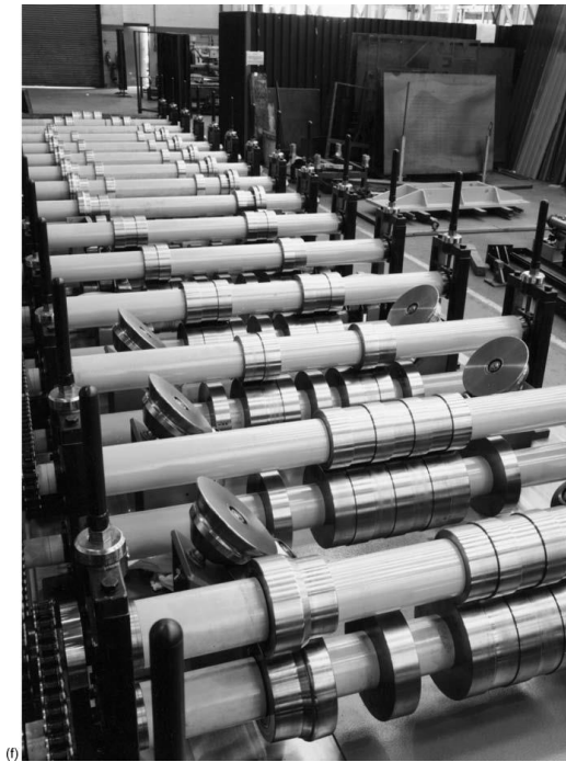
Şekil 3.7 : Rollform hattı üzerinde kullanılan çeşitli makaralar [1]
