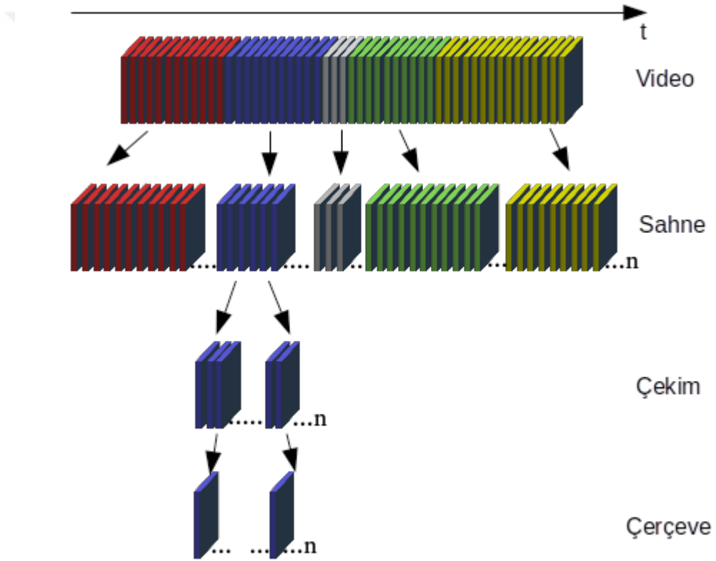
Şekil 3.1 Video içeriğinin hiyerarşik temsili
