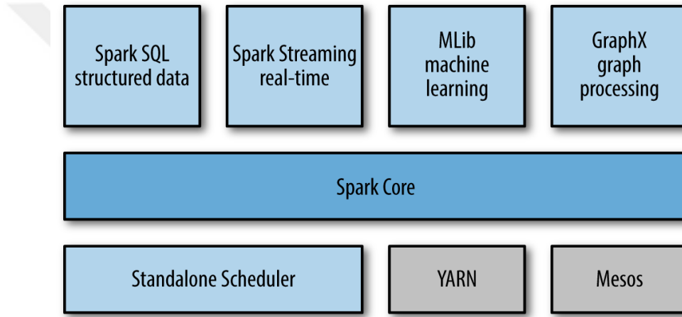
Şekil 3.9 Apache Spark bileşenleri [97]
