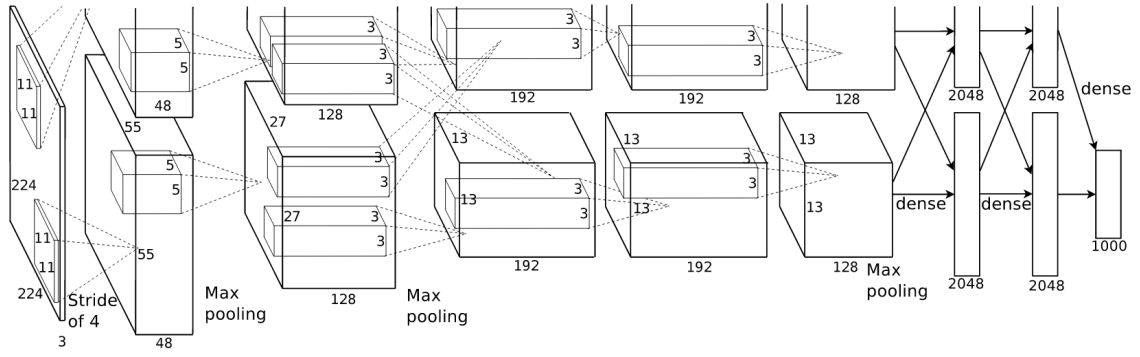
Şekil 4.3 AlexNet mimarisi [14]
