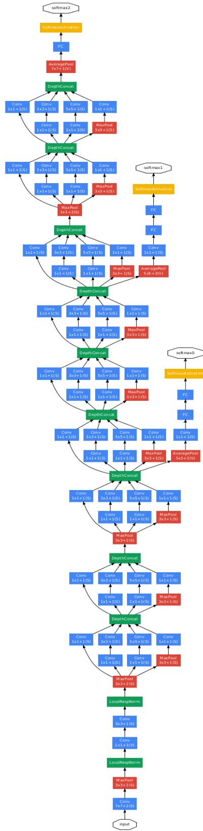
Şekil 4.4 GoogLeNet mimarisi [15]
