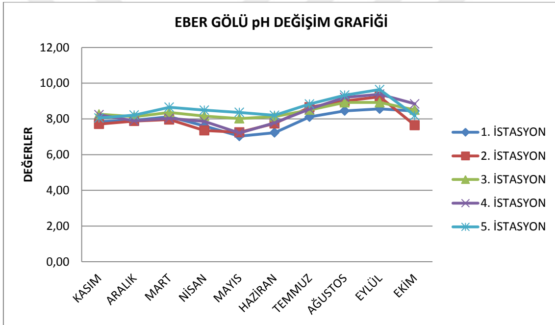
Şekil 4.2 Eber gölü istasyonlarında pH'ın aylara göre değişimi.
