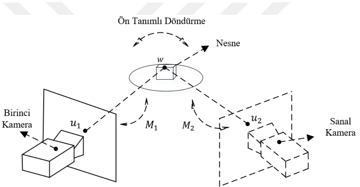
Şekil 2.14. Bir Kamera ve Döndürme İşlemi ile İki Farklı Görüntünün Elde Edilmesi
