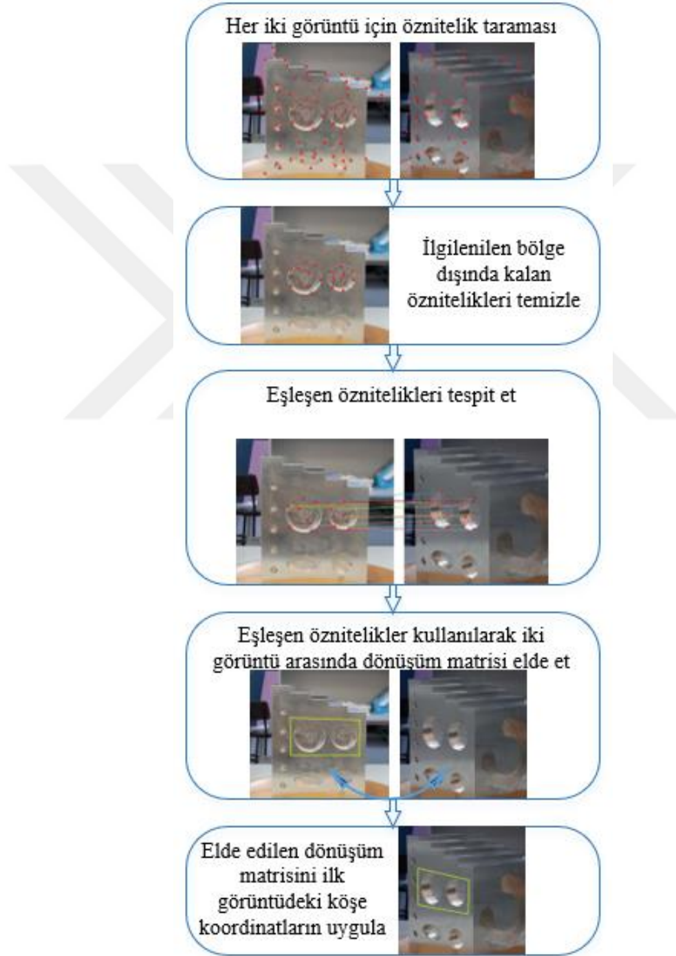
Şekil 2.15. İlgilenilen Bölgenin İkinci Görüntü Üzerinde Yeniden Oluşturulması [47]
