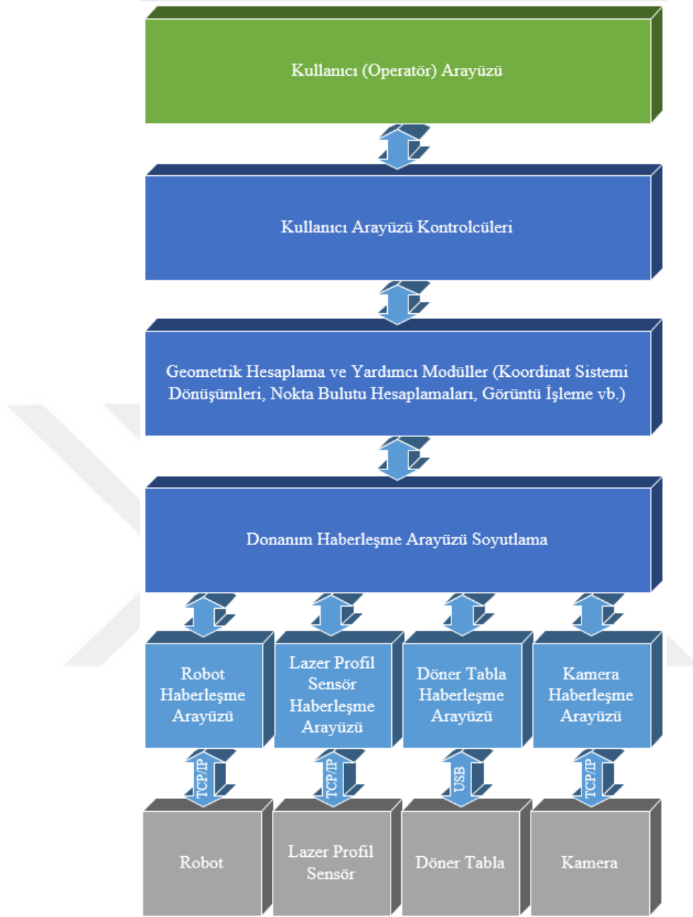
Şekil 3.2. Yazılım Mimarisi
