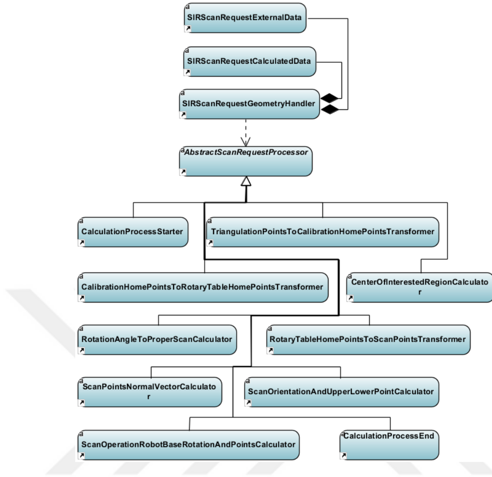
Şekil 3.7. Lazer Tarama Robot Hareket Planı Oluşturma Modülü
