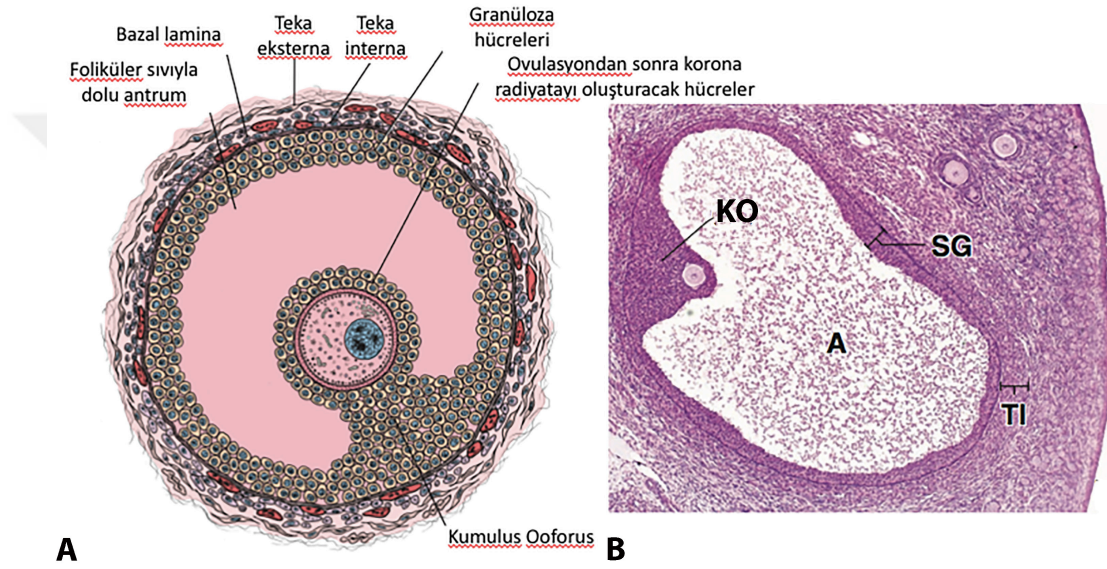
Şekil 2.8. Graaf (olgun) folikülü. A. Kumulus ooforusun içine gömülü oositi içeren geniş antrumlu matür folikülün şematik çizimi. B. Graaf (olgun) folikülün fotomikrografı. A: Antrum; CO: Kumulus ooforus; SG: Stratum granülozum; TI: Teka interna (Ross ve Pawlina, 2013).
