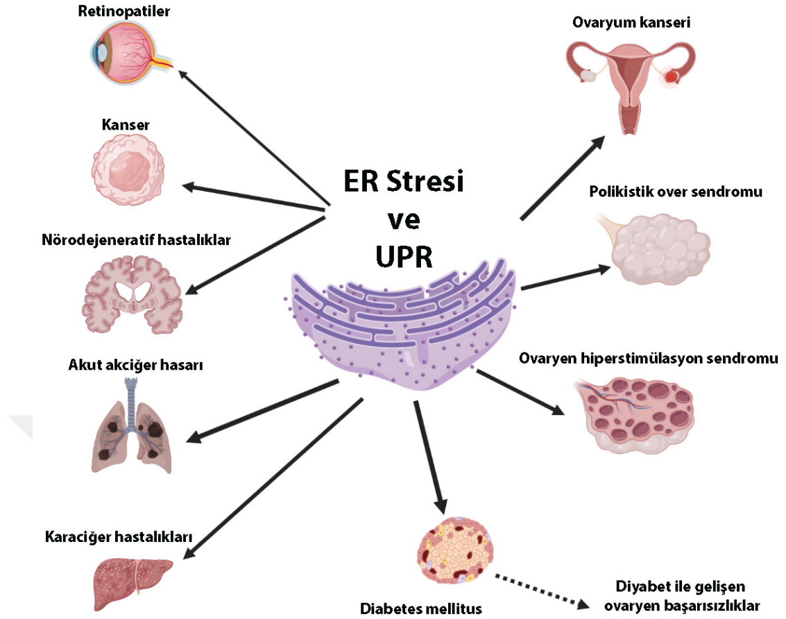
Şekil 2.15. UPR ve ilişkili hastalıklar (Huang ve ark., 2017).
