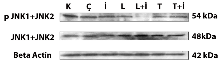
Şekil 4.15. Ovaryum örneklerinin total ve fosforile JNK1+JNK2 protein band görüntüleri. Histogram grafiğinde gösterilen veriler ort \pm SEM olarak ifade edilir. Tek yönlü varyans analizi ve Tukey'in çoklu karşılaştırma testi uygulandı. a P < 0.05 kontrol grubundan farklı olduğunu, b P < 0.05 çözgen grubundan farklı olduğunu, c P < 0.05 DM+ İnsülin grubundan farklı olduğunu, d P < 0.05 DM+Linagliptin grubundan farklı olduğunu, e P < 0.05 DM+ Linagliptin+ İnsülin grubundan farklı olduğunu temsil etmektedir.
