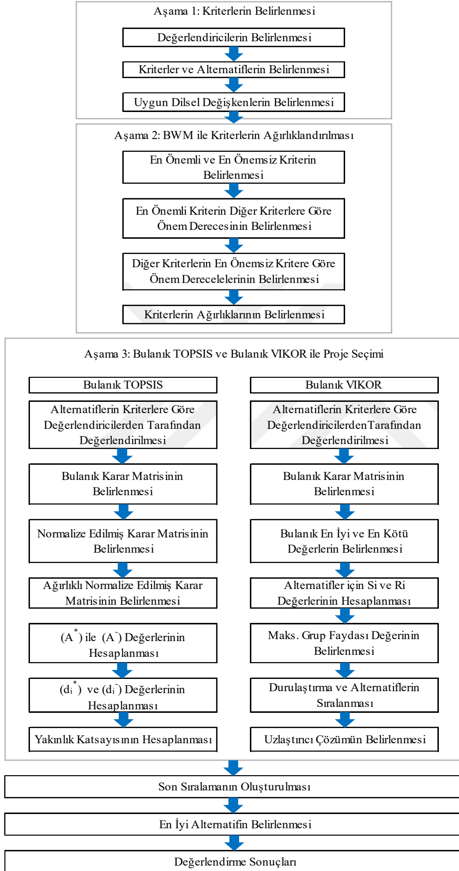
Şekil 3.1. Fizibilite etüdü seçimi için adımlar
