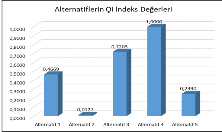
Şekil 4.4. Alternatiflerin Q_i indeks değerleri
