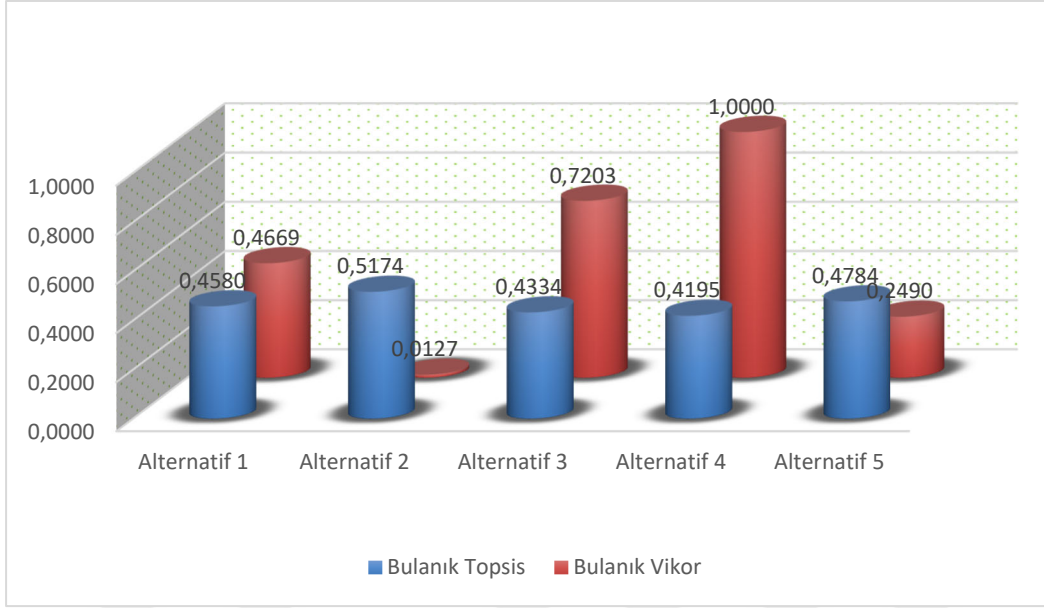
Şekil 4.6. Bulanık TOPSIS ve bulanık VIKOR yöntemlerinin sonuçlarının karşılaştırılması
