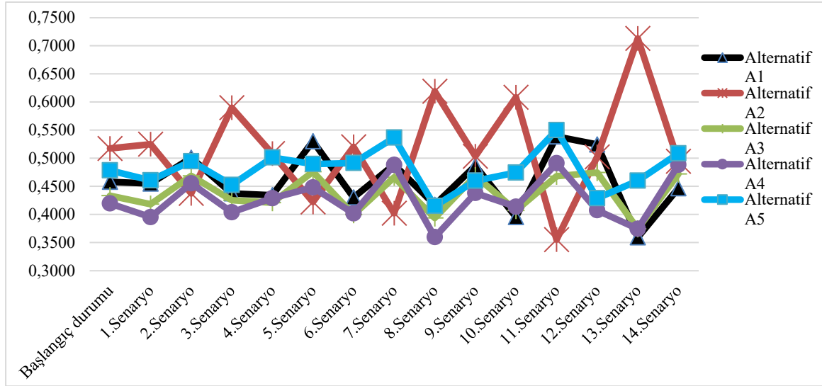
Şekil 4.3. Bulanık TOPSIS duyarlılık analizi sonuçları
