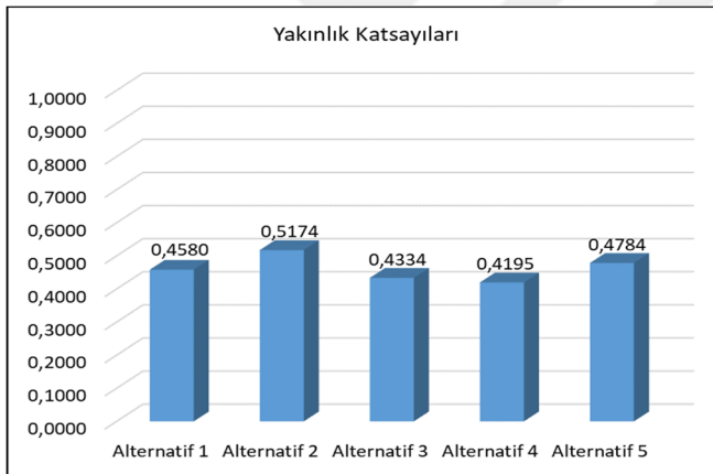
Şekil 4.2. Fizibilite etütlerinin yakınlık katsayıları
