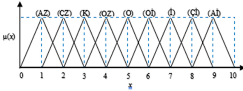
Şekil 4.1. Dilsel değişkenler için üyelik fonksiyonları
