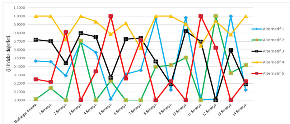
Şekil 4.5. Bulanık VIKOR duyarlılık analizi sonuçları
