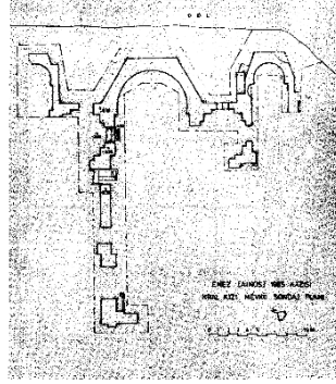
Şekil 3.18. Enez Kral Kızı Mevkii Kilisesi planı (Erzen, 1986)
