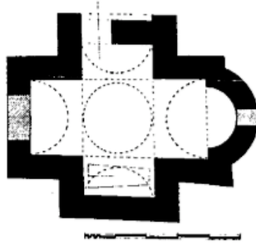
Şekil 3.17. Enez Has Yunus Bey Türbesi planı (Eyice, 1969)
