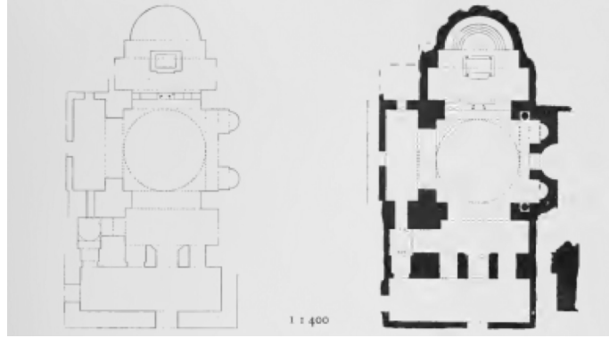
Şekil 3.46. Herakleia katedrali zemin kat planı. Soldaki çizim E. Kalinka'ya, sağdaki Josef Strzygowski'ye aittir (Strzygowski, 1898)
