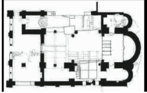
Şekil 3.13. Enez Aya Sofya Kilisesi/Fatih Camii rölövesi (Başaran ve Başaran, 2012)
