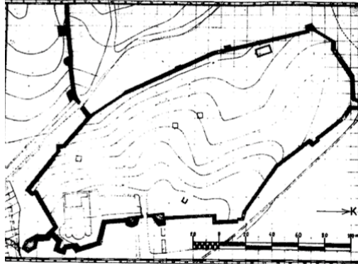
Şekil 3.12. Enez kalesi planı (Erzen, 1974)
