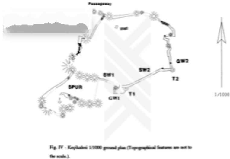
Şekil 3.25. Keçikalesi planı (Kaya, 1997)
