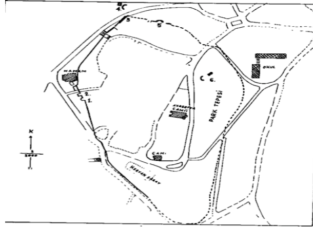
Şekil 3.33. Vize Kalesi planı (Dirimtekin, 1963)
