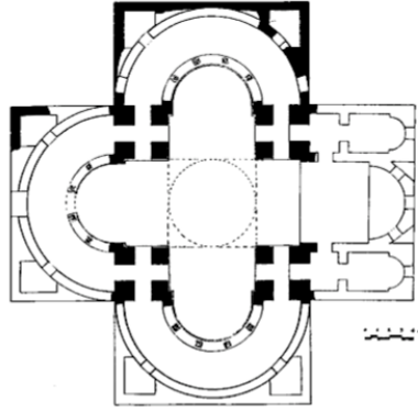
Şekil 3.5. Edirne Aya Sofya Kilisesi'nin Papazotos tarafından Choisy temel alınarak çizilen zemin kat planı (Papazotos, 1992-1994c)
