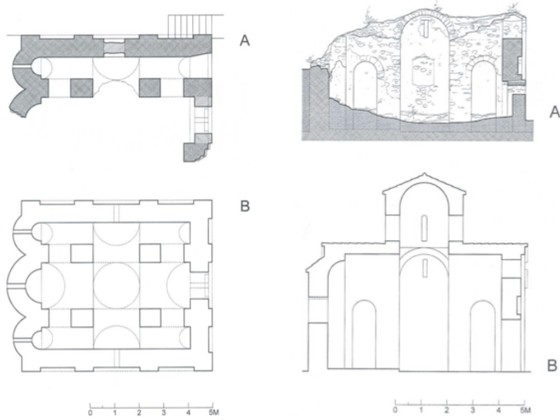
Şekil 3.28. Kaynarca'daki Kimisis tis Theotoku (Panayia) Kilisesi. A. Rölöve B. Restitüsyon (Mamalukos, 2004)
