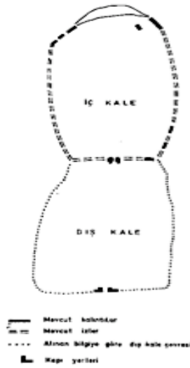
Şekil 3.56. Zesuthera Kalesi planı (Dirimtekin, 1974)
