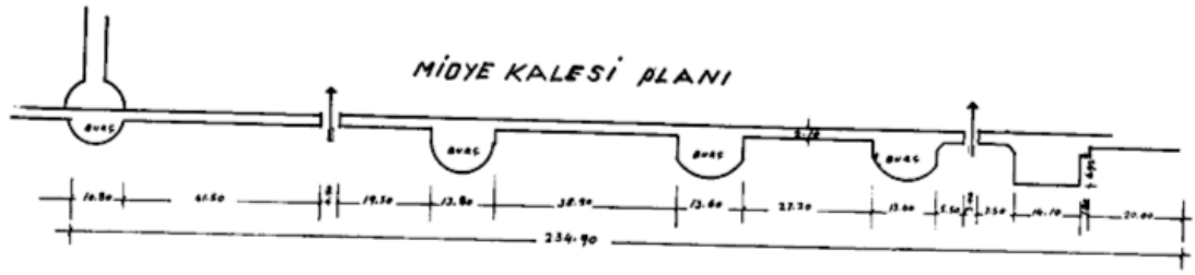
Şekil 3.37. Kıyıköy (Midye) Kalesi planı (Dirimtekin, 1963b)
