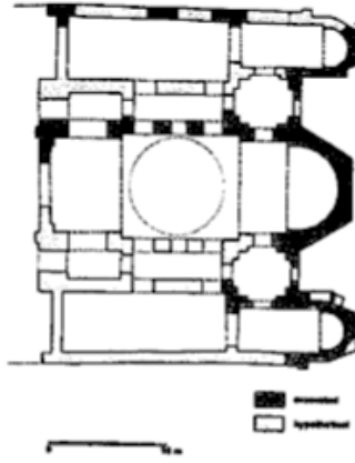
Şekil 3.19. Erzen'in planından hareketle Ousterhout ve Bakirtzis tarafından çizilen Enez Kral Kızı Mevkii Kilisesi'nin hipotetik planı (Ousterhout ve Bakirtzis, 2007)
