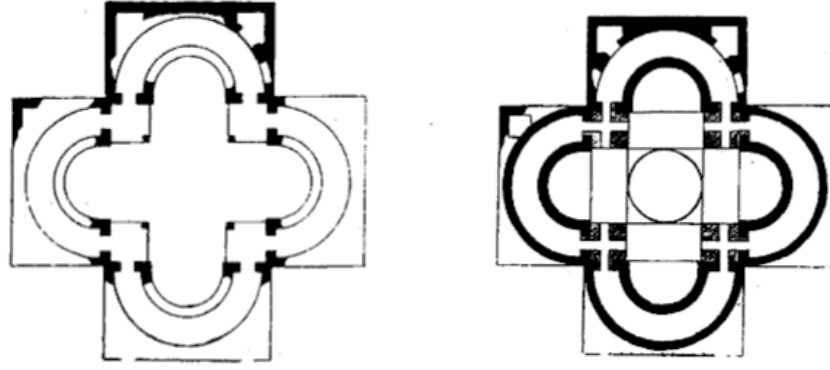
Şekil 3.4. Choisy'ye göre Edirne Aya Sofya Kilisesi'nin ilk dönem planı (sol). Choisy'ye göre yapının sonradan yapılan değişiklikleri gösterir planı (sağ) (Papazotos, 1992-1994c)
