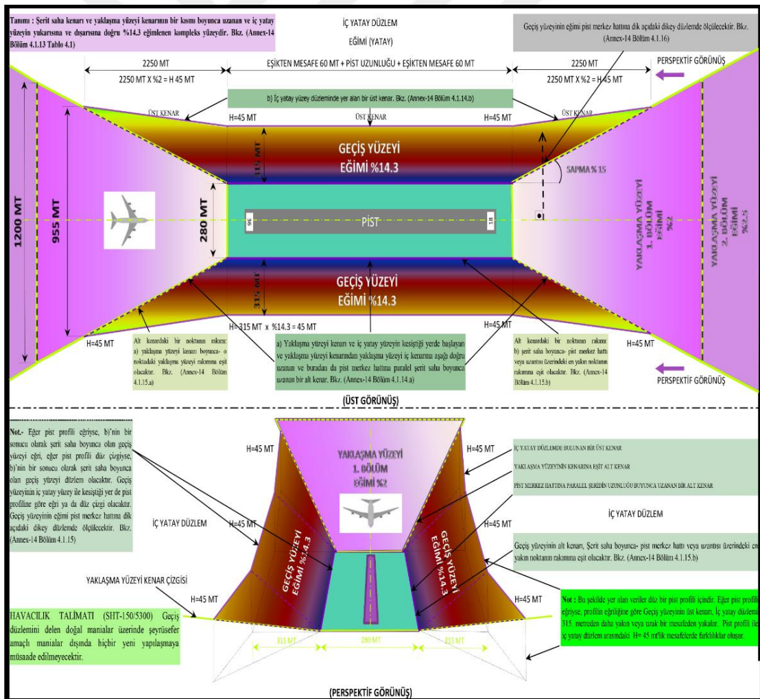
Görsel 8.1. Pist Referans Kodu 3 ve 4 olan pistler için geçiş yüzeyi (DHMI, 2020)
