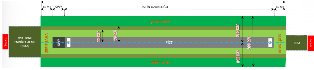
Görsel 2.19. Pist sonu emniyet alanı (RESA) (DHMI ders notu, 2021)
