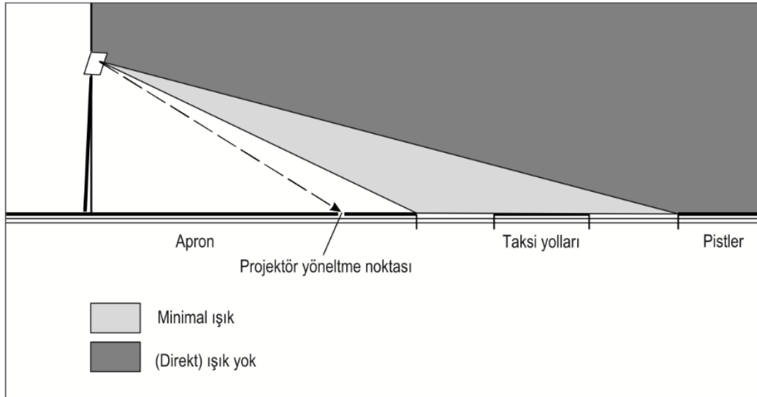
Görsel 2.11. Göz kamaştırıcı ışıktan kaçınmak için yöneltme şekli (ICAO Aerodrome Design Manuel (Doc 9157) Part 4 Visual Aids)
