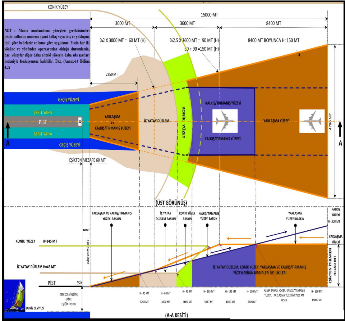
Görsel 9.1. Pist referans kodu 3 veya 4 olan pistler için yüzeylerin birbiri ile ilişkileri (DHMİ, 2020)
