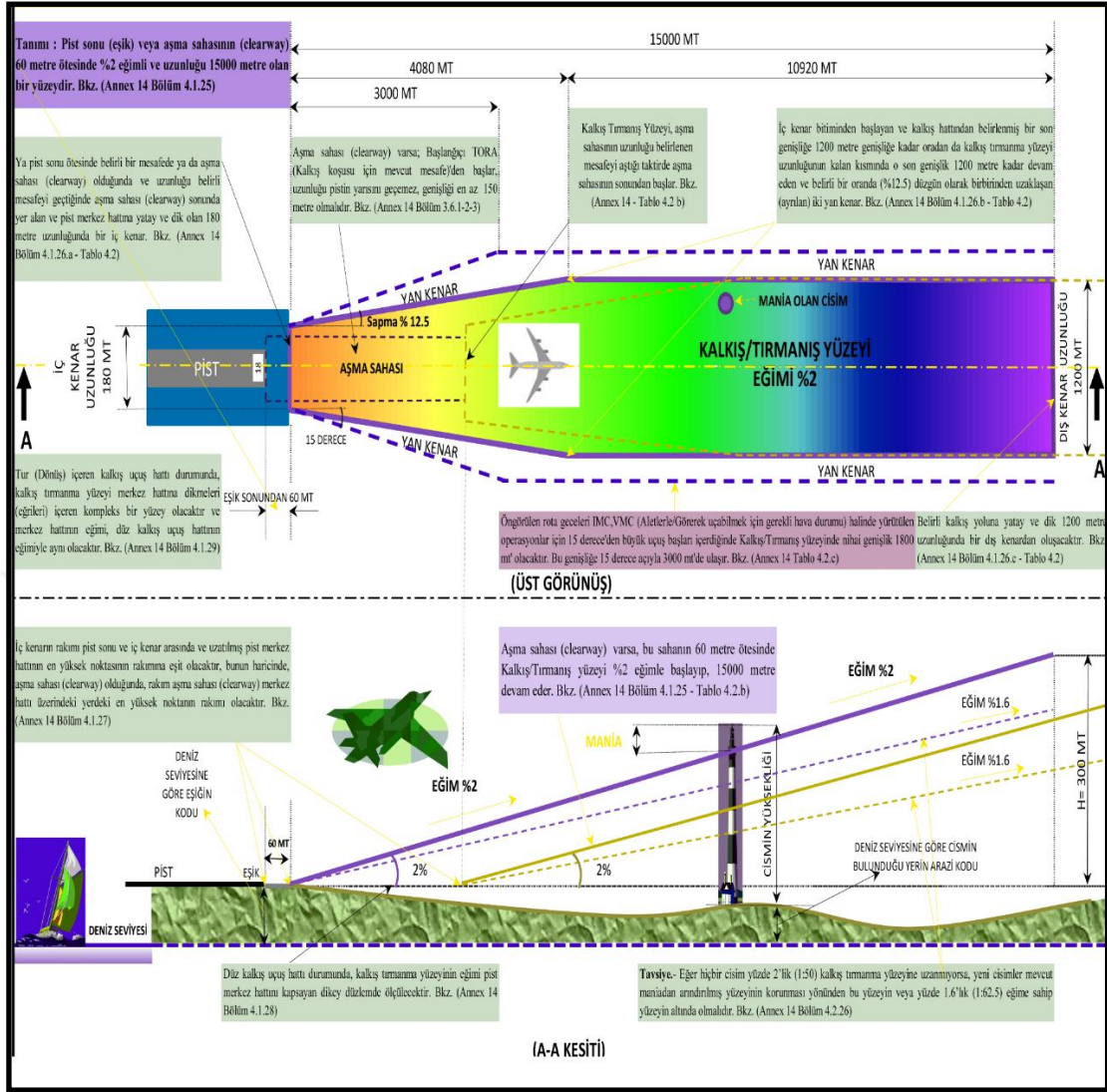
Görsel 8.6. Pist Referans Kodu 3 ve 4 olan pistler için kalkış tırmanış yüzeyi (DHMİ, 2020)
