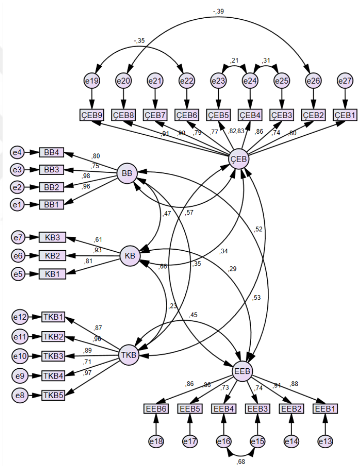
Şekil 5. 1. Cittaslow Katılım ve Farkındalık Ölçeği'nin Path Diyagramı ve Faktör Yükleri
