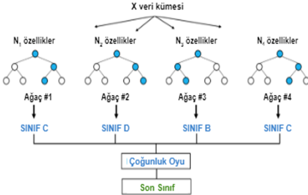
Şekil 2.9 Rastgele orman algoritması örneği (Zengin 2024).
