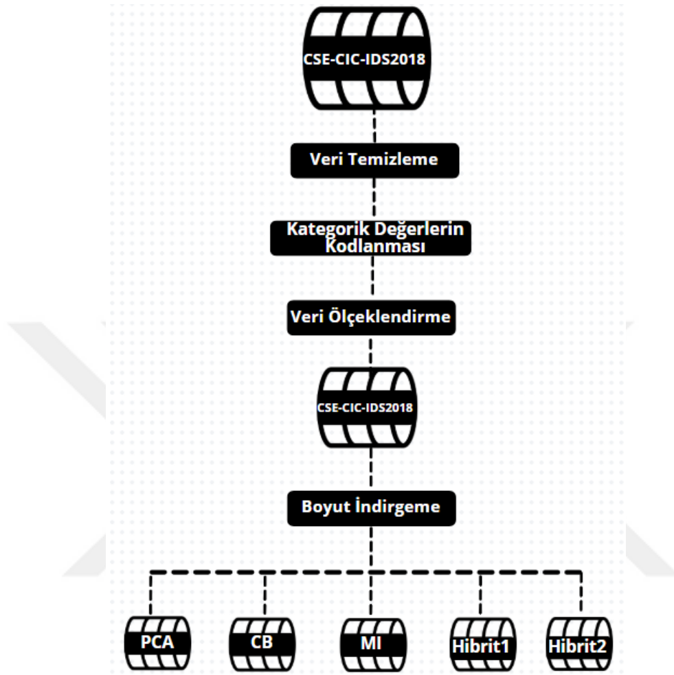
Şekil 3.3 Veri setine uygulanan veri ön işlem adımları
