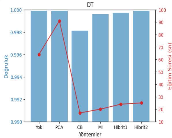
Şekil 4.4 Model başarısı ve eğitim süresi karşılaştırması
