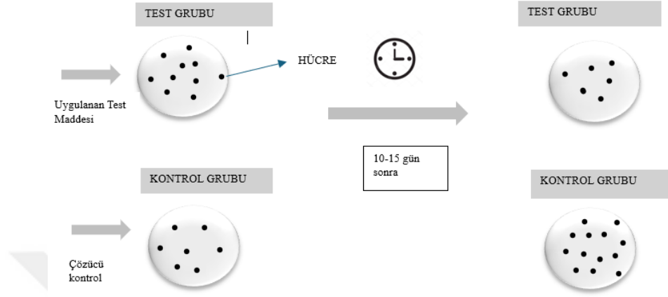
Şekil 2.4: Koloni formasyon deneyinin akışının şematik olarak gösterimi (Gökhaner,2018)
