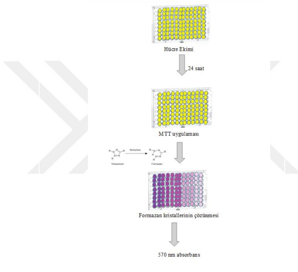
Şekil 2.3: MTT testinin yapılışı (Erkekoğlu ve Baydar,2021)
