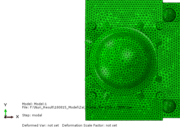
Şekil 5.37 : Sonlu elemanlar modeli plan görünüşü.
