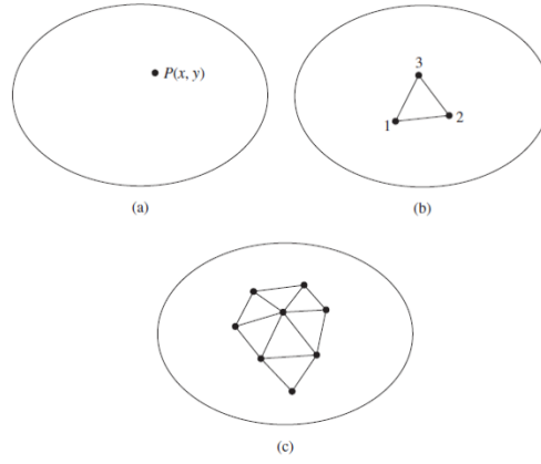
Şekil 3.5 : SEY - Temel kavramlar a) genel bir P(x,y) değişkeni b) üçgen sonlu eleman c) üçgen sonlu eleman ağı [50,74].
