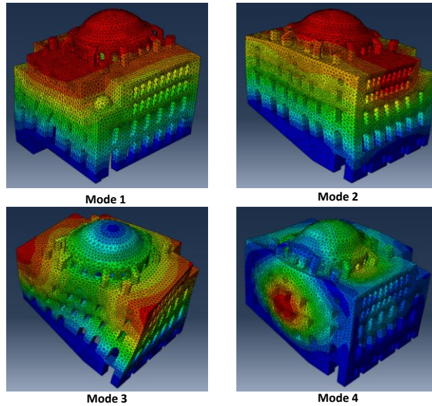
Şekil 5.38 : Yapının ilk 4 mod şekli.
