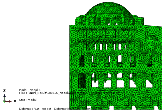
Şekil 5.36 : Sonlu elemanlar modeli doğu cephesi görünüşü.
