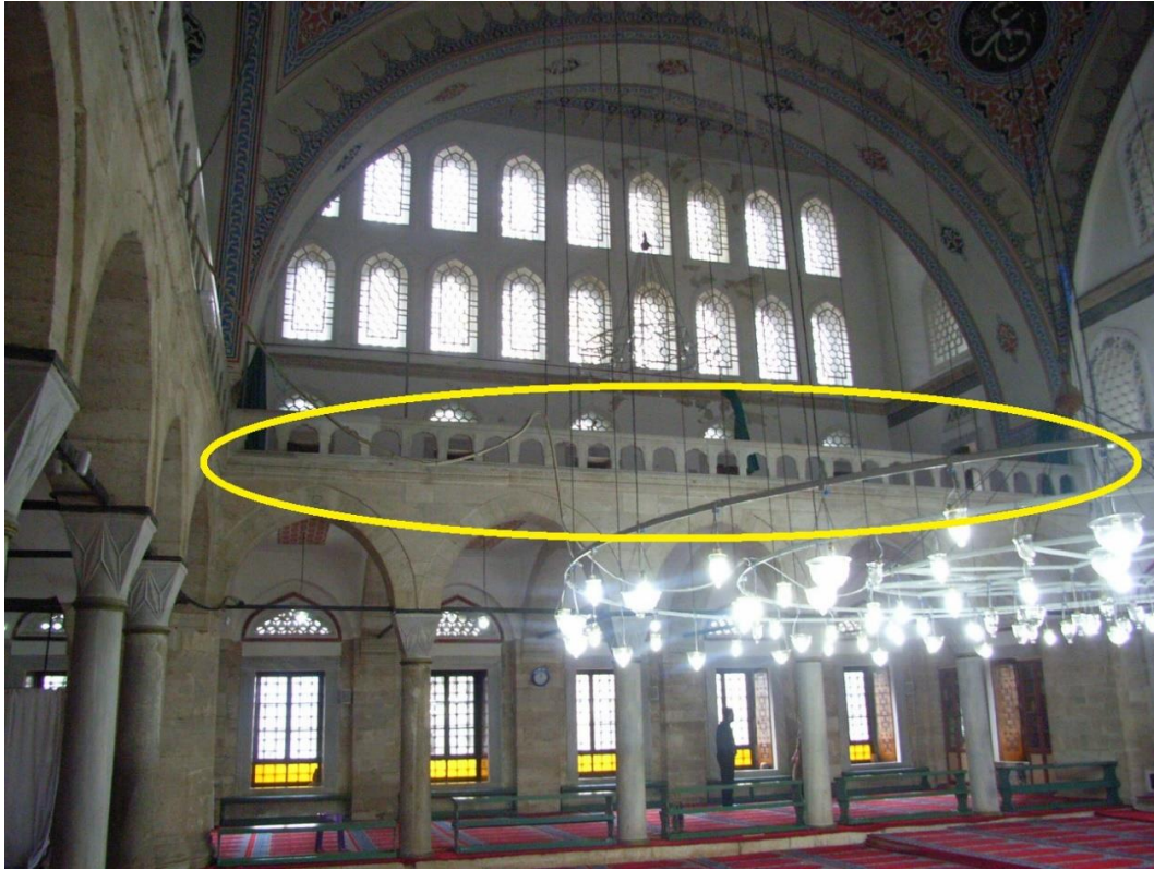
řekil 5.15 : Zal Mahmut Pařa Camii, 1950'li yıllarda kırılan gerginin bulunduğ  b lge.
