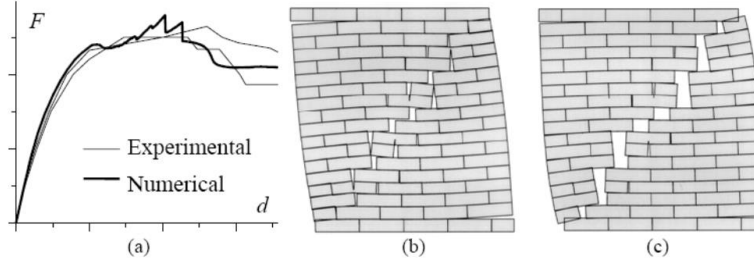
Şekil 3.2 : Yığma duvarın mikro model analizi a) Kuvvet-Yer değiştirme diyagramı b,c) Maksimum ve nihai yüklerdeki deformasyonlar [67].
