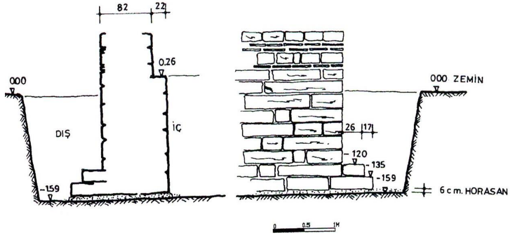
řekil 2.2 : Ayvansaray Hacı Hüsrev Cami 17. Yüzyıl temel detayı [10].
