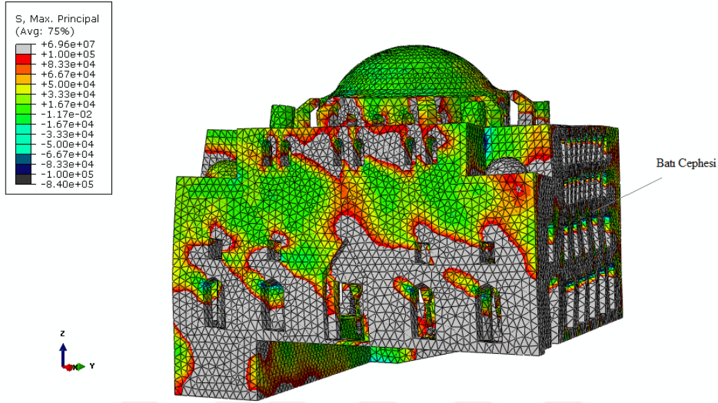
Şekil 5.46 : (G+EY45 0 ) Batı cephesinde meydana gelen 1,78 MPa değerindeki çekme gerilmesi.
