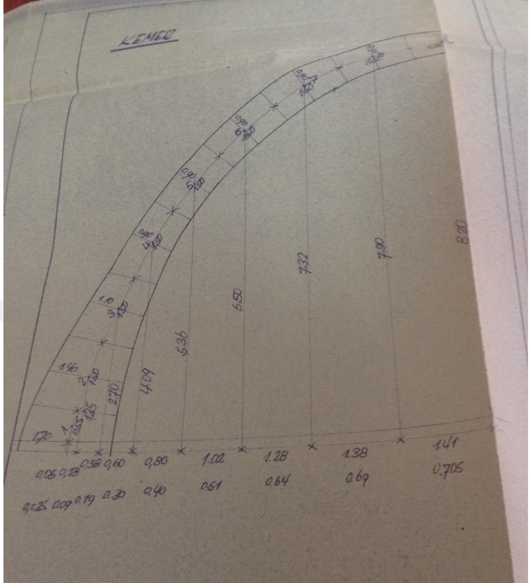
Şekil B.13 : Zal Mahmut Paşa Camii, takviye projesi hesapları (1960) [114].
