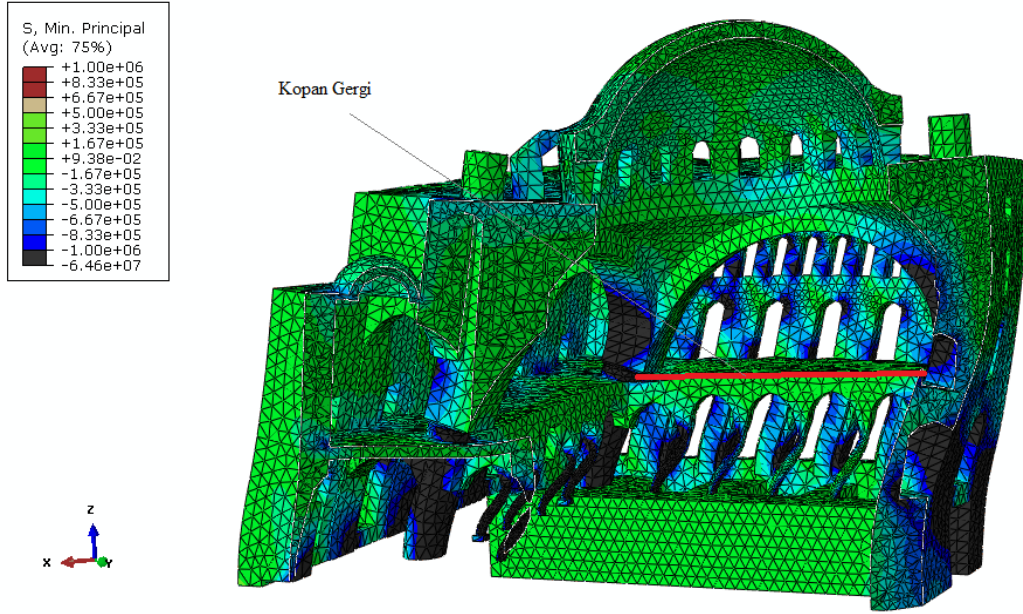
Şekil 5.43 : (G+EY45 0 ) Mahfil katındaki rijit fil ayağında meydana gelen 2,46 MPa değerindeki basınç gerilmesi.
