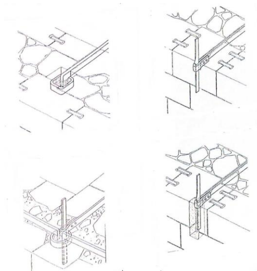
Şekil 2.21 : Mesnetleme sistemleri; simitli mesnetleme, açık kılıçlı mesnetleme, simitli mesnete açık bağlantı [39].
