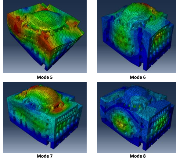
Şekil 5.39 : Yapının 5,6,7 ve 8. Mod şekilleri.
