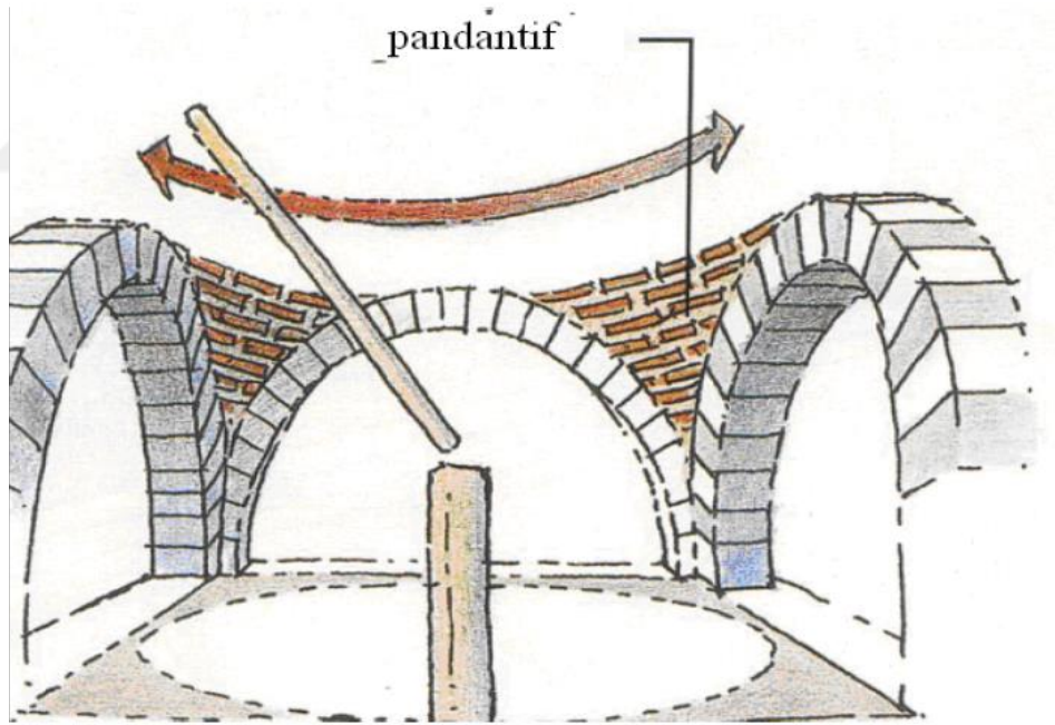
Şekil 2.10 : Pandantif detayı [26].
