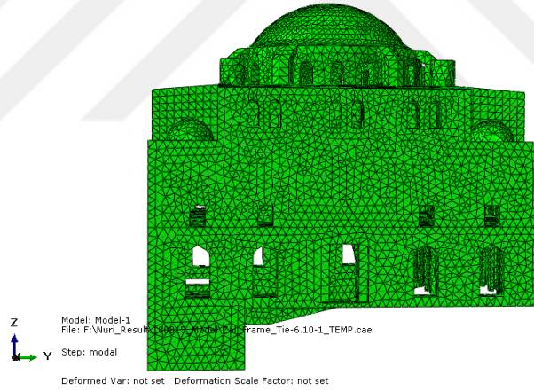
Şekil 5.35 : Sonlu elemanlar modeli güney (giriş) cephesi görünüşü.
