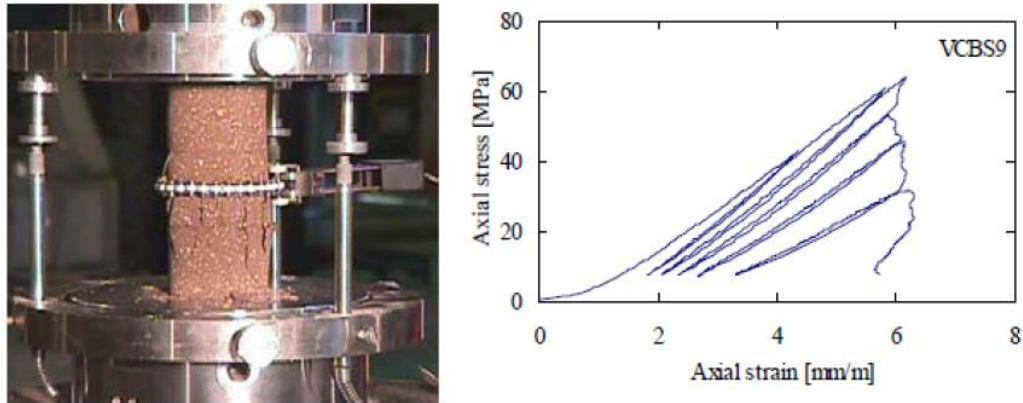
Şekil 2.26 : Silindirik tuğlanın çevrimli basınç deneyi ve tipik gerilme-şekil değiştirme eğrisi [50,67].
