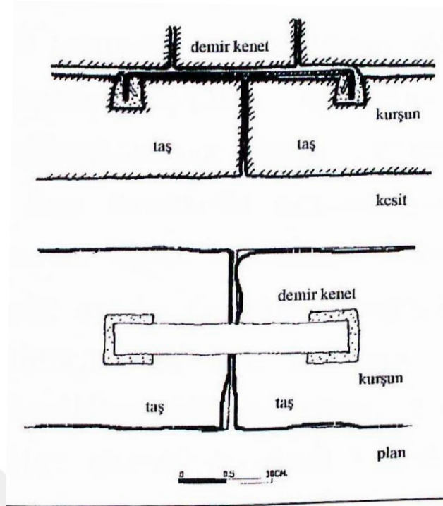
Şekil 2.11 : Demir kenet detayı [10].
