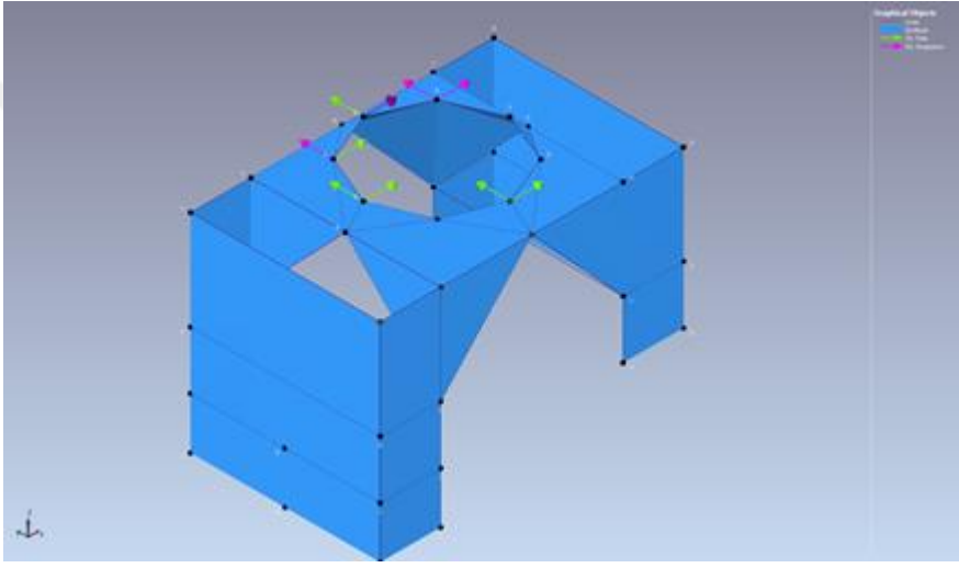
Şekil 5.32 : Zal Mahmut Paşa Camii, Artemis programı basitleştirilmiş modeli.
