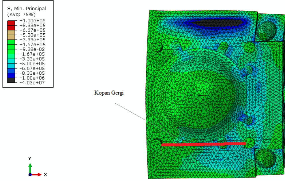
Şekil 5.41 : (G-EX) Batı cephesi çatıda meydana gelen 1,30 değerindeki MPa basınç gerilmesi.
