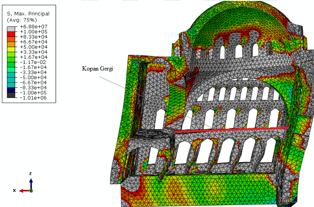
Şekil 5.47 : (G-EX) Kopan gerginin bulunduğu ana kemerde meydana gelen 1,78 MPa değerindeki çekme gerilmesi.
