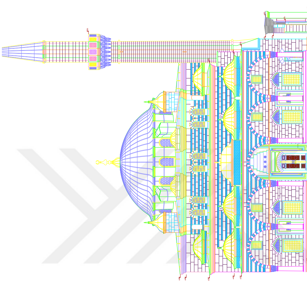
Şekil A.1 : Zal Mahmut Paşa Camii, kuzey cephesi rölevesi.
