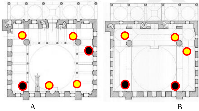
Şekil 5.25 : İvmeölçer yerleşim planı, a) cami giriş katı b) cami kadınlar mahfili katı
