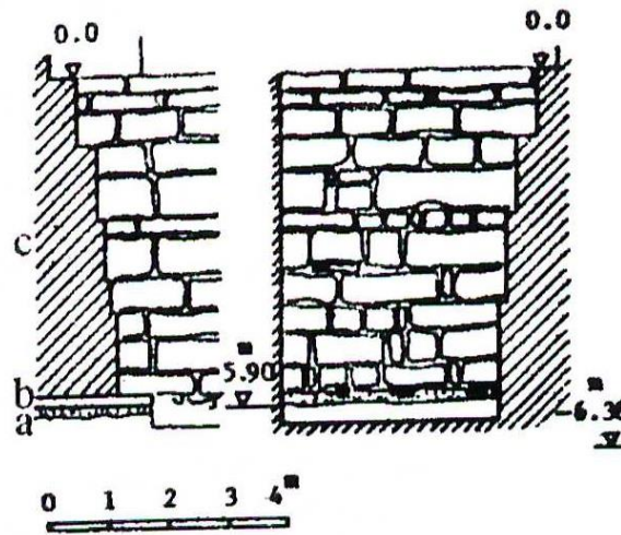
Şekil 2.1 : Süleymaniye Camisi temel kesiti. Kible duvarlarının kuzey ucunda açılan sondaj çukurunda: a. Kum katmanı, b. Ahşap ızgara, c. Anpatmanlı temel [11].
