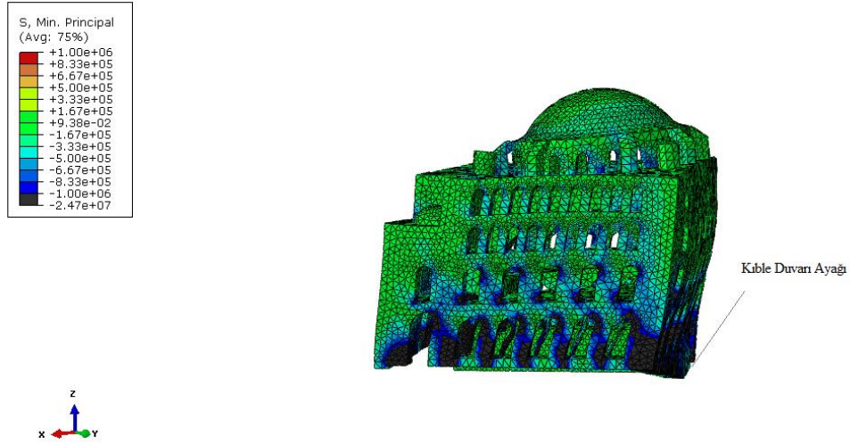
Şekil 5.45 : (G-EY45 0 ) Kible duvarı ayaklarında meydana gelen 2,7 Mpa değerindeki basınç gerilmesi.
