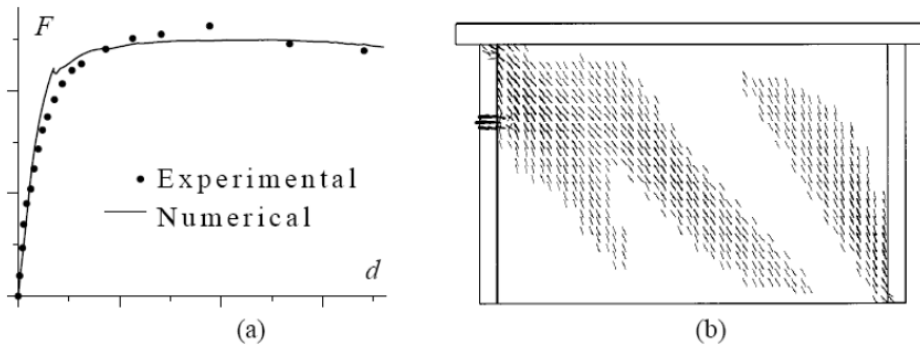
Şekil 3.3 : Yığma duvar makro model analizi a) kuvvet-yer değiştirme diyagramı b) nihai yükte deformasyon şekli [67].
