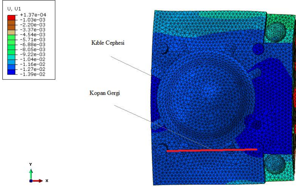
Şekil 5.48 : (G-EX) Kible duvarı tepe orta noktasında meydana gelen 0,0013m değerindeki yer değiştirme.
