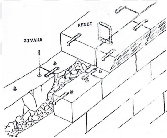
Şekil 2.19 : Yanaşık derzli kesme taş duvar örgüsü [39].
