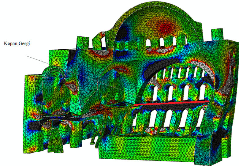
Şekil 5.51 : (G+EY) Batı cephesi meydana gelen 0,85 MPa değerindeki kayma gerilmesi.
