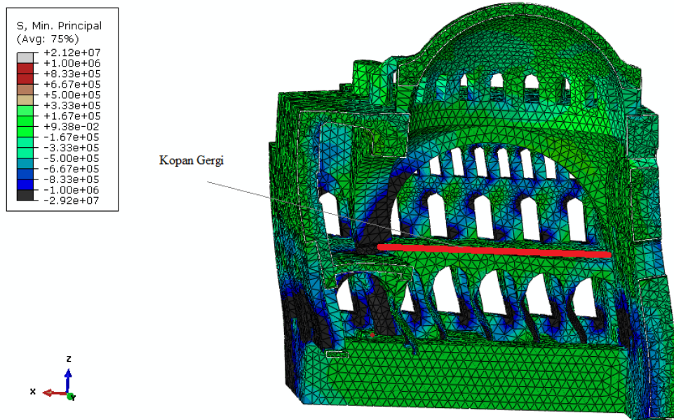
Şekil 5.42 : (G+EX) Giriş katında fil ayağında meydana gelen 3,78 MPa değerindeki basınç gerilmesi.
