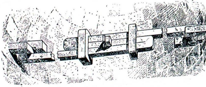
Şekil 2.20 : Fatih Medresesi (1463-70) demir gergi detayı [46].
