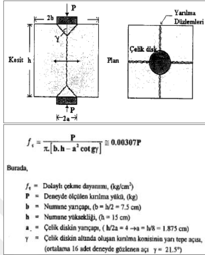
Şekil 2.24 : Çift zımbalama deneyi ile dolaylı çekme dayanımının belirlenmesi [59].
