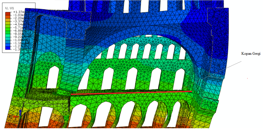
Şekil 5.49 : (G-EX) Kopan gerginin ana kemerinde meydana gelen 0,0012m değerindeki yer değiştirme.
