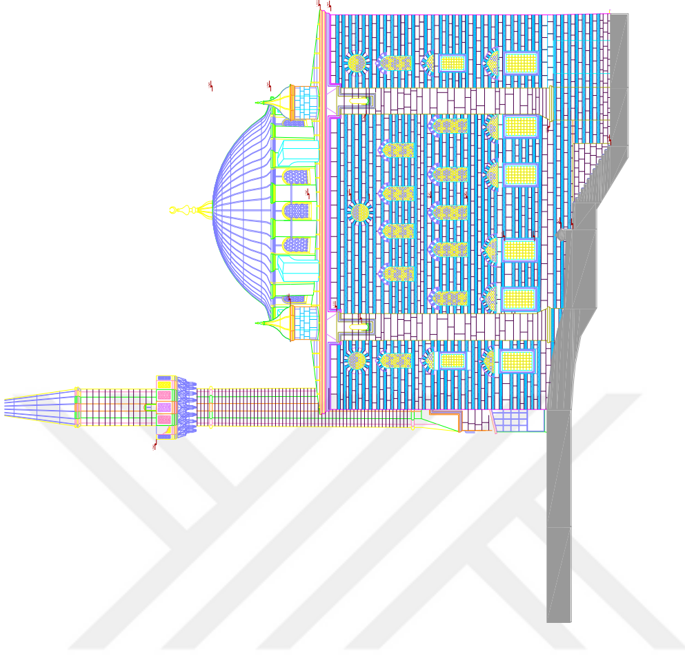
Şekil A.3 : Zal Mahmut Paşa Camii, güney cephesi rölevesi.
