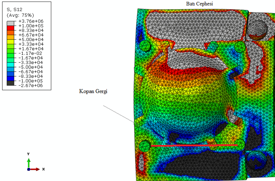
Şekil 5.50 : (G-EX) Batı cephesi çatıda meydana gelen 1,03 MPa değerindeki kayma gerilmesi.
