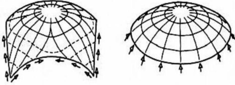
Şekil 2.3 : Kubbe yük şeması [20].
