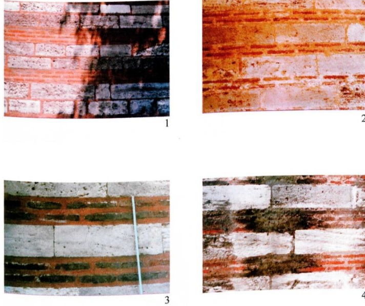
Şekil 2.13 : Tuğla taş almalı duvar örgüsü. 1- Zincirlikuyu Atik Ali Paşa Camisi (1511), 2- Silivrikapı Hadım İbrahim Paşa Camisi (1551), 3- Eyüp Zal Mahmut Paşa Camisi (1580), 4- Beşiktaş Sinan Paşa Camisi (1555) [6].
