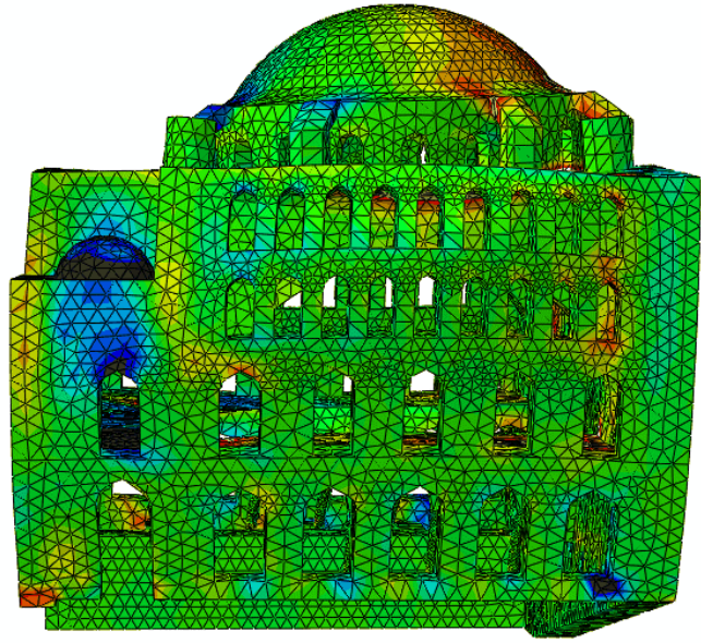
Şekil 5.51 : (G+EY) Batı cephesi meydana gelen 0,85 MPa değerindeki kayma gerilmesi.
