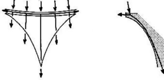
Şekil 2.6 : Pendantif yük şeması [21].
