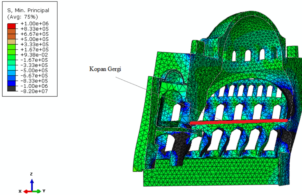
Şekil 5.44 : (G+EY45 0 ) Kopan gerginin bulunduğu ana kemerde meydana gelen 1,65 Mpa değerindeki basınç gerilmesi.
