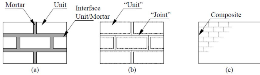
Şekil 3.1 : Model yaklaşımları. a) detaylı mikro b) basit mikro c) makro modelleme [67].
