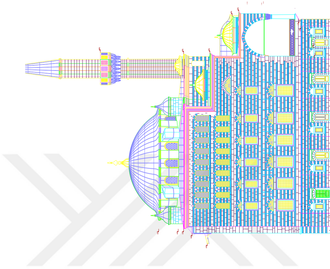
Şekil A.2 : Zal Mahmut Paşa Camii, doğu cephesi rölevesi.
