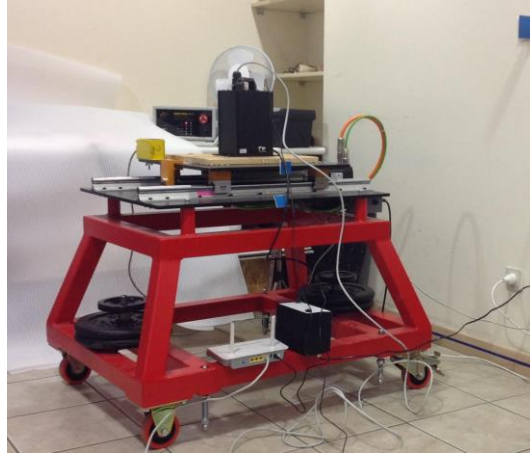
Şekil 5.23 : Sarsma tablası üzerinde test edilen ivmeölçer.
