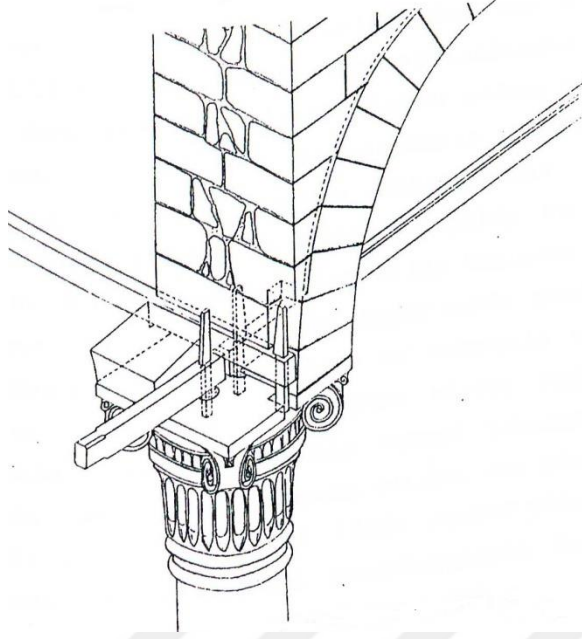
Şekil 2.22 : Topkapı Sarayı Hazine revağında demir gergilerin sütun başlığına mesnetlenme detayı [39].
