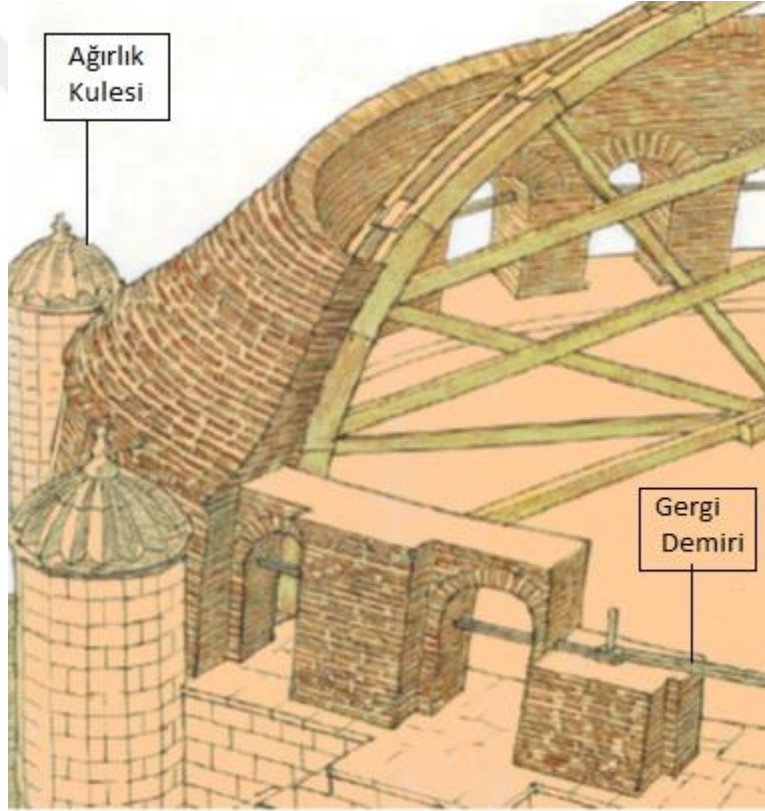
Şekil 2.4 : Kubbe detayı [26].
