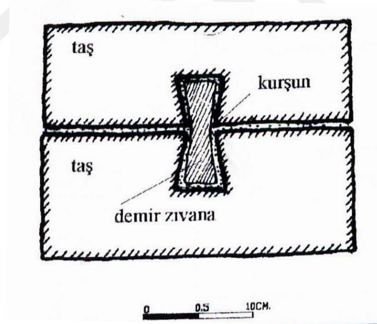
Şekil 2.12 : Demir zivana detayı [10].
