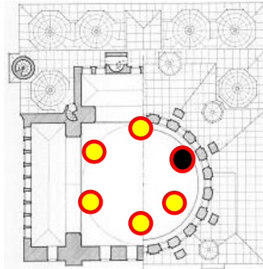
Şekil 5.26 : İvmeölçer yerleşim planı, cami kubbesi.
