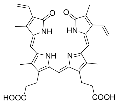
Biliverdin 2
