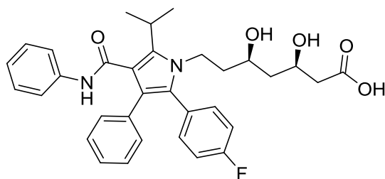
Atorvastatin
