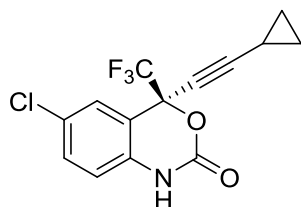
Efavirenz 41
