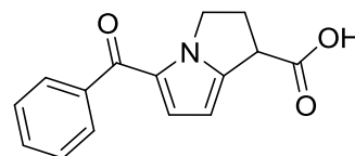
Ketorolac
