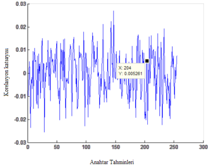
Şekil 6.9 : AES algoritmasının maskeli gerçekleştirilmesi için kombinezonsal yöntem kullanılarak elde edilen korelasyon sonucu
