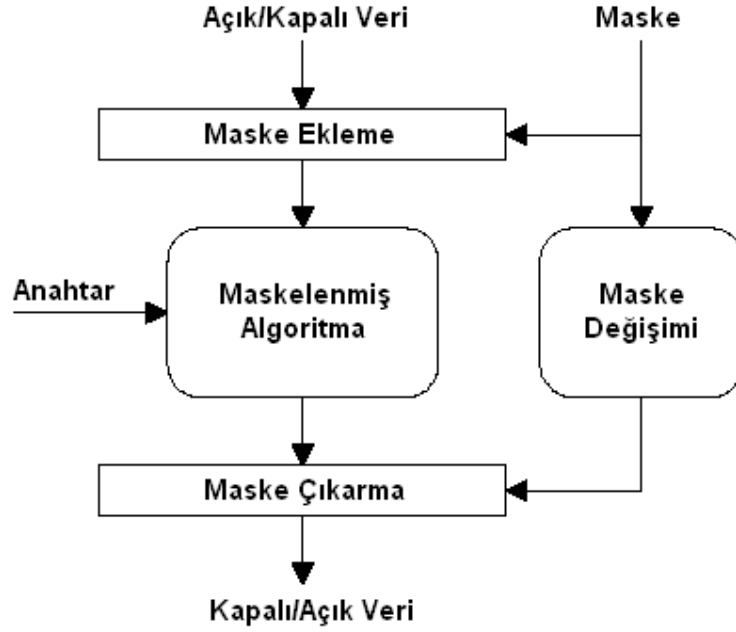
Şekil 3.7 : AES Algoritması maskeli gerçeklemesi [11]
