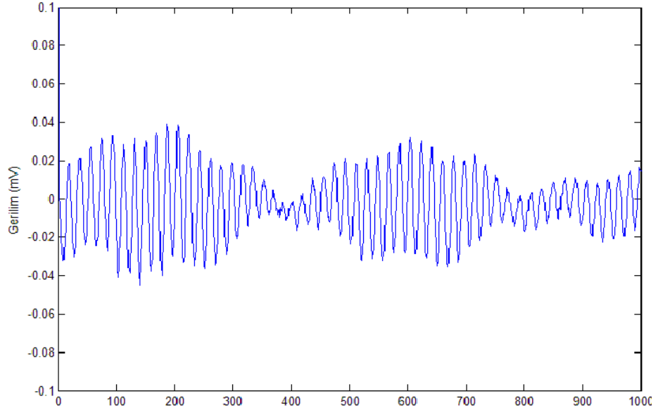
Şekil 2.2 : Tasarlanmış EM alıcısı ile alınmış işaret
