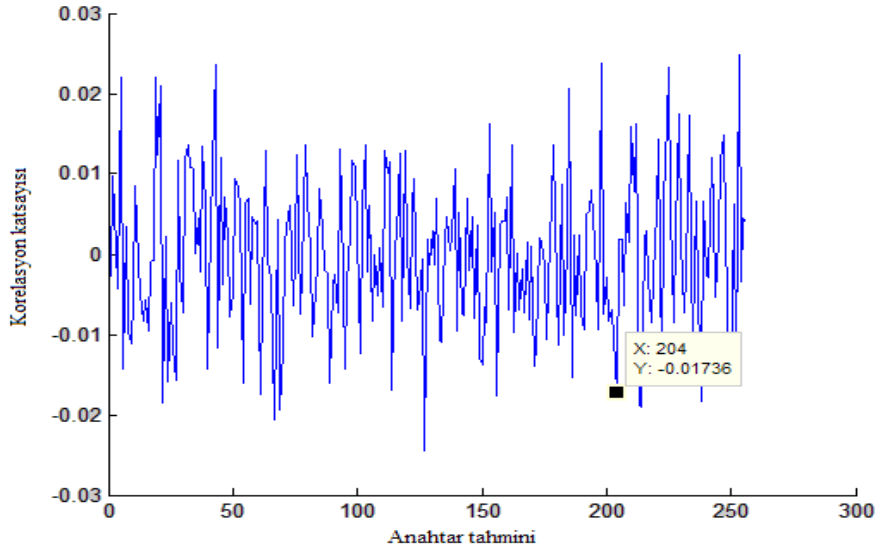
Şekil 6.7 : AES algoritmasının maskeli gerçekleştirilmesi için kümülanlı kullanılarak oluşturulan korelasyon sonucu
