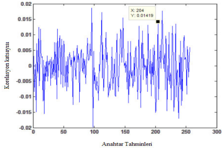
Şekil 6.10 : AES algoritmasının maskeli gerçekleştirilmesi için kombinezonsal yöntem ve kümülanlı kullanılarak oluşturulan korelasyon sonucu
