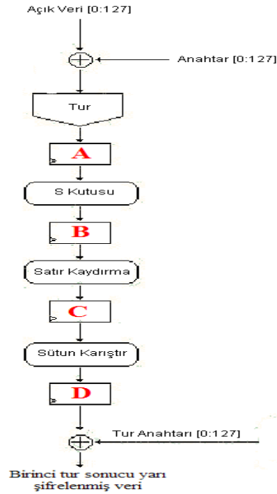
Şekil 3.9 : AES algoritması ilk tur işlemleri
