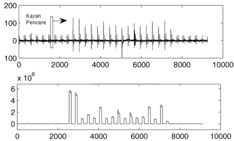
Şekil 2.1 : Orijinal ve kümülanı alınmış işaret
