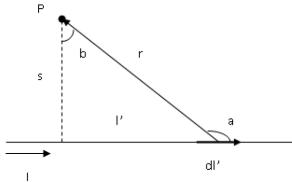
Şekil 2.4 : Üzerinden akım geçirilen telin s uzaklığındaki manyetik davranışı
