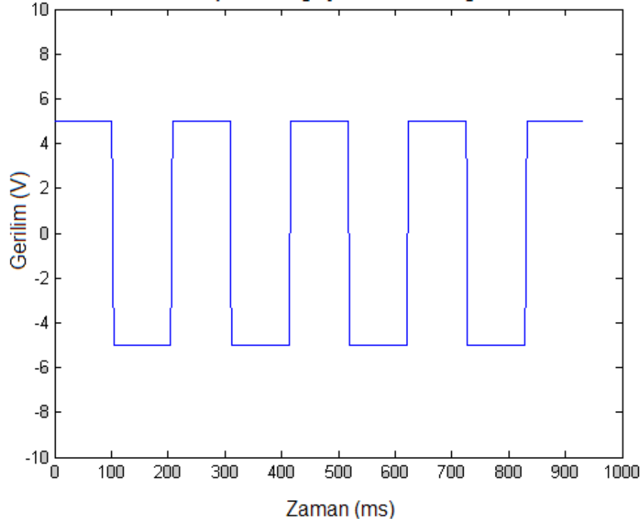
Şekil 4.4 : Akım yolundan geçirilen kare dalga
