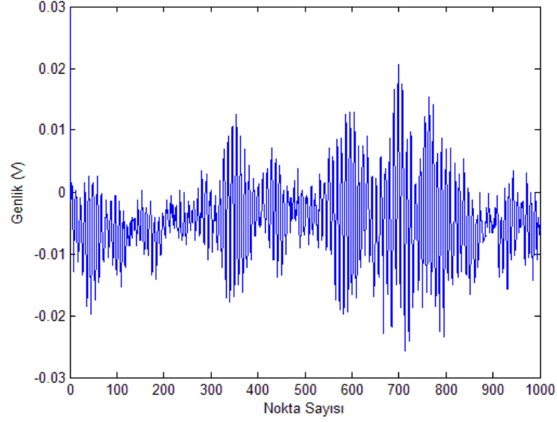
Şekil 6.8 : AES algoritmasının maskeli gerçeklemesi için bayt yer değiştirme işlemi kaydedici ölçümü
