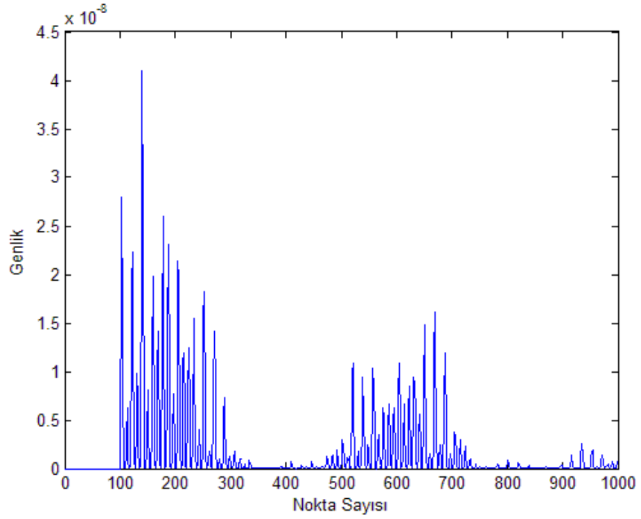
Şekil 2.3 : Tasarlanmış EM alıcısı ile alınmış işaretin kümülanı alınmış şekli
