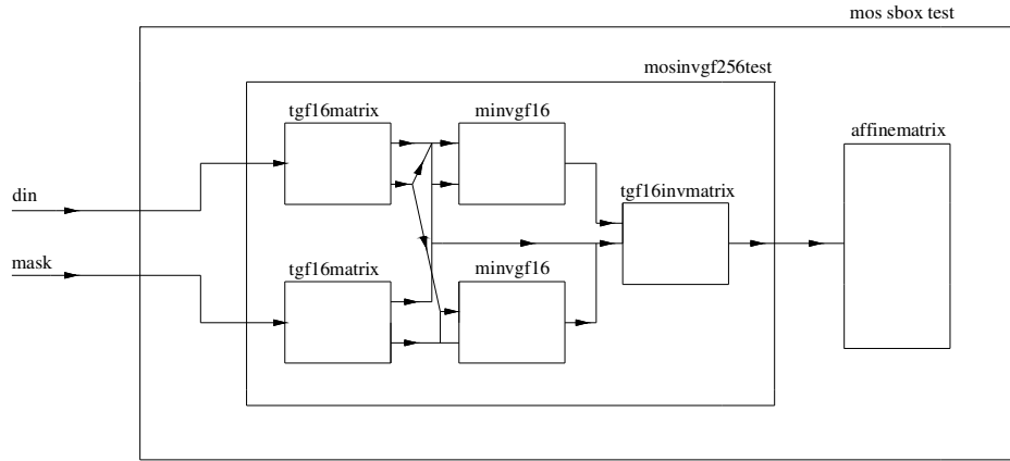
Şekil 3.8 : Tahmin değerleri için geçişleri sayılan kombinezonsal kısım
