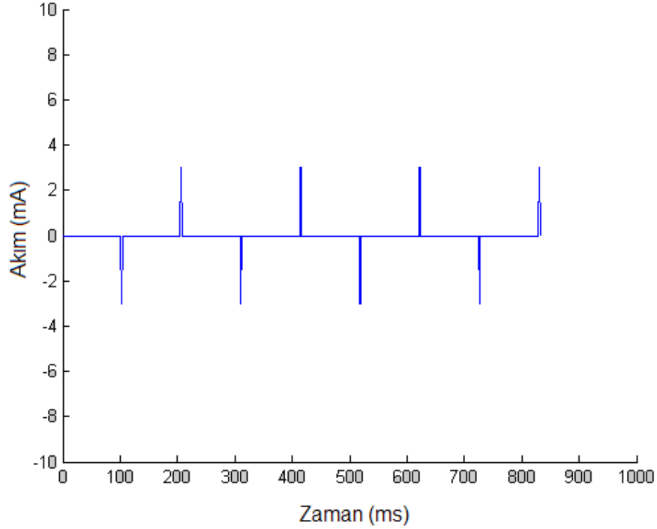
Şekil 4.5 : Manyetik alan alıcısı çıkışı
