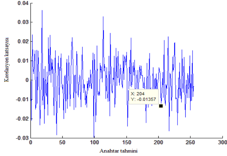
Şekil 6.6 : AES algoritmasının maskeli gerçekleştirilmesi için korelasyon sonucu
