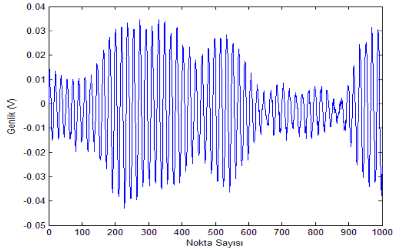
Şekil 6.3 : AES algoritmasının maskesiz gerçeklemesi için satır kaydırma işlemi kaydedici ölçümü
