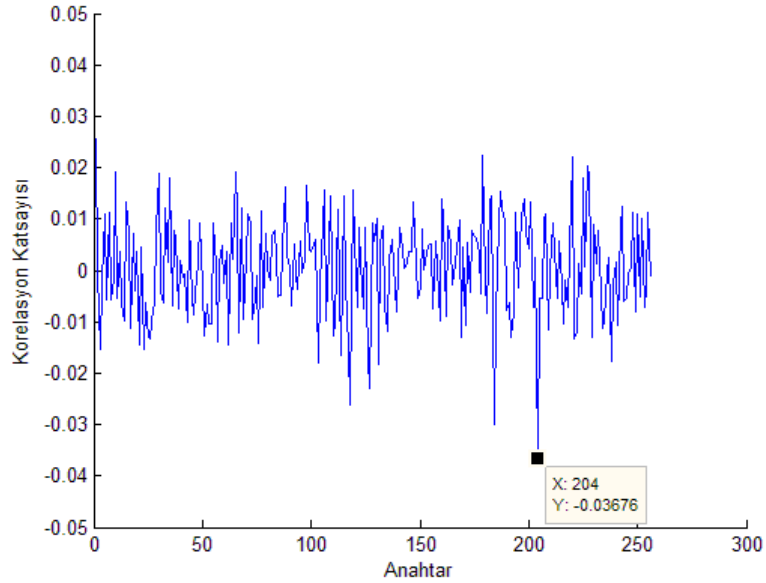
Şekil 6.4 : AES algoritmasının maskesiz gerçekleştirilmesi için korelasyon sonucu
