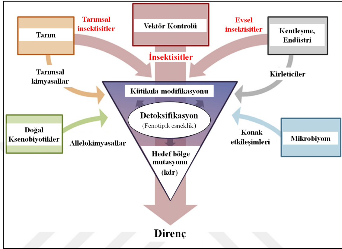
Şekil 5.1. Sivrisineklerde piretroit direncini etkileyen çevresel faktörlerin şematik gösterimi (Nkya vd. 2013)
