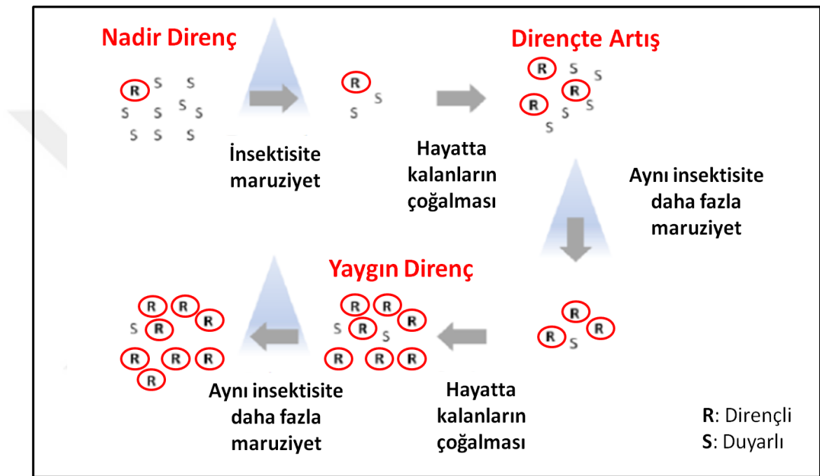
Şekil 2.8. Bir sivrisinek popülasyonunda insektisitlere direnç gelişimi ile ilgili olası senaryo (IRAC 2011)
