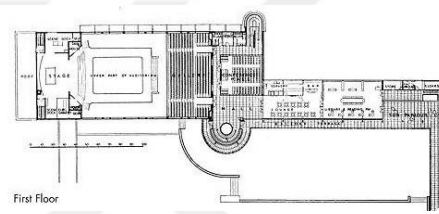
Resim 5.8. De La Warr Planı (Aslanoğlu, 2010)
