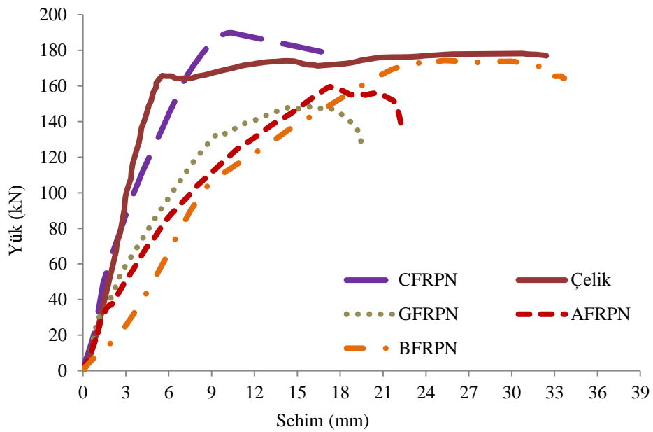
Şekil 4.85. Çelik ve nervürlü donatılı döşemelerin yük-sehim grafiği
