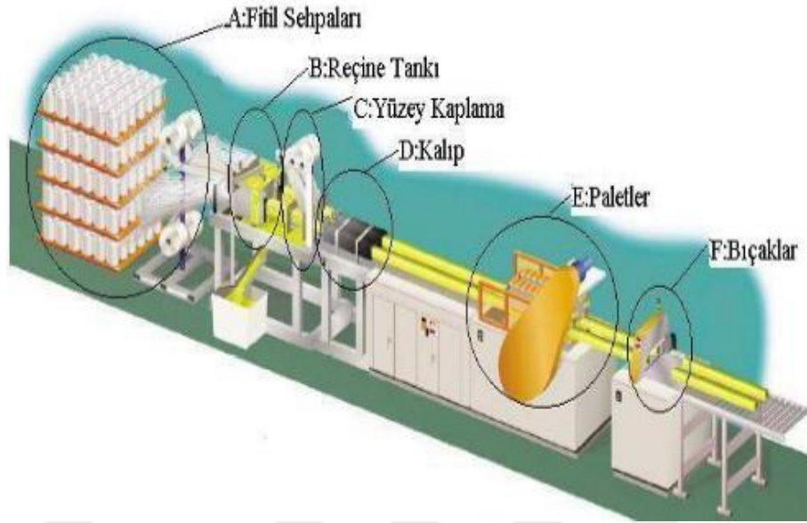
Şekil 3.1. Pultrüzyon yöntemi şeması [22].
