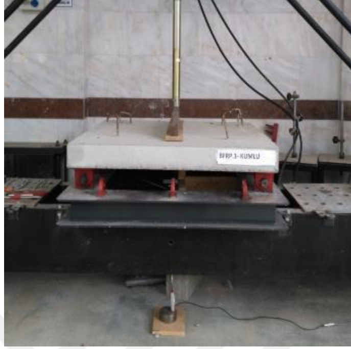
Şekil 4.39. BFRPK donatılı döşeme kırılma öncesi
