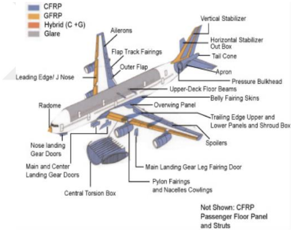
Şekil 2.9. Yolcu uçağı kısımlarında kullanılan FRP kompozitler [16].
