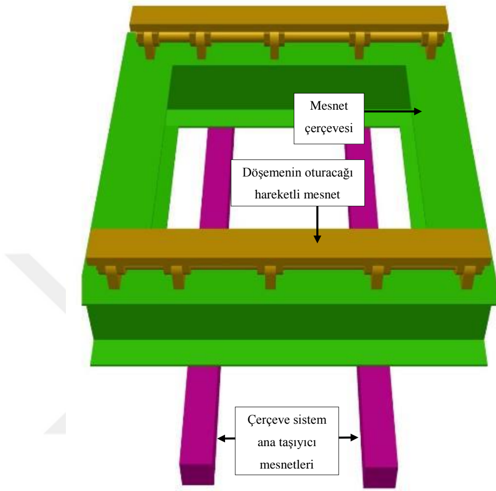
Şekil 4.31. Döşeme deneyi için hazırlanmış mesnet düzeneği
