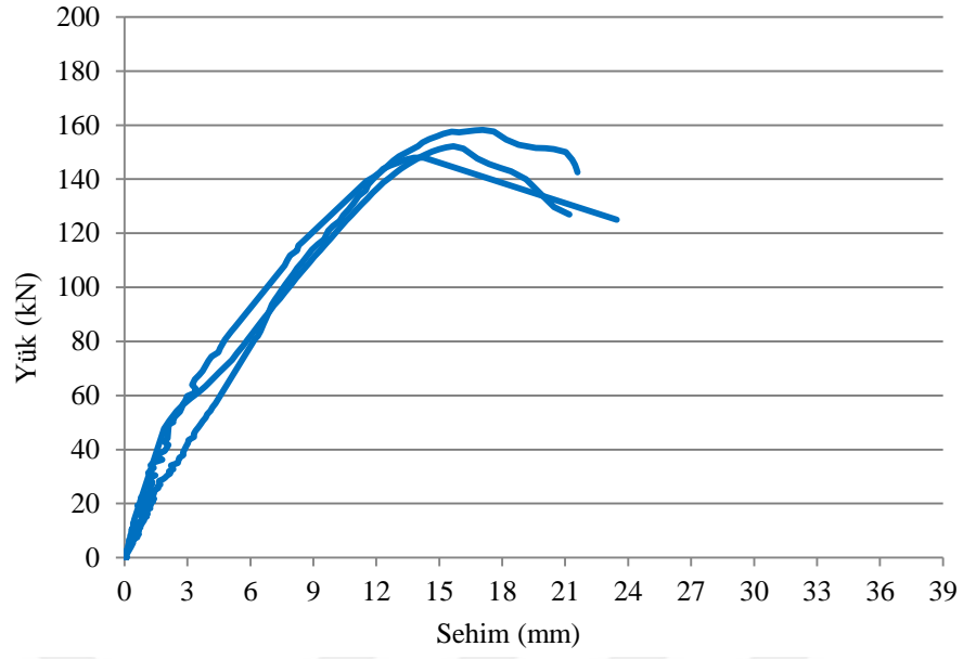
Şekil 4.54. AFRPK donatılı döşeme yük-sehim grafiği
