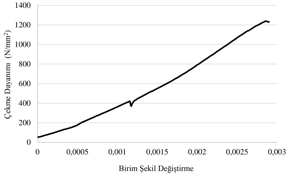
Şekil 4.47. AFRP donatı çekme dayanımı-birim şekil değıştirme grafiđi
