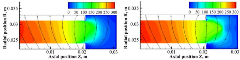
(d) Potential distribution (V)
