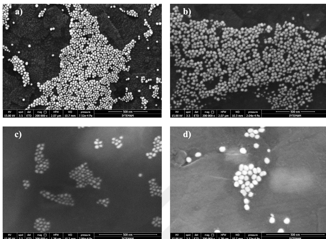
Figure 4.5. SEM images of conjugated AuNPs. a) 20 nm RGD/NLS-AuNP, b) 40 nm RGD/NLS-AuNP, c) 20 nm NLS-AuNP, d) 40 nm NLS-AuNP.
