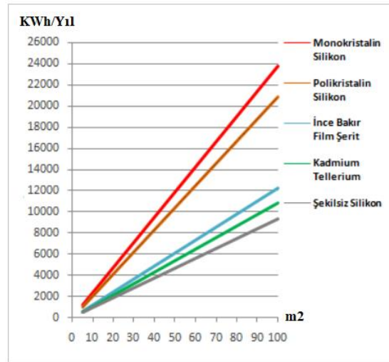
Şekil 5.10. BAYRAMIÇ PV Tipi-Alan-Üretilebilecek Enerji (KWh-Yıl) [3]
