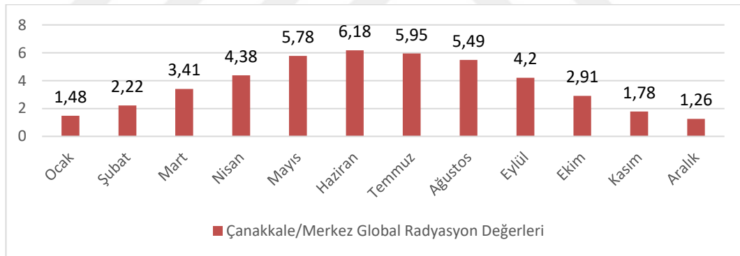
Şekil 5.2. Merkez global radyasyon değerleri (KWh/m 2 -gün) [3]
