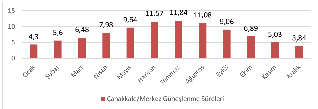
Şekil 5.3. Merkez güneşlenme süreleri (Saat) [3]
