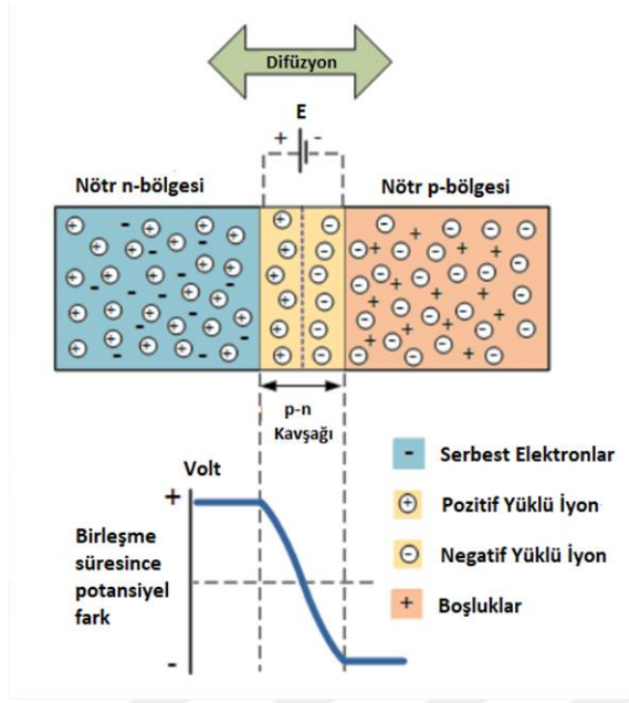
Şekil 2.3. p-n eklemnin çalışma ilkesi
