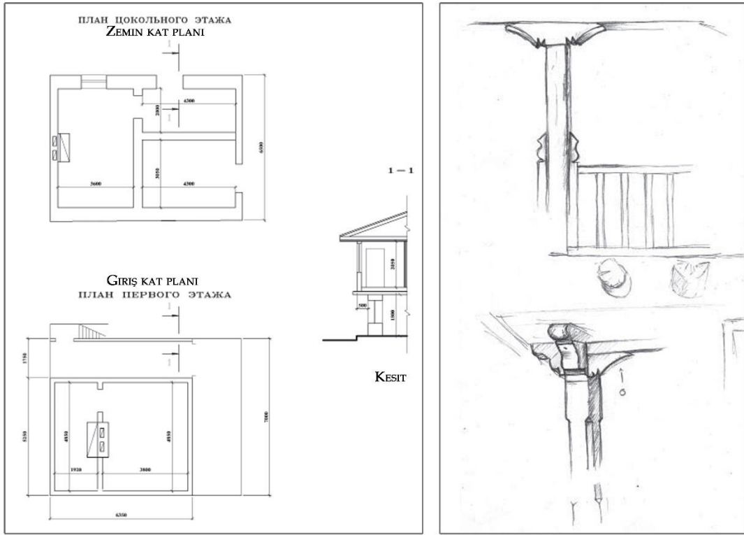
BÜYÜK ÖZENBAŞ KÖYÜNDE KERPIÇ EVİN KAT PLANI. HAZIRLAYAN: R. SARANAEV
