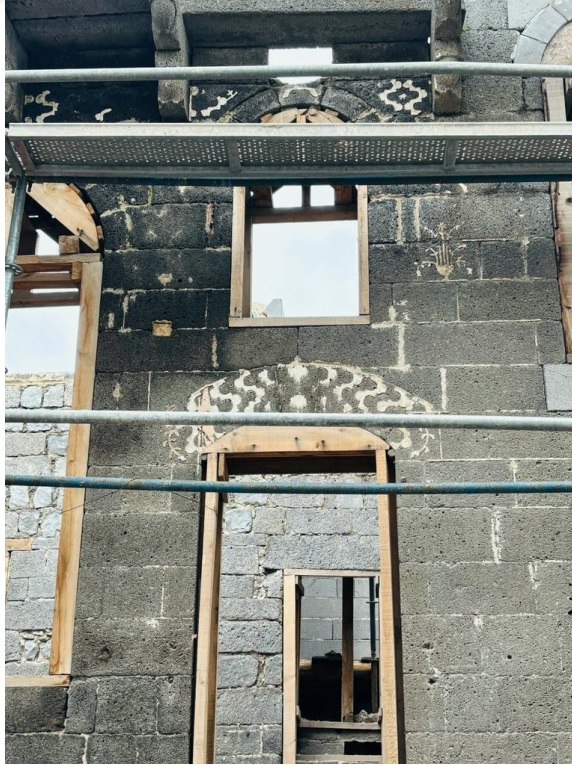
Fotoğraf 344. Konut 33'ün Güney Cephesindeki Oda Kapısının Detayı
