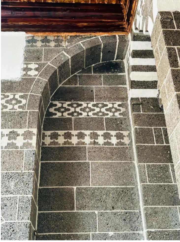
Fotoğraf 206. Konut 22'nin Güney Cephesindeki Eyvanın S ve C Kıvrımlı ve Şemse Motifli Süsleme Detayı
