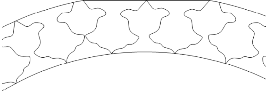
Fotoğraf 358. Konut 34'ün Batı Cephesindeki Sivri Kemerli Nişin Altındaki Basık Kemerli Niş Detay
