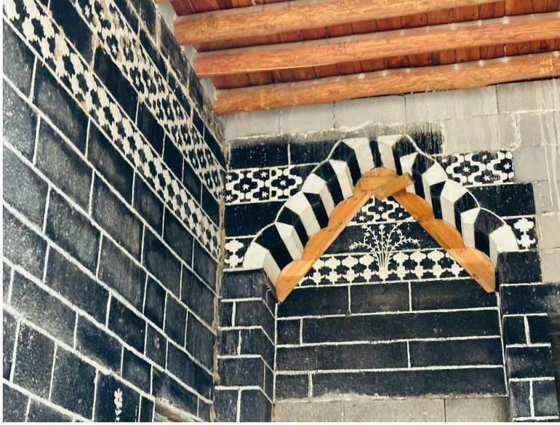
Fotoğraf 65. Konut 9'un Zemin Katta Doğu Cephesindeki Eyvan ve Niş Detayı
