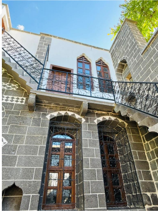
Fotoğraf 168. Konut 20'nin Güney Cephesinde Yapının Doğusunda Yer Alan Odanın Basık Kemerli Pencere Nişleri
