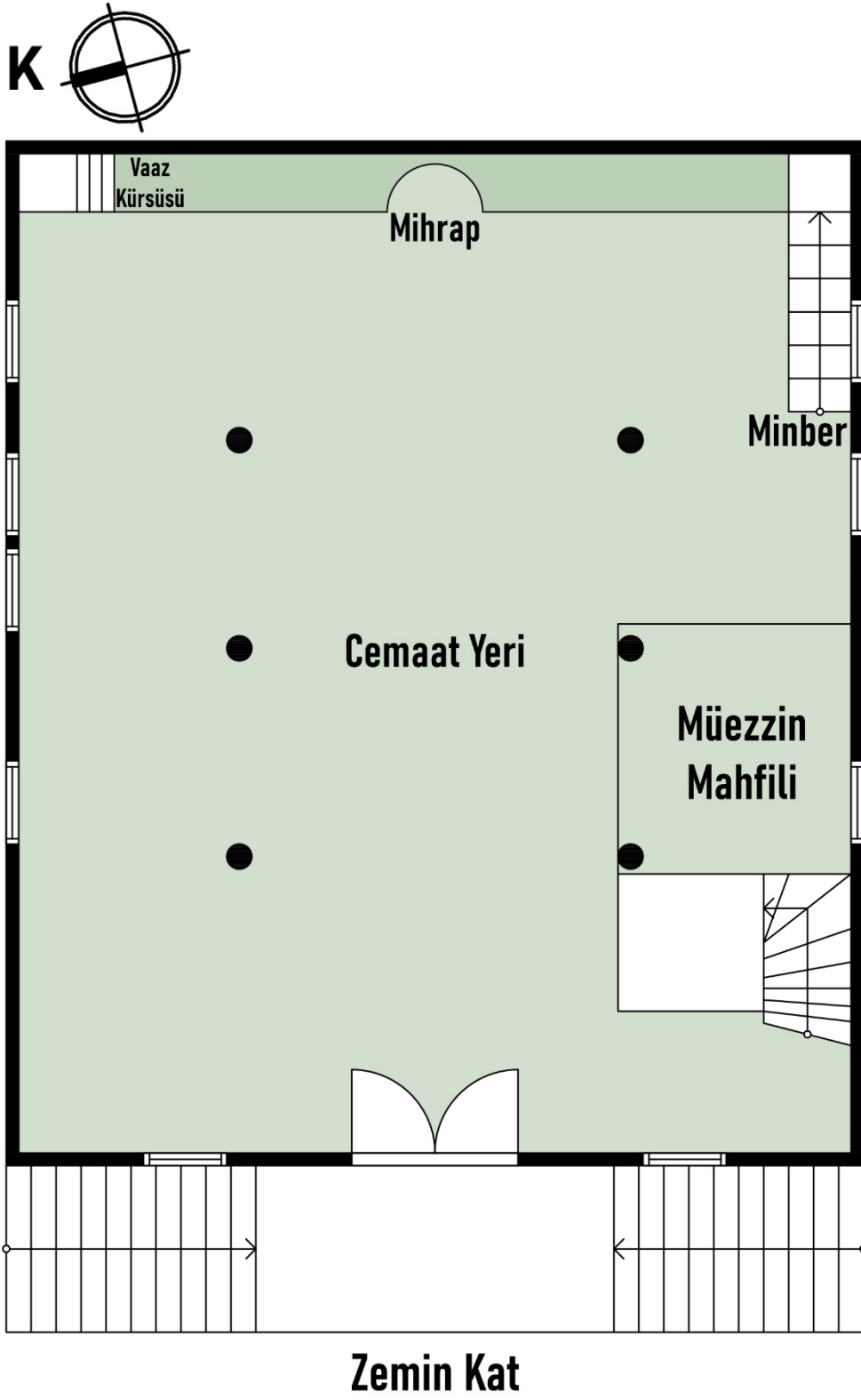
Şekil 4.7. Nüzhetiye Köyü Tarihi Ahşap Camii Zemin Kat Planı Krokisi
