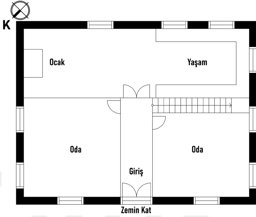
Şekil 4.21. Nüzhetiye Köyü'nde Geleneksel Yapım Tekniğiyle Yapılmış Bir Konuta Ait Zemin Kat Planı Krokisi
