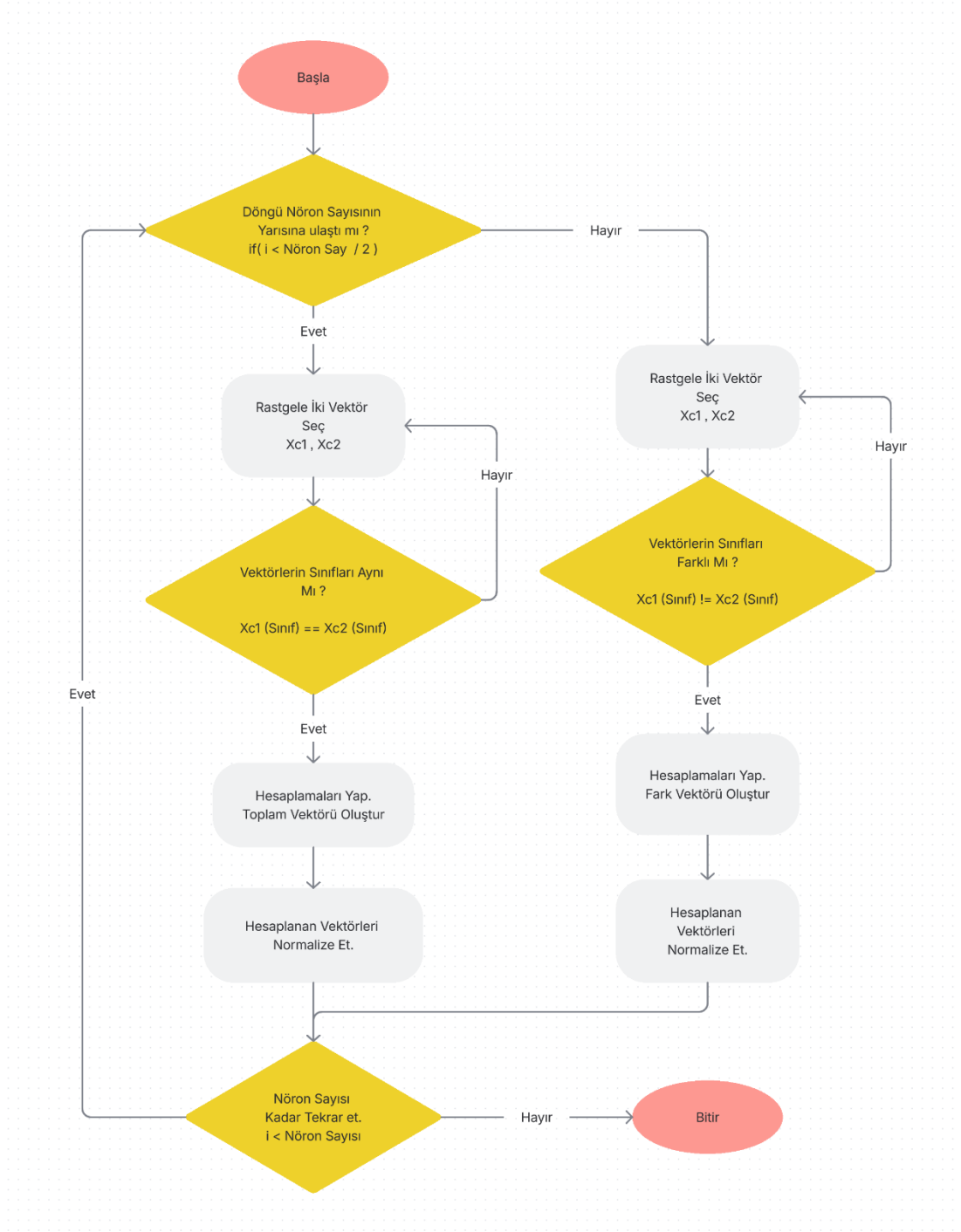
Şekil 2.12 M-CNN ağındaki tam bağlı katman ağırlıklarının belirleme işlemleri akış şeması.
