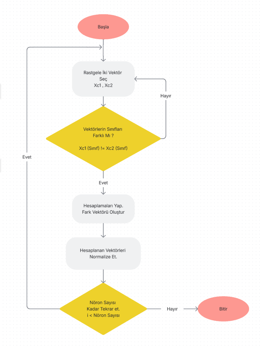
Şekil 2.8 D-CNN ağındaki tam bağlı katman ağırlıkları ve eşik parametreleri belirleme işlemleri akış şeması.
