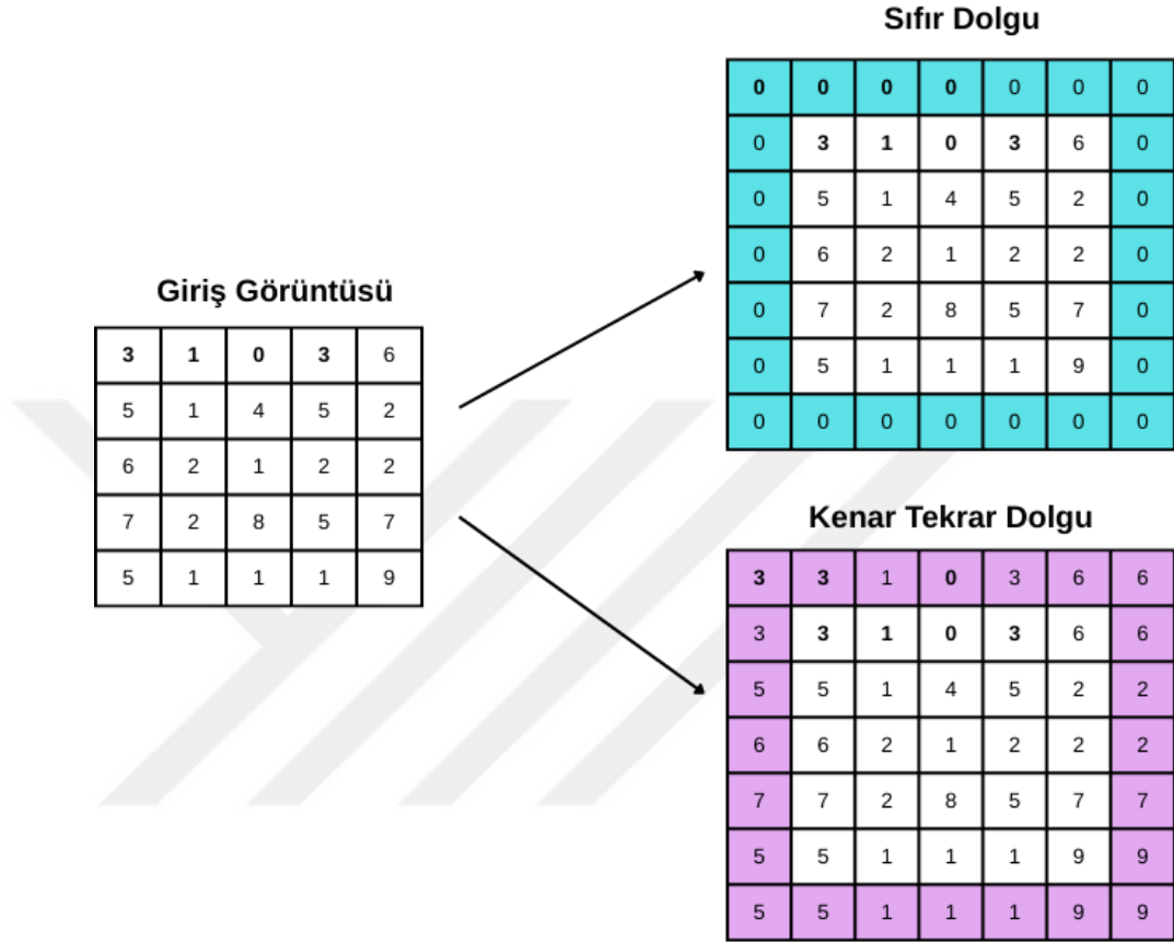
Şekil 2.4 Sıfır dolgu ve kenar tekrar dolgu örnekleri.
