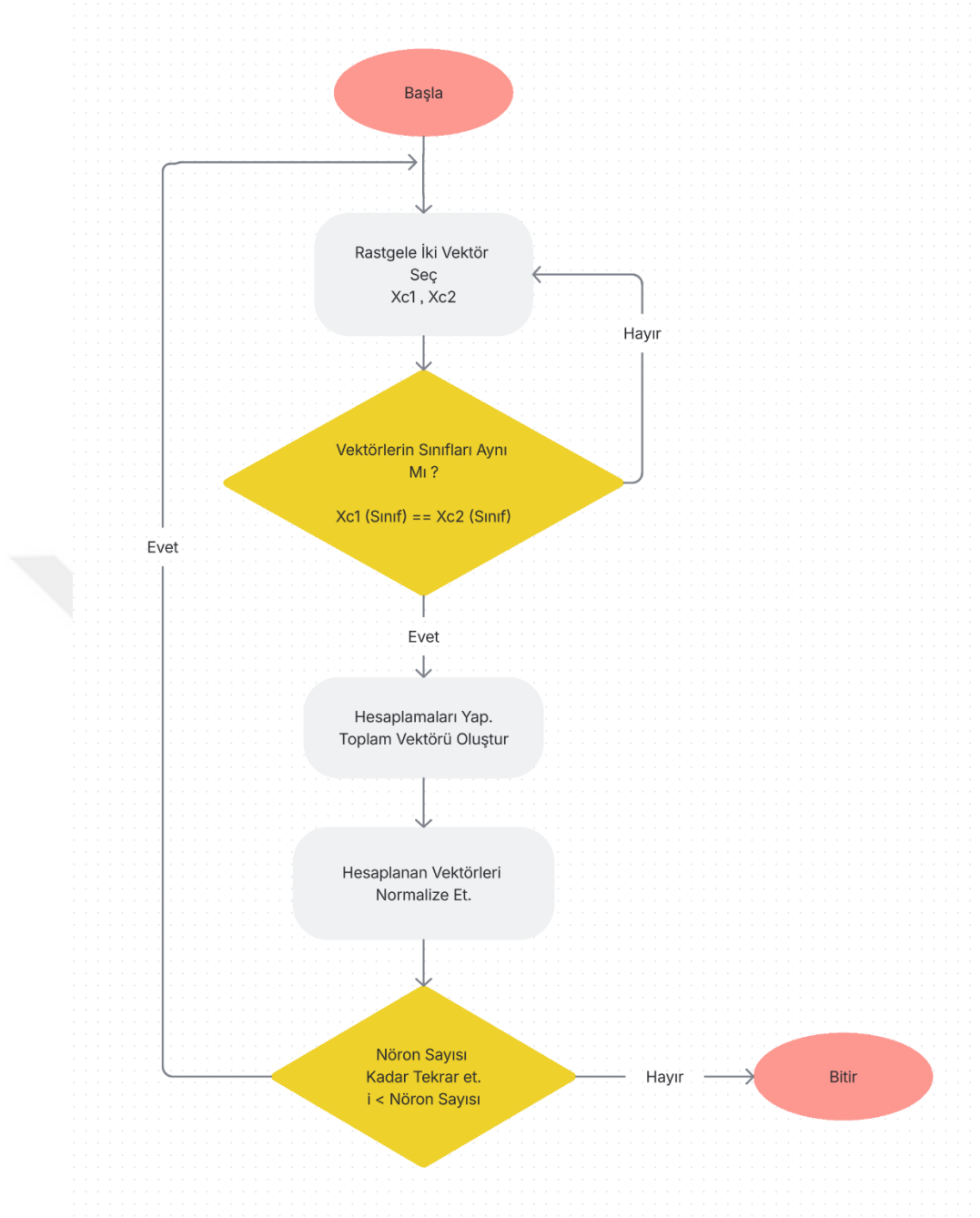
Şekil 2.10 S-CNN ağındaki tam bağlı katman ağırlıklarının belirleme işlemleri akış şeması.
