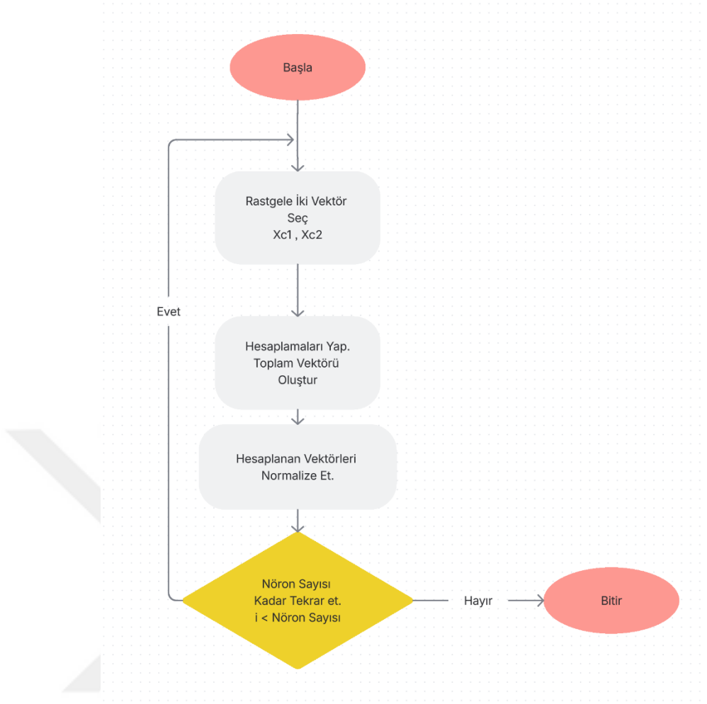
Şekil 2.11 RS-CNN akış şeması.
