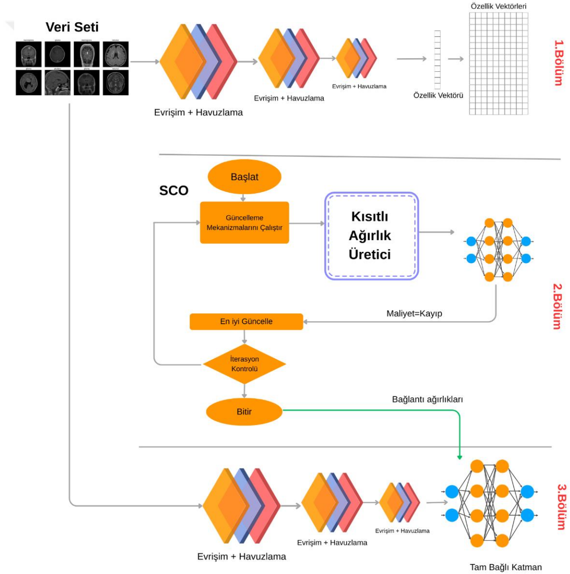
Şekil 2.15 OptiConNet modelinin mimarisi.
